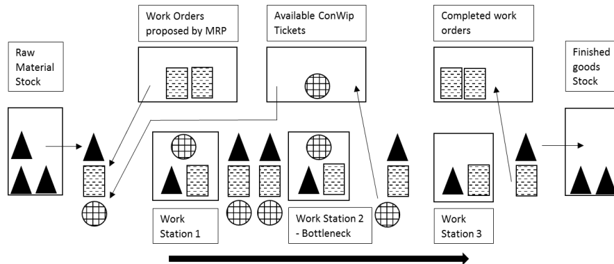
Figure 12. ConWip raccourci pour prendre en compte le goulet d'étranglement.
