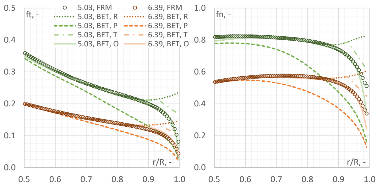
Fig. 5 Distribution radiale de coefficients de couple (gauche) et force de trainee (droite) pour TSR 5,03 (vert) et 6,39 (rouge) – resultats numeriques FRM et CFD-BET pour des corrections de la perte d'extrémité de la pale differentes : sans correction (R), modele de Prandtl (P [10]), Takahashi (T [11]), propre (O)
