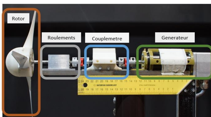
Fig. 1 Banc d'essais T1 (sans boîtier); rotor placée dans la configuration sous le vent (l'écoulement vers la gauche)
