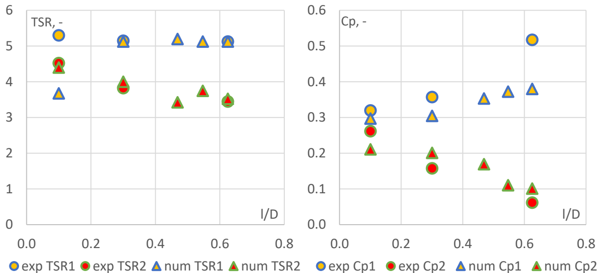
Fig. 7 TSR (gauche) et C_p (droite) de deux rotors achevées pour coefficient de puissance C_p totale de système est maximal, en fonction de distance entre rotors I/D : expérience vs. simulation CFD-BET
