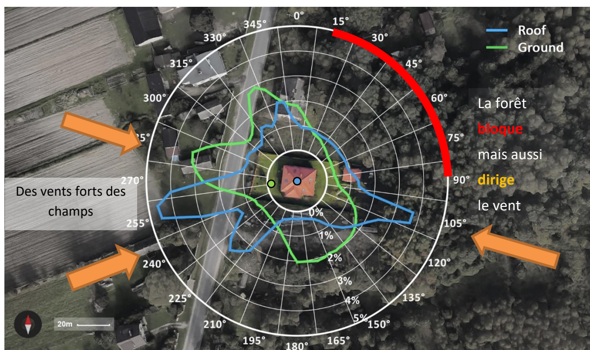
Fig. 10 La rose des vents préparée pour le site étudié: zone suburbaine (Brójce, près de Łódź); mesures à 2 hauteurs (repérées par des points): 2,25 m (« Ground », vert) et 10 m (« Roof », bleu)
