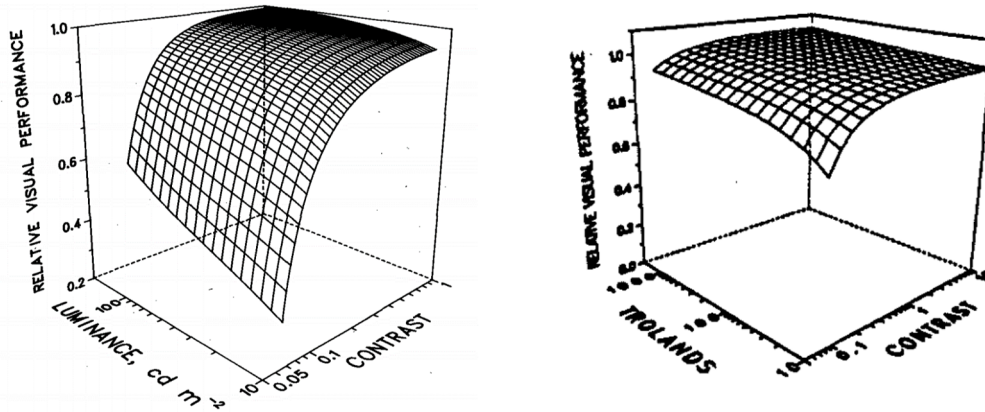
FIGURE 36 – Exemple de performance visuelle pour deux tailles de cible différentes Images tirées de [Rea & Ouellette, 1991]
