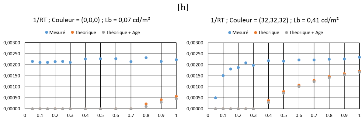
FIGURE 72 – Performance théorique et réelle pour l’expérimentation de détection des stimuli contrastés, conditions 0 et 32.
