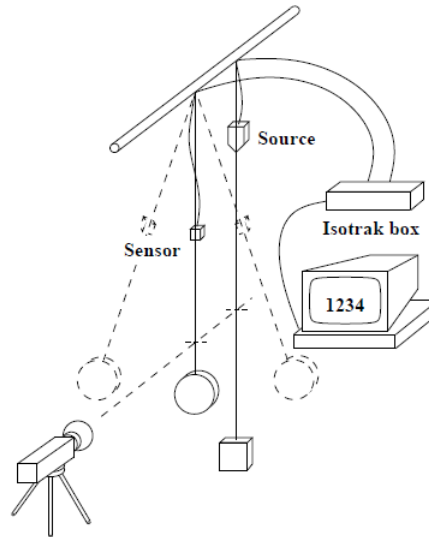
FIGURE 75 – Méthode du pendule pour le calcul de la latence. Image tirée de [Liang et al. , 1991]
