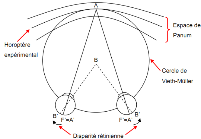
FIGURE 9 – Horoptères théorique et empirique, Aire de Panum et disparités rétinienne. Image tirée de [Neveu, 2012].
