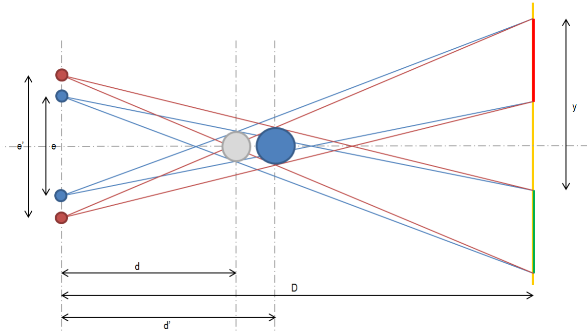
FIGURE 20 – Schématisation de la différence de profondeur stéréoscopique perçue en fonction de la distance interoculaire
