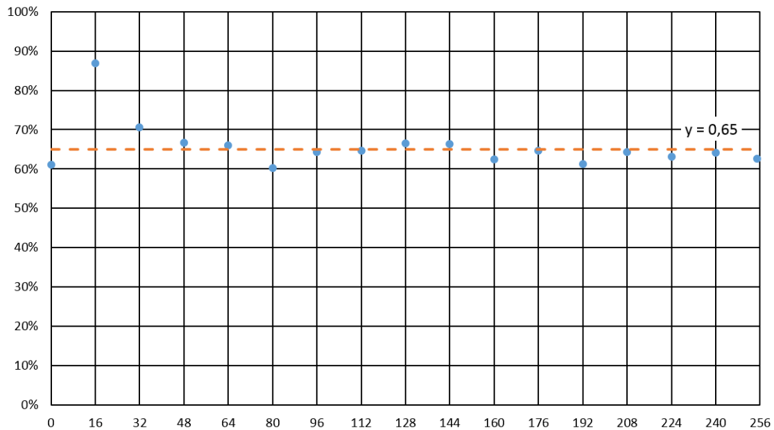
FIGURE 68 – Pourcentage d'absorption en fonction du niveau de gris affiché.
