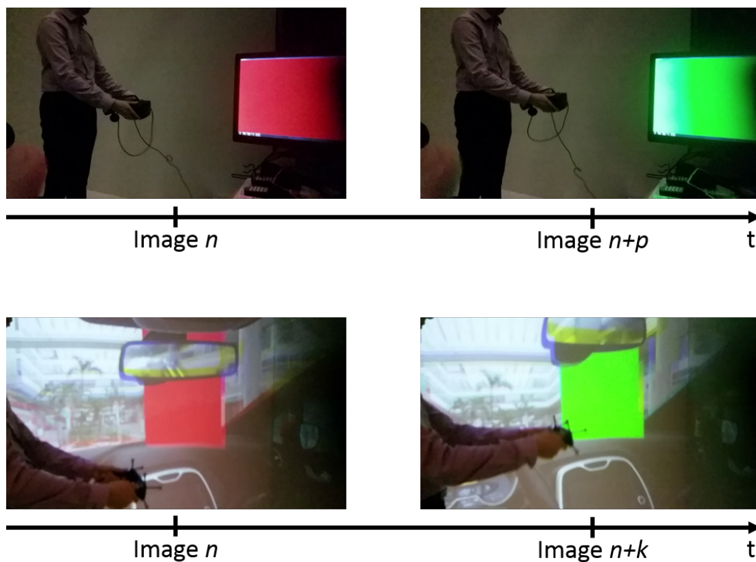
FIGURE 81 – Technique de mesure de la latence.
