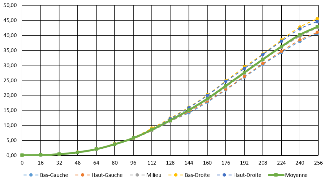
FIGURE 61 – Evolution de la luminance en fonction du niveau de gris sur les cinq points de mesure et leur moyenne.
