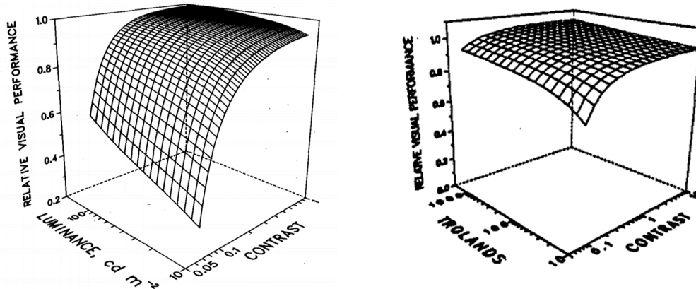
FIGURE 36 – Exemple de performance visuelle pour deux tailles de cible différentes Images tirées de [Rea & Ouellette, 1991]
