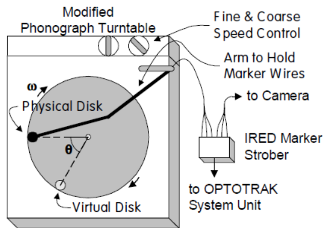
FIGURE 76 – Méthode de la table tournante pour le calcul de la latence. Image tirée de [Swindells et al. , 2000]. La position du disque physique est appliqué au disque dans la scène virtuelle. Les deux images sont superposées et on mesure l'écart angulaire entre les deux. A partir de la vitesse de rotation on peut remonter à la latence.
