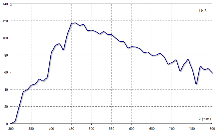
FIGURE 17 – Spectre de l'illuminant D65 (CIE)
