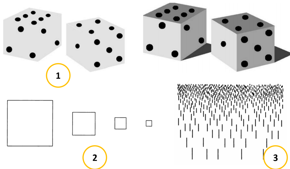
FIGURE 19 – Illustration d'indices de profondeur Ombres (1, image tirée de [ANSES, 2014]), taille et gradient de profondeur (2 et 3, images tirées de [Glassner, 1995]).
