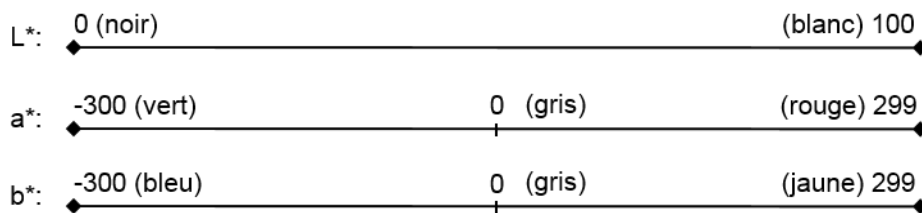
FIGURE 14 – Composantes de l'espace CIELAB
