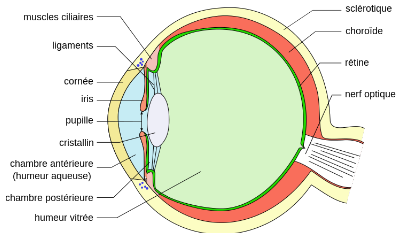
FIGURE 4 – Structure de l'œil
