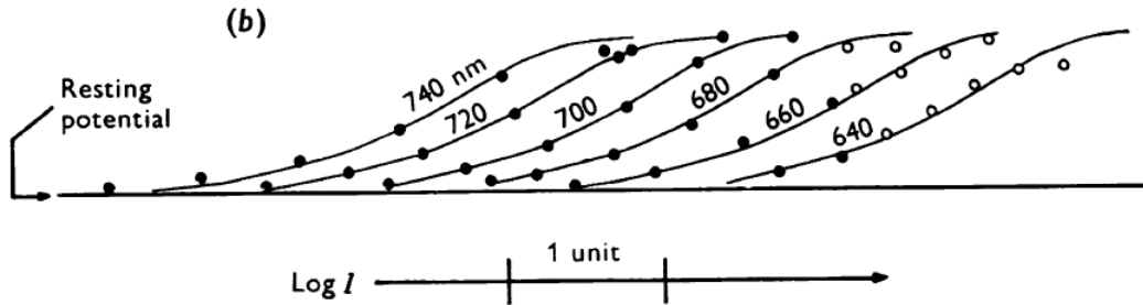
FIGURE 58 – Illustration de l'effet de compression. Image tirée de [Naka & Rushton, 1966]
