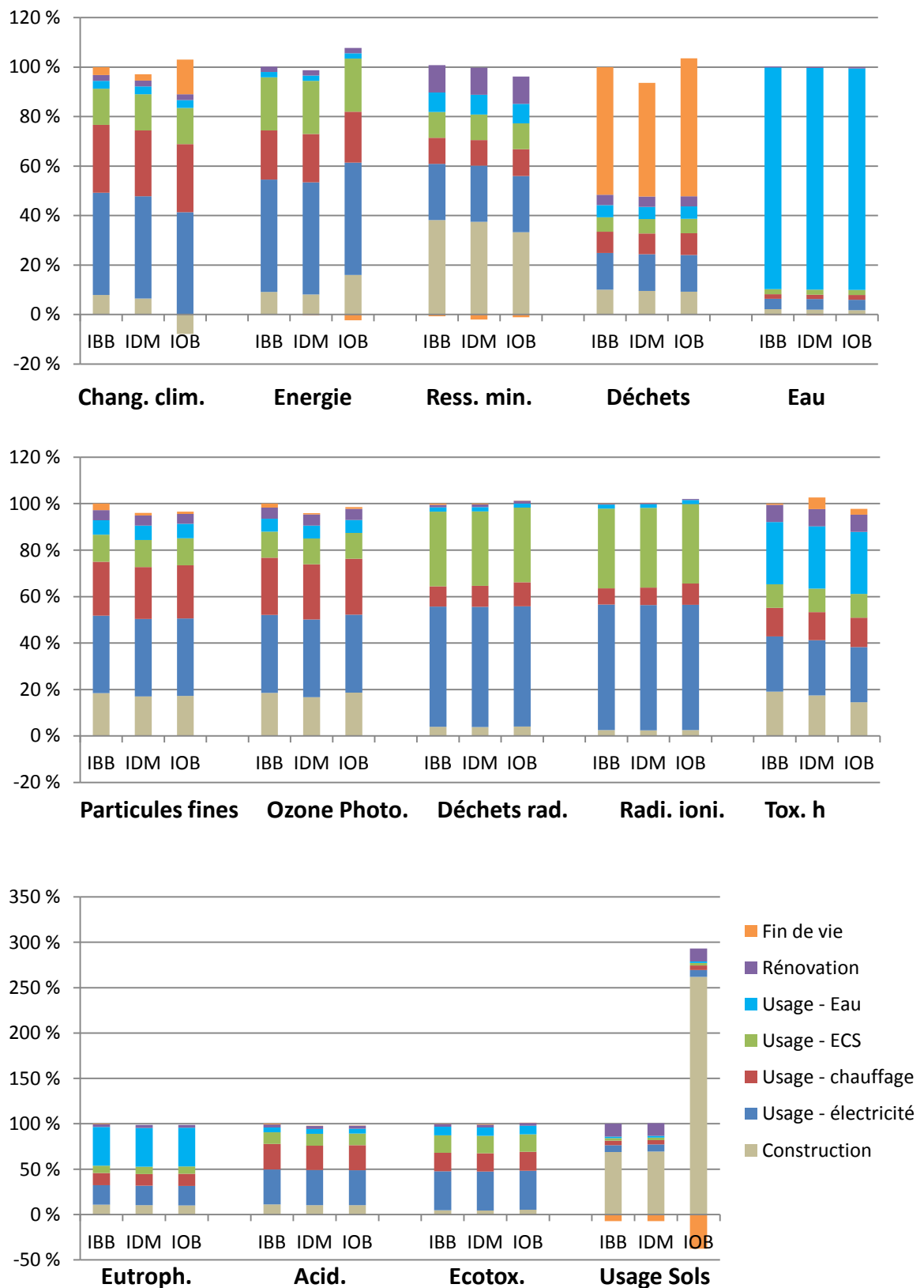
Figure 2-10. Comparaison des variantes constructives (la variante IBB sert de référence, et les impacts des autres variantes sont exprimés relativement à cette variante)
