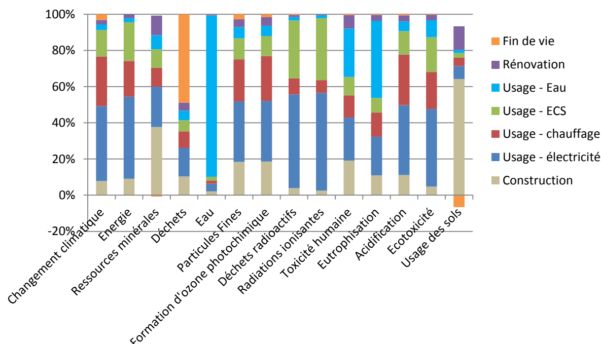
Figure 2-8. Analyse de contribution pour la maison IBB, énergie électricité
