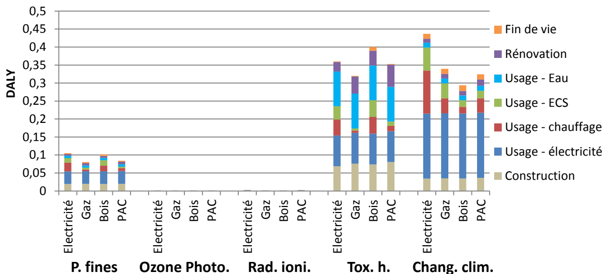
Figure J-33. Analyse de contribution pour l'aire de protection « santé humaine », comparaison de variantes énergétiques
