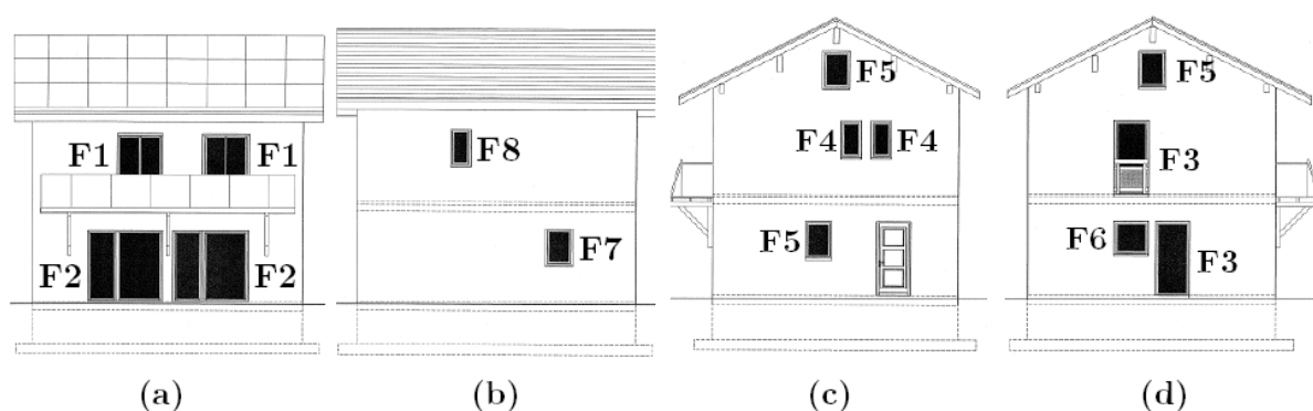
Figure M-56. Emplacement des fenêtres sur les façades (a) sud, (b) nord, (c) est et (d) ouest des maisons INCAS
