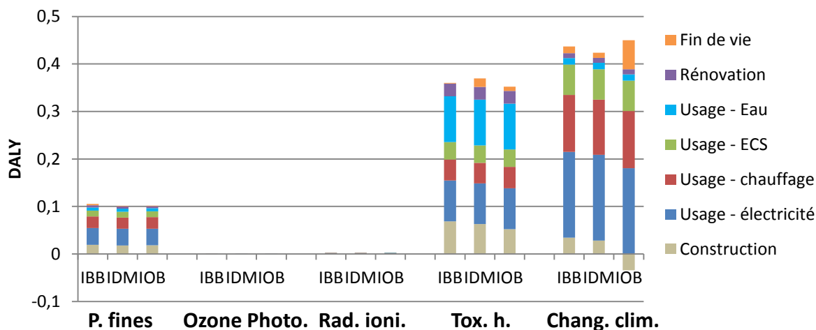
Figure J-32. Analyse de contribution pour l'aire de protection « santé humaine », comparaison de variantes constructives
