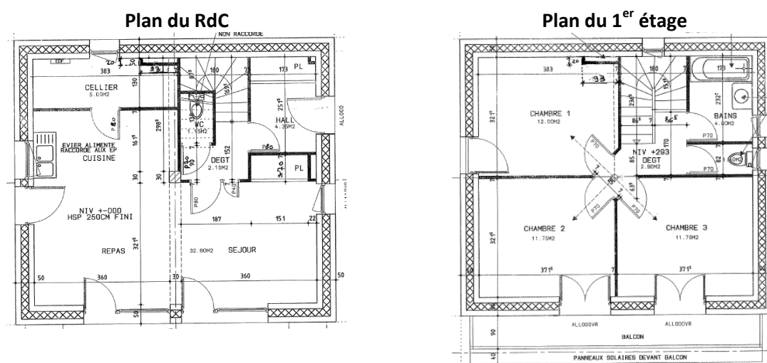
Figure 2-5. Plans des niveaux habitables de la maison IDM
