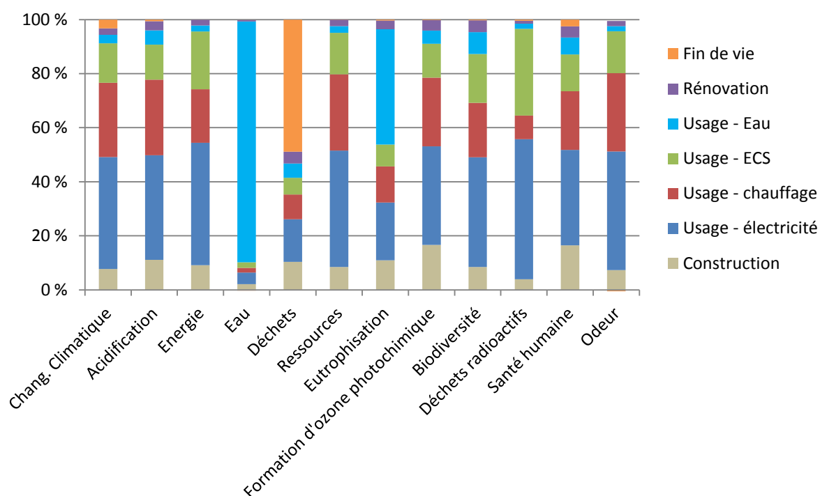
Figure J-18. Analyse de contribution pour la maison IBB, énergie électricité, mix marginal dérivé pour les usages d'électricité, mix marginal annuel pour la contextualisation des matériaux, et fins de vie précisées, avec la base v3.2
