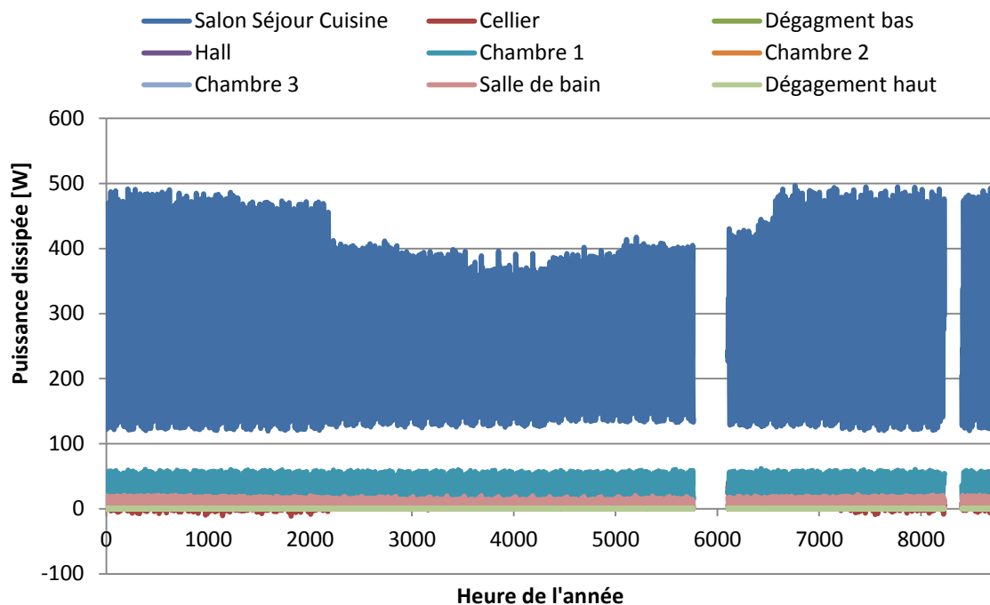
Figure J-8. Profil annuel moyen de puissance dissipée par les appareils électriques
