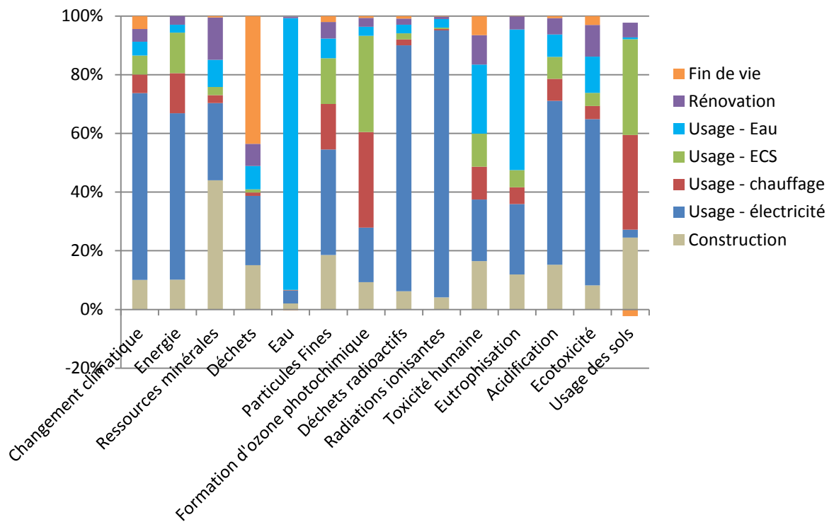
Figure J-26. Analyse de contribution pour la maison IDM, énergie bois
