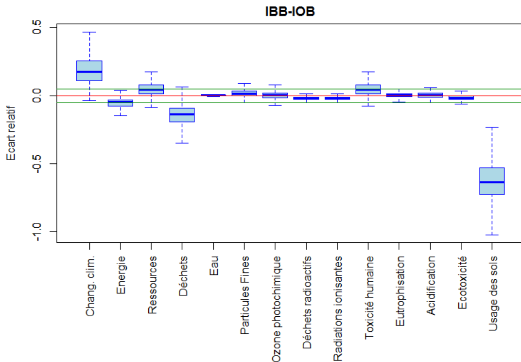
Figure 4-30. Distributions des écarts relatifs sur la comparaison de variante IBB-IOB, sans amélioration de la caractérisation des incertitudes
