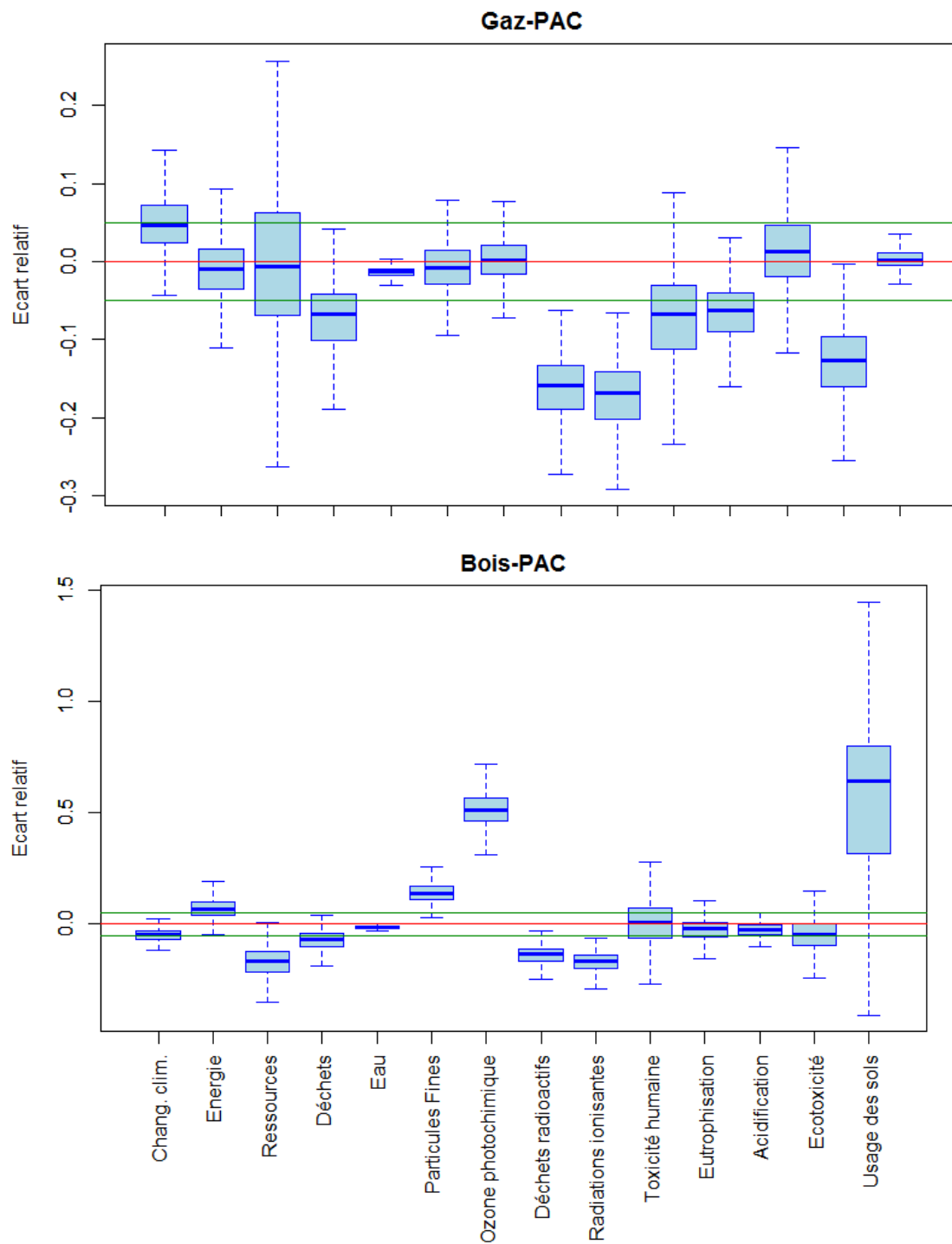
Figure N-78. Écart relatif entre les valeurs d'impact pour toutes les paires de variantes énergétiques
