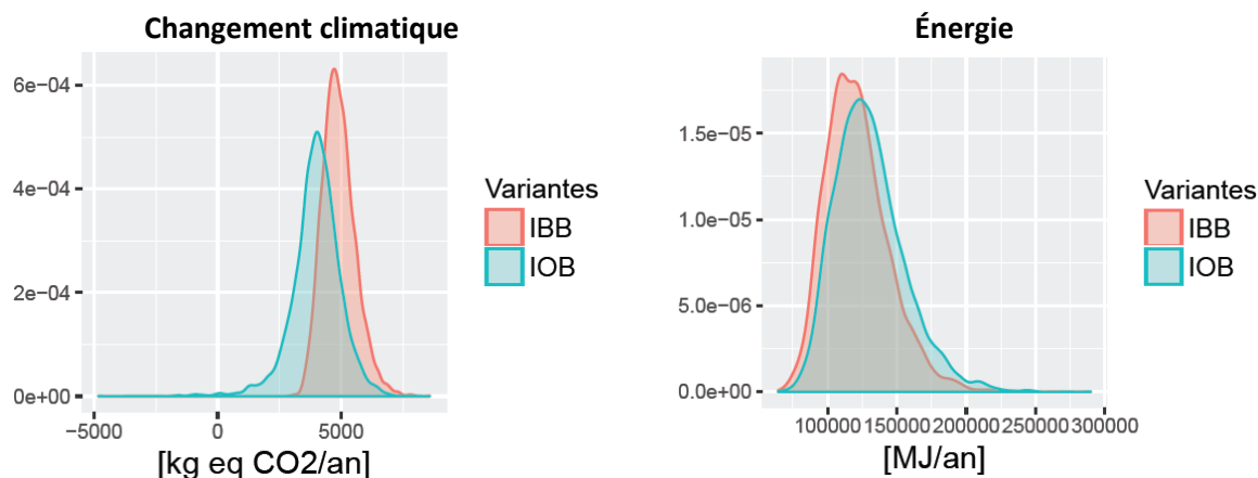
Figure 4-10. Distributions de probabilité en sortie pour les variantes IBB et IOB après avoir précisé les incertitudes sur les facteurs les plus influents
