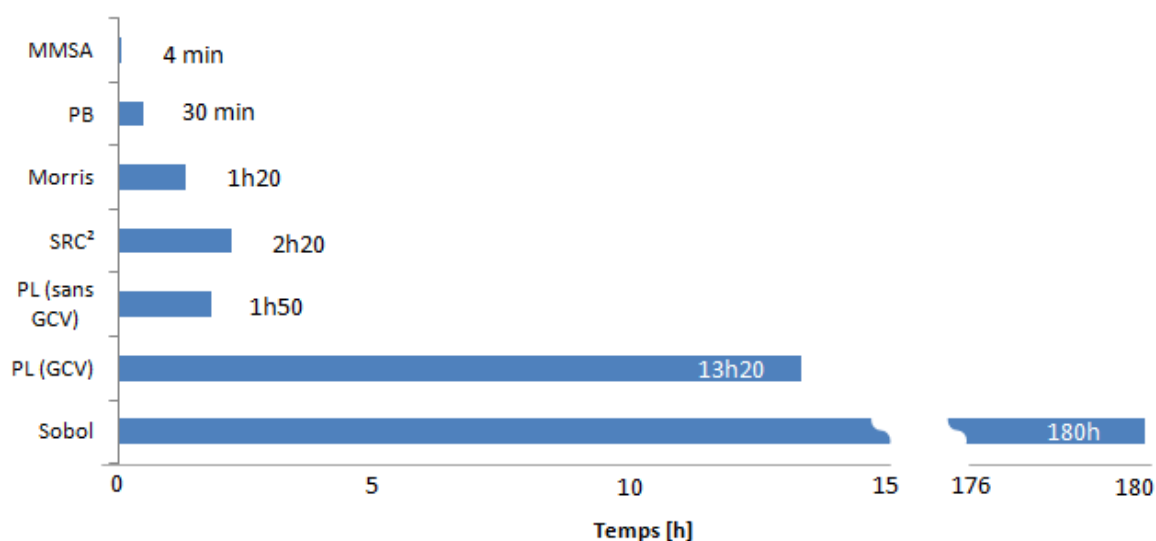
Figure 3-10. Comparaison des temps de calcul des six méthodes d'AS
