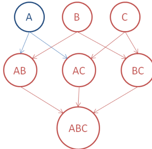
Figure E-5. Indice de sensibilité de premier ordre du facteur A pour un modèle à trois facteurs, issu de Faivre et al. (2013)
