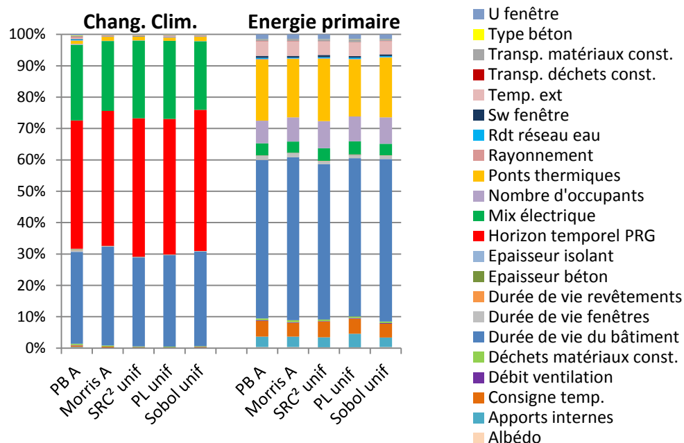
Figure 3-14. Comparaison de l'influence relative des facteurs incertains pour les méthodes adaptées
