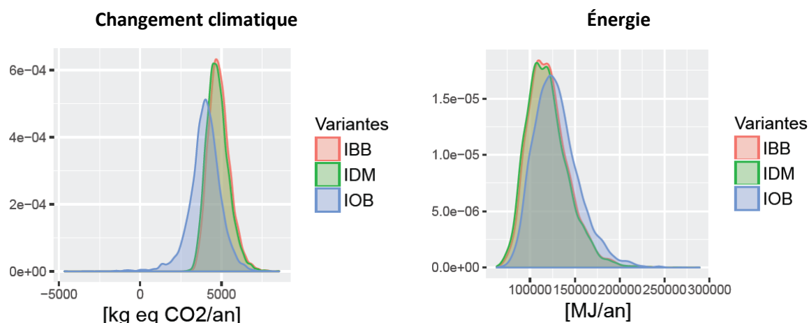
Figure 4-17. Distributions de probabilité en sortie pour les variantes IBB, IOB et IDM
