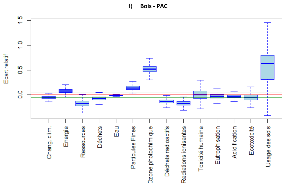
Figure 4-32. Écart relatif entre les valeurs d'impact pour toutes les paires de variantes énergétiques pour l'ensemble des occupations avant amélioration de la caractérisation des incertitudes sur les facteurs
