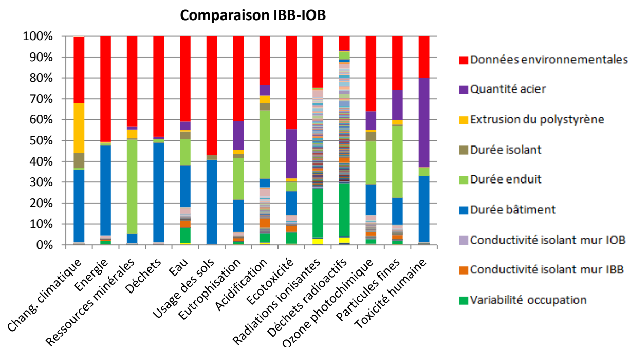
Figure 4-8. Criblage de Morris sur la différence entre les valeurs d'impact des variantes IBB et IOB
