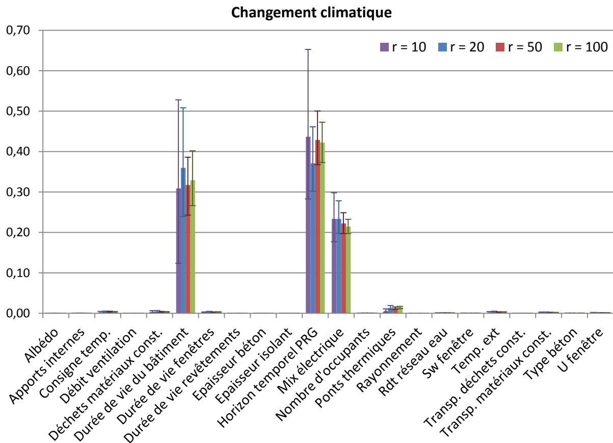
Figure L-51. Intervalles de confiance à 95 % calculés par bootstrap, pour Morris-A
