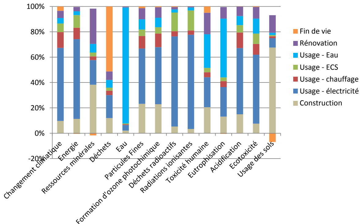
Figure J-27. Analyse de contribution pour la maison IDM, énergie électricité, PAC
