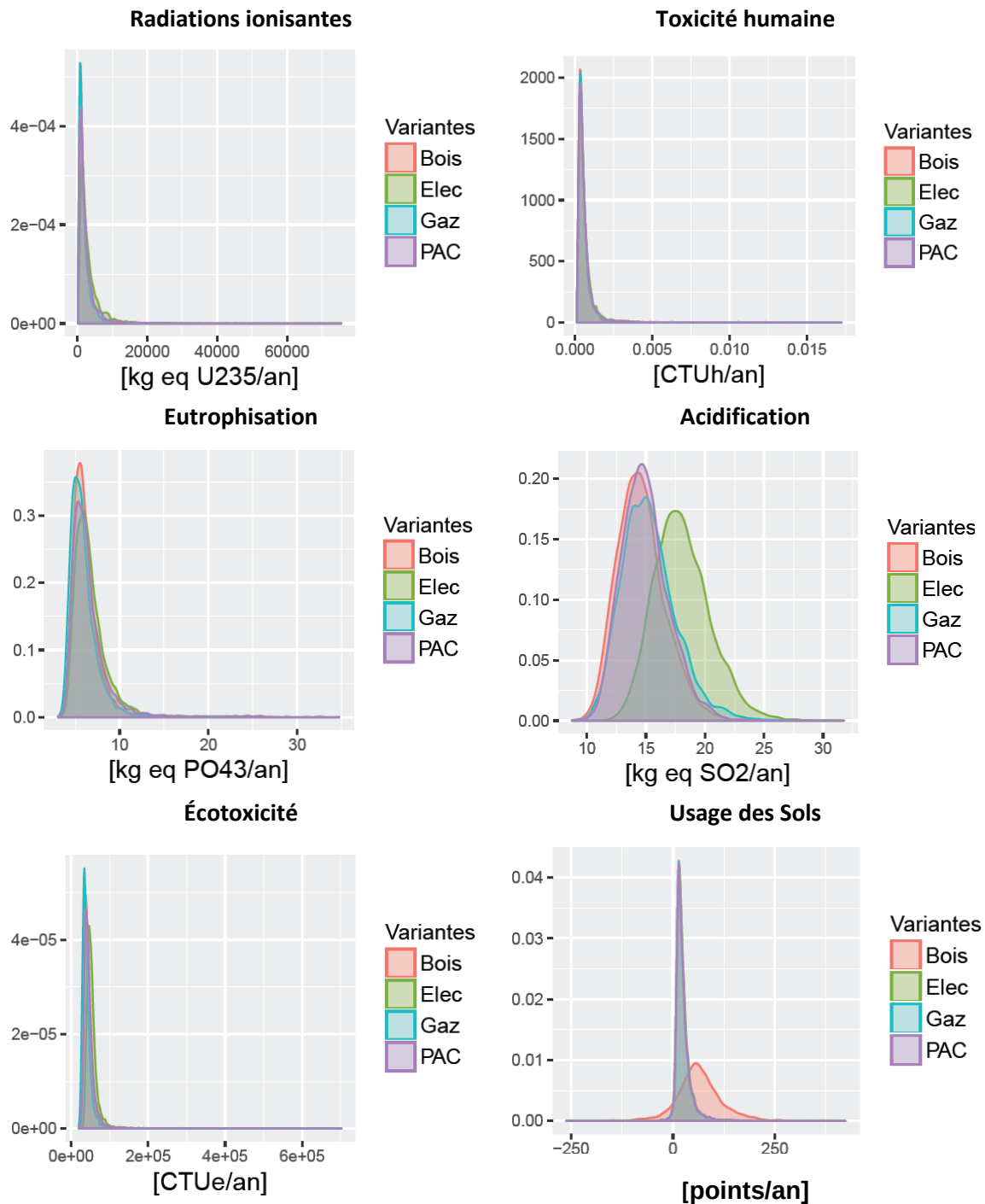
Figure N-76. Distributions de probabilité en sortie pour les variantes IBB et IOB pour tous les indicateurs
