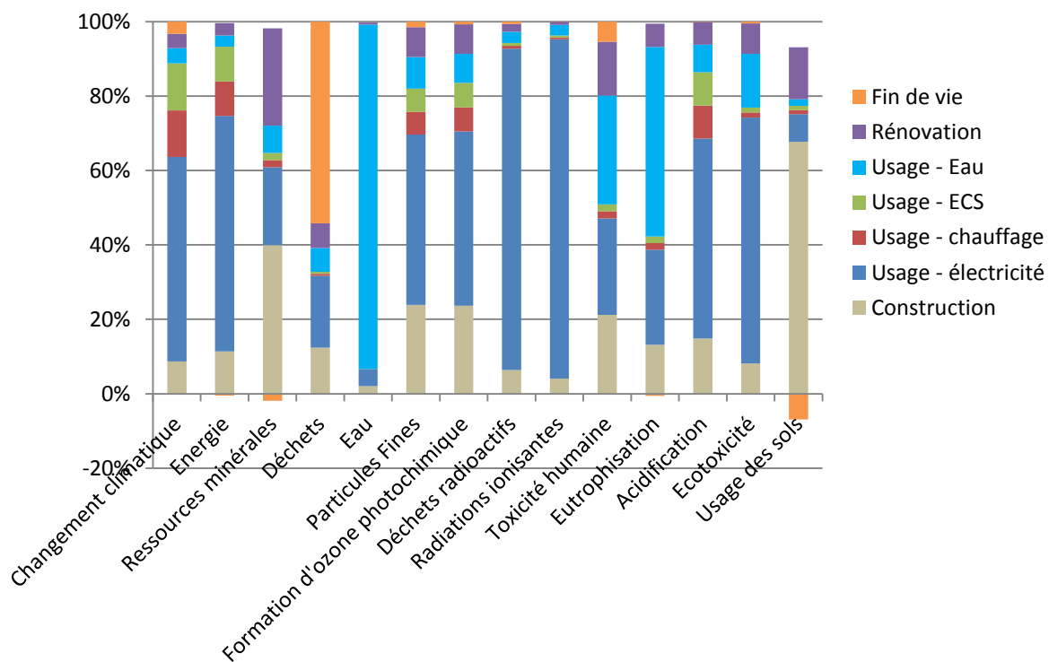
Figure J-25. Analyse de contribution pour la maison IDM, énergie gaz
