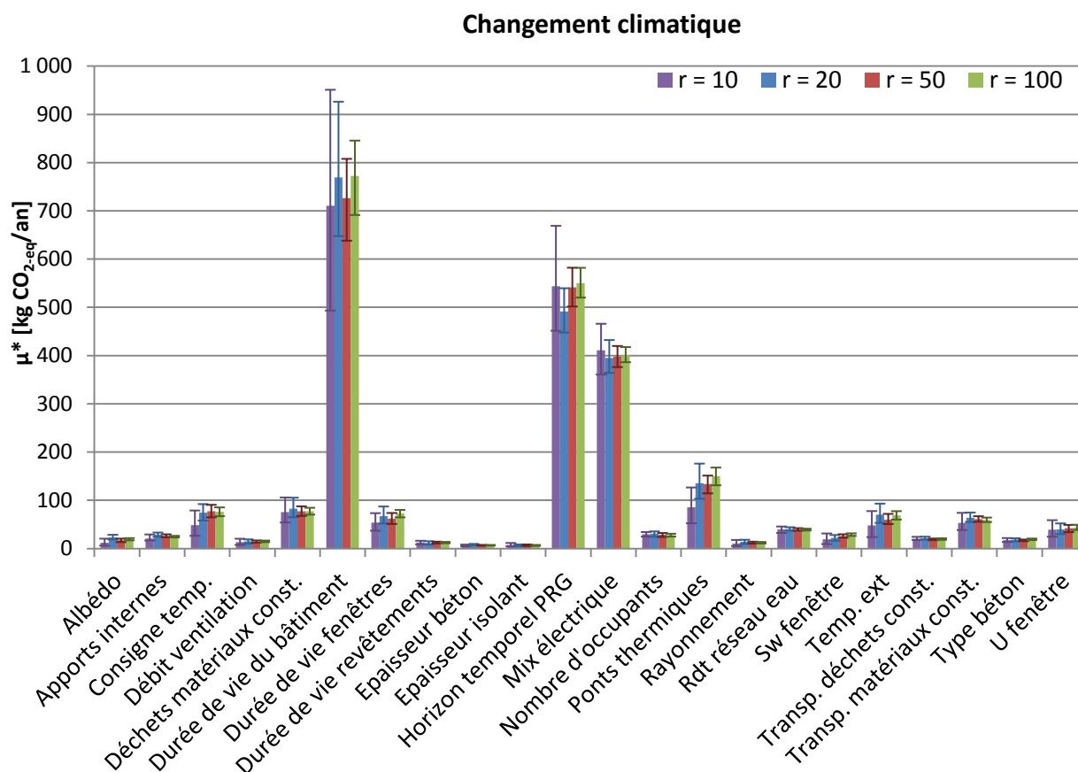
Figure L-39. Intervalles de confiance à 95 % calculés par bootstrap sur \mu^* pour l'indicateur de changement climatique
