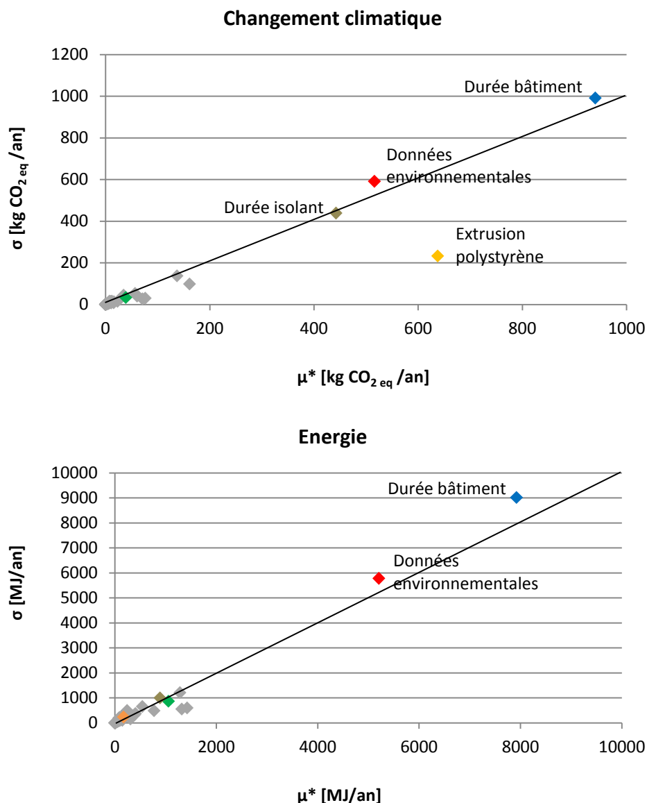
Figure N-67. Graphiques de Morris pour la comparaison de variante IBB-IOB
