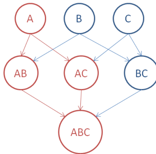
Figure E-6. Indice de sensibilité total du facteur A pour un modèle à trois facteurs, issu de Faivre et al. (2013)
