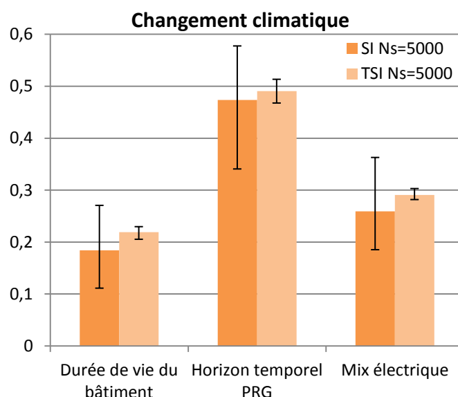
Figure 3-7. Intervalles de confiance à 95 % pour les indices de sensibilité de premier ordre (SI) et totaux (TSI) pour l'indicateur de changement climatique
