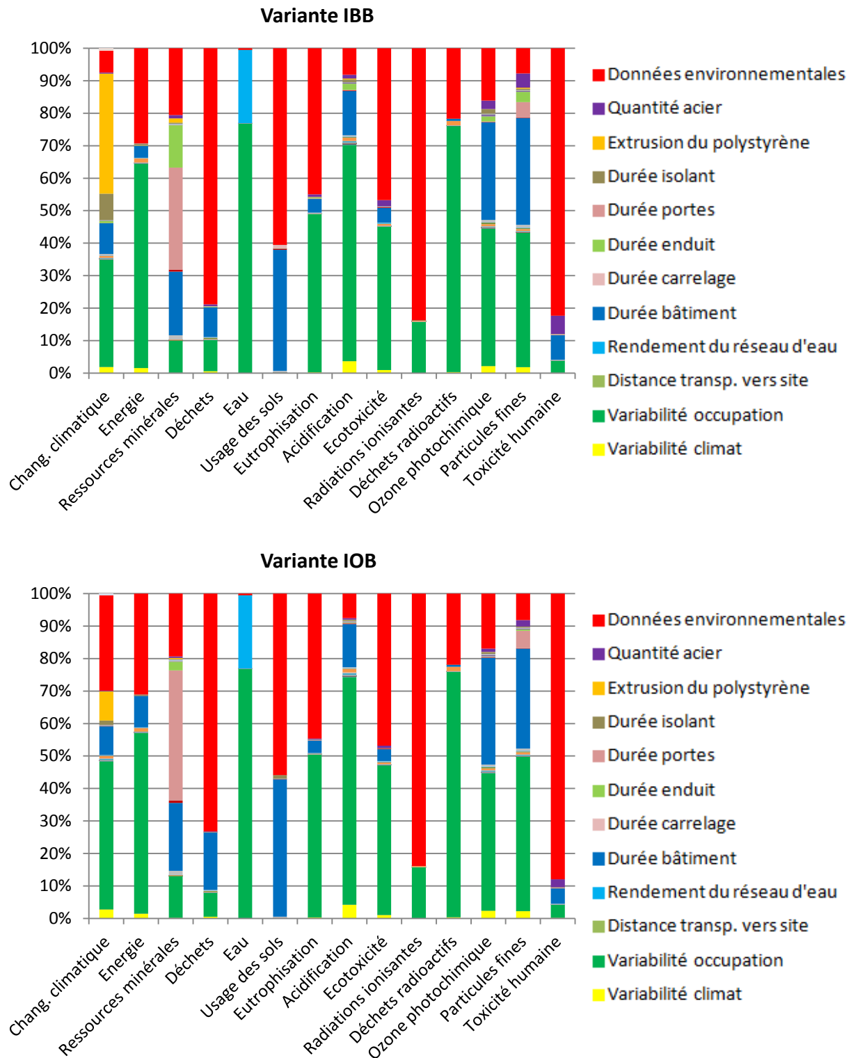
Figure N-66. Influence relative des facteurs incertains avec l'option 2 du criblage de Morris adapté
