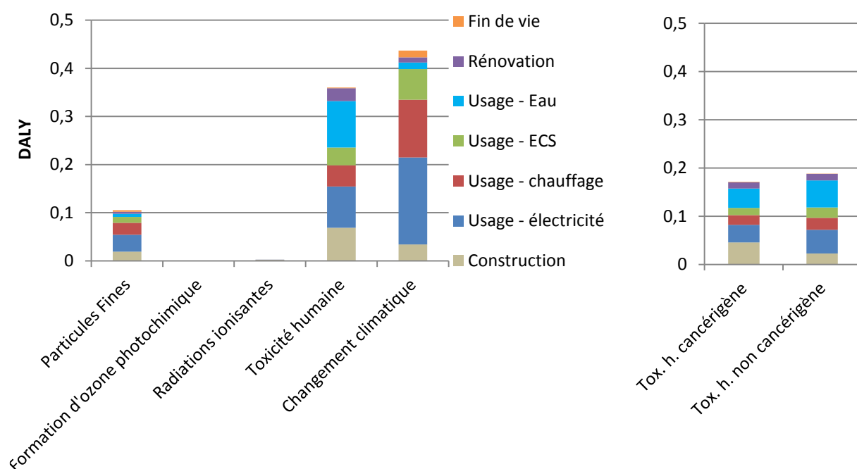
Figure 2-9. Analyse de contribution pour l'aire de protection santé humaine, pour la maison IBB, énergie électricité
