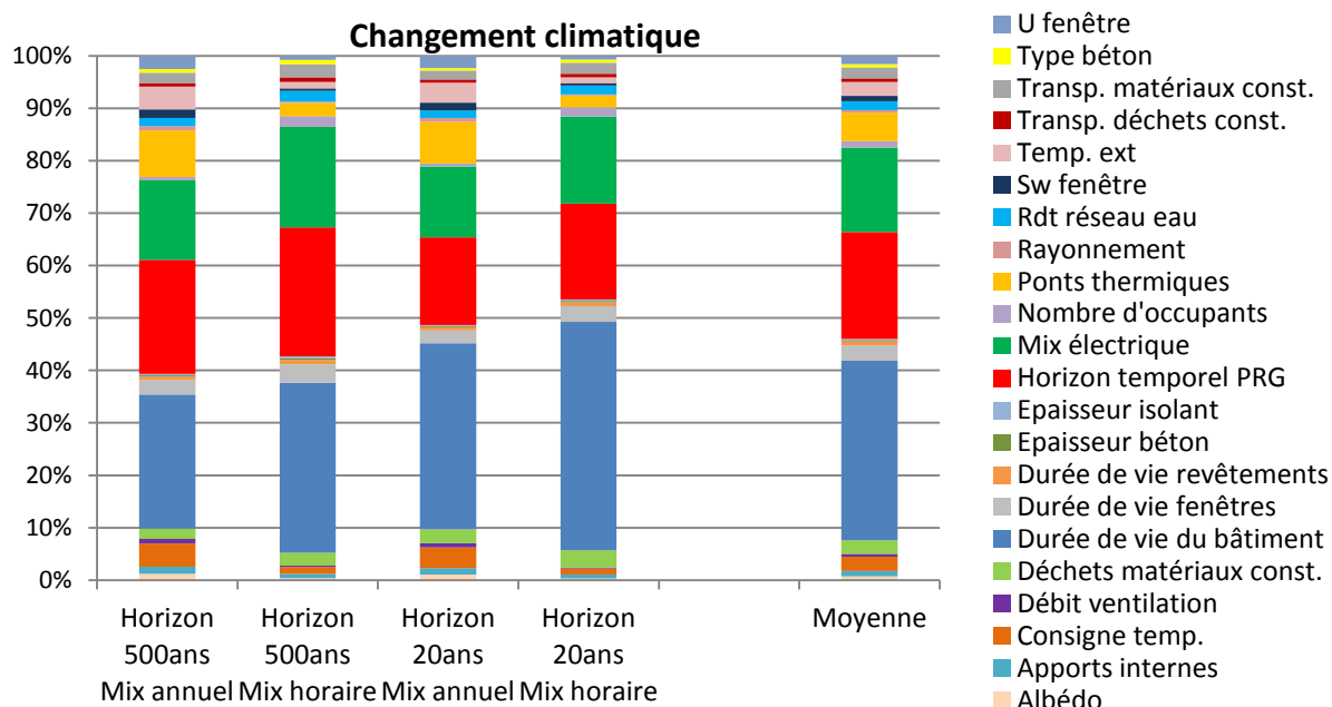
Figure L-36. Effet du choix de la référence pour deux variables catégorielles pour l'indicateur de changement climatique
