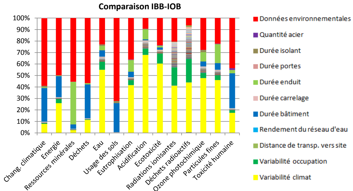
Figure N-71. Influence relative des facteurs incertains avec l'option 2 du criblage de Morris adapté en utilisant les distributions affinées
