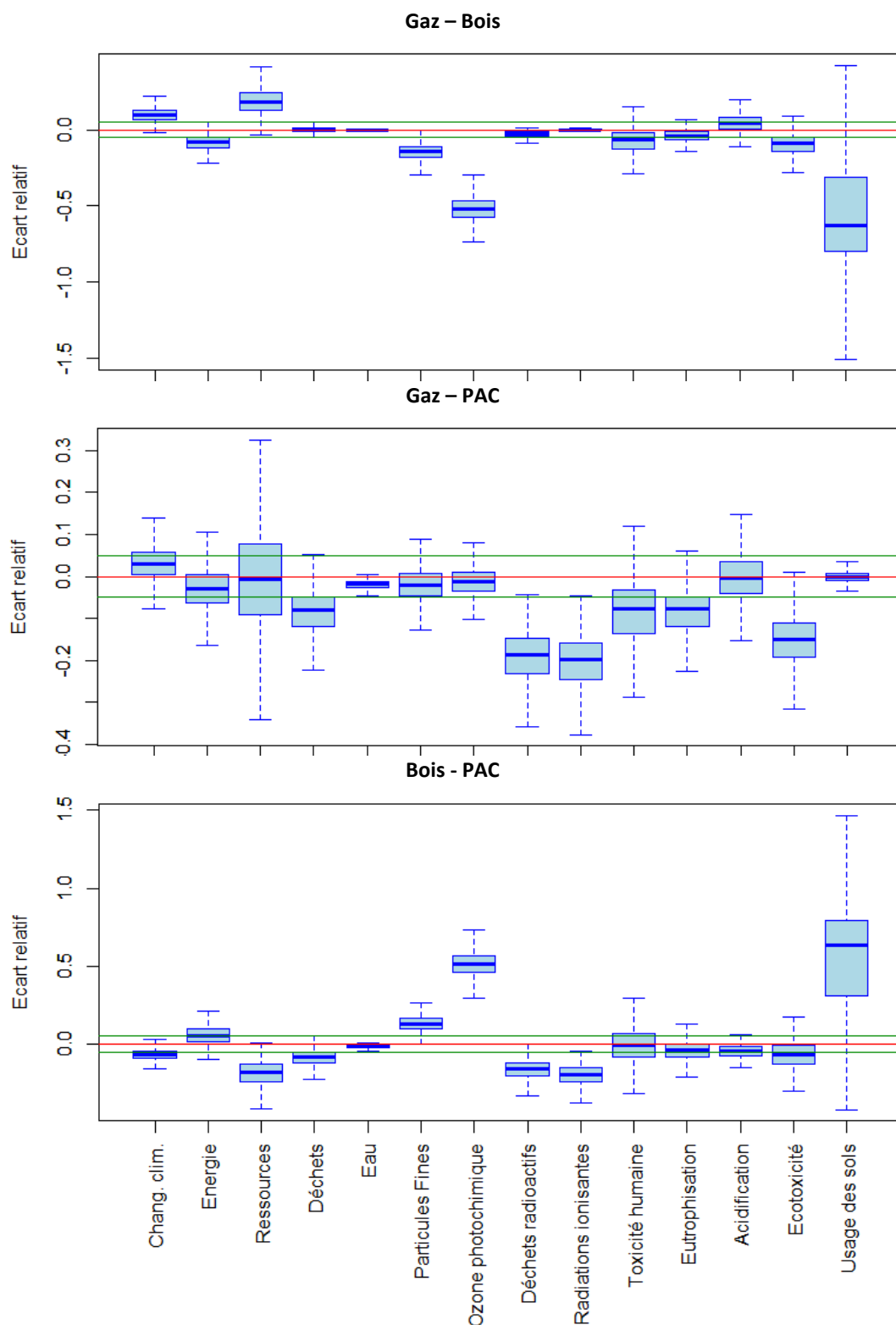
Figure N-81. Écart relatif entre les valeurs d'impact pour toutes les paires de variantes énergétiques avant amélioration de la caractérisation des incertitudes sur les facteurs
