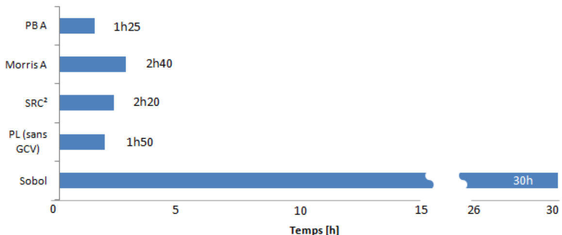
Figure 3-13. Comparaison des temps de calcul des méthodes adaptées
