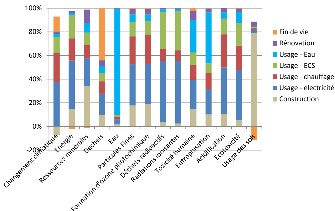
Figure J-28. Analyse de contribution pour la maison IOB, énergie électricité
