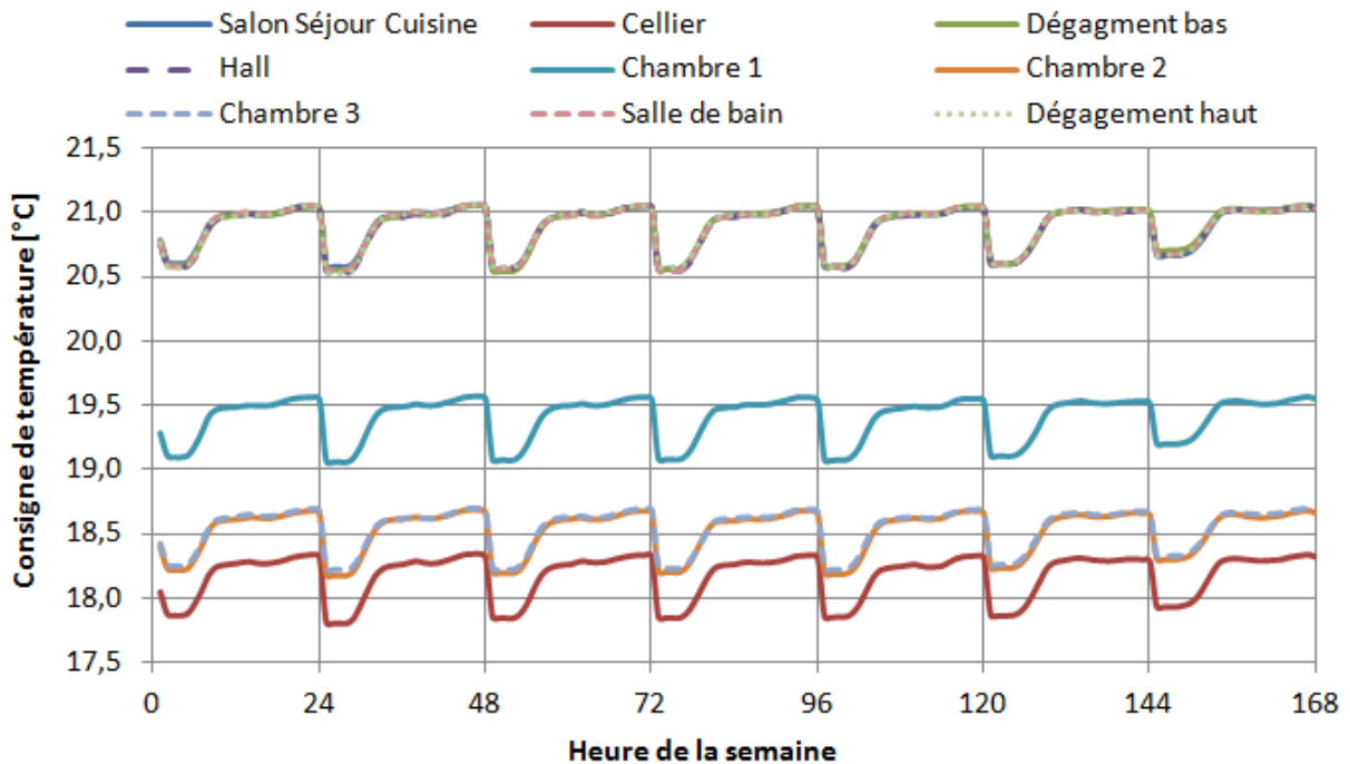
Figure J-10. Profil hebdomadaire de température par zone, hors période de vacances
