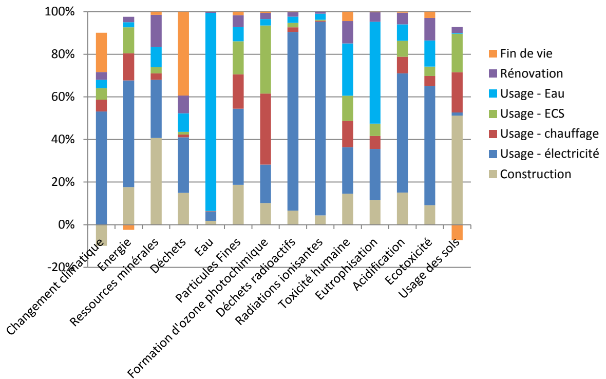
Figure J-30. Analyse de contribution pour la maison IOB, énergie bois
