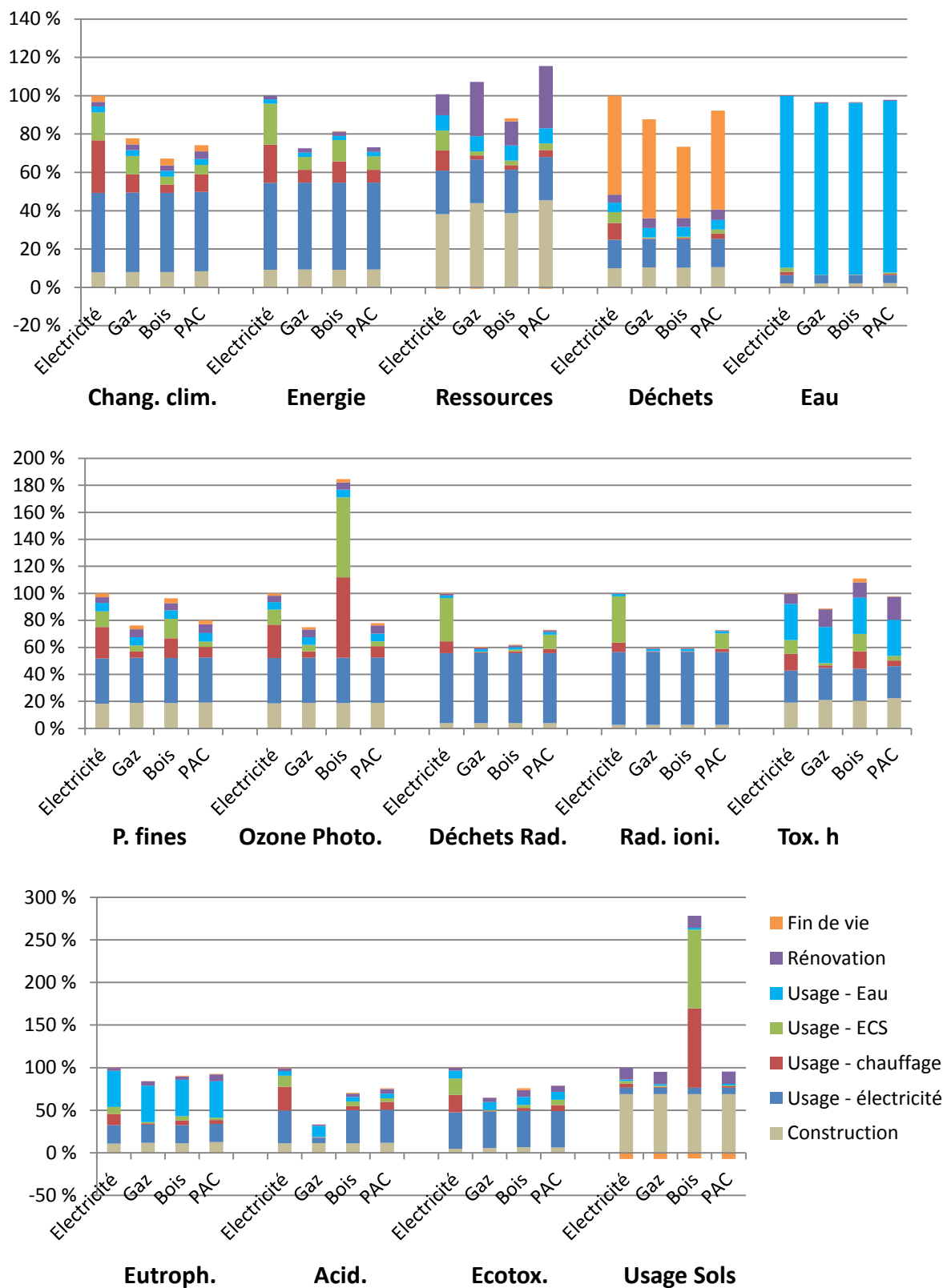
Figure 2-11. Comparaison des variantes énergétiques (la variante électricité sert de référence, et les impacts des autres variantes sont exprimés relativement à cette variante)
