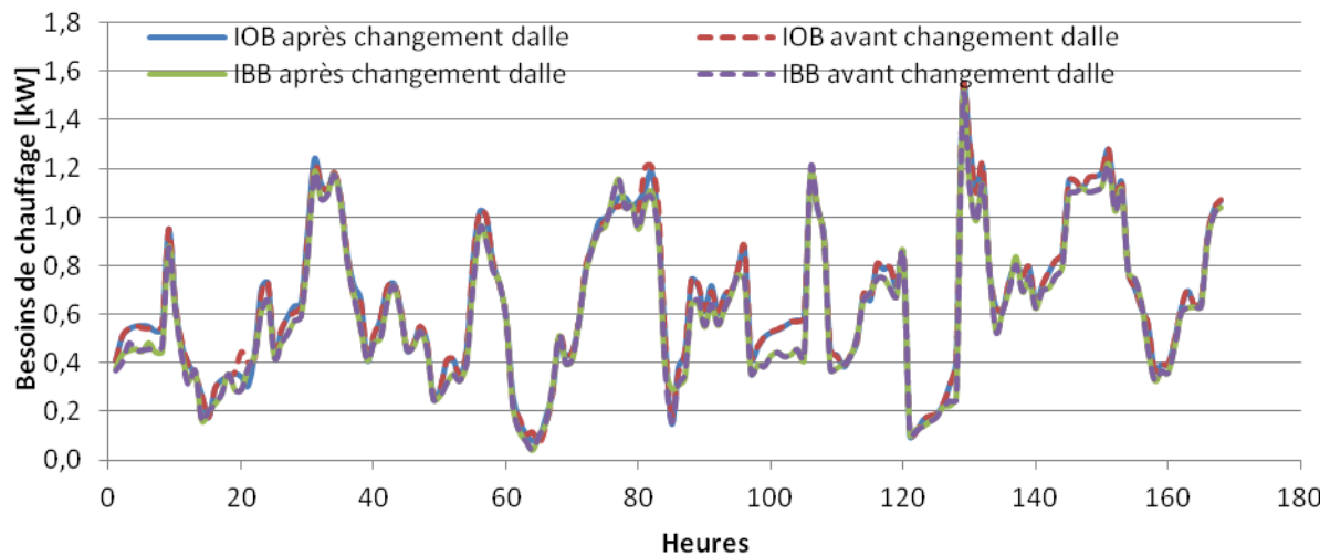
Figure N-68. Évolution des besoins de chauffage au cours de la deuxième semaine de l'année dans les maisons IBB et IOB avant et après modification de la capacité thermique volumique de la dalle
