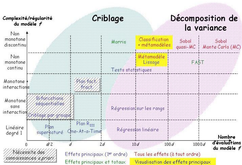
Figure 1-7. Grille de choix des méthodes d'analyse de sensibilité (Iooss, 2011)
