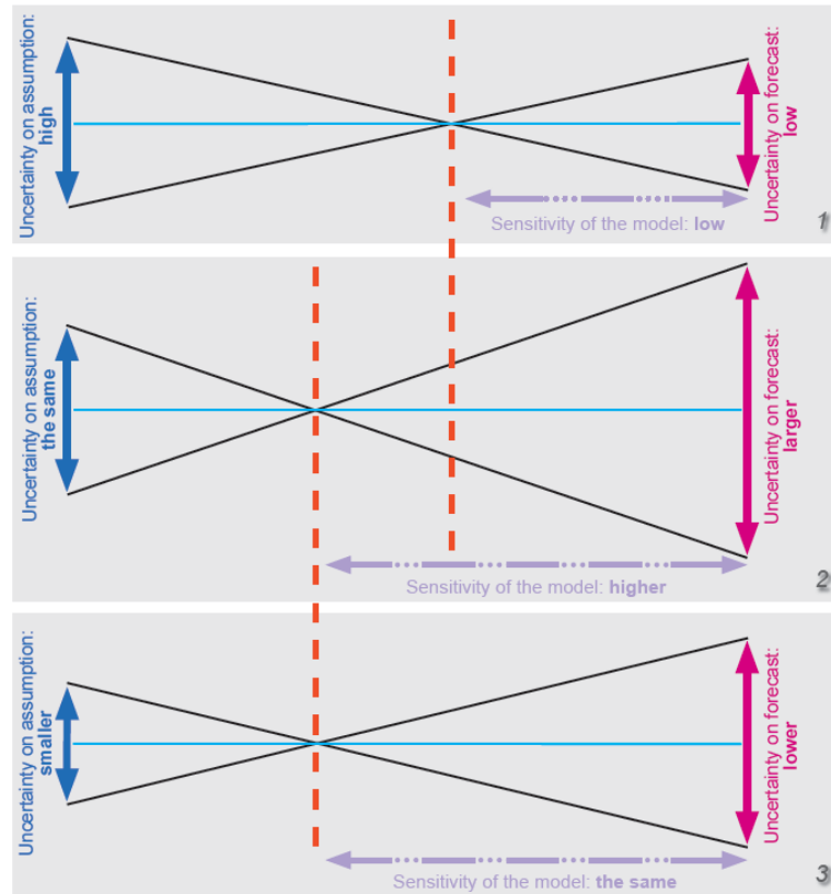
Figure 1-5. Lien entre incertitude de sensibilité (Chouquet, 2007)
