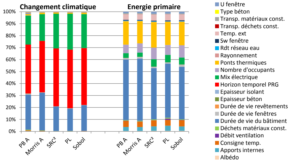
Figure 3-15. Comparaison de l'influence relative des facteurs incertains pour les méthodes adaptées dans un cas réel
