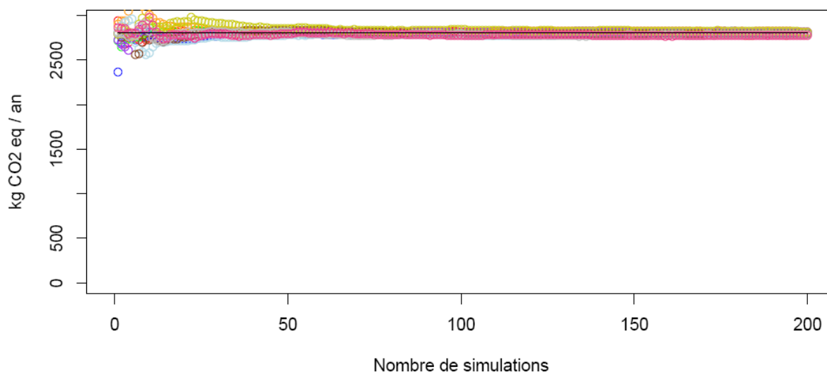
Figure 4-5. Convergence des résultats pour les incertitudes sur les données environnementales sur le changement climatique
