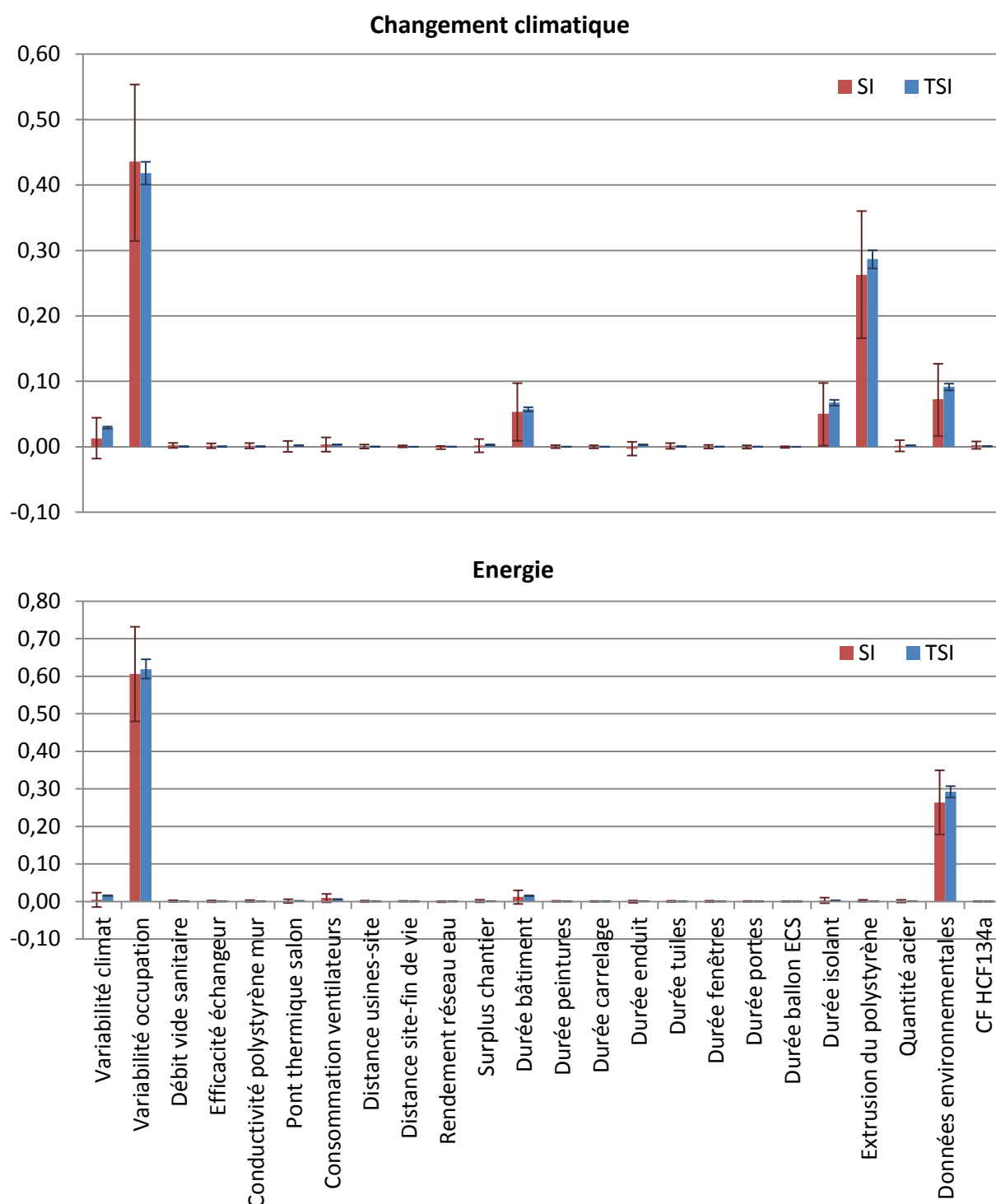
Figure M-64. Indices de Sobol de 1 er ordre et totaux
