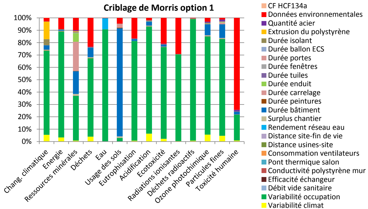
Figure M-61. Influence relative des facteurs incertains avec l'option 1 du criblage de Morris adapté
