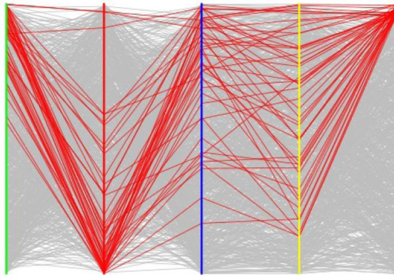
Figure E-4. Exemple de graphique cobweb issu de Iooss and Ribatet (2009)
