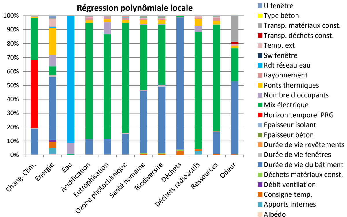
Figure L-47. Influence relative des facteurs incertains avec la régression polynômiale locale.
