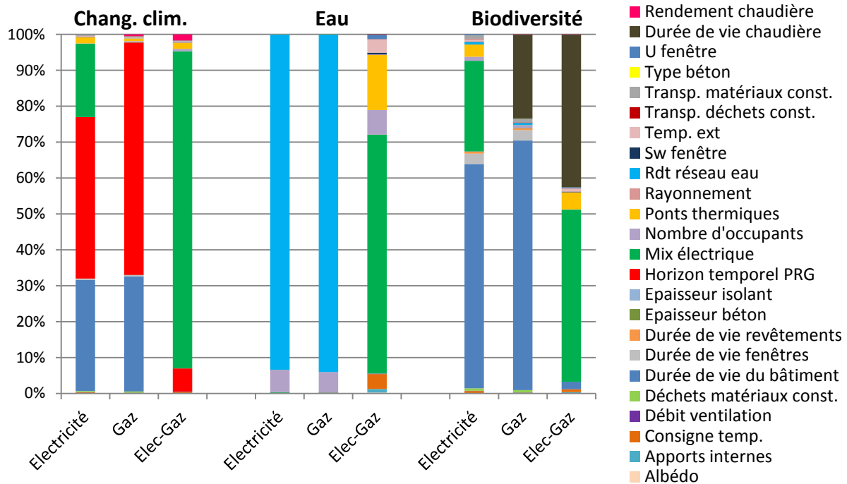
Figure 4-2. Facteurs incertains identifiés par la méthode de Morris adaptée pour deux variantes, indépendamment et en comparaison de variantes
