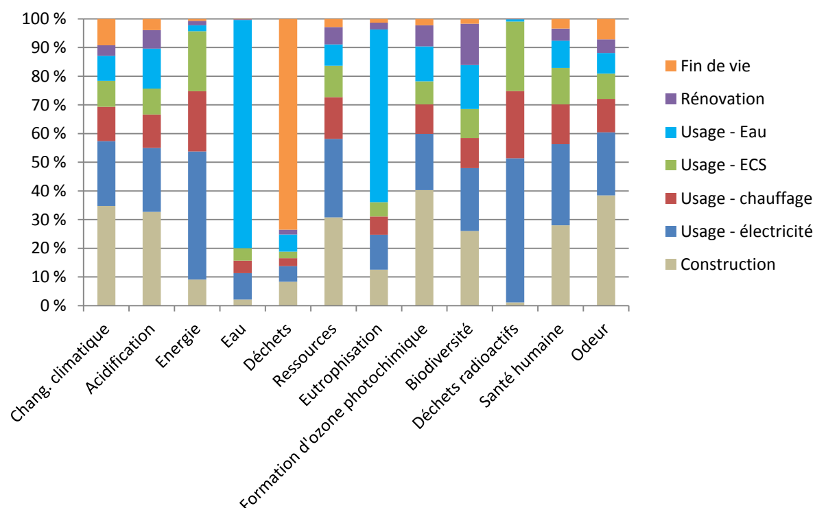
Figure 2-6. Analyse de contribution pour la maison IBB, énergie électrique
