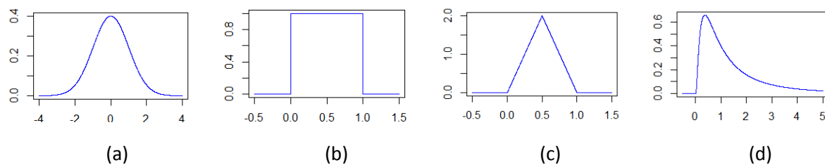
Figure 1-6. Distributions de probabilité (a) normale, (b) uniforme, (c) triangulaire, (d) log-normale
