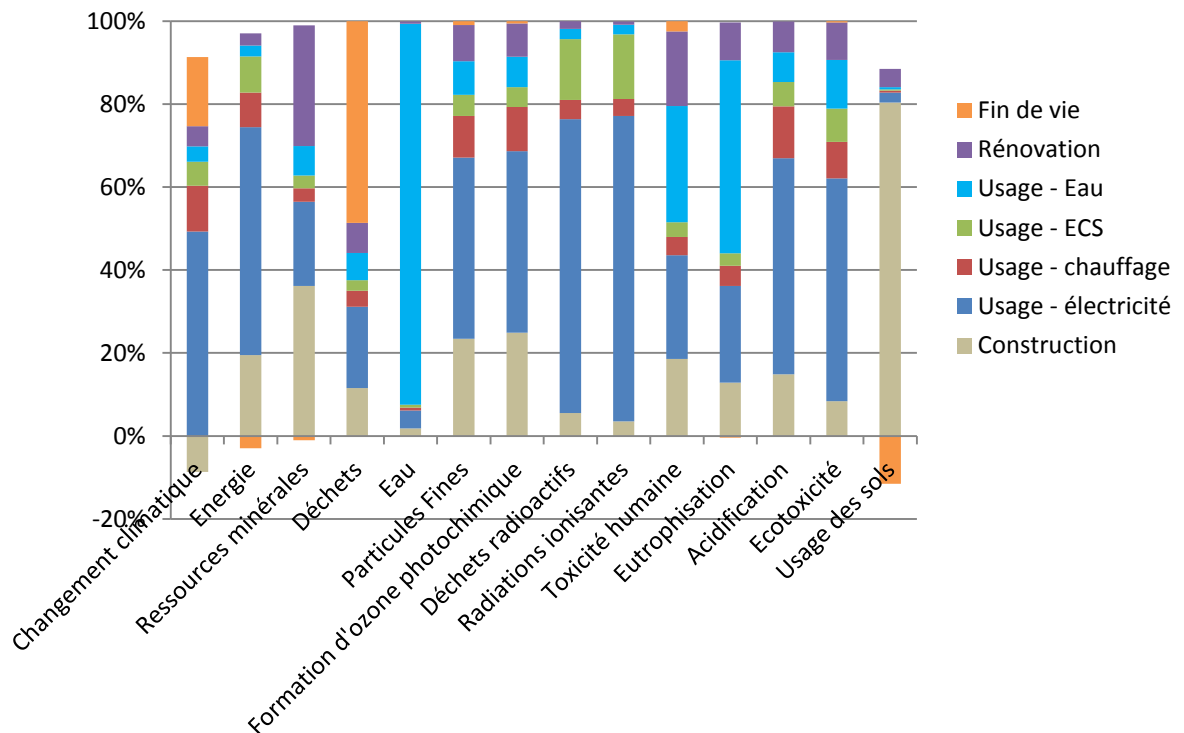
Figure J-31. Analyse de contribution pour la maison IOB, énergie électricité, PAC
