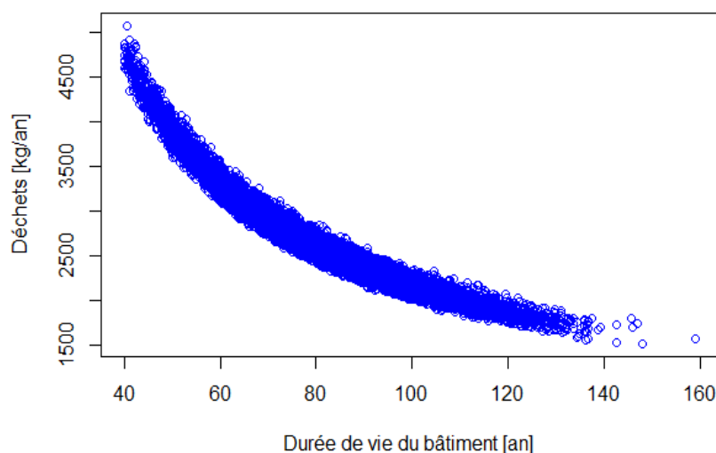
Figure L-46. Nuage de points des déchets produits en fonction de la durée de vie du bâtiment
