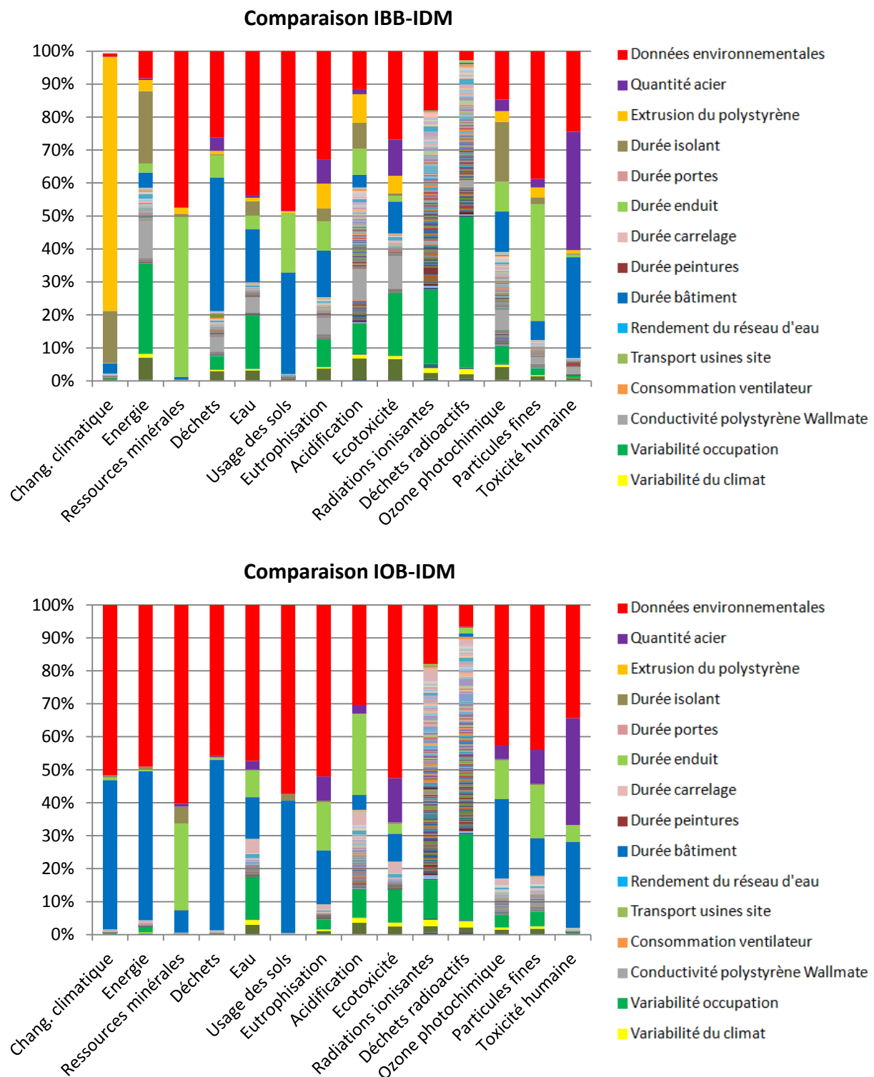
Figure N-72. Influence relative des facteurs incertains avec l'option 2 du criblage de Morris adapté pour IDM, IBB-IDM, IBB-IOB et IOB-IDM
