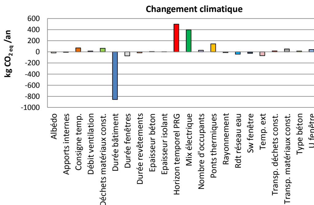
Figure L-34. Indice de sensibilité de tous les facteurs incertains pour l'indicateur de changement climatique
