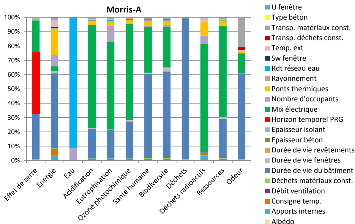
Figure L-52. Influence relative des facteurs incertains avec le criblage de Morris-A
