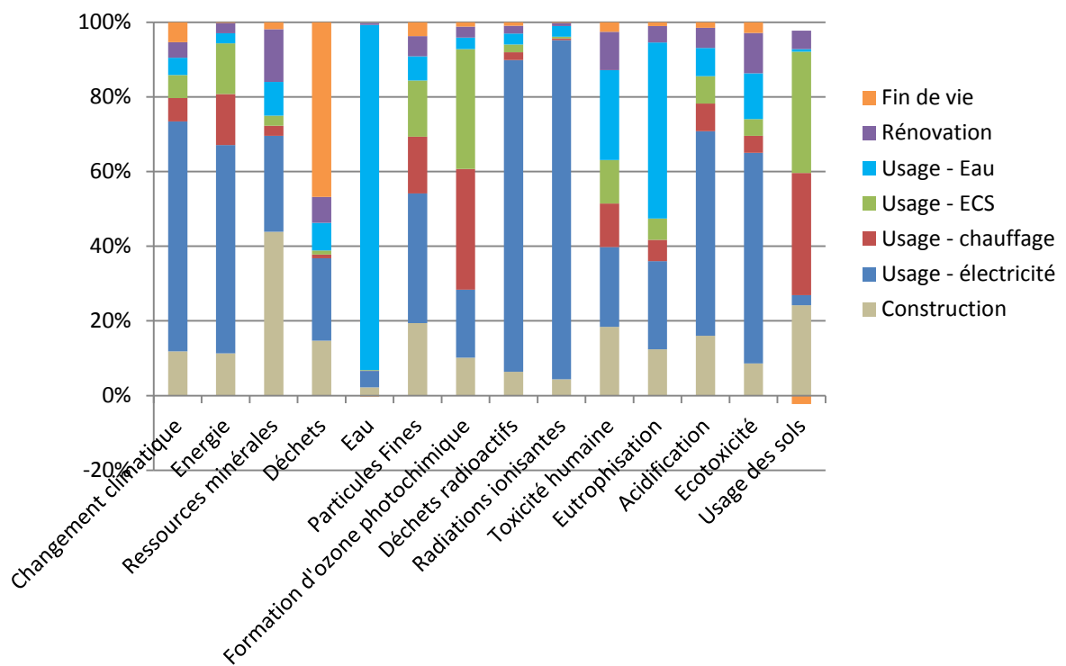
Figure J-22. Analyse de contribution pour la maison IBB, énergie bois
