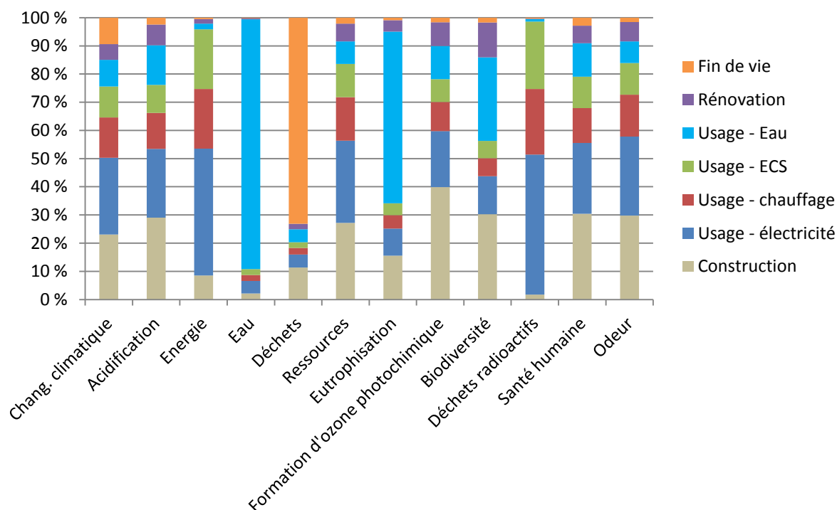
Figure J-12. Analyse de contribution pour la maison IBB, énergie électricité avec la base v2.2
