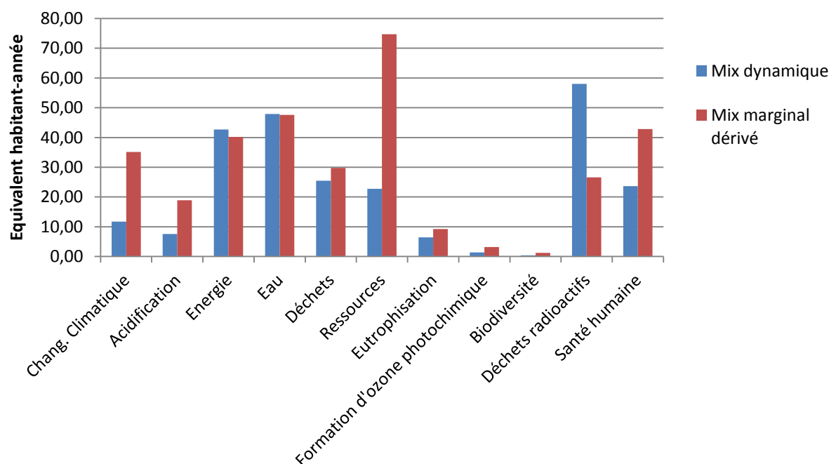
Figure J-15. Résultats normalisés pour la maison IBB, énergie électricité, avant et après changement du mix
