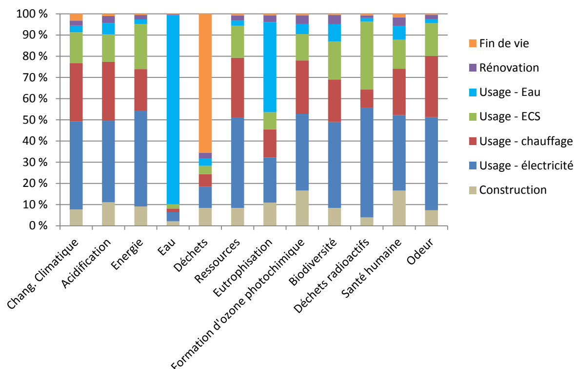
Figure J-14. Analyse de contribution pour la maison IBB, énergie électricité, mix marginal dérivé, avec la base v3.2
