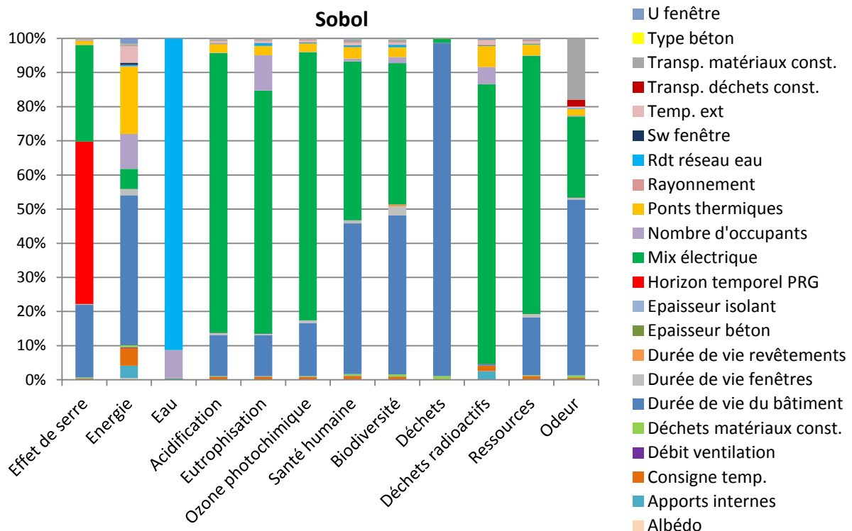
Figure 3-8. Influence relative des facteurs incertains avec la méthode de Sobol
