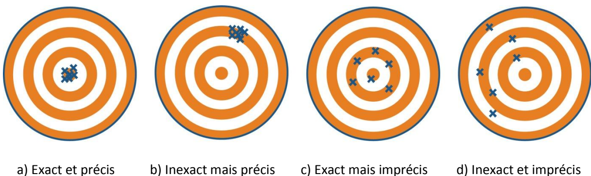
Figure 1-2. Exactitude et précision 5
