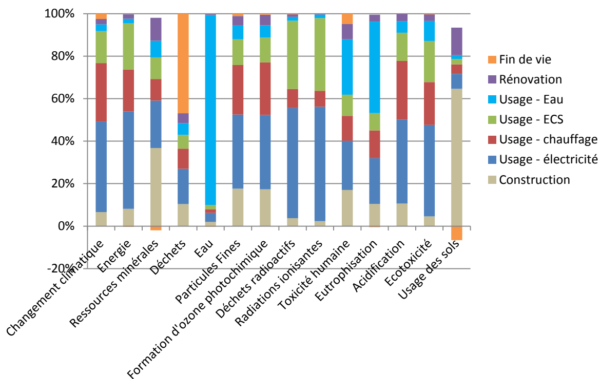
Figure J-24. Analyse de contribution pour la maison IDM, énergie électricité
