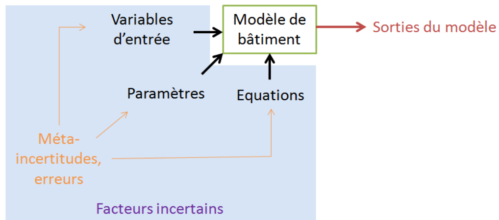
Figure 1-1. Sources d'incertitudes sur les sorties des modèles
