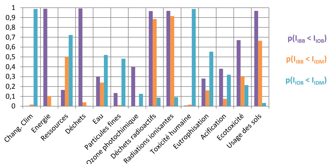
Figure 4-18. Probabilités qu'une variante soit meilleure qu'une autre pour les trois couples de variantes
