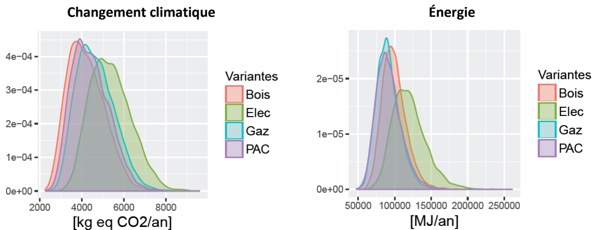
Figure 4-25. Distributions de probabilité en sortie pour les variantes Électricité, Gaz, Bois et PAC
