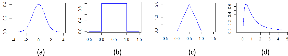
Figure D-2. Distributions de probabilité (a) normale, (b) uniforme, (c) triangulaire, (d) log-normale
