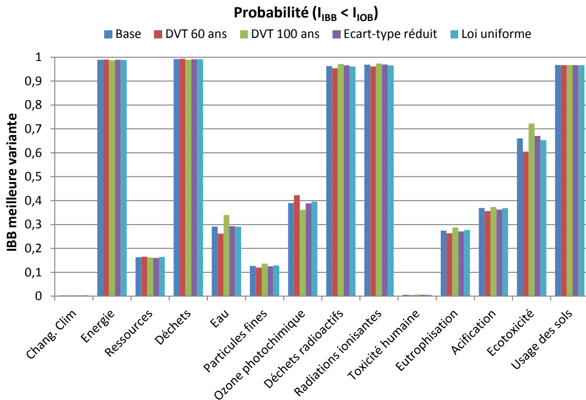
Figure 4-28. Évolution de la probabilité que IBB soit la meilleure variante en fonction des hypothèses prises sur la caractérisation de l'incertitude sur la durée de vie
