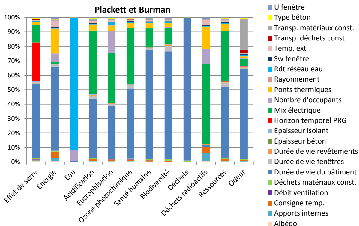
Figure L-38. Influence relative des facteurs incertains avec le plan de Plackett et Burman
