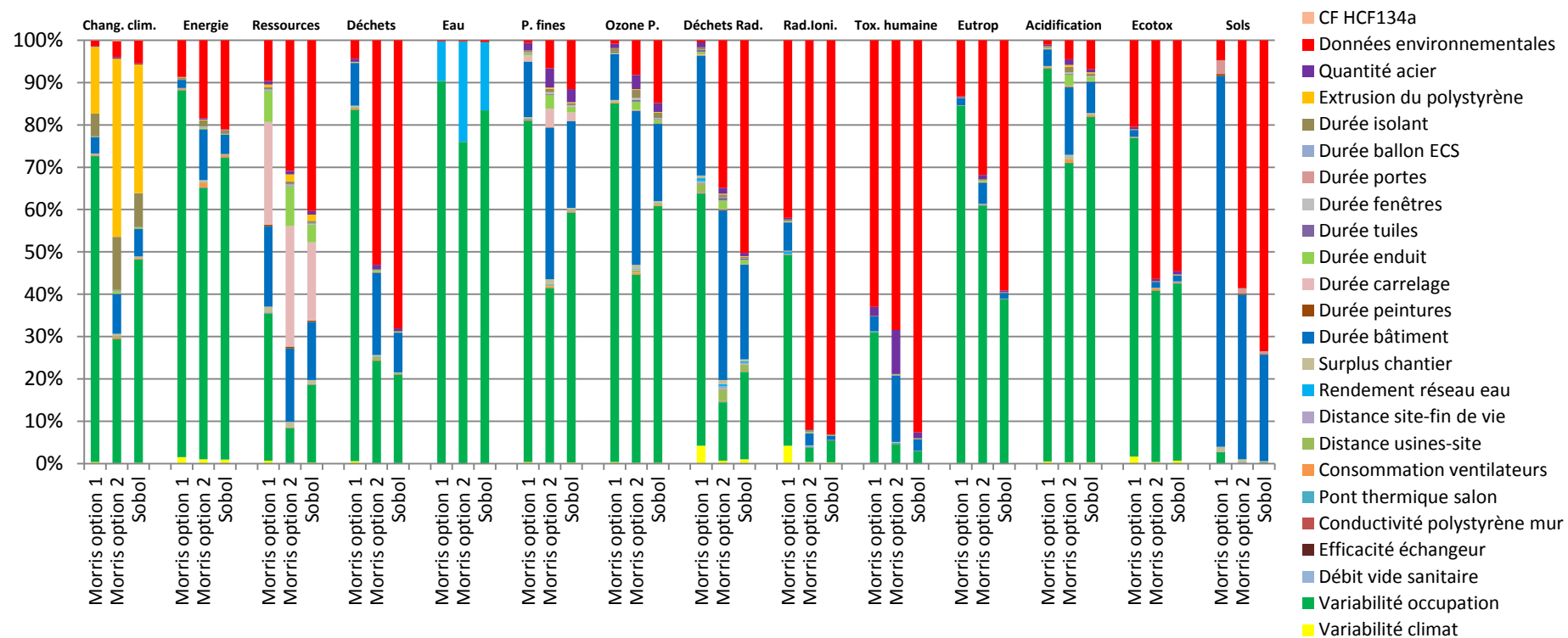
Figure M-65. Comparaison de l'influence relative des facteurs incertains avec les trois méthodes
