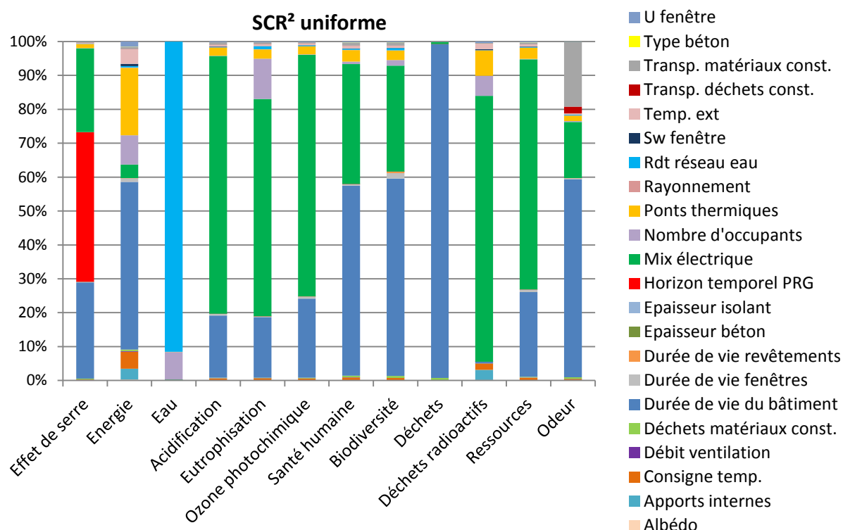
Figure L-53. Influence relative des facteurs incertains avec SRC 2 pour des lois uniformes
