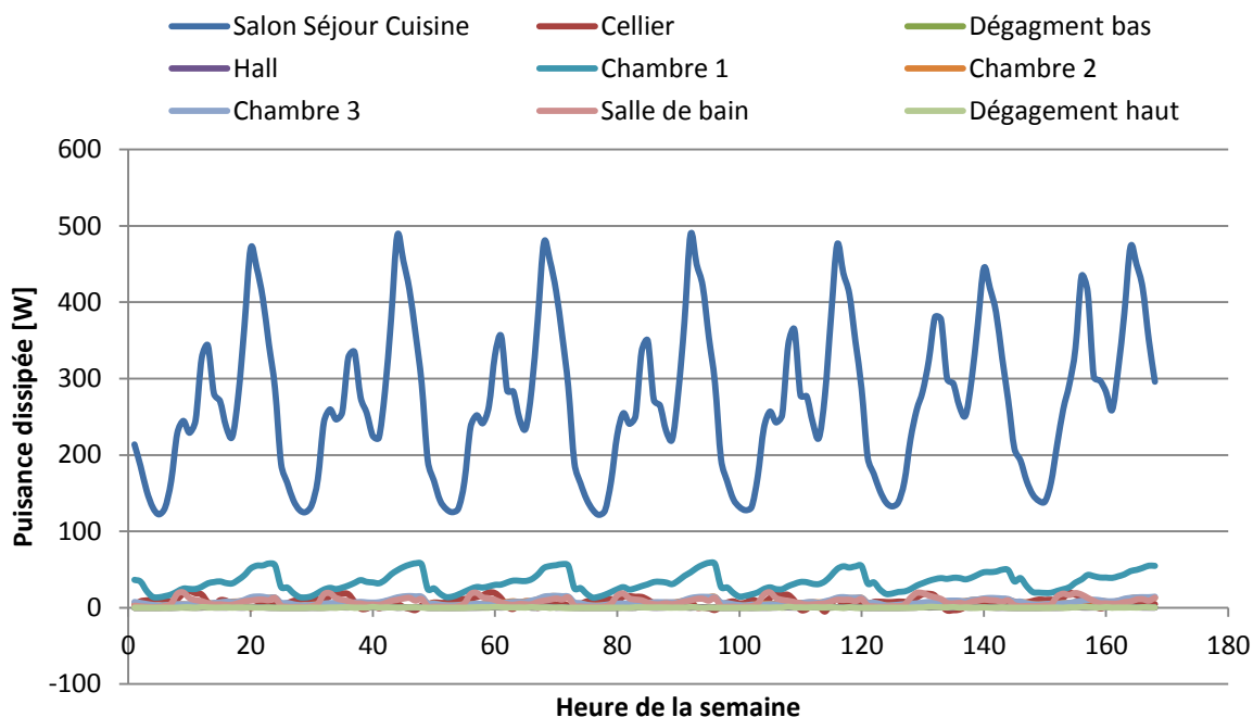
Figure J-8. Profil annuel moyen de puissance dissipée par les appareils électriques
