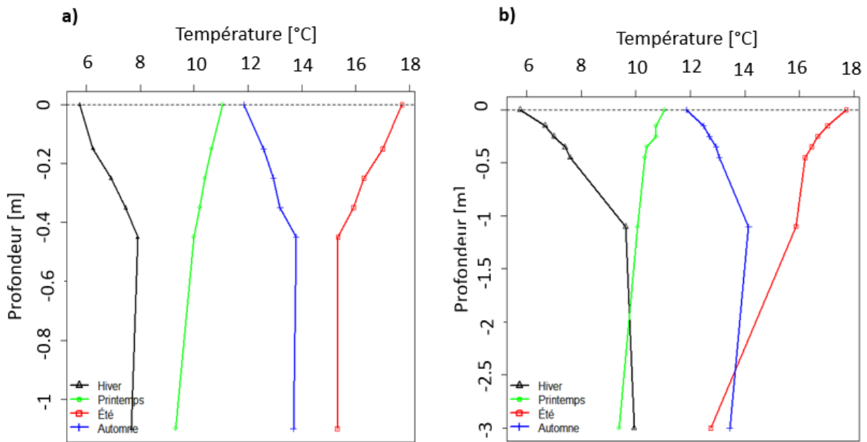
Figure 2.26 : Profils de température hyporhéiques saisonniers au droit de la station MOLONARI 1 (a : Rive gauche, b : Rive droite).
