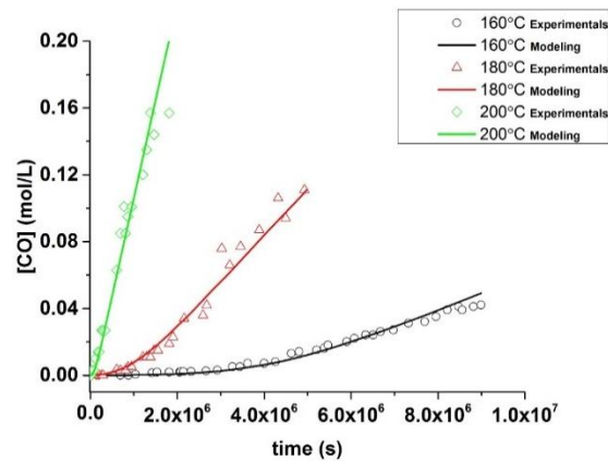
Figure 8 : Comparaison expérience-simulations de l'évolution des produits d'oxydation à 160 °C, 180 °C et 200 °C.
