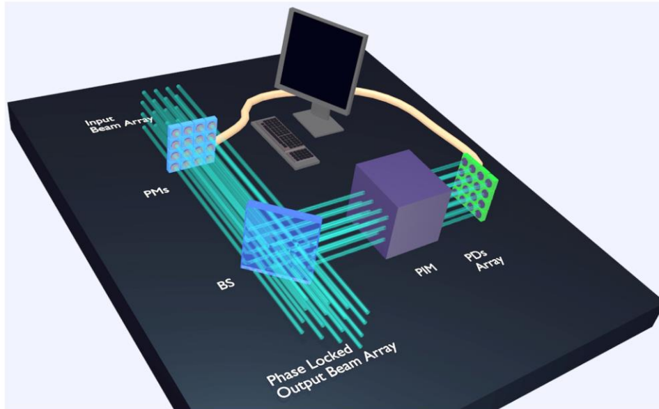
Figure I-19 : Schéma de principe du système laser de combinaison cohérente utilisant la méthode de Phase Intensity Mapping (PIM) [48].
