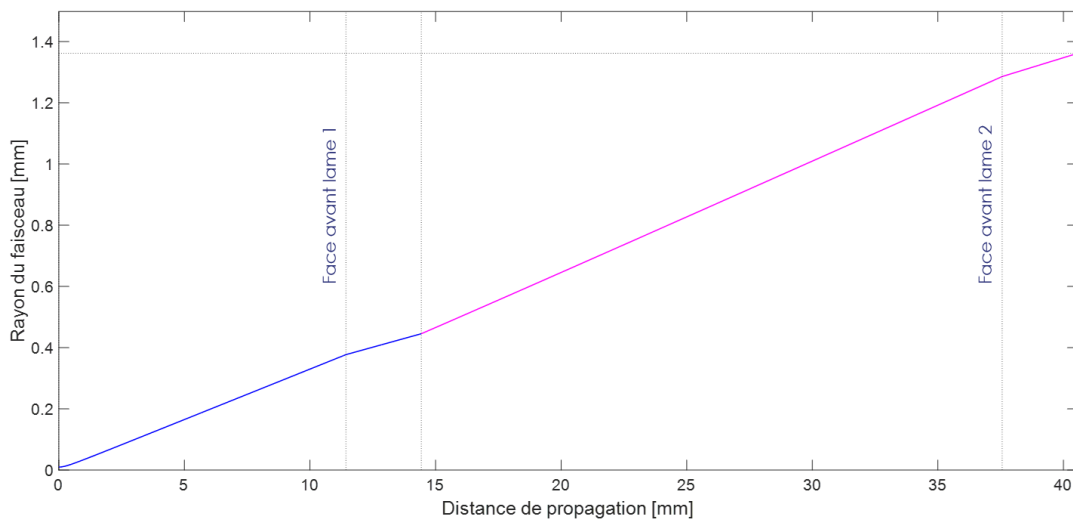
Figure IV-9 : Evolution du rayon du faisceau en sortie de tête optique en fonction de la distance de propagation
