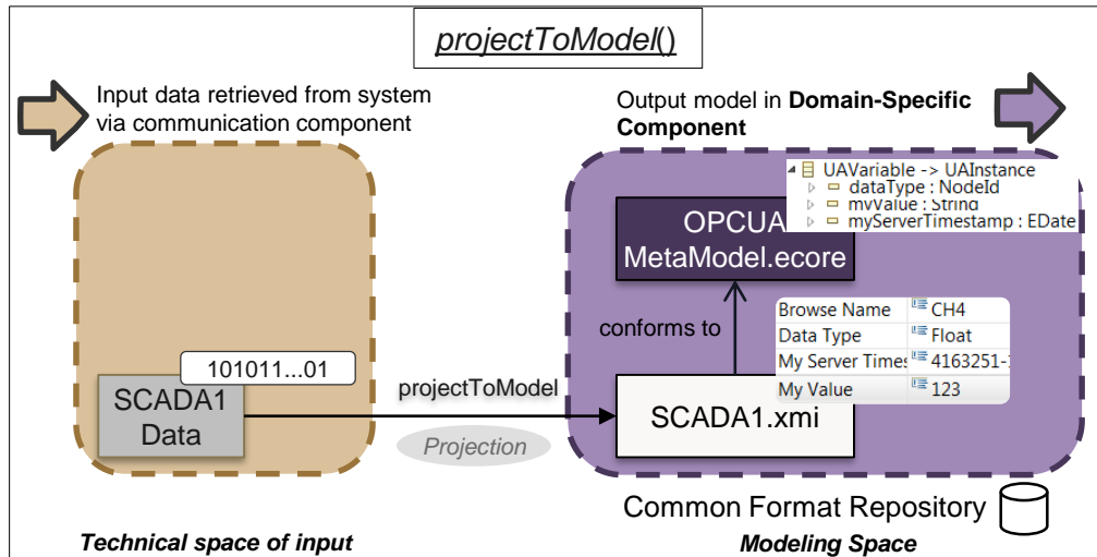
FIGURE 4.5 – Exemple de projection de données de système SCADA1
