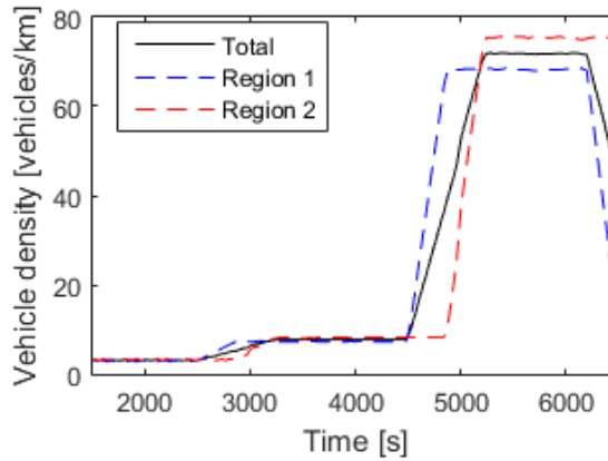
FIGURE 10 – Densité véhiculaire dans le scénario testé en fonction du temps, mesurée dans les régions 1 et 2, et densité dans la totalité du segment d'autoroute qui comprend les deux régions.
