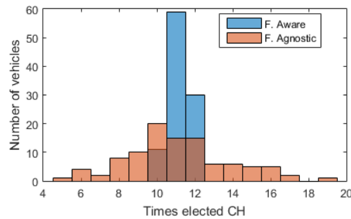
FIGURE 16 – Histogramme du nombre final de fois que chaque véhicule a servi comme CH.
