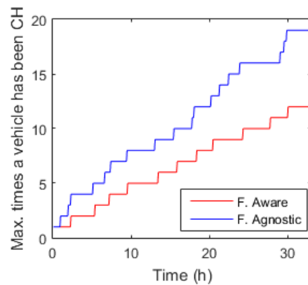
FIGURE 14 – Nombre maximum de fois qu'un véhicule a servi comme CH en fonction du temps.
