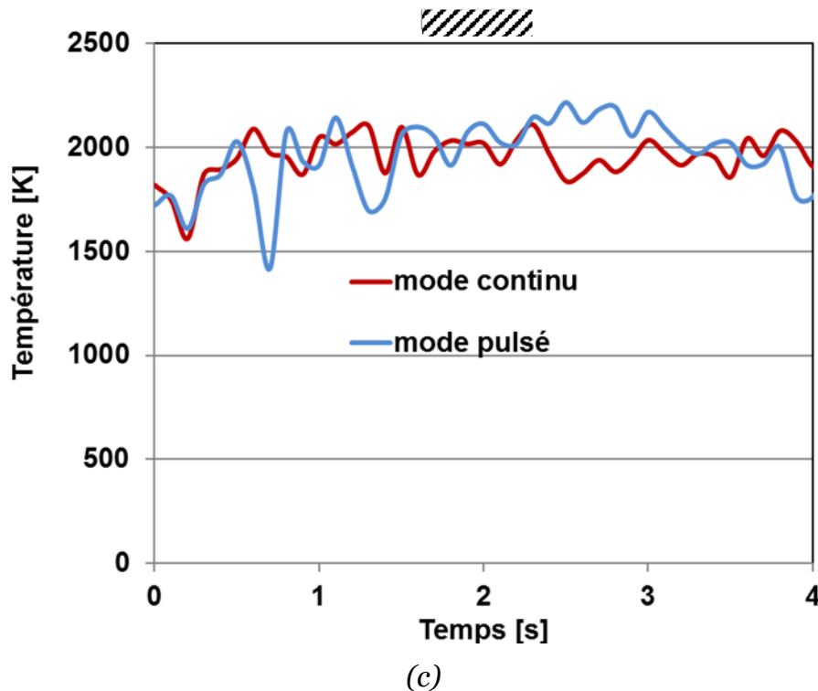
Figure 62 : Mesure de température par pyrométrie UV sur des essais de découpe à ; (a) XW ;(b) XW et (c) XW.
