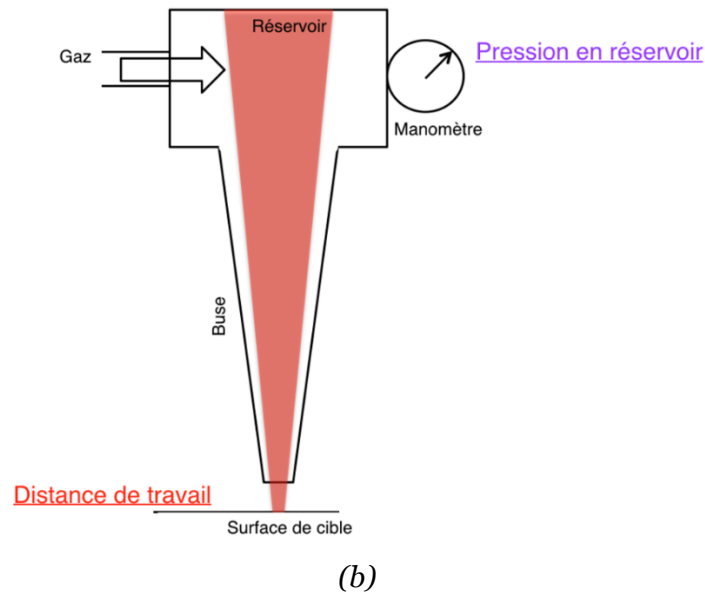
Figure 25 : (a) dispositif expérimental ;(b) schématisation du dispositif expérimental
