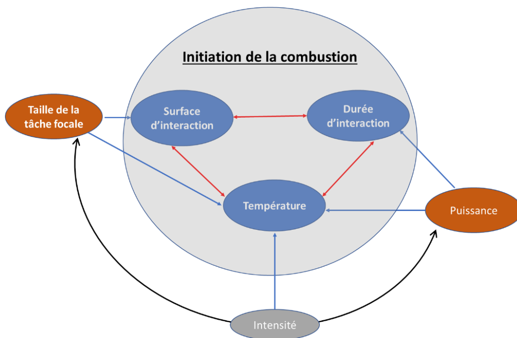
Figure 63 : Les principaux éléments entrant en jeu dans l'initiation de la combustion
