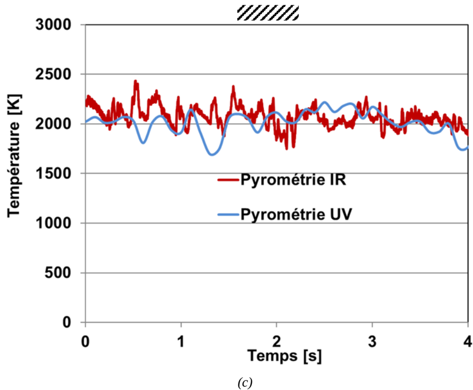
Figure 60 : Mesure de température par pyrométrie IR sur des essais de découpe à ; (a) XW ;(b) XW et (c) XW.
