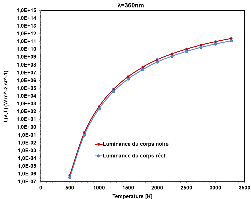
Figure 48 : Luminance du corps noir (émissivité \varepsilon = 1 ) et du corps réel (émissivité \varepsilon = 0,5 ) en fonction de la température
