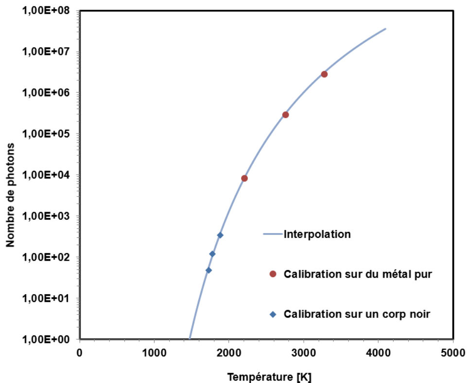
Figure 53 : Interpolation du nombre de pontons en fonction de la température.
