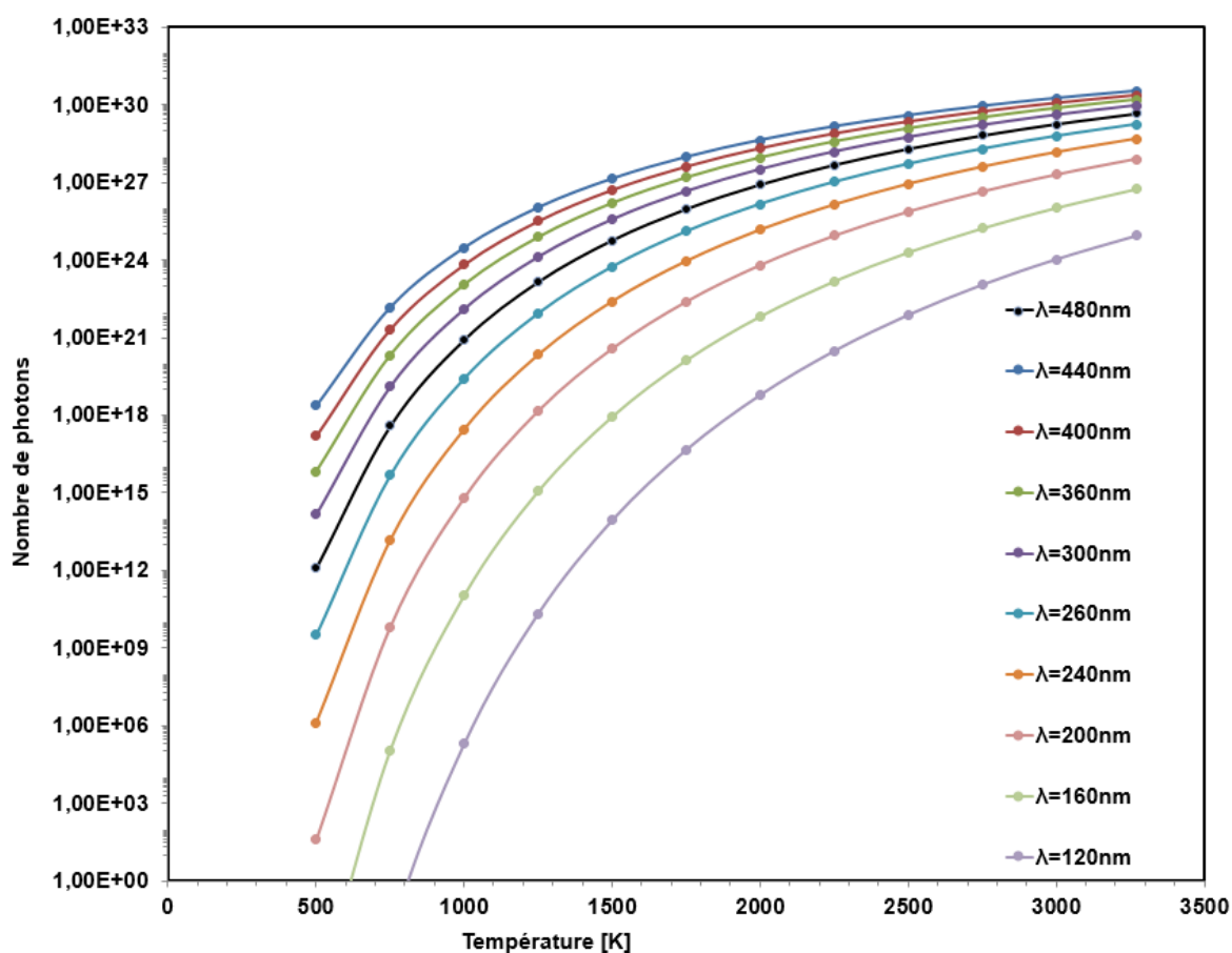
Figure 50 : Evolution d'un nombre de photon émis par un corps noir en fonction de la température à différentes longueurs d'onde
