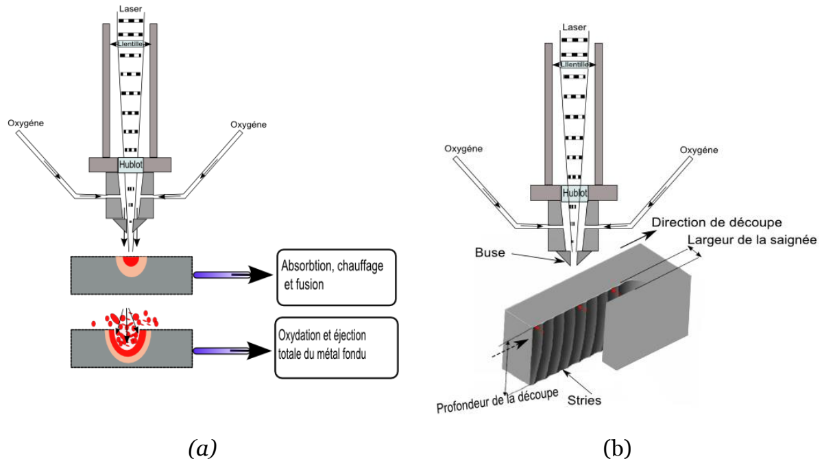
Figure 14 : Découpe laser (a) initiation (b) découpe
