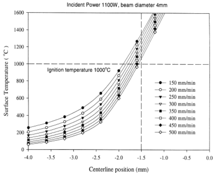
Figure 10 : Température en surface de l'acier de 20mm d'épaisseur en fonction de la vitesse (a) pour une puissance incidente de 700W, (b) pour une puissance incidente de 1100W[2].
