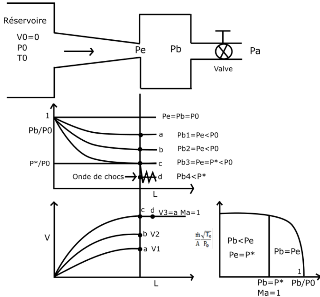
Figure 41 : Écoulement et ondes de choc dans une buse convergente
