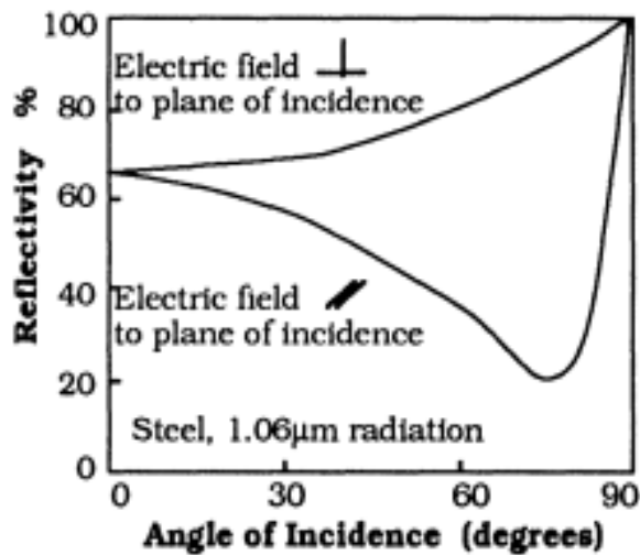
Figure 21 : Réflectivité de l'acier en fonction de l'angle d'incidence d'un faisceau (longueur d'onde de 1.06μm)[29]
