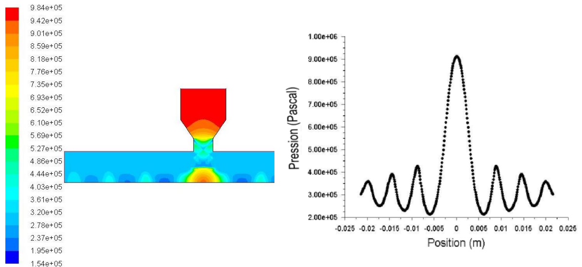
Figure 45 : Profil de pression en sortie de buse et jusqu'à la surface de l'échantillon (a) 3 bar (b) 6 bar (c) 9 bar
