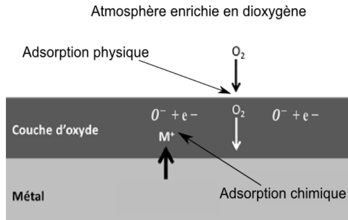
Figure 8 : Processus d'oxydation
