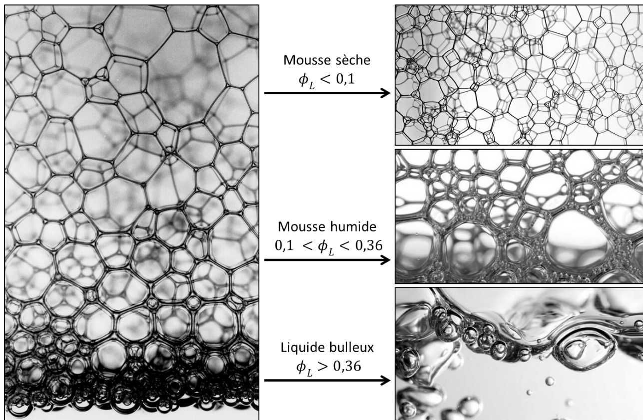
Figure 3 : Illustration d'une mousse avec un gradient de fraction liquide volumique. En bas, la mousse est en contact avec une solution liquide, sa fraction liquide est importante et les bulles sont à peine en contact ponctuel. Au-dessus, la fraction liquide volumique diminue et les bulles entrent en contact en se partageant un film comme surface commune. Les bulles se déforment progressivement avec la diminution de la fraction liquide volumique et forment finalement des polyèdres au sein d'une mousse sèche.
