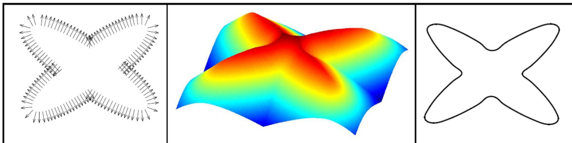
FIGURE 2.16 – (À gauche) Nuage de points orienté. (Au centre) Fonction implicite calculée par IMLS à partir des points. (À droite) Surface reconstruite en prenant l’iso-zéro de la fonction implicite. (Figure reproduite de (KOLLURI, 2005))
