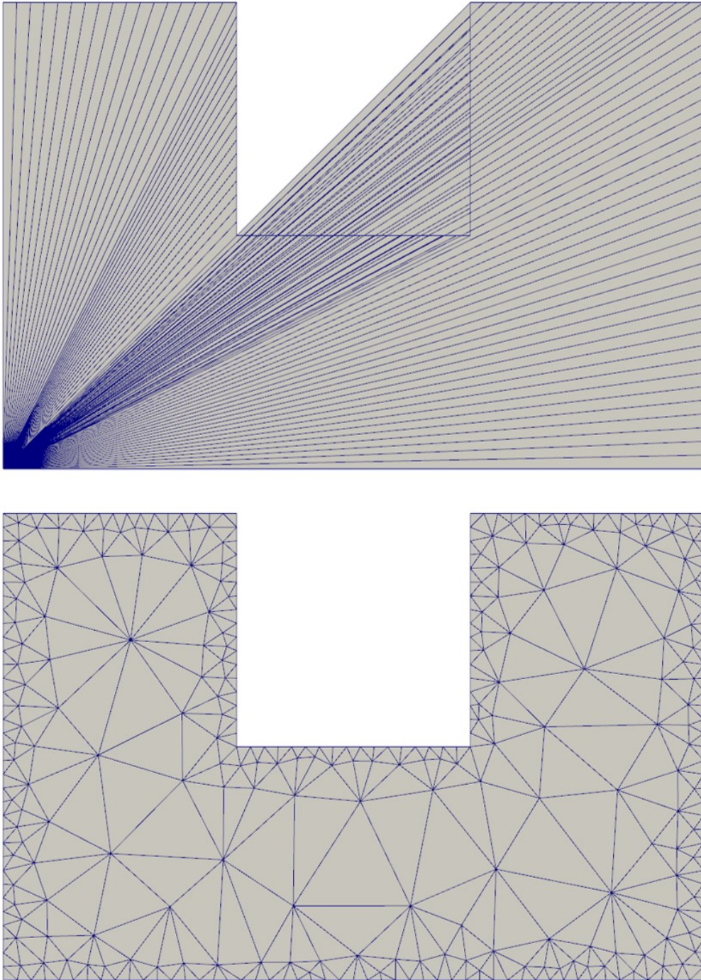
FIGURE B.5 – Résultats obtenus à partir d'un contour 2D non convexe qui comporte 203 nœuds. (En haut) état initial. (En bas) après 200 itérations le maillage comporte 571 triangles.
