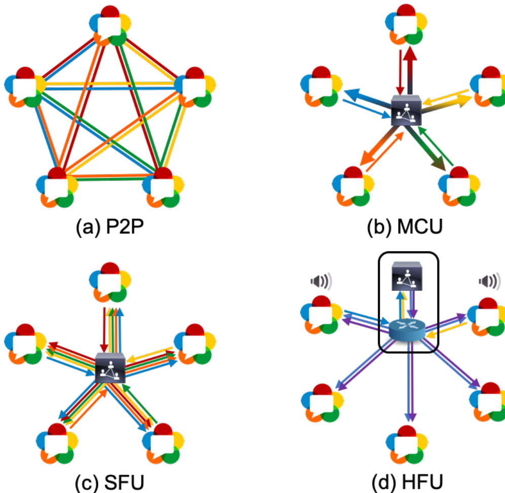
Figure 5.3: WebRTC (a,b,c) and hICN-RTC (d) architectures
