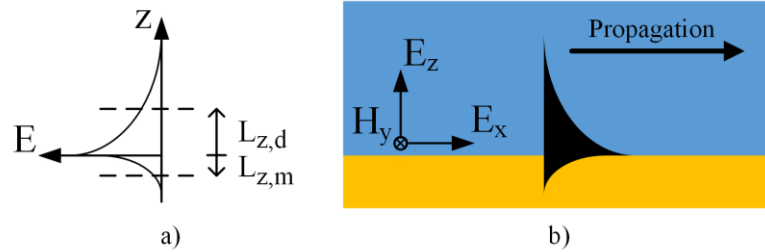
Figure 2.5 – Schéma du profil d'intensité des plasmons de surface lors de la propagation. a) L'énergie de l'onde évanescente décroît spatialement dans les matériaux (z). La profondeur de pénétration L_z est définie par la diminution de l'amplitude par un facteur 1/e . b) L'onde propagative évanescente est atténuée dans la direction de propagation (x).
