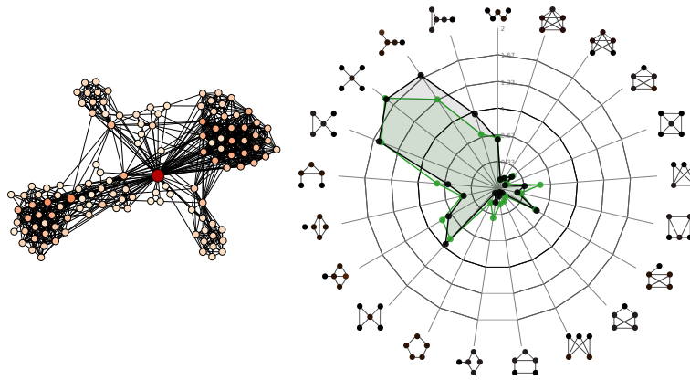
FIGURE 5.17 – centroïde étoilé
