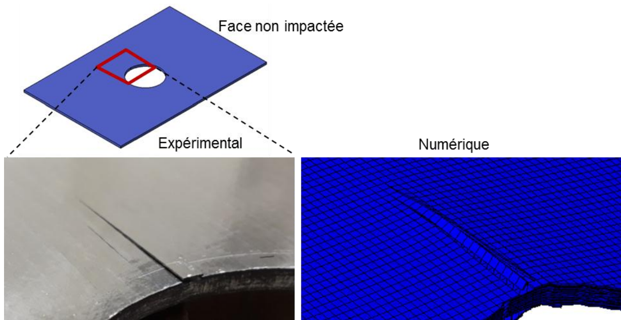
Figure 5-14 – Présence des échantillons localisés en bord de trou sur la face non impactée
