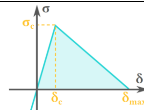
Figure 2-15 – Principales lois de comportement des éléments cohésifs
