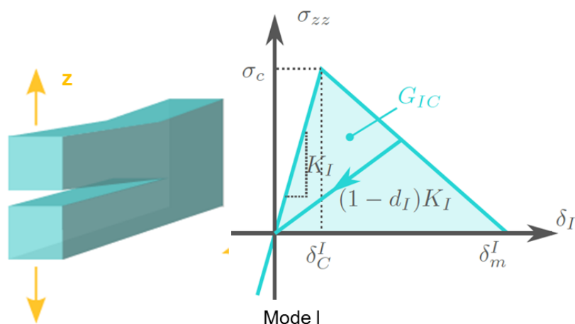
Figure 2-16 – Loi linéaire par morceaux décrivant le comportement d'un élément cohésif en mode d'ouverture (mode I) [Son11]
