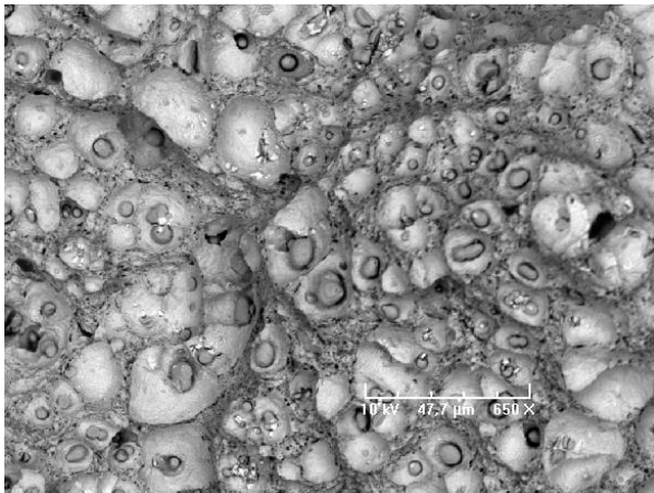
Figure V-44 : Faciès de rupture des essais au zirconium grossissement x650
