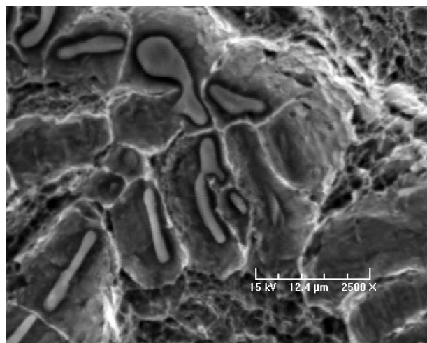
Figure V-41 : Faciès de rupture, premiers essais au lanthane, grossissement x2500
