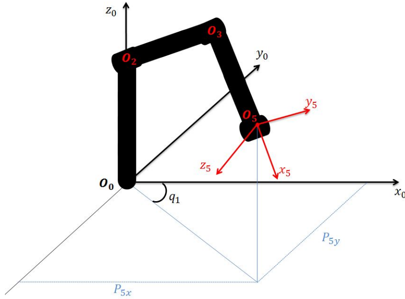
FIGURE 8.3 – L'angle de la première articulation du robot
