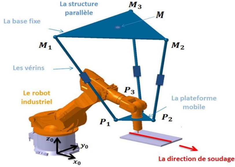
FIGURE 5.13 – La structure parallèle ajoutée au robot industriel
