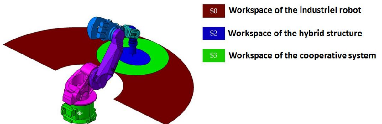
FIGURE 6.34 – L'espace de travail de la structure hybride et du système coopératif
