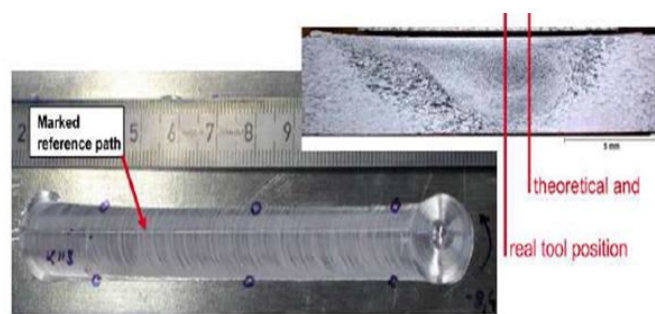
FIGURE 3.9 – Déviations de l'outil de sa trajectoire désirée [101]
