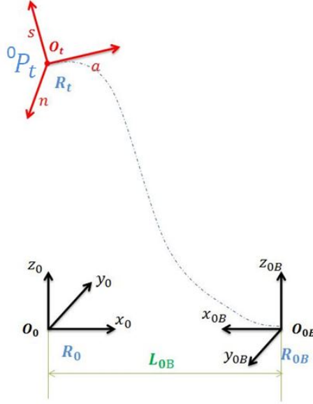
FIGURE 6.6 – La représentation de la position relative des repères R_t , R_{02} par rapport à R_0
