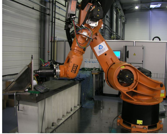
FIGURE 4.10 – La mesure des raideurs [36]
