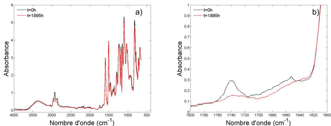
Figure A2:4: Spectres FTIR de DGEBA-DDS avant et après 1895h en immersion dans l'eau à 70°C a) dans la gamme 4000-400 \text{cm}^{-1} b) 1800-1600 \text{cm}^{-1} .
