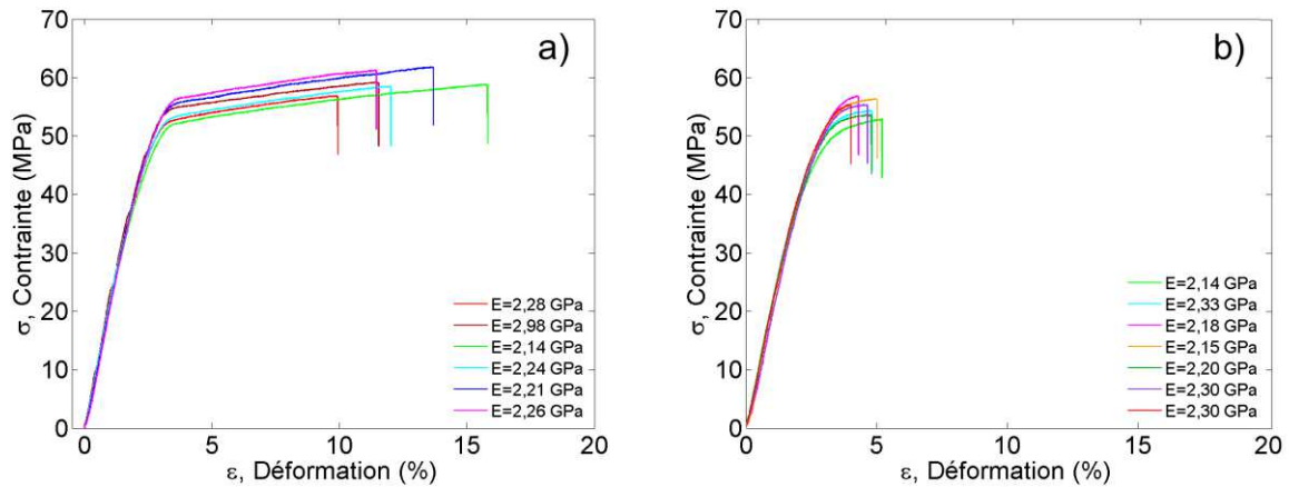
Figure 3:30 : Influence de la grille en polyamide sur les propriétés mécaniques à l'état initial a) sans grille b) avec grille.
