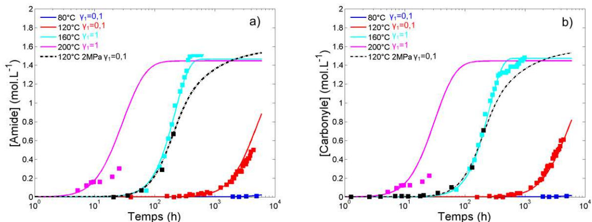
Figure 4:31: Comparaison des modélisations et des données expérimentales à 80°C, 120°C, 160°C, 200°C pour DGEBA-DDS a) amides b) carbonyles.
