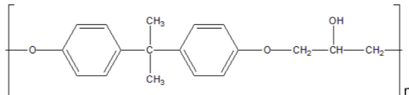
Figure 2:4: Structure chimique du motif de répétition de PKHJ.
