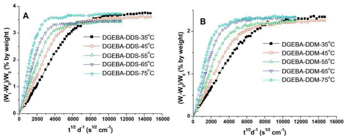
Figure 1:17: Courbes de sorption pour les réseaux DGEBA/DDS et DGEBA/DDM à différentes températures[101].
