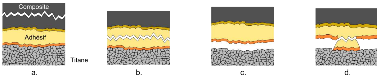
Figure 1:14 : a) Rupture cohésive du substrat (ici le composite) b) Rupture cohésive dans l'adhésif c) Rupture adhésive (ex : Titane/Adhésif) d) Rupture mixte.
