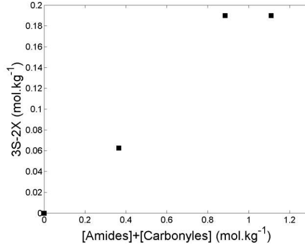
Figure 3:20: Evolution des coupures de chaînes (S) et réticulation (X) en fonction de la concentration en produits d'oxydation à 120°C.
