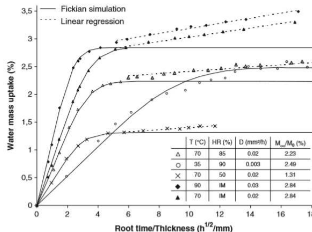
Figure 1:35: Courbes de sorptions d'une résine époxy/amine et la déviation de la loi de Fick aux temps longs.
