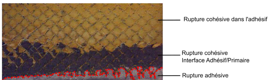
Figure 2:11: Exemple de quantification de la proportion de rupture adhésive/cohésive sur éprouvette de cisaillement simple avec primaire après 1000 h de vieillissement humide (70°C et HR 85%).
