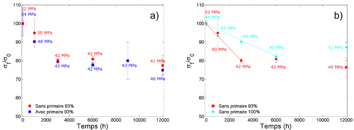
Figure 3:12 : Influence du primaire sur des éprouvettes réticulées à 93% avec (■) et sans (●) primaire (a) et influence du taux de réticulation (■) 93% et (▲) 100% (b).
