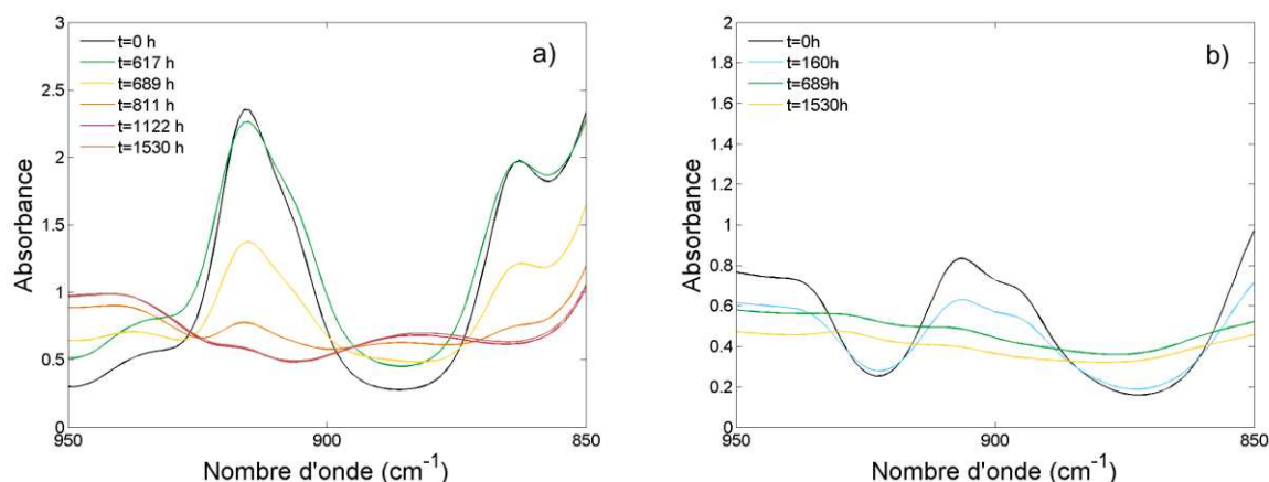
Figure 4:38 : Spectres FTIR des monomères à 120°C dans la gamme 950-850 cm -1 a) DGEBA b) TGMDA
