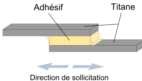
Figure 2:8: Schéma d'une éprouvette de cisaillement simple.
