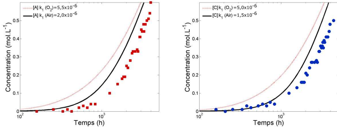
Figure 4:28: Comparaison des simulations (trait) avec les données expérimentales (■ pour les amides, et ● pour les carbonyles) de DGEBA-DDS à 120°C sous 2 MPa et sous air.
