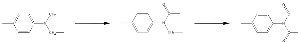
Figure 4:19: Voie possible de formation des imides à des temps longs d'exposition ou à haute température.
