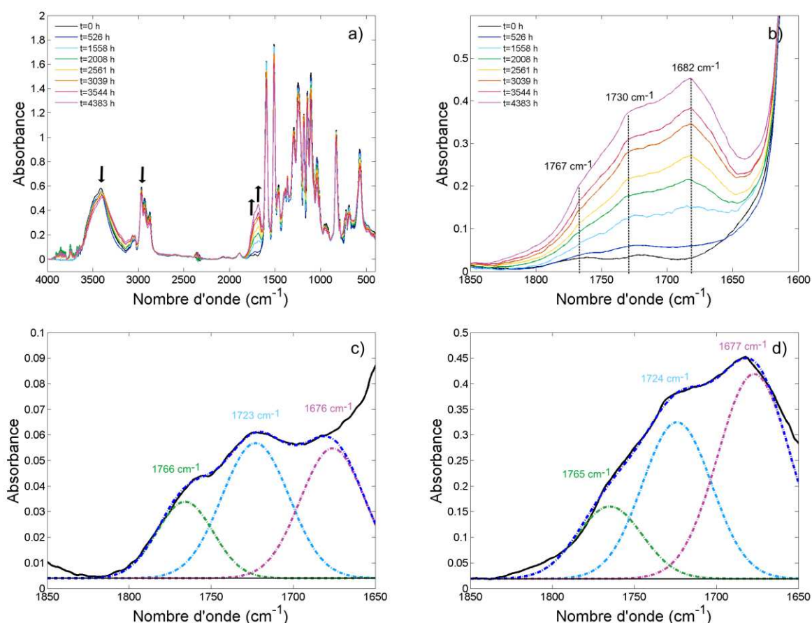
Figure 4:3: Spectres FTIR de DGEBA-DDS sous air à 120^{\circ}\text{C} a) Dans la gamme 4000-400\text{ cm}^{-1} b) Dans la gamme 1850-1600\text{ cm}^{-1} . Spectres déconvolués après c) 526 h d) 4383 h d'exposition.
