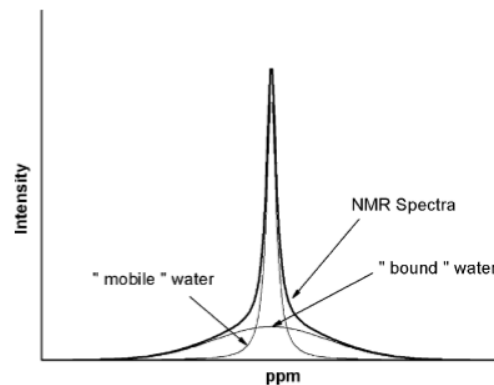
Figure 1:18: Décomposition d'un pic RMN ^2\text{H} : la base large correspond au signal de l'eau liée, et le pic étroit au signal des molécules d'eau libres[104].
