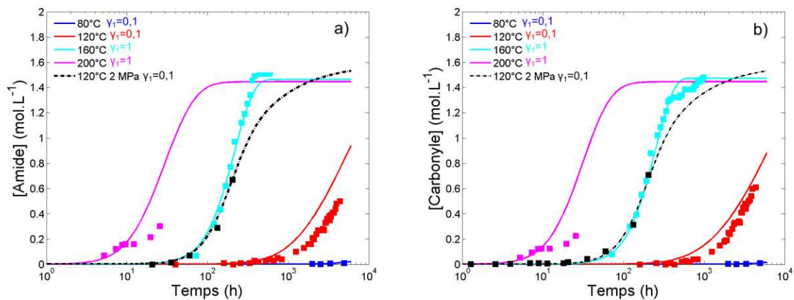
Figure 4.30 : Comparaison des simulations avec les données expérimentales (points) pour les réseaux TGMDA-DDS et DGEBA-DDS sous air et sous excès d'oxygène (2 MPa) à 120°C a) Amides b) Carbonyles.
