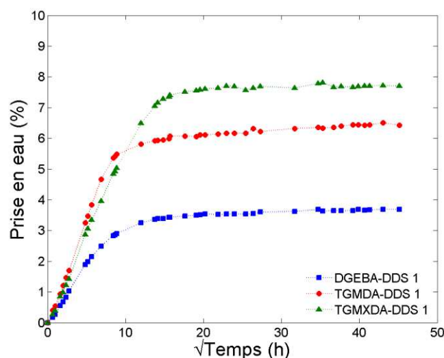
Figure 5:6: Courbes de sorptions des systèmes binaires modèles en immersion dans l'eau à 70°C.
