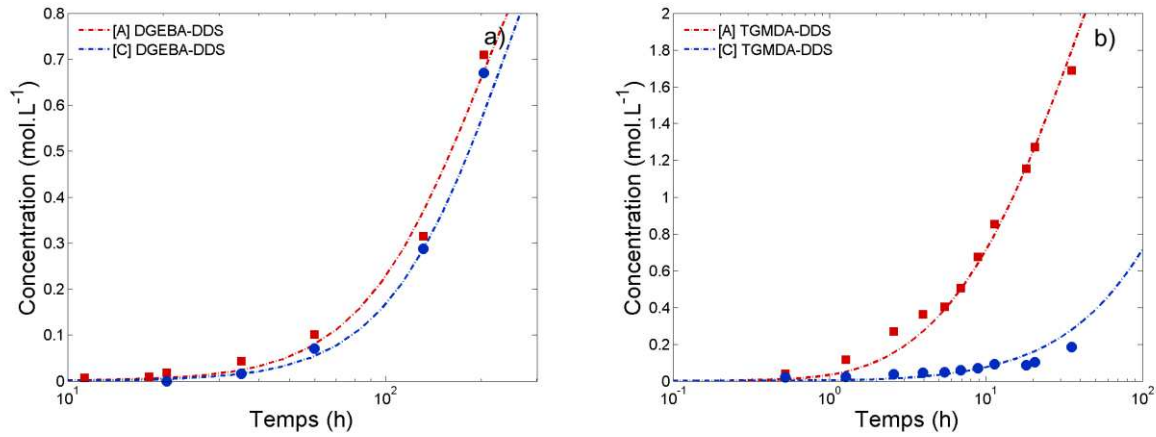
Figure 4:27 : Comparaison des simulations (trait) avec les données expérimentales (■ pour les amides et ● pour les carbonyles) sous 2 MPa d'oxygène pour a) DGEBA-DDS et b) TGMDA-DDS.
