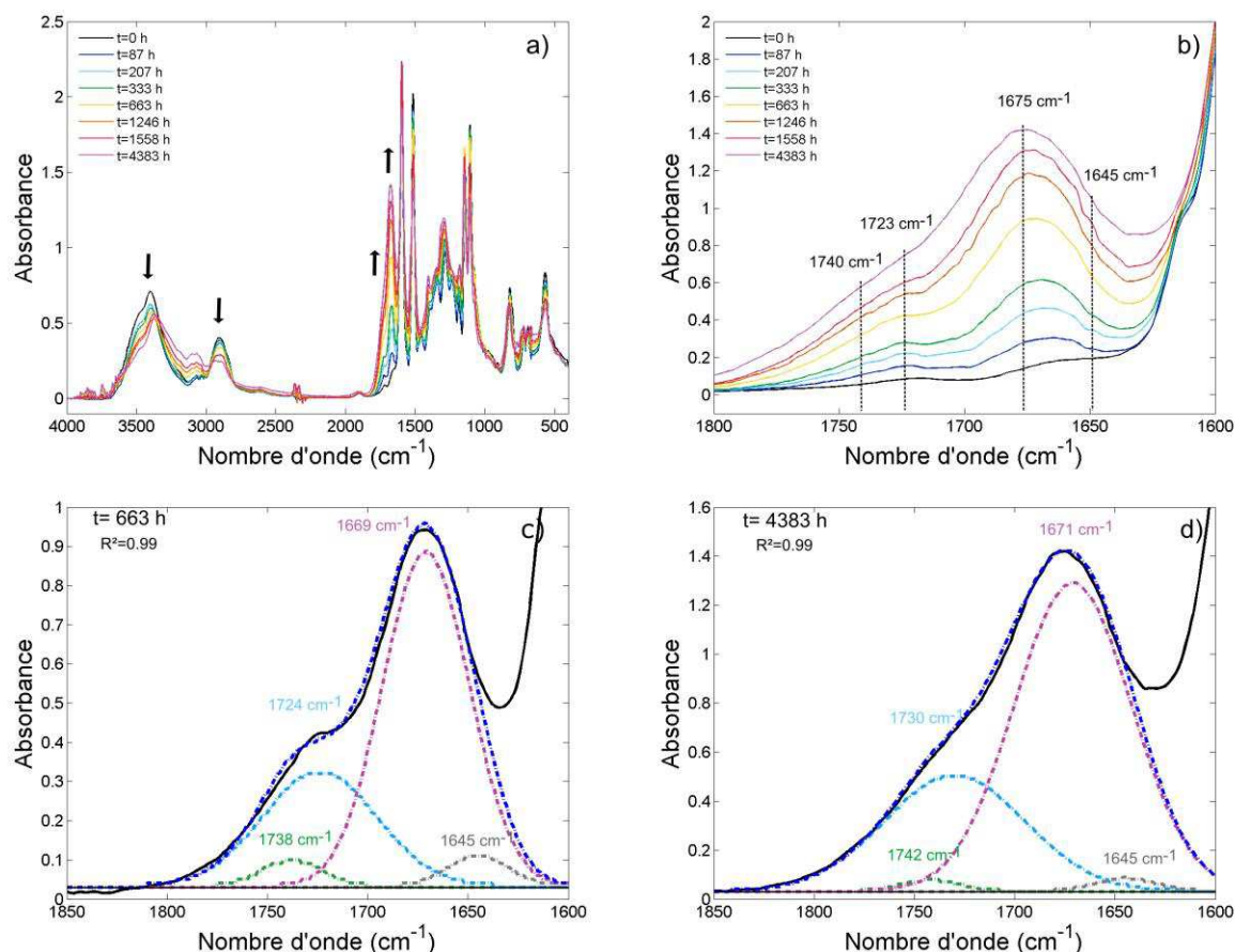
Figure 4.5: Spectres FTIR de TGMDA-DDS sous air à 120°C a) Dans la gamme 4000-400 \text{cm}^{-1} b) Dans la gamme 1850-1600 \text{cm}^{-1} . Spectres déconvolués après c) 663 h d'exposition d) 4383 h d'exposition.
