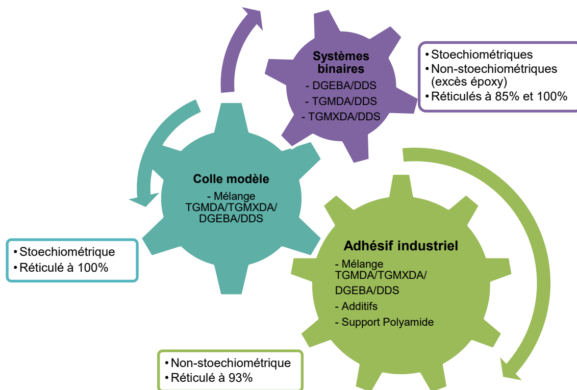
Figure 2:2 : Stratégie d'étude et présentation des principaux matériaux d'étude.
