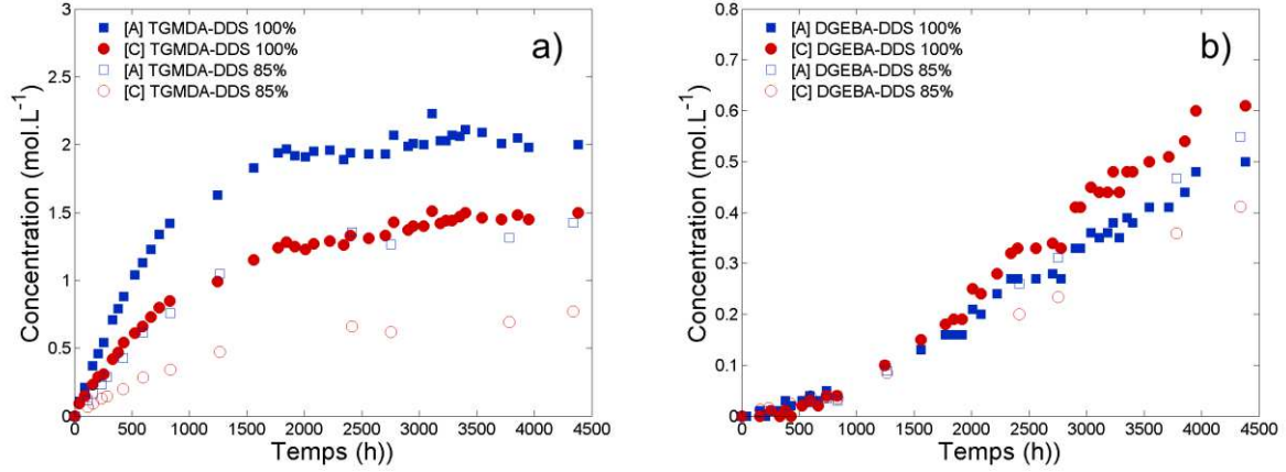
Figure 3:27: Evolution de la formation de carbonyles [C] et amides [A] en fonction du taux de réticulation (85% et 100%) a) TGMDA-DDS b) DGEBA-DDS.
