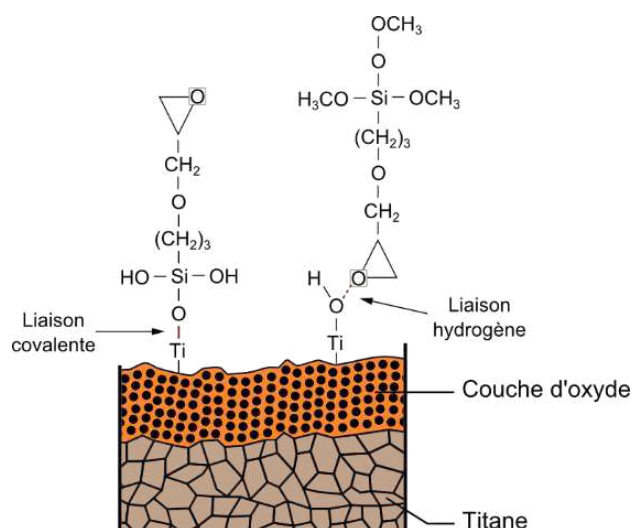
Figure 1:6: Chimisorption du primaire à la surface de l'oxyde soit par liaisons covalentes ou liaisons hydrogènes.
