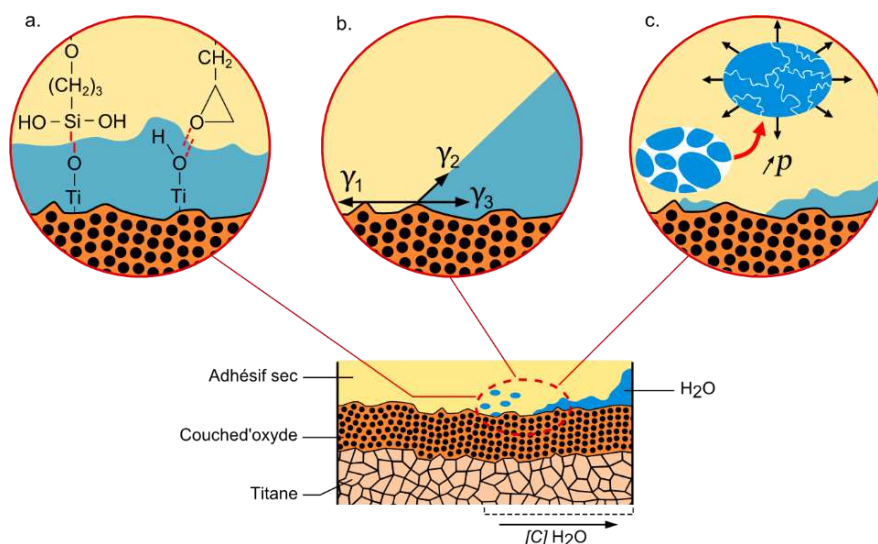
Figure 1:21: Mécanismes d'endommagement des interfaces Métal/Adhésif : a) Dégradation chimique b) Diffusion capillaire c) Augmentation de la pression osmotique et formation de larges vacuoles.
