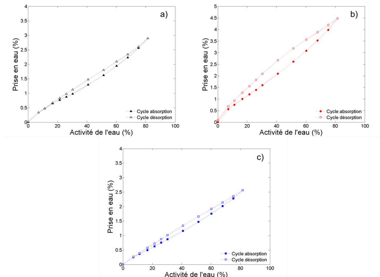
Figure A1:2 : Evolution de la quantité d'eau à l'équilibre à 70°C lors d'un cycle d'absorption et de désorption pour a) l'adhésif b) TGMDA-DDS et c) DGEBA-DDS.
