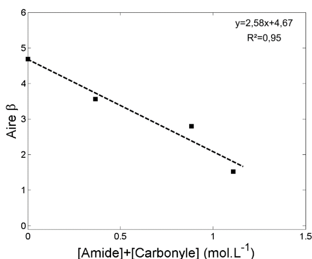
Figure 4:1: Corrélation entre la concentration en produits d'oxydation et la diminution de la relaxation \beta dans l'adhésif industriel.
