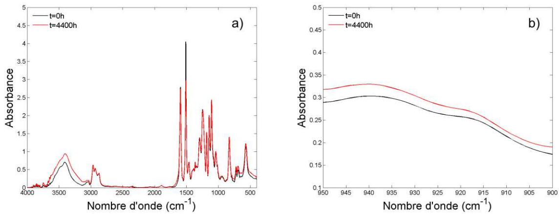
Figure 5:8: Spectres FTIR de DGEBA-DDS 1.2 avant et après 4400 h en immersion dans l'eau à 70°C a) dans la gamme 4000\text{-}400\text{ cm}^{-1} b) 950\text{-}900\text{ cm}^{-1} .
