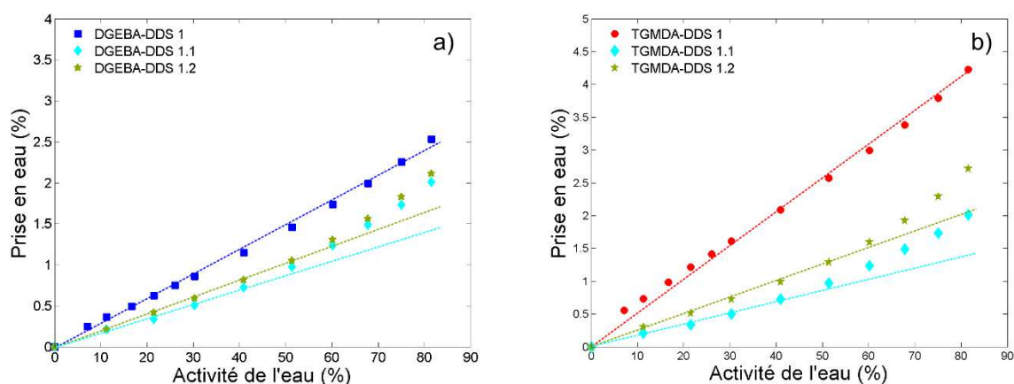
Figure 5:9: Evolution de la quantité d'eau à l'équilibre à 70°C en fonction de l'activité de l'eau et de la stœchiométrie pour les systèmes modèles a) DGEBA-DDS et b) TGMDA-DDS.
