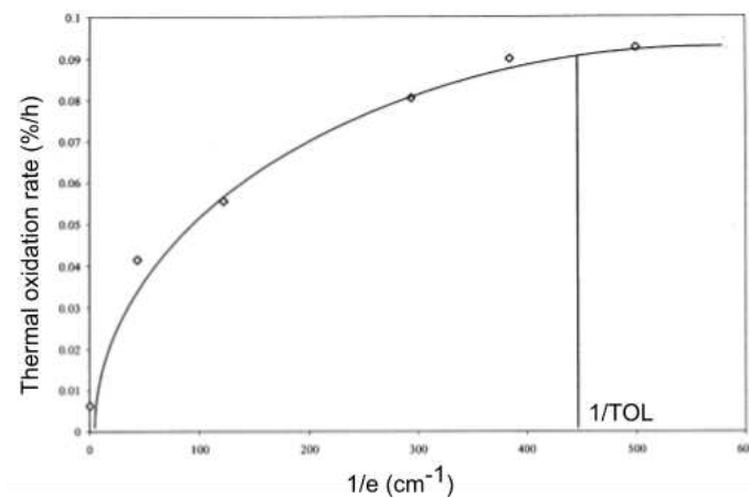
Figure 1:33: Vitesse d'oxydation en fonction de l'inverse de l'épaisseur dans un réseau époxy/amine[152].
