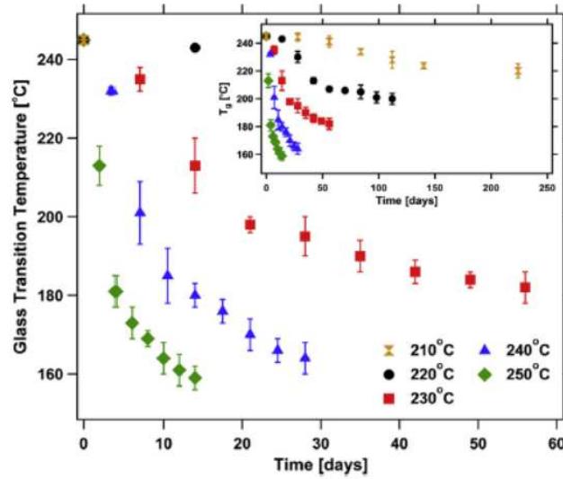
Figure 1:31: Variation de la température de transition vitreuse d'un réseau EPON828-1031/DDS, mesurée par DMA, sous air à 210, 220, 230, 240 et 250°C[172].
