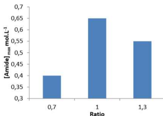
Figure 1:28: Histogramme comparant les concentrations maximales des amides pour différentes stœchiométries (avec R=[A]/[E] ) pour des films époxy/amine à 110°C sur 2500h[39].
