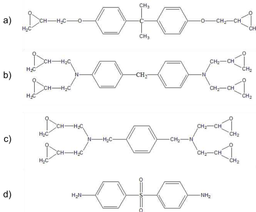
Figure 2:3: Structure des monomères utilisés dans la formulation des systèmes modèles a) DGEBA b) TGMMDA c) TGMXDA d) DDS.
