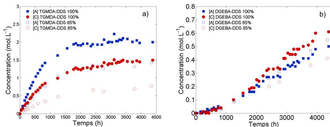
Figure 4:37 : Evolution de la formation de carbonyles [C] et amides [A] en fonction du taux de réticulation (85% et 100%) a) TGMDA-DDS b) DGEBA-DDS
