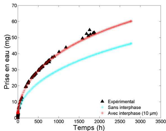
Figure 5:5: Simulation de la cinétique d'eau absorbée par l'assemblage avec une diffusion à l'interface 100 fois plus rapide.
