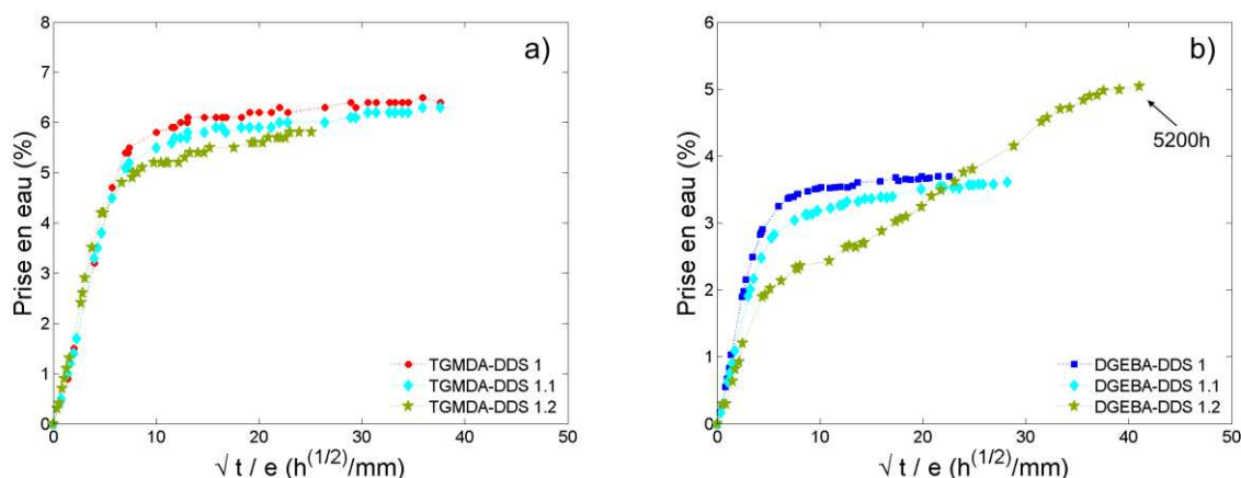
Figure 5:7: Courbes de sorptions des réseaux DGEBA-DDS et TGMDA-DDS stœchiométriques et non-stœchiométriques à 70°C en immersion dans l'eau.
