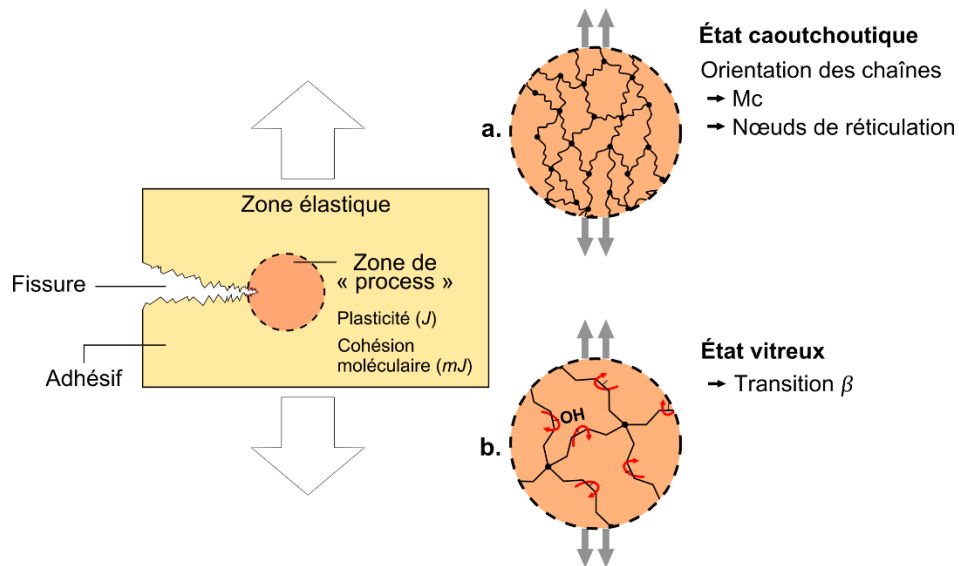
Figure 3:23: Schéma récapitulatif du modèle de plasticité confinée de type Dugdale[54] avec les différents paramètres clés a) à l'état caoutchoutique b) à l'état vitreux.
