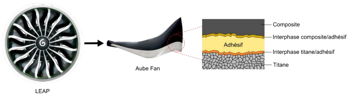
Figure 1:1 : Composition de l'aube FAN.
