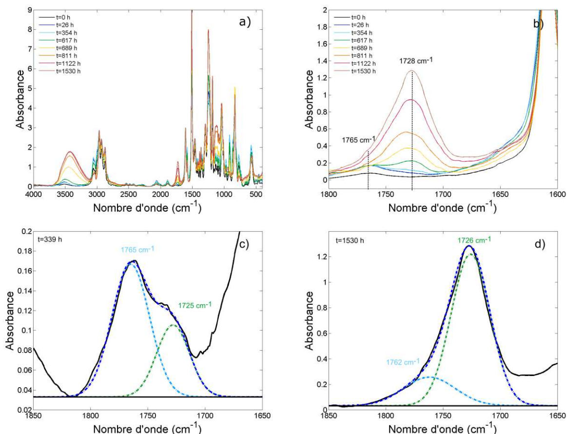
Figure 4:10 : Spectres FTIR du monomère DGEBA sous air à 120^{\circ}\text{C} a) Dans la gamme 4000-400\text{ cm}^{-1} b) Dans la gamme 1850-1600\text{ cm}^{-1} . Spectres déconvolués après c) 339 h d'exposition d) 1530 h d'exposition.
