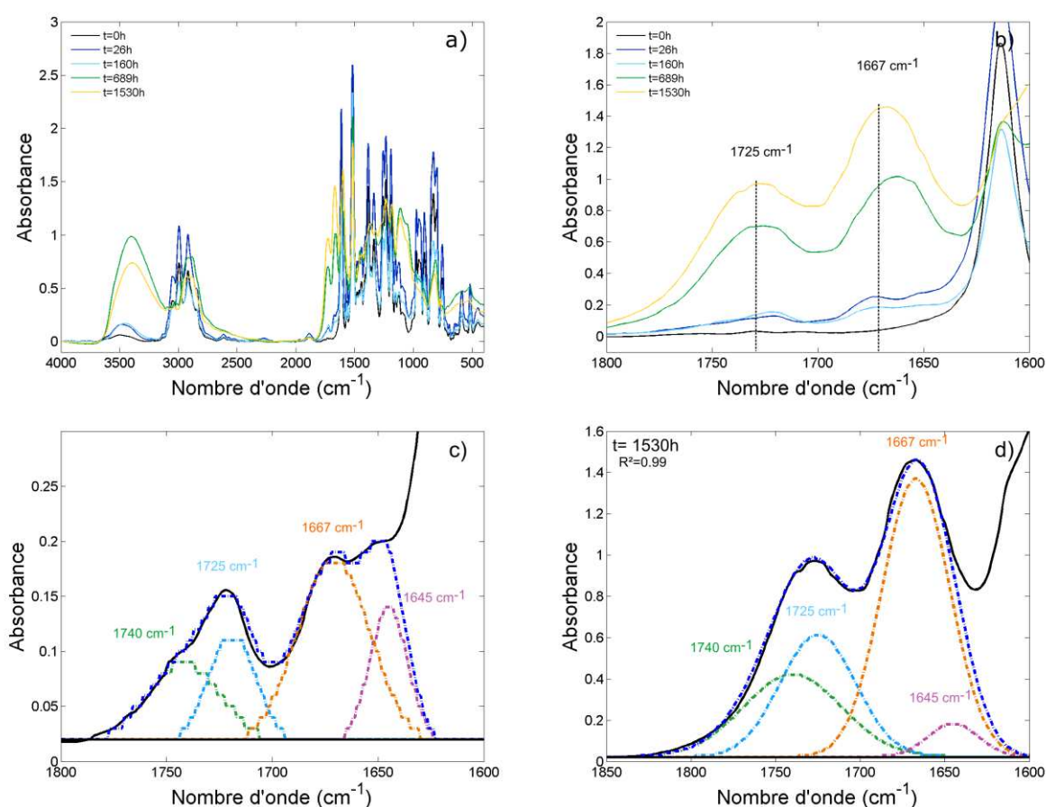
Figure 4:6 : Spectres FTIR du monomère TGMDA sous air à 120°C a) Dans la gamme 4000-400 cm^{-1} b) Dans la gamme 1850-1600 cm^{-1} . Spectres déconvolués après c) 160 h d'exposition d) 1530 h d'exposition.
