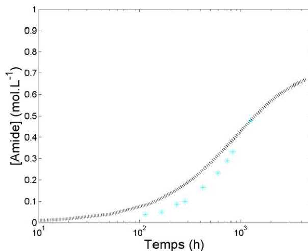
Figure 4.36 : Comparaison entre la modélisation et les données expérimentales à 120°C pour les amides de la colle modèle [PH] = 1,6 \text{ mol.L}^{-1} .
