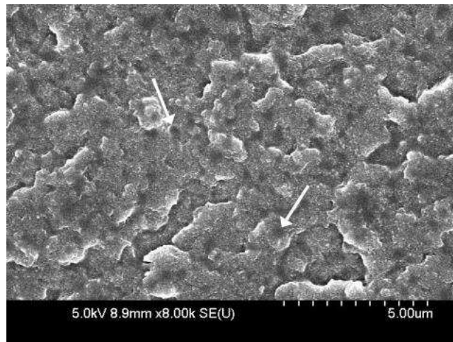
Figure 3:29: Observations MEB de la séparation de phase entre la matrice époxy et les additifs présents sous forme de particules (~ 500nm).
