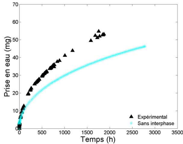
Figure 5:4: Simulation de la cinétique d'eau absorbée par l'assemblage en négligeant la diffusion interfaciale.
