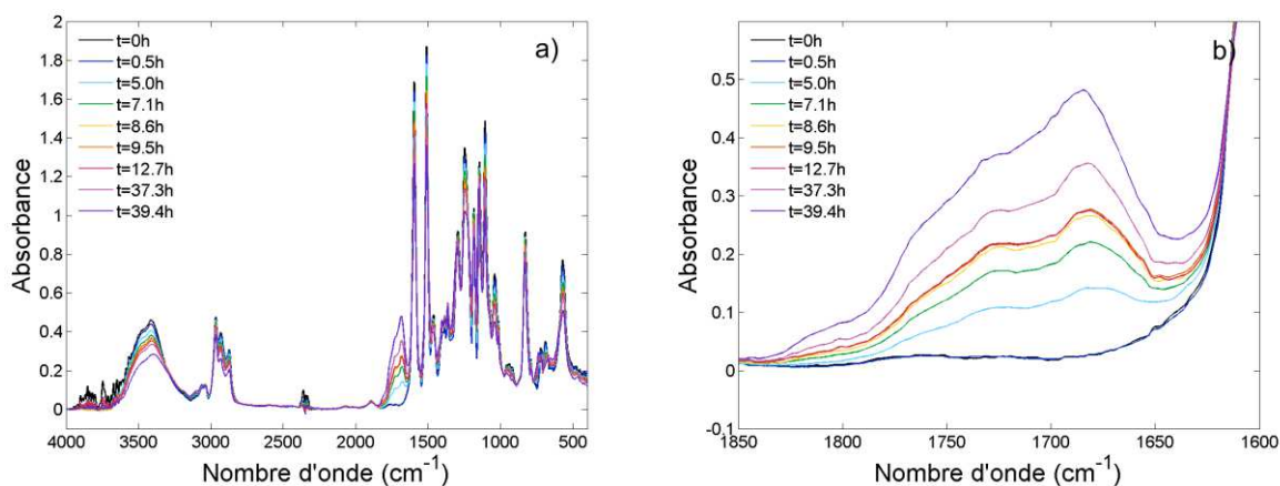
Figure 4.4 : Spectres FTIR de DGEBA-DDS sous air à 200°C a) Dans la gamme 4000-400 \text{cm}^{-1} b) Dans la gamme 1850-1600 \text{cm}^{-1} .
