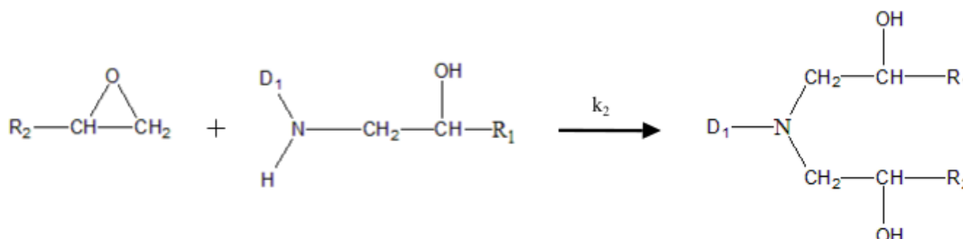
Figure 1:11: Réaction entre une amine secondaire et une fonction époxyde.
