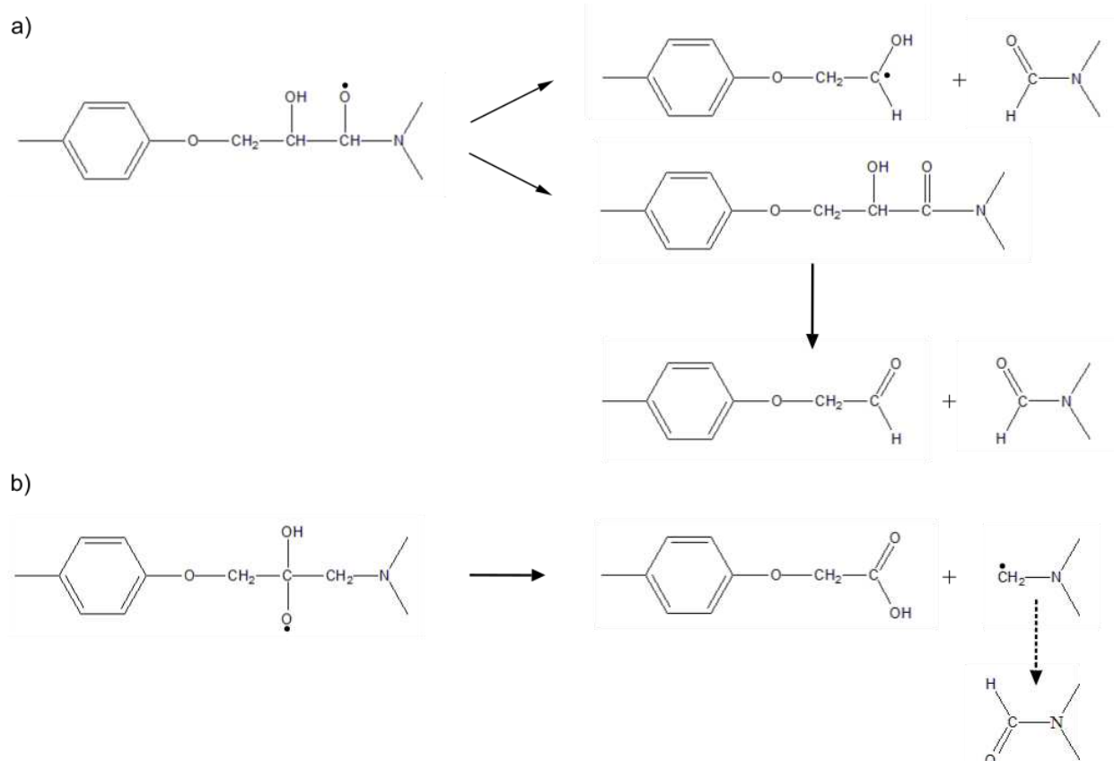
Figure 4:18: Voies possible de formation des dérivés amides par l'attaque des méthylènes en position \alpha (a) ou \beta (b) de l'azote.
