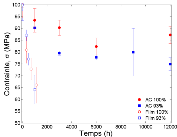
Figure 3:16: Comparaison des évolutions des contraintes à rupture entre les assemblages collés (AC) et les tractions sur adhésif.
