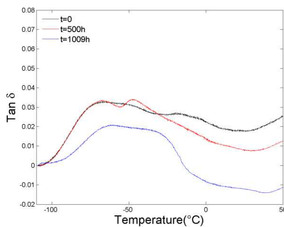
Figure 3:22: Evolution de la relaxation \beta de l'adhésif avec le support polyamide réticulé à 93% au cours d'un vieillissement thermique à 120°C.
