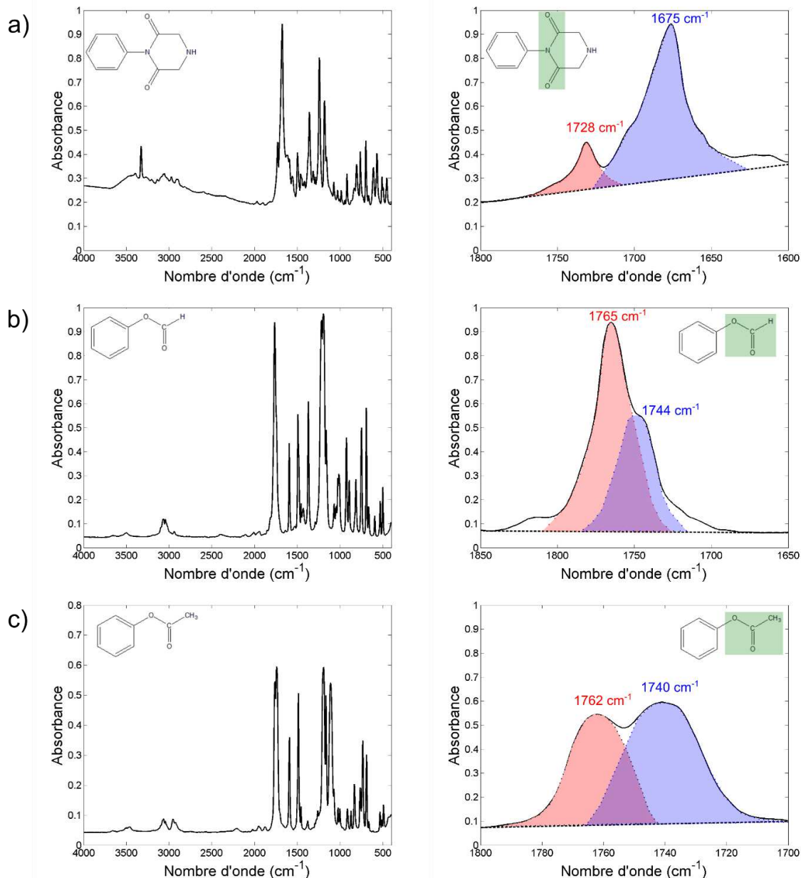
Figure 2:12: FTIR des molécules modèles et détermination des nombres d'onde caractéristiques a) Imide b) Formate de phényle c) Acétate de phényle.
