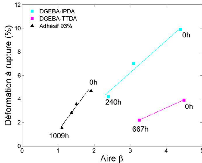
Figure 3:25: Evolution de l'aire sous \beta au cours d'un vieillissement thermique.
