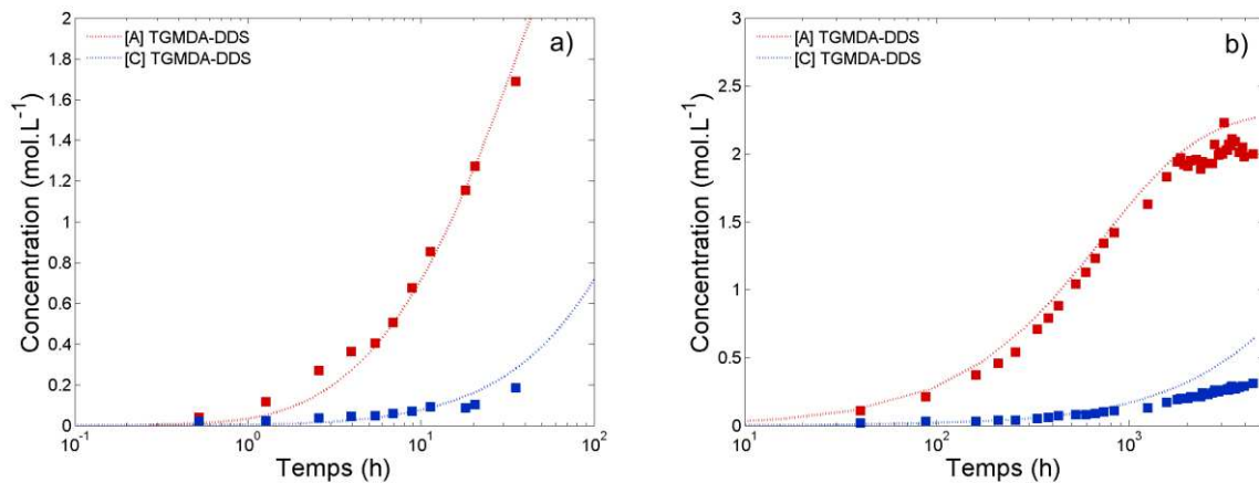
Figure 4:29: Comparaison des simulations (trait) avec les données expérimentales (■ pour les amides et ■ pour les carbonyles) de TGMDA-DDS à 120°C avec les constantes de vitesse k_1 déterminées sous pression d'oxygène a) sous 2 MPa d'oxygène et b) sous air.
