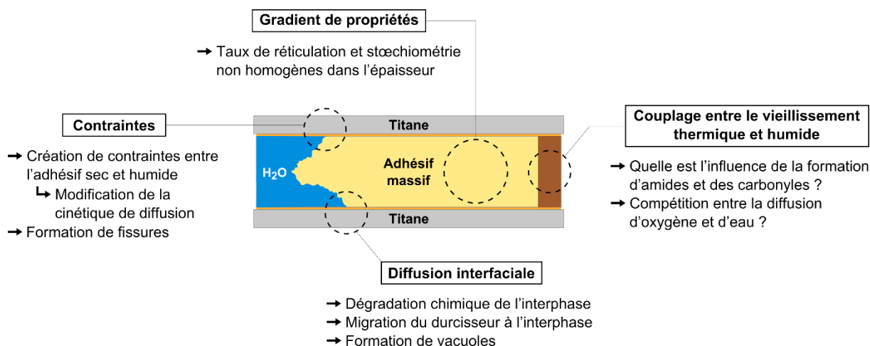
Figure 5:1:Principaux verrous de la modélisation du vieillissement humide au sein des assemblages collés.
