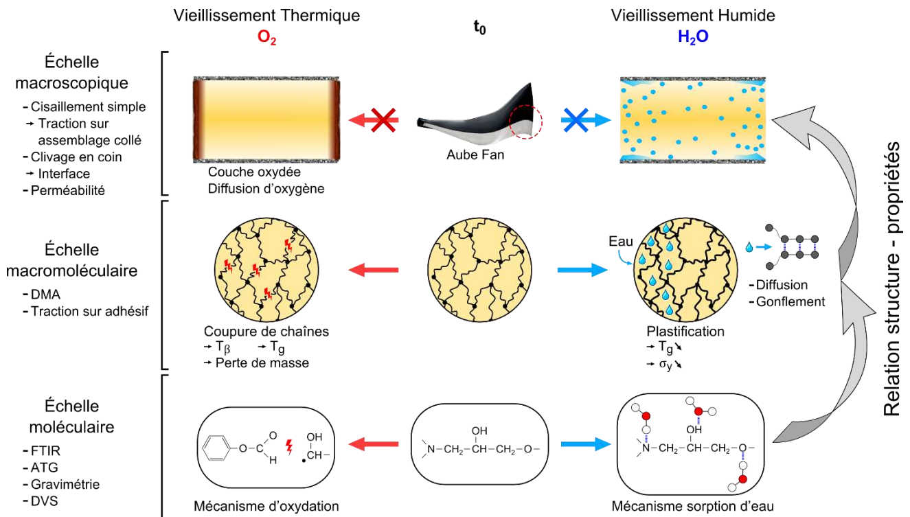
Figure 2:1: Approche multi-échelle pour la prédiction de la durée de vie des assemblages collés et les principales techniques expérimentales associées.
