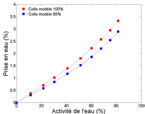
Figure 5.10: Evolution de la quantité d'eau à l'équilibre à 70°C en fonction de l'activité de l'eau pour la colle modèle réticulée à 100% (■) et 85% (■).
