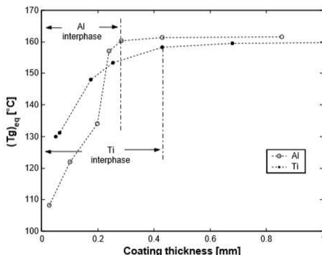
Figure 1:5 : Variation de la température de transition vitreuse en fonction de la distance du métal pour Aluminium et le Titane[27].
