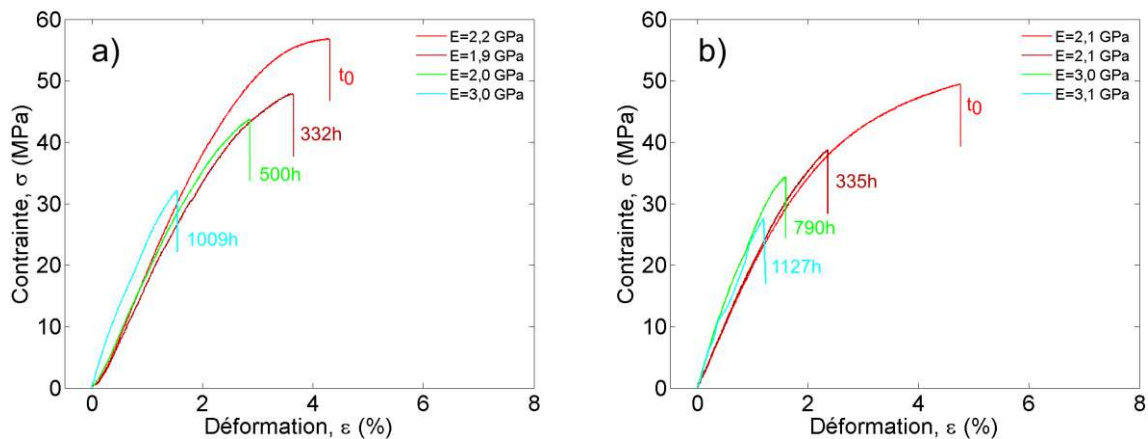
Figure 3:14: Evolution des courbes de traction a) Adhésif réticulé à 93% b) Adhésif réticulé à 100%.
