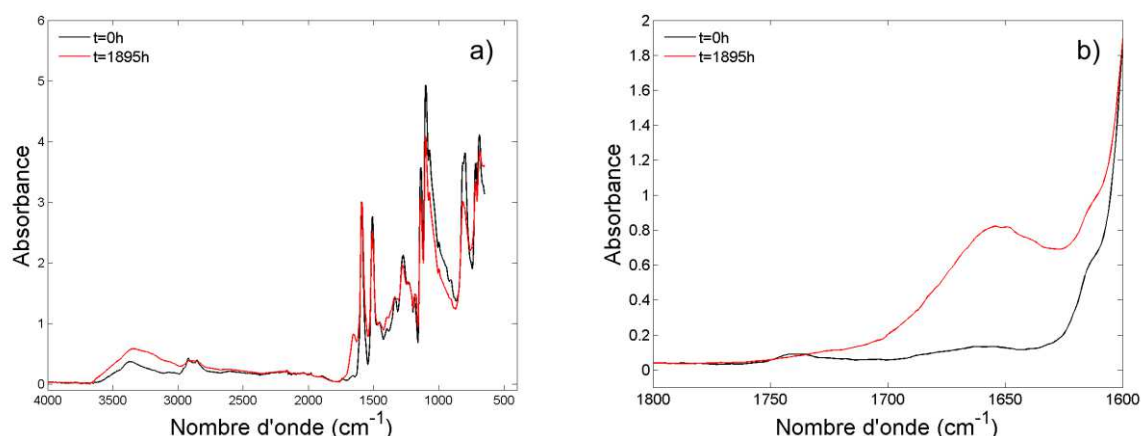
Figure A2:2 : Spectres FTIR de TGMDA-DDS avant et après 1895h en immersion dans l'eau à 70°C a) dans la gamme 4000-400 \text{cm}^{-1} b) 1800-1600 \text{cm}^{-1} .
