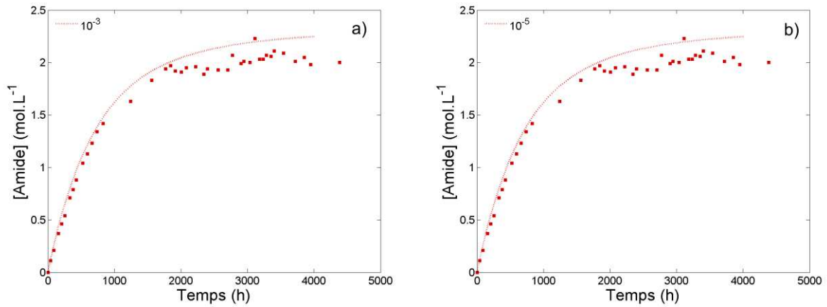
Figure 4:24: Influence de la concentration initiale en POOH : a) [POOH] = 10^{-3} \text{ mol.L}^{-1} b) [POOH] = 10^{-5} \text{ mol.L}^{-1} .
