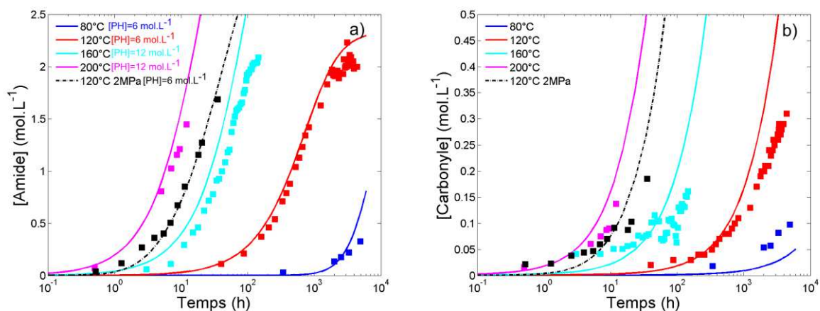
Figure 4:32: Comparaison entre les modélisations et les données expérimentales à 80°C, 120°C, 160°C, et 200°C pour TGMDA-DDS a) amides b) carbonyles.
