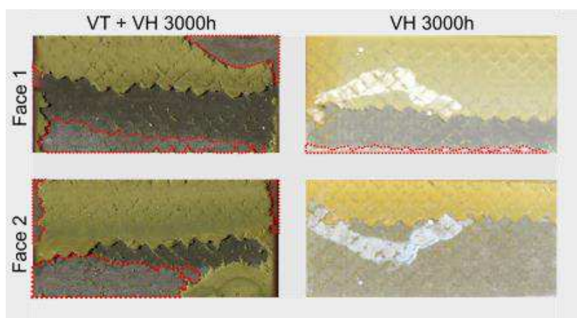
Figure A2:6 : Faciès de rupture des éprouvettes de cisaillement simple vieilles à gauche 3000h à 120°C puis 3000h à 70°C et 85% d’humidité et à droite 3000h à 70°C et 85% d’humidité. Les zones de ruptures adhésives sont entourées en rouge.
