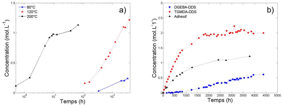
Figure 3:9 : a) Influence de la température sur les cinétiques de formation des amides pour l'adhésif industriel à 80, 120 et 200°C. b) Comparaison de la concentration en amide à 120°C pour TGMDA-DDS (●), DGEBA-DDS (■) et l'adhésif (▲).
