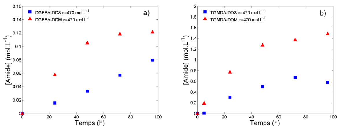
Figure 4:7: Evolution des concentrations en amides pour les réseaux (a) DGEBA-DDS et DGEBA-DDM (b) TGMDA-DDS et TGMDA-DDM sous air à 160^\circ\text{C} .
