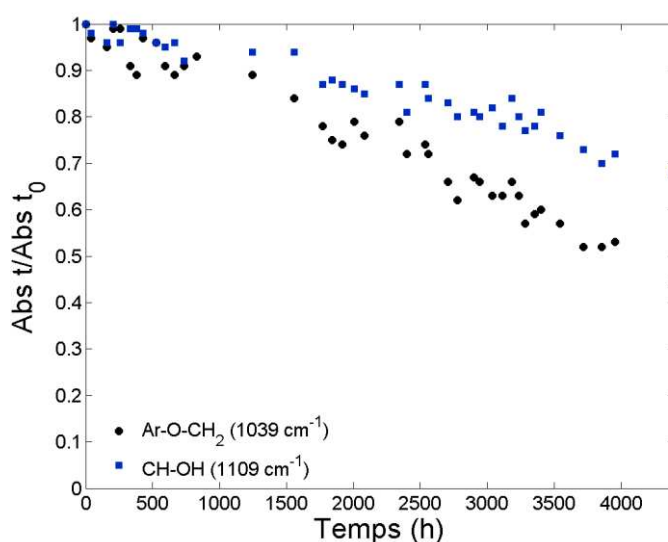
Figure 4:11 : Absorbance relative de la liaison éther et alcool au cours du temps à 120°C dans le réseau DGEBA-DDS.
