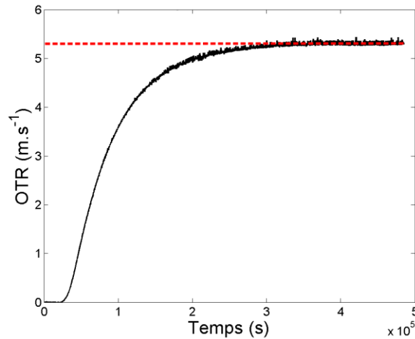
Figure 2:14: Mesure de l'OTR en fonction du temps pour un film d'adhésif industriel à 23°C.
