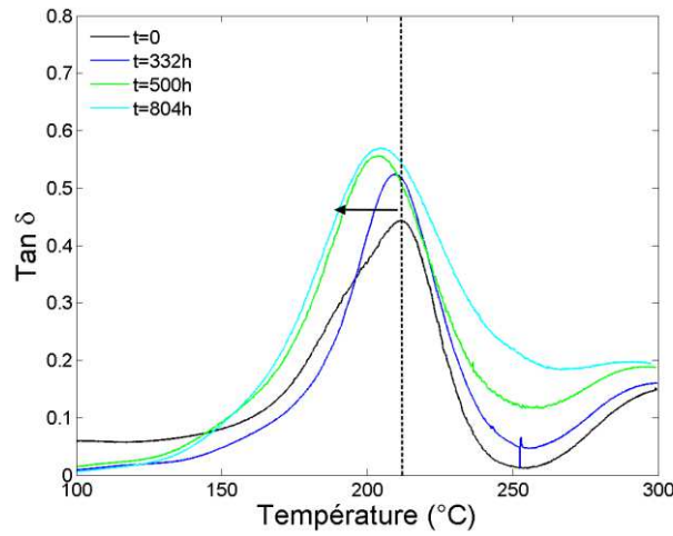
Figure 3:19: Evolution de T_g pour l'adhésif réticulé à 93% lors d'un vieillissement à 120°C.
