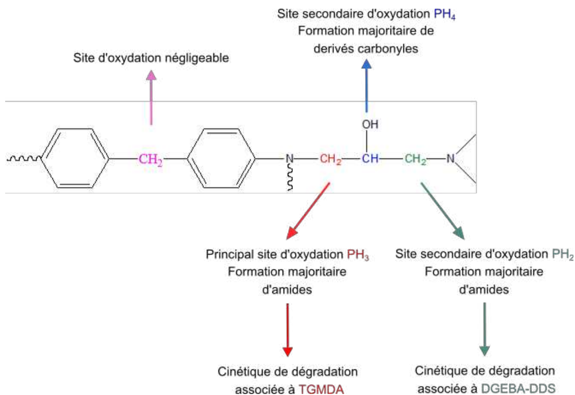
Figure 4:22: Stratégie d'étude pour la modélisation de TGMDA-DDS à 120°C.
