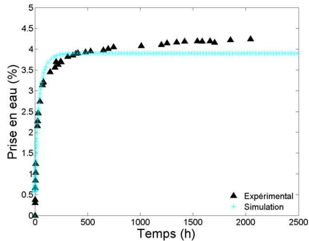
Figure 5:3: Courbe expérimentale et simulation de la courbe par Abaqus.
