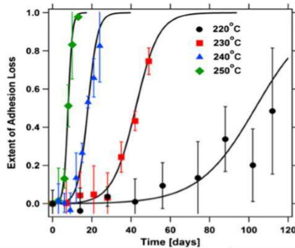
Figure 1:34: Perte d'adhésion en fonction du temps et de la température d'oxydation[181].
