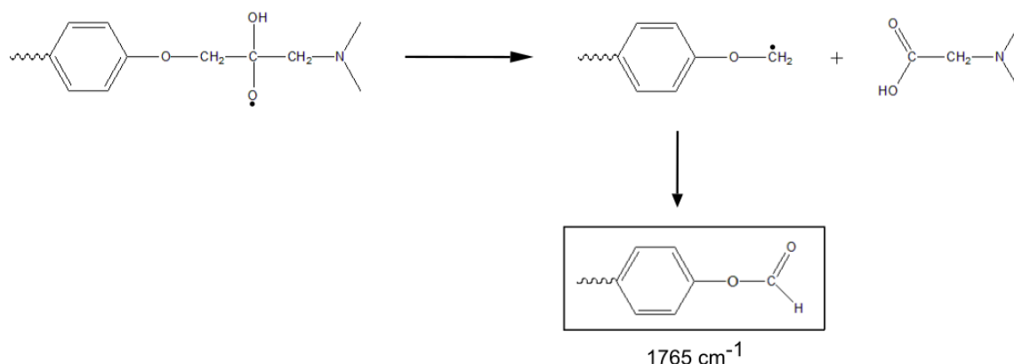
Figure 4:16: Voies possible de formation des dérivés formiates par l'attaque de l'alcoyle en position \alpha de l'alcool.
