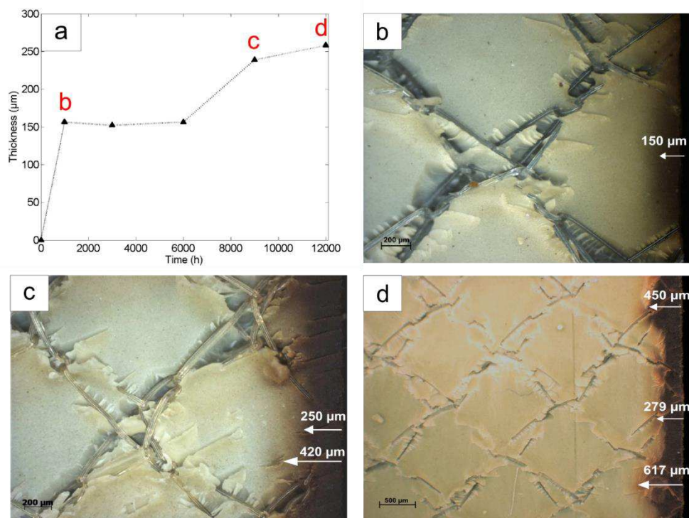
Figure 3:5 : a) Epaisseur de la couche oxydée (estimée ici comme la zone foncée) en fonction du temps de vieillissement. Observations des couches oxydées des assemblages à 120^\circ\text{C} au microscope optique après b) 1000 h c) 9000 h et d) 12000 h.
