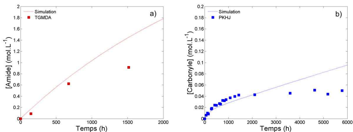
Figure 4:25: Comparaison des simulations (trait) avec les données expérimentales (■ pour TGMDA et ■ pour PKHJ) à 120°C sous air.
