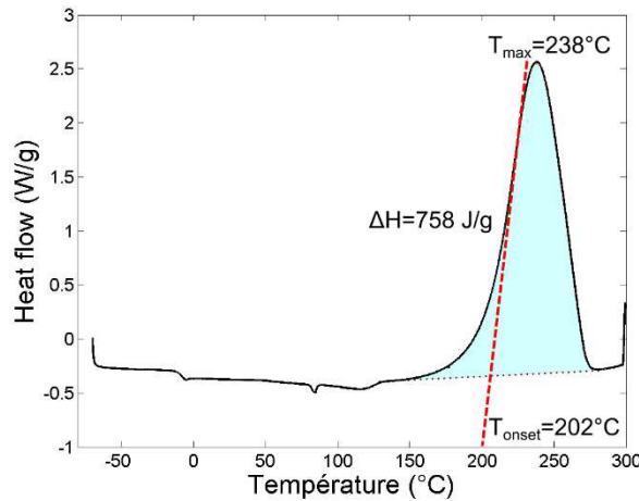
Figure 2:5 : Exemple de thermogramme de la réticulation du réseau TGMDA-DDS à 10^{\circ}\text{C}.\text{min}^{-1} de -80^{\circ}\text{C} à 300^{\circ}\text{C} sous azote.
