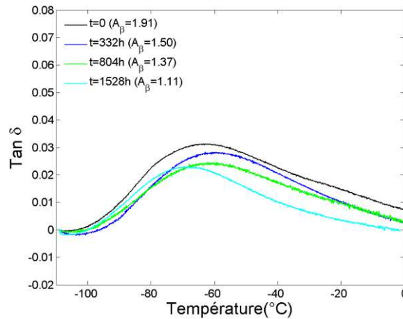
Figure 3:21: Evolution de la relaxation \beta de l'adhésif réticulé à 93% au cours d'un vieillissement thermique à 120°C.
