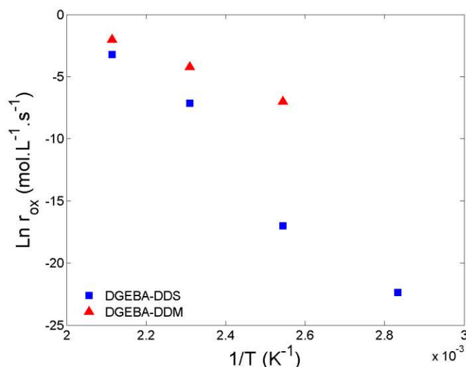
Figure 4:14: Diagramme d'Arrhenius pour la formation des amides dans la gamme de température de 120°C à 200°C pour DGEBA-DDS (■) et DGEBA-DDM (▲).
