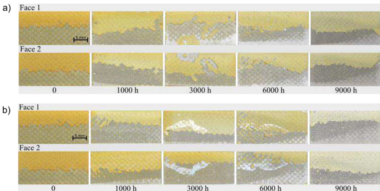
Figure 3:4 : Observations par microscopie optique des faciès de rupture des éprouvettes de cisaillement simple a) avec primaire b) sans primaire après un vieillissement humide à 70°C et 85% de taux d'humidité relative.
