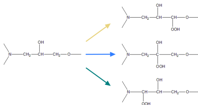
Figure 1:22: Formations possibles des hydroperoxydes dans les réseaux époxy/amine[145].
