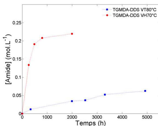
Figure A2:3: Cinétique de formation des amides pour le système TGMDA-DDS à 80^{\circ}\text{C} (■) et à 70^{\circ}\text{C} en immersion dans l'eau (●).
