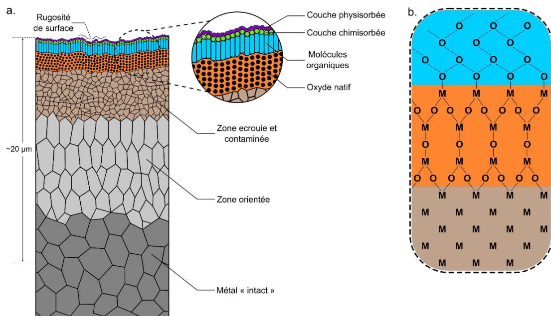
Figure 1:4: a) Composition et microstructure d'une surface métallique b) Composition chimique des couches superficielles.
