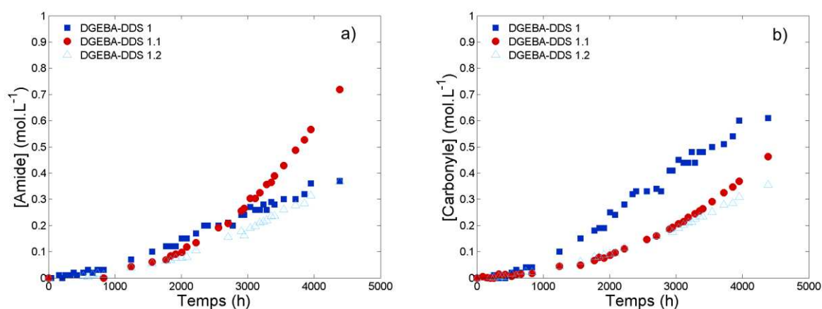
Figure 4:39: Influence de la stœchiométrie sur les cinétiques de formation de DGEBA-DDS a) Amides b) Carbonyles
