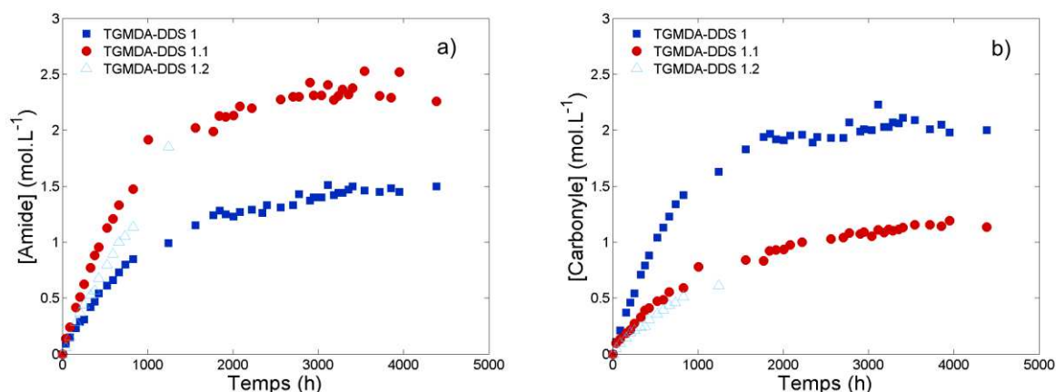
Figure 4:40: Influence de la stœchiométrie sur les vitesses de formation des a) Amides b) Carbonyles
