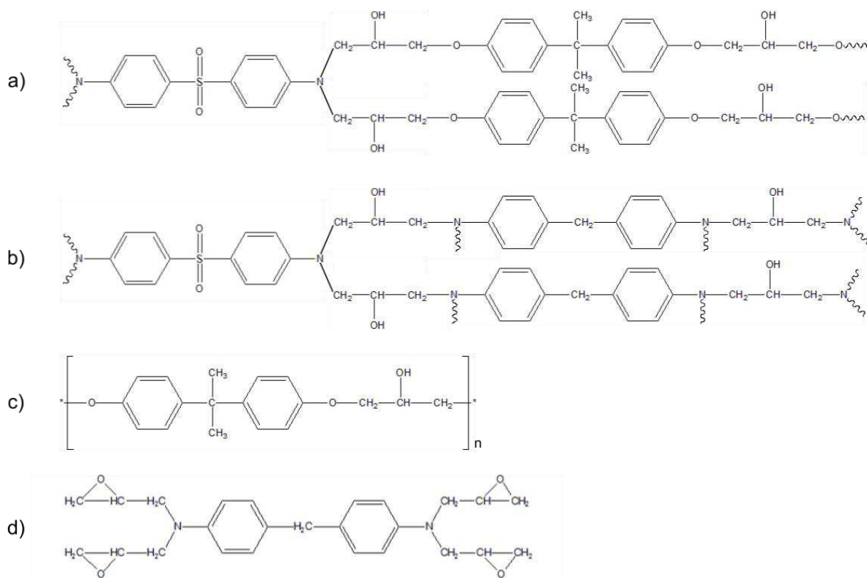
Figure 4.2: Structures des différents systèmes étudiés a) DGEBA-DDS, b) TGMDA-DDS, c) PKHJ, d) TGMDA.
