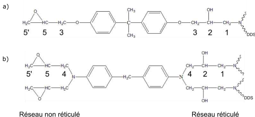
Figure 3:28: Sites oxydables dans les réseaux a) DGEBA-DDS b) TGMDA-DDS suivant le taux de réticulation
