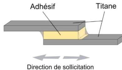
Figure 1:16: Schéma d'une éprouvette de cisaillement simple.
