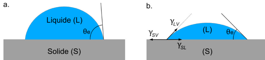
Figure 1:3 : Goutte en surface d'une surface plane dans le cas a) d'une mauvaise mouillabilité b) d'une bonne mouillabilité.
