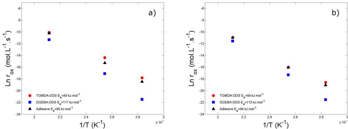
Figure 3:10: Diagramme d'Arrhenius pour la formation des produits d'oxydation amides (a) et carbonyles (b) dans la gamme de température de 80 à 200°C pour TGMDA-DDS (●), DGEBA-DDS (■) et l'adhésif (▲).
