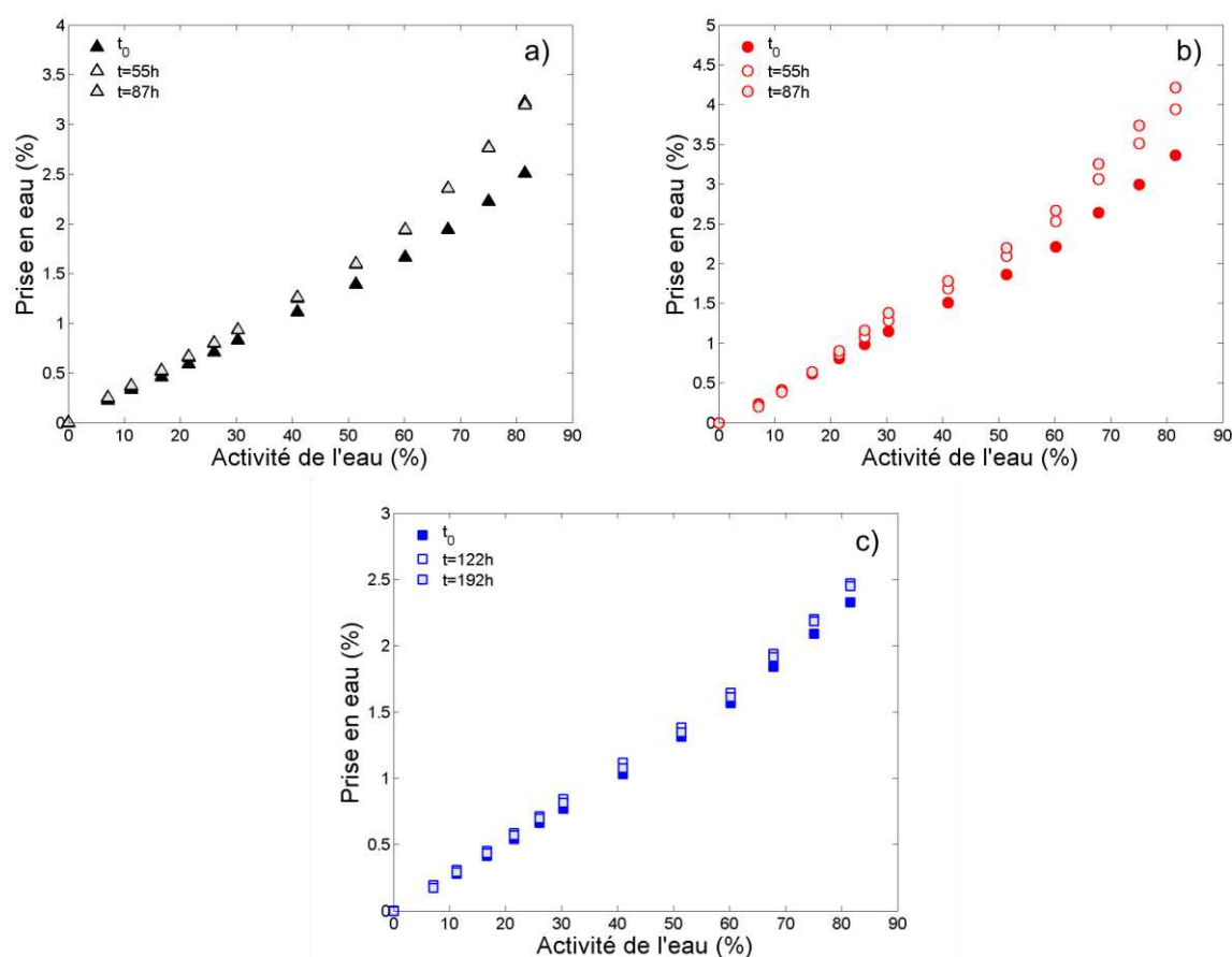
Figure 5:11: Evolution de la quantité d'eau à l'équilibre à 70°C en fonction de l'activité de l'eau et du taux d'oxydation pour a) l'adhésif b) TGMDA-DDS et b) DGEBA-DDS.
