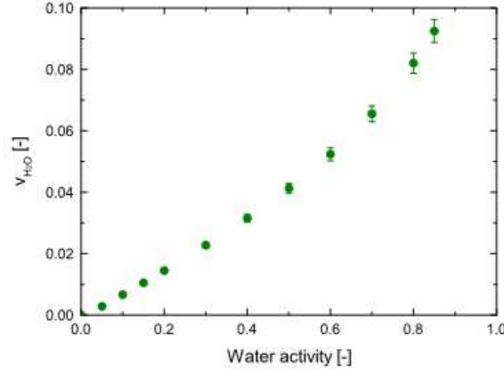
Figure 1:19: Evolution du volume d'eau en fonction de l'activité de l'eau pour le PA66 à 40°C[107].
