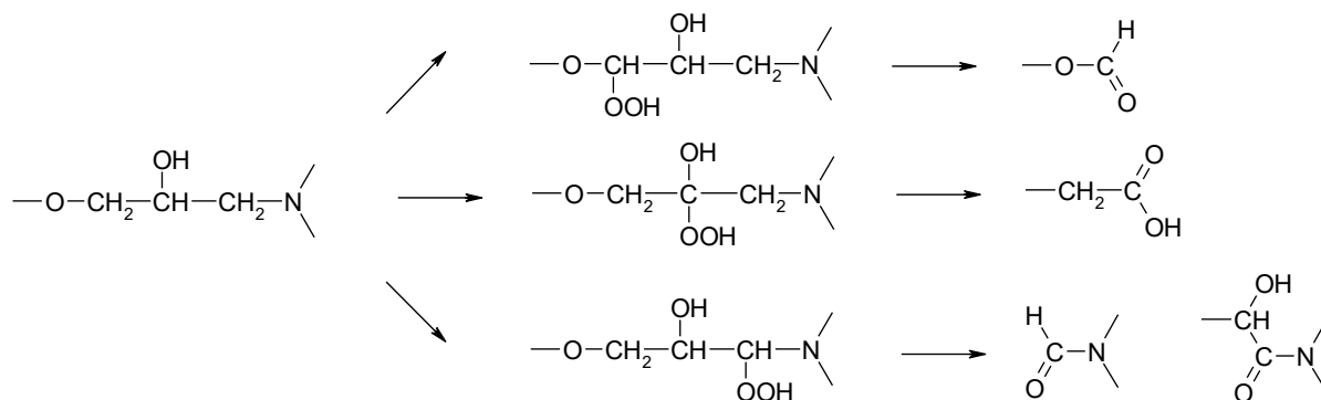
Figure 3:11 : Formation des produits d'oxydation dans les systèmes époxy/amine[9].
