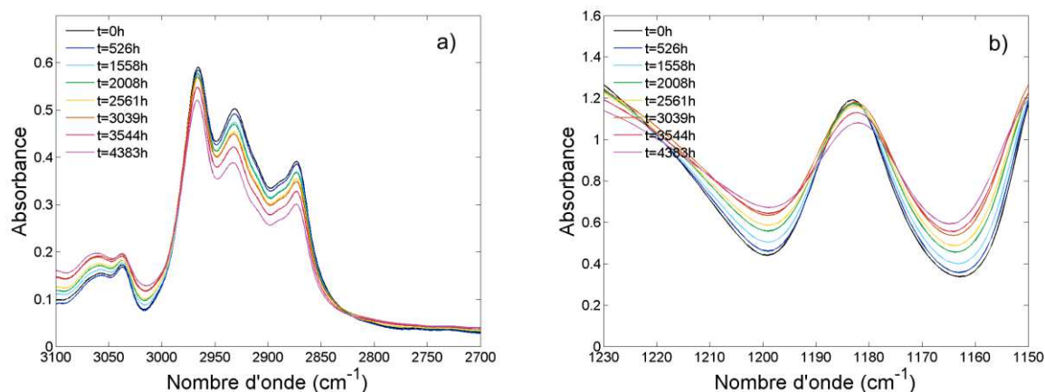
Figure 4:12 : Spectres FTIR de DGEBA-DDS sous air à 120°C a) Dans la gamme 3100-2700 cm^{-1} b) Dans la gamme 1230-1150 cm^{-1} .
