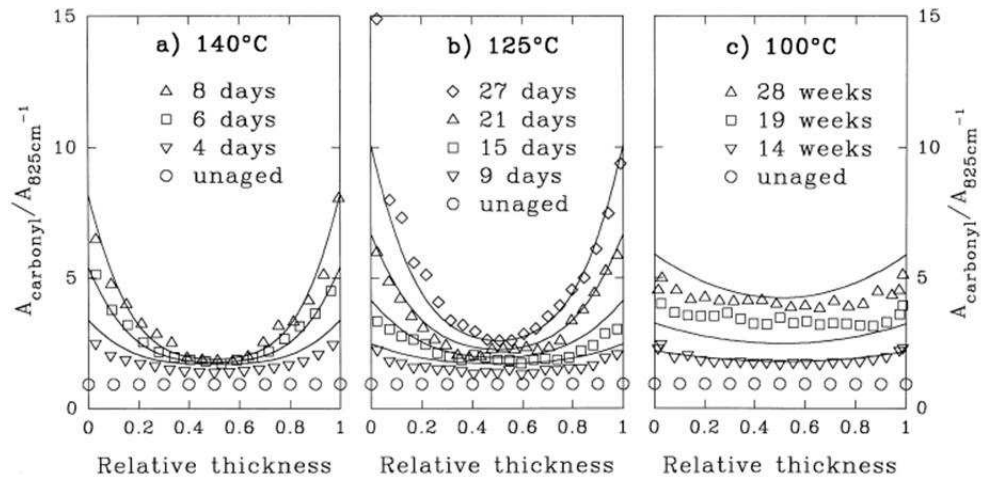
Figure 1:32: Profils des carbonyles dans le néoprène à différentes températures (a) 140°C, (b) 120°C, (c) 100°C[174].
