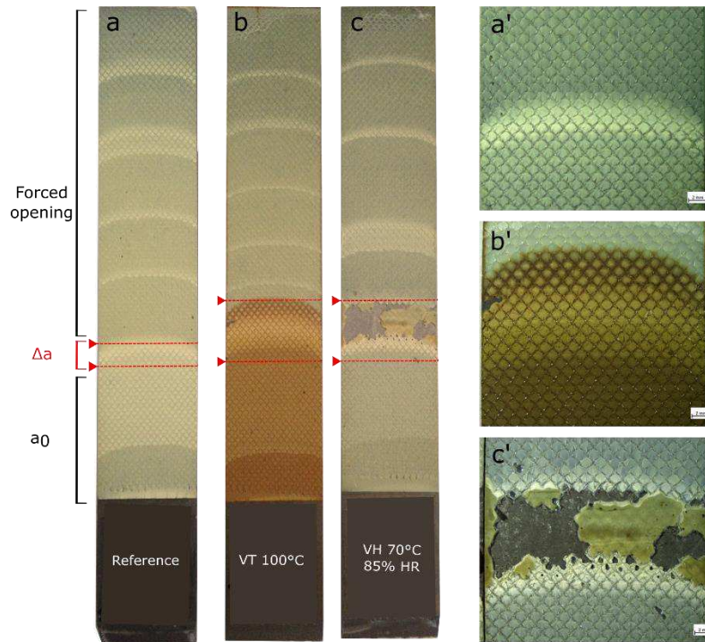
Figure 3:2 : Observation en microscopie optique des éprouvettes de clivage en coin après 3700 h de vieillissement a) Référence à 23°C et 50% d'humidité b) Vieillissement thermique à 100°C c) Vieillissement humide à 70°C et 85% d'humidité. Les flèches rouges indiquent la position de la fissure à t_0 et à la fin du vieillissement avant l'ouverture forcée. Les images a', b' et c' correspondent aux zones endommagées lors des différents vieillissements.
