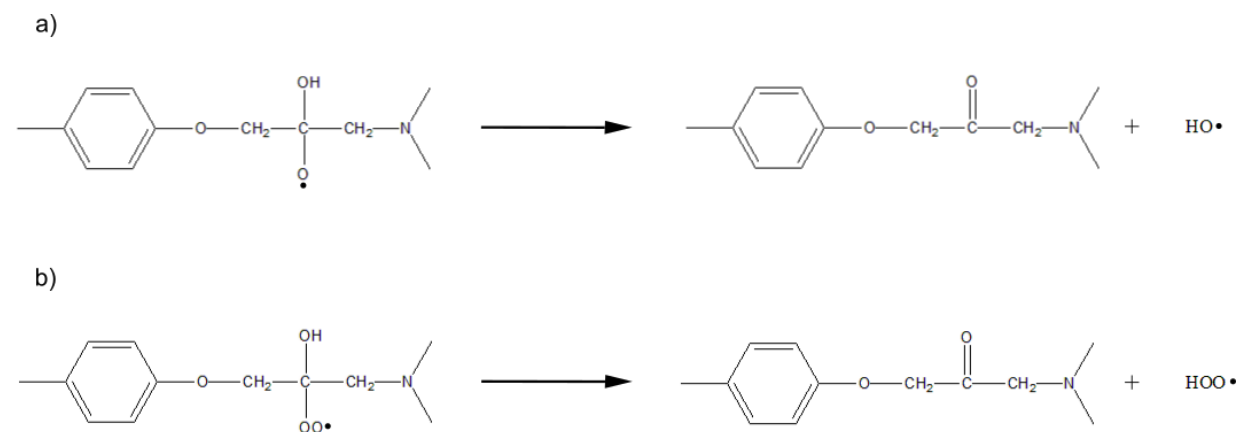
Figure 4:17: Voies possibles de formation des cétones par oxydation du méthine dans la position \alpha de l'alcool.
