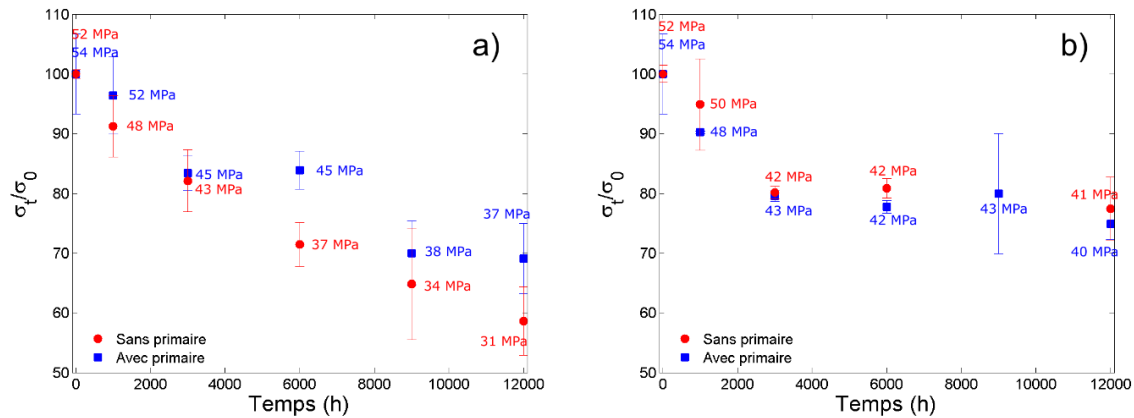
Figure 3.1: Valeurs relatives des contraintes à rupture des éprouvettes de cisaillement simple avec primaire (■) et sans primaire (●) pour a) le vieillissement humide b) le vieillissement thermique.
