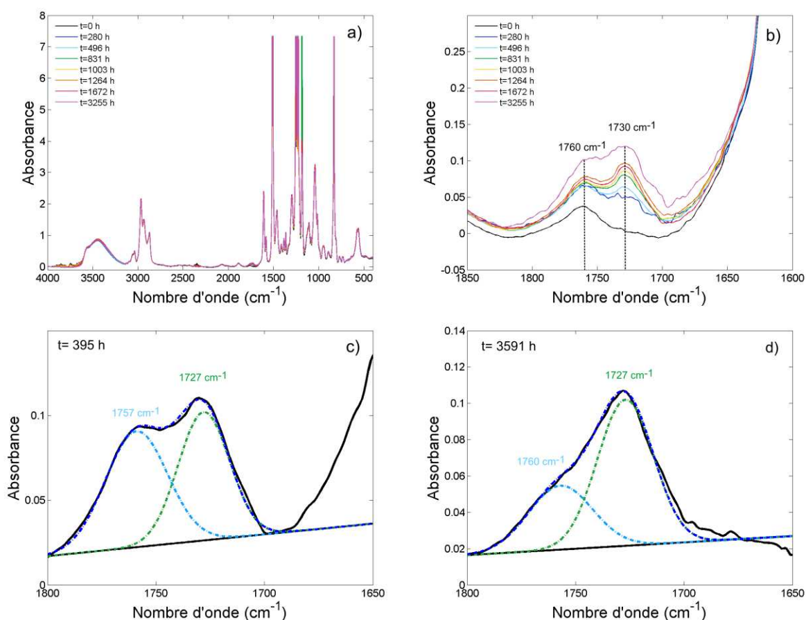
Figure 4:8: Spectres FTIR de PKHJ sous air à 120^\circ\text{C} a) Dans la gamme 4000\text{--}400\text{ cm}^{-1} b) Dans la gamme 1850\text{--}1600\text{ cm}^{-1} . Spectres déconvolués après c) 395\text{ h} d'exposition d) 3591\text{ h} d'exposition.
