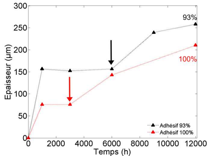
Figure 3:26: Epaisseur des couches oxydées en fonction du temps de vieillissement et du taux de réticulation, les flèches noires indiquent l'apparition des fissures.
