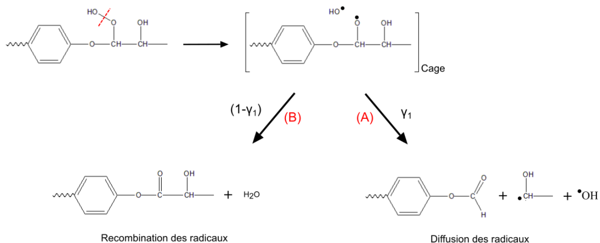
Figure 4:26 : Mécanismes de décomposition des hydroperoxydes dans PKHJ.
