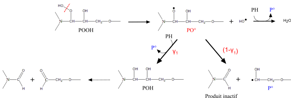
Figure 4:23: Exemple de décomposition d'un hydroperoxyde (ici P_2OOH ) par voie unimoléculaire.
