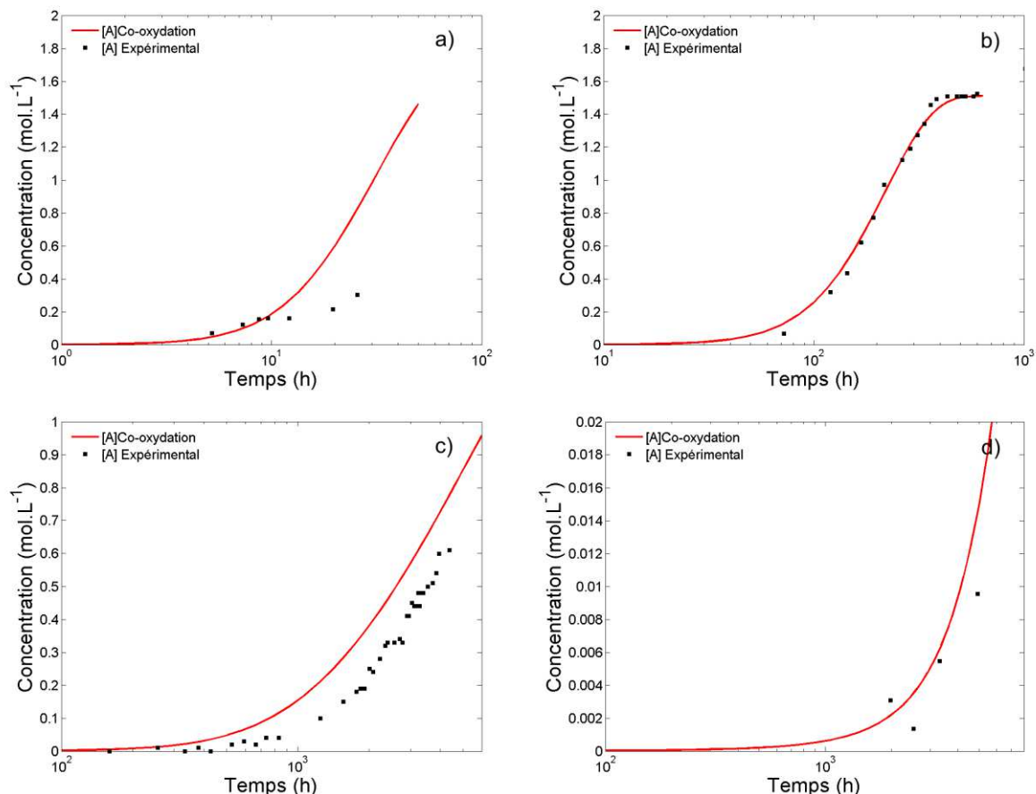
Figure 4:34: Comparaison entre les modélisations de co-oxydation et les données expérimentales pour les amides à 200°C (a), 160°C (b), 120°C (c) et 80°C (d).
