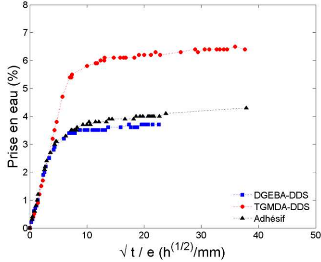
Figure 3.7 : Courbes de sorptions de l'adhésif et des systèmes binaires modèles en immersion dans l'eau à 70°C.
