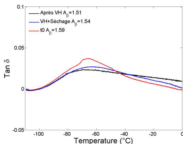
Figure A1:4: Evolution de la transition \beta au cours du vieillissement humide.
