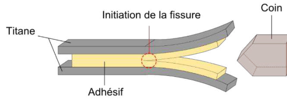
Figure 1:15 : Schéma d'une éprouvette de clivage en coin.
