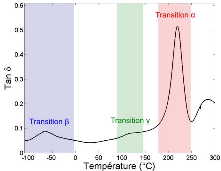
Figure 2:13: Analyse DMA de l'adhésif industriel à l'état initial et illustration des principales transitions visibles entre -110°C et 300°C.
