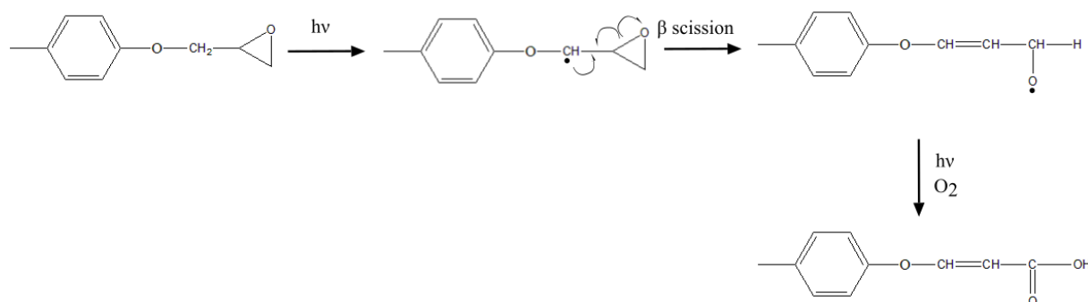
Figure 1:29: Formation d'un acide carboxylique insaturé lors de l'irradiation du monomère DGEBA.
