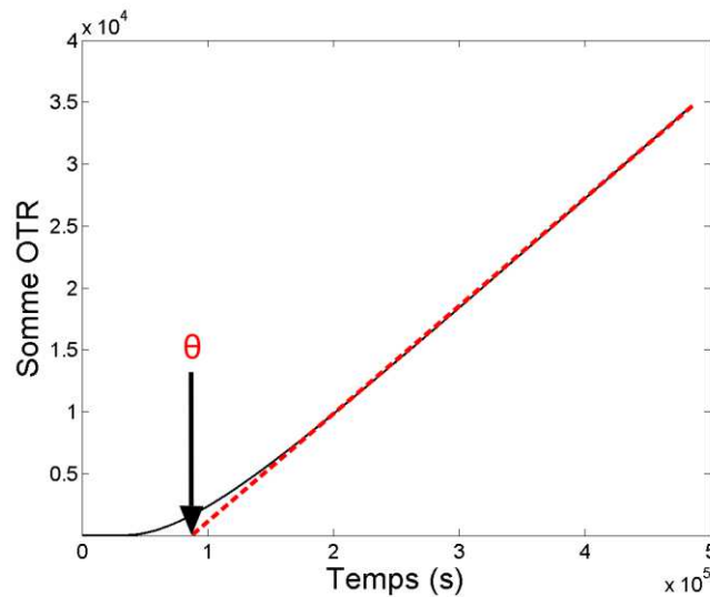
Figure 2:15: Somme des OTR en fonction du temps pour un film d'adhésif industriel à 23°C.
