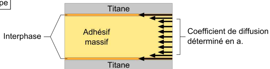
Figure 5:2 : Stratégie d'étude pour la détermination d'un coefficient de diffusion à l'interphase Titane/Adhésif.
