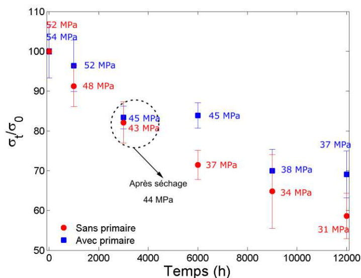
Figure A1:1: Contraintes à rupture des éprouvettes de cisaillement simples avec primaire vieillis à 70°C et 85% d'humidité relative.
