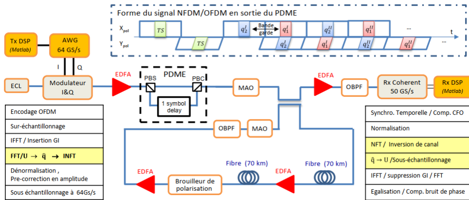
Figure 5.2: Dispositif expérimental. Insert: structure de la trame NFDML/OFDM multiplexée en polarisation, Etapes du traitement signal Tx/Rx (en blanc: OFDM, couleur: étapes spécifiques NFDML)
