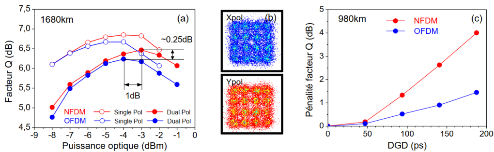
Figure 5.3: Performances obtenues: (a) résultats NFDML et OFDM en mono- et double polarisation, (b) Constellation s NFDML à -3dBm, (c) Sensibilité à la DGD.
