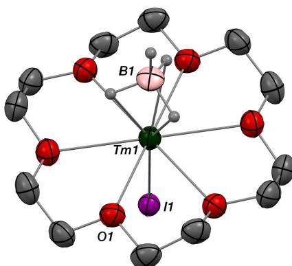
(a) ORTEP de 3.1 , les atomes d'hydrogène ont été masqués pour des raisons de clarté. Distances (Å) et angles (°) choisis : Tm1-O1B 2,639(5) ; Tm1-O2B 2,661(5) ; Tm1-O3B 2,652(4) ; Tm1-I2 3,1164(3) ; I2-Tm1-I2#2 180,0
