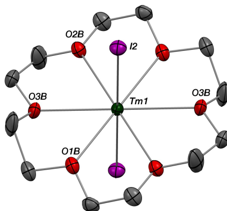
(a) ORTEP de 3.1 , les atomes d'hydrogène ont été masqués pour des raisons de clarté. Distances (Å) et angles (°) choisis : Tm1-O1B 2,639(5) ; Tm1-O2B 2,661(5) ; Tm1-O3B 2,652(4) ; Tm1-I2 3,1164(3) ; I2-Tm1-I2#2 180,0
