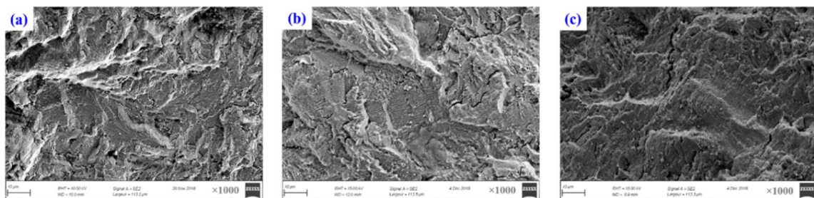
Figure III.43 : Image MEB des faciès de rupture des éprouvettes testées en fatigue équi-biaxiale dans l'eau distillée à la température ambiante
