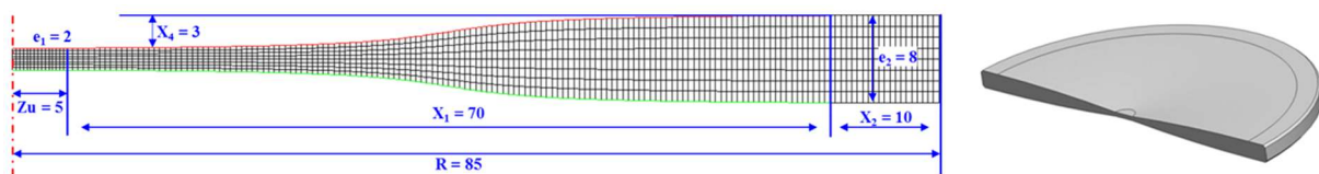
Figure III.4 : Géométrie de l'éprouvette imposée par les contraintes technologiques (mm)
