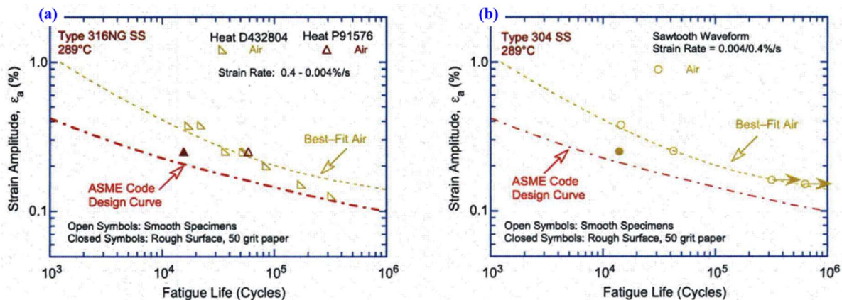
Figure I.9 : Effet de la rugosité de la surface sur la durée de vie en fatigue des aciers inoxydables austénitiques de type (a) 316NG et (b) 304L dans l'air [25]
