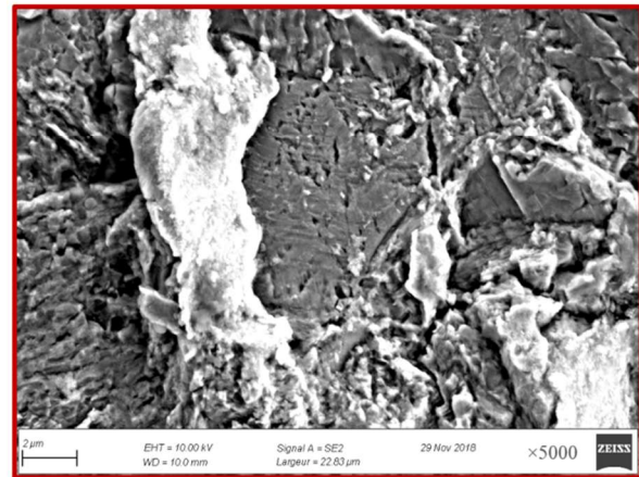
Figure III.28 : Aspect faciès de rupture pour différents agrandissement d'une éprouvette testée en fatigue équi-biaxiale dans l'eau distillée à la température ambiante en imposant une flèche de 1,1 mm
