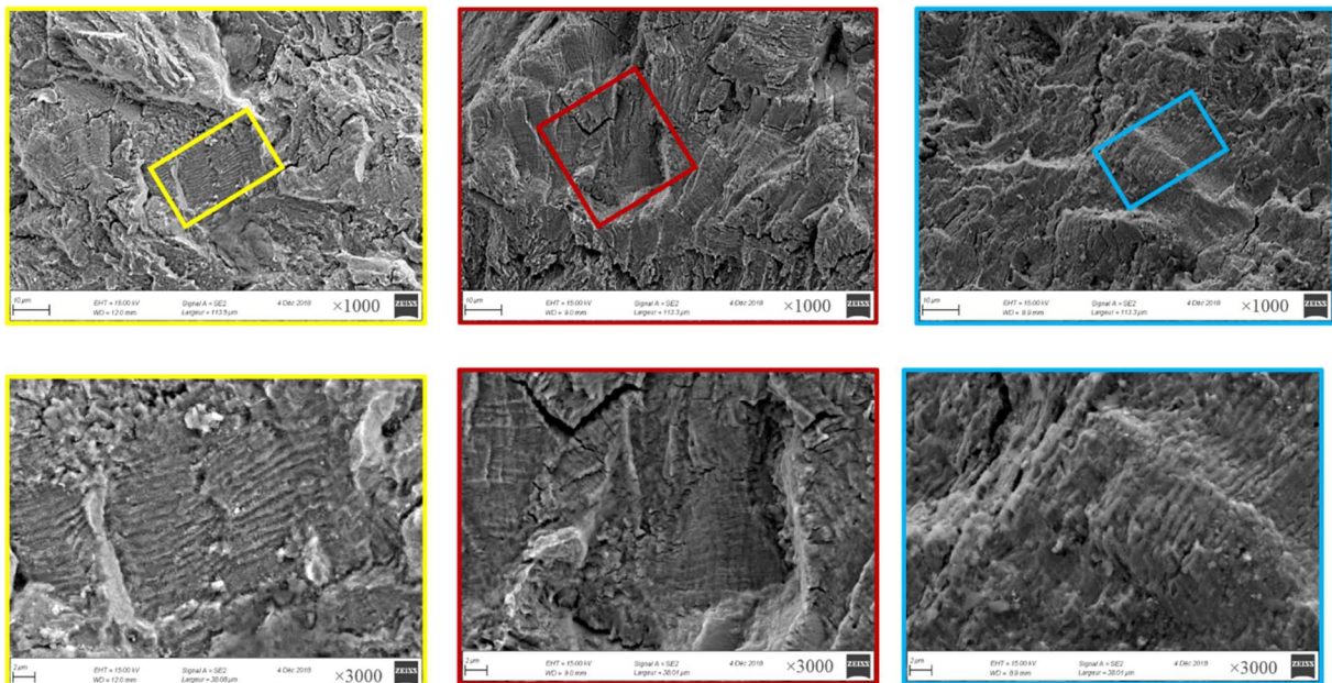
Figure III.27 : Aspect faciès de rupture à différent agrandissement d'une éprouvette testée en fatigue équi-biaxiale dans l'eau distillée à la température ambiante 743B-G (LVDT = 1,4 mm)
