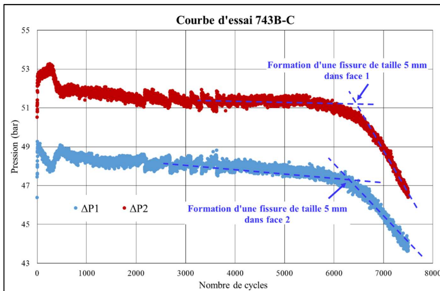
Figure IV.19 : Détection du nombre des cycles à la formation d'une fissure de 5 mm dans chaque face de l'éprouvette 743B-C testée en fatigue équilibrée à la température ambiante
