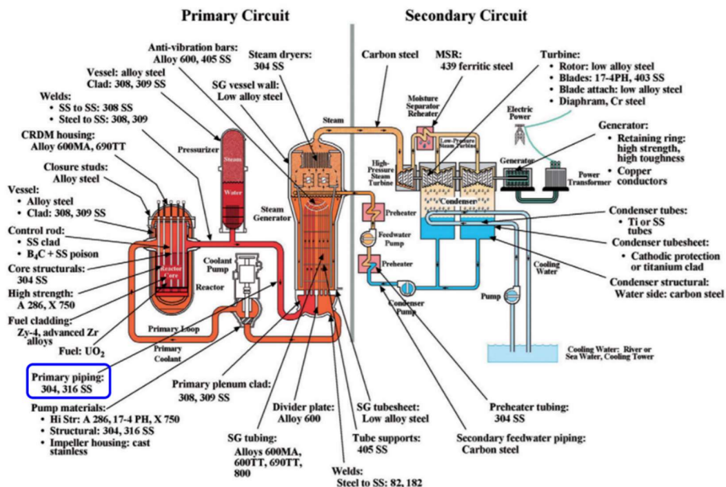
Figure i.1 : Les matériaux utilisés dans le réacteur type REP 1
