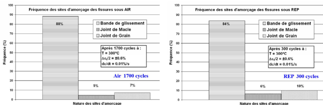
Figure I.47 : Comparaison de la nature des sites d'amorçage entre l'air et le milieu eau primaire REP [4]
