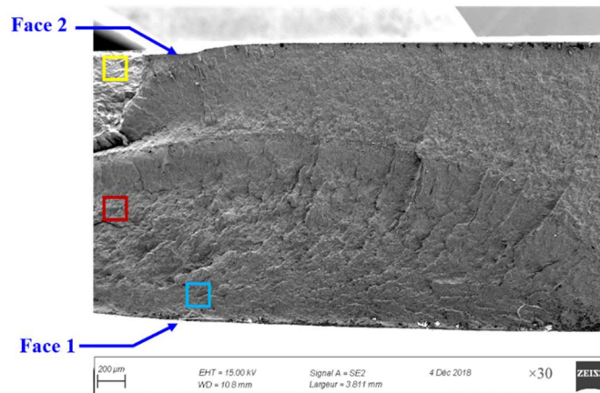
Figure III.26 : Analyse des fissure dans 743B-G (LVDT = 1,4 mm) (agrandissement x30)
