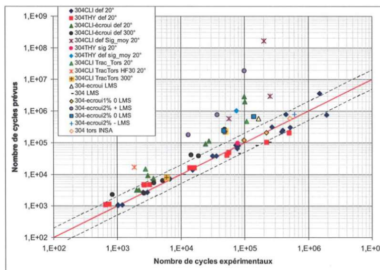
Figure I.16 : Evaluation du critère de Manson-Coffin [38]
