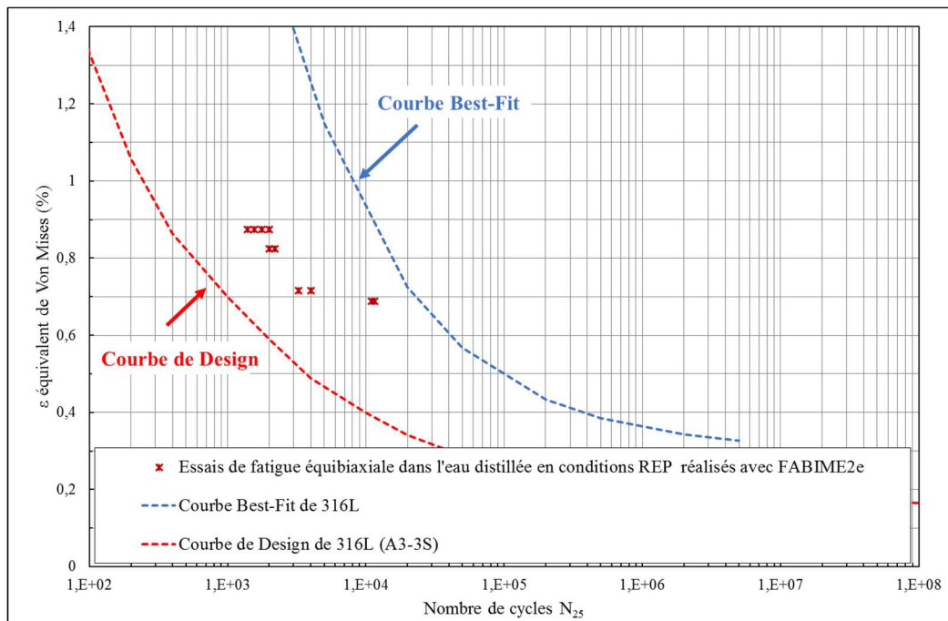
Figure ii.1 : Evolution de la déformation en fonction de la durée de vie des éprouvettes testées en fatigue équi-biaxiale dans l'eau distillée en conditions REP
