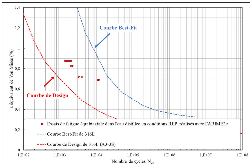
Figure IV.35 : Evolution de la déformation en fonction de la durée de vie des éprouvettes testées en fatigue équi-biaxiale dans l'eau distillée en conditions REP
