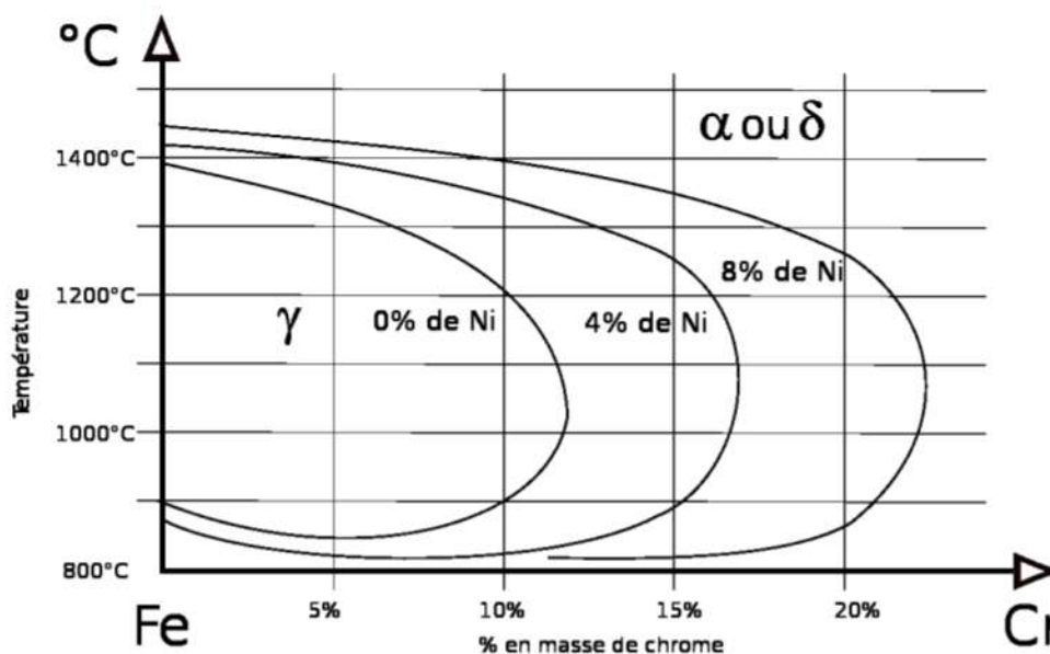
Figure II.2 : Coupe du diagramme ternaire fer-chrome-nickel reflétant l'influence du nickel sur l'extension de la boucle \gamma [2]
