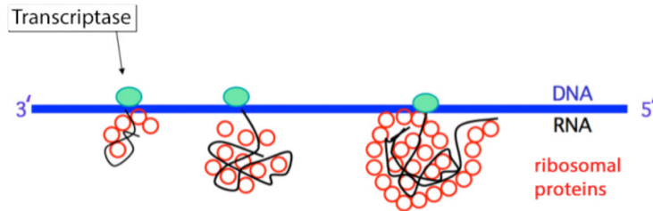
Figure III.3: L’hypothèse du “gradient d’assemblage” : les progrès de la synthèse d’ARNr définissent le progrès de l’assemblage.
