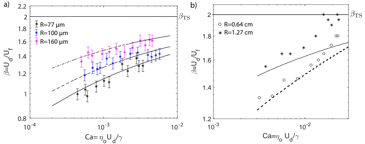
FIGURE 5.3: (a) Mesures expérimentales de mobilité \beta de bulle d'air dans de l'huile FC-40 en fonction du nombre capillaire pour trois rayons différents. La ligne noire horizontale est la solution de Taylor & Saffman [4]. Les lignes en tiret-pointillé, en tirets et en trait plein sont les courbes théoriques de la mobilité calculées à l'aide du modèle exposé en section 5.2 pour chaque rayon de bulle ; (b) Mesures expérimentales de mobilité de Maruvada & Park [9] pour des bulles dans de l'huile silicone ( 2H_o = 1.8 \text{ mm} , \gamma = 21 \text{ mN/m} , \eta_o = 97 \text{ mPa.s} ) pour deux rayons différents. La ligne noire horizontale est la solution de Taylor & Saffman [4]. Les lignes en tirets et en trait plein sont les courbes théoriques de la mobilité calculées pour les deux rayons de bulle.
