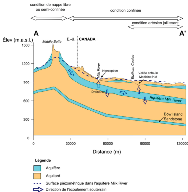
Figure 3.11 Coupe hydrogéologique de l'aquifère Milk River située le long d'une ligne d'écouement. La localisation de la coupe est indiquée au chapitre 6 (Figure 6.2).
