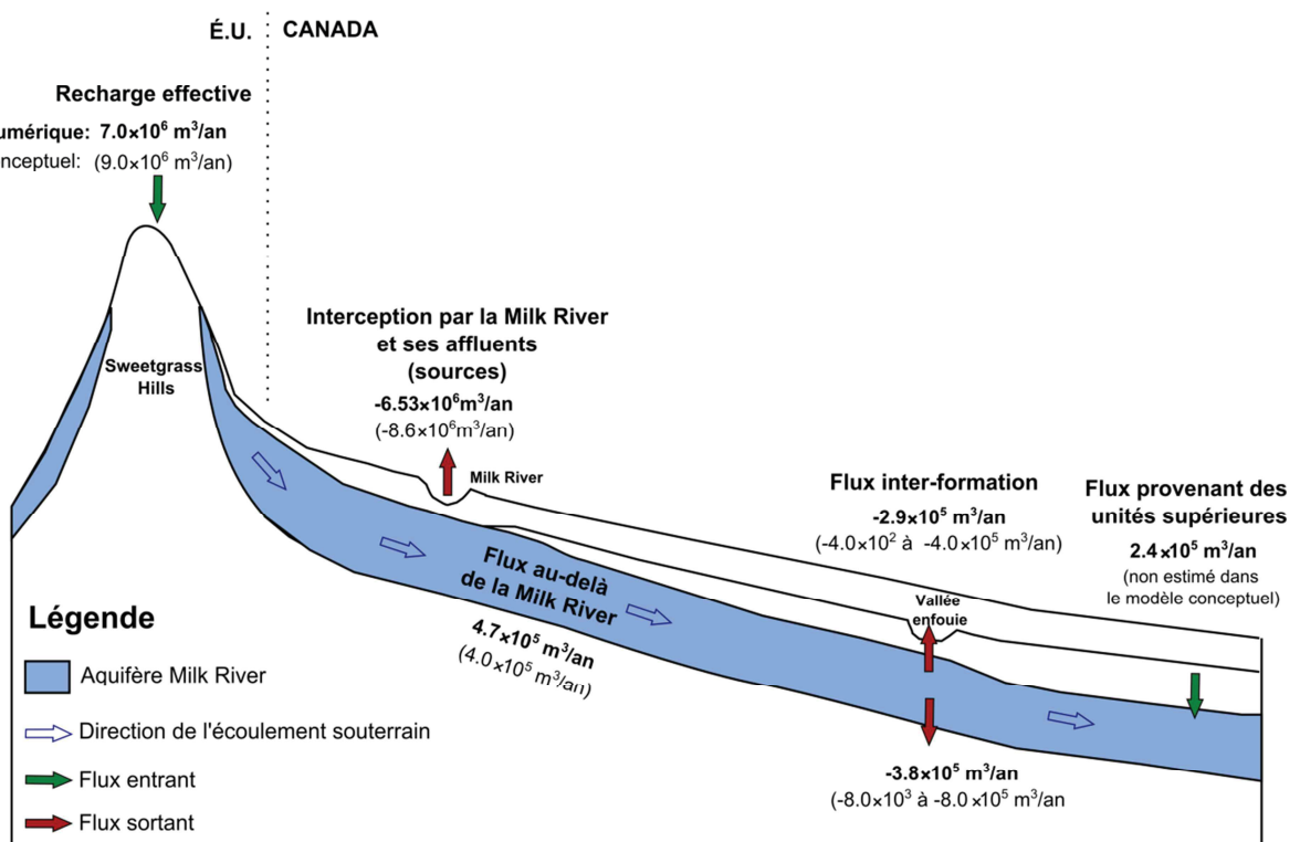
Figure 3.19 Comparaison entre les composantes du bilan en eau souterraine issues du modèle conceptuel (valeurs en caractère gras) (Pétré et al. 2016) et du modèle numérique d'écoulement
