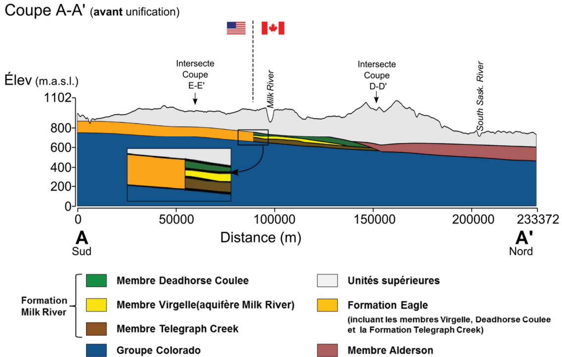
Figure 3.1 Coupe géologique transfrontalière avant l'unification du cadre stratigraphique.
