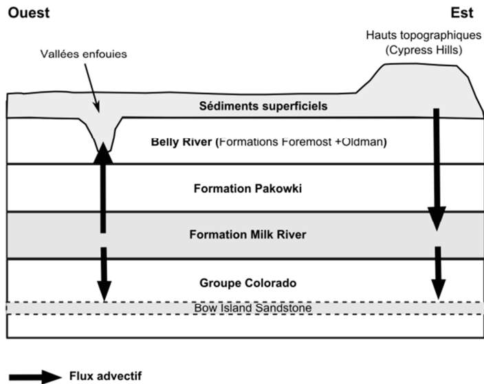
Figure 3.8 Gradients hydrauliques verticaux au sud de l'Alberta entre a) les sédiments superficiels et l'aquifère Milk River et b) l'aquifère Milk River et l'unité de grès sous-jacente Bow Island. c) diagramme représentant les tendances des flux verticaux (pas à l'échelle).
