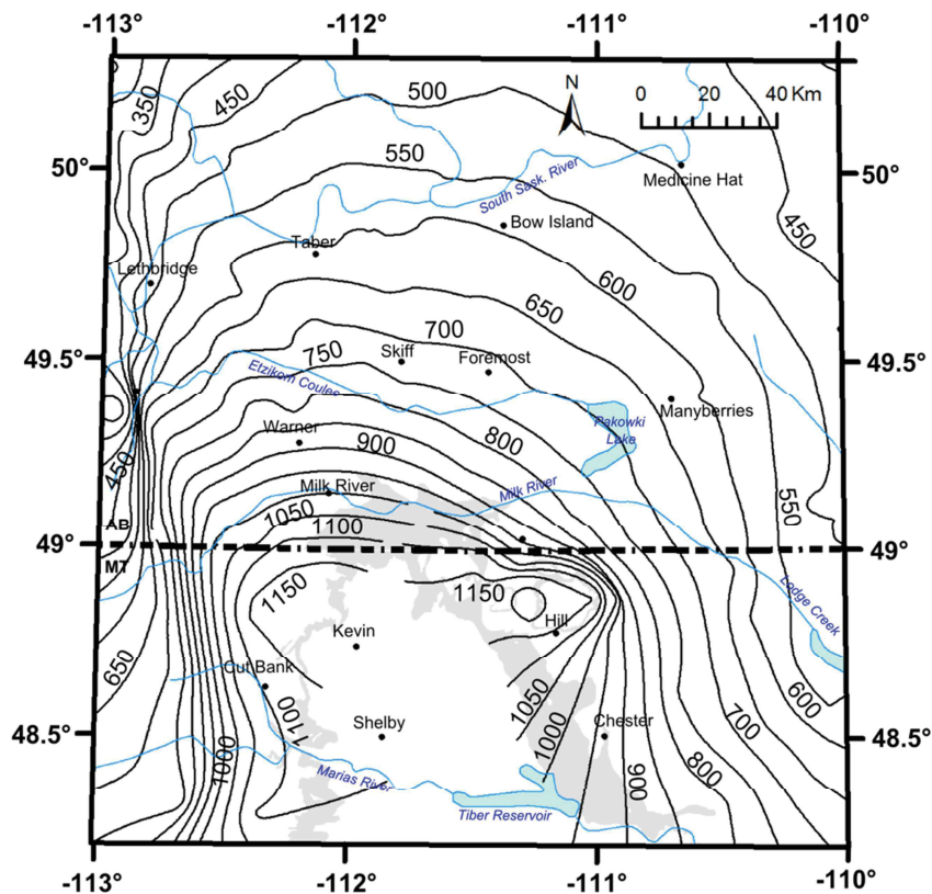
Figure 3.4 Élévation du toit de la Formation Milk River. L'intervalle entre chaque contour est de 50 m. L'aire grise correspond à la zone d'affleurement (ou de sous-affleurement) de la Formation Milk River.
