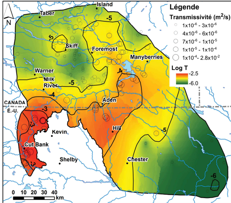
Figure 3.6 Carte transfrontalière de la transmissivité T de l'aquifère Milk River (valeurs krigées à partir des points de données disponibles indiqués sur la carte).
