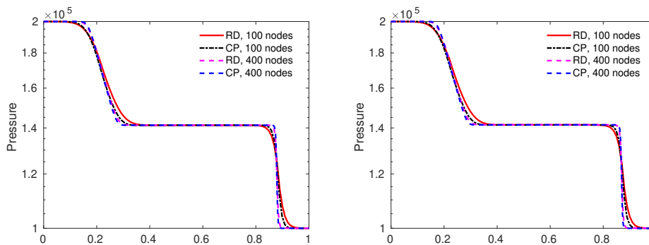
FIGURE 5.5 – Tube à choc d’un mélange liquide-vapeur à t = 0.8\text{ms} . Comparaison de la pression pour la formulation RD non-conservative et l’approche conservative CLAWPACK (CP) pour différents maillages - sans transfert de masse (à gauche) et avec transfert de masse (à droite).
