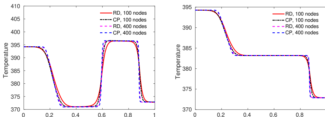
FIGURE 5.6 – Tube à choc d’un mélange liquide-vapeur à t = 0.8\text{ms} . Comparaison de la température pour la formulation RD non-conservative et l’approche conservative CLAWPACK (CP) pour différents maillages - sans transfert de masse (à gauche) et avec transfert de masse (à droite).
