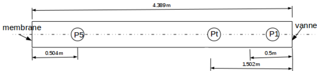
FIGURE 6.1 – Configuration expérimentale de l'expérience de Canon [120]
