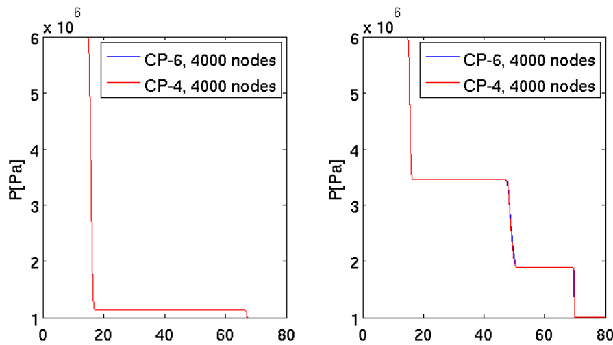
FIGURE 4.12 – Profil de la pression obtenu pour la résolution d’une dépression dans une conduite de CO_2 (à gauche sont présentés les résultats sans transfert de masse et à droite ceux obtenus avec transfert de masse)
