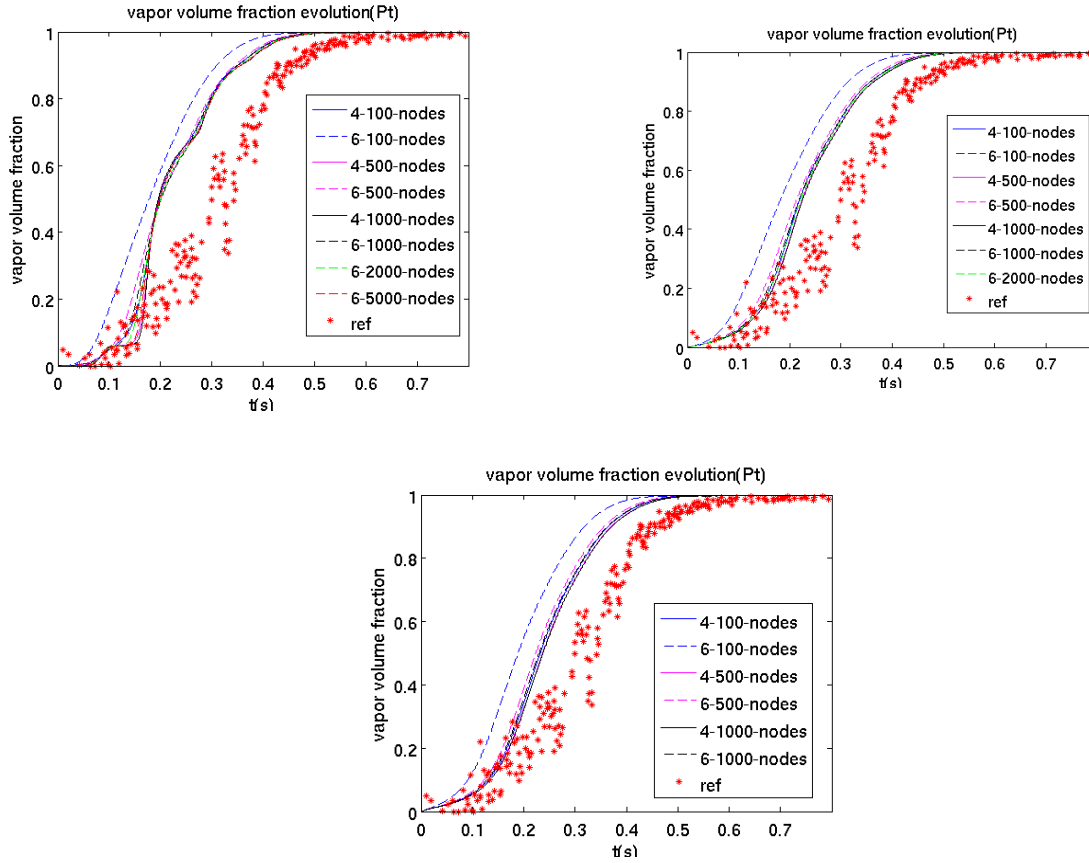
FIGURE 6.4 – Profil de la fraction volumique de vapeur du capteur Pt pour l'expérience de Canon obtenu avec les modèles à quatre équations et à six équations (à gauche : \Theta_t = 0 , à droite : \Theta_t = \Theta_{bilicki1} , au centre : \Theta_t = \Theta_{bilicki2} )
