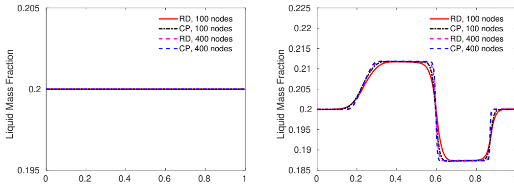
FIGURE 5.7 – Tube à choc d’un mélange liquide-vapeur à t = 0.8\text{ms} . Comparaison de la fraction de masse liquide pour la formulation RD non-conservative et l’approche conservative CLAW-PACK (CP) pour différents maillages - sans transfert de masse (à gauche) et avec transfert de masse (à droite).
