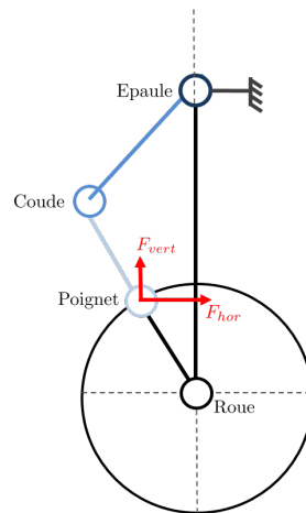
Figure 1.14 – Schéma du modèle 2D du système 4-barres "sujet-FRM" [Richter, 2001; Leary et al., 2012]
