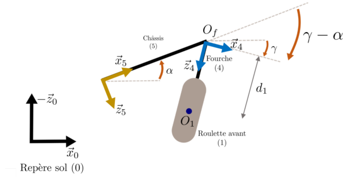
Figure 4.4 – Repères associés à la fourche avant à la roulette avant équivalente
