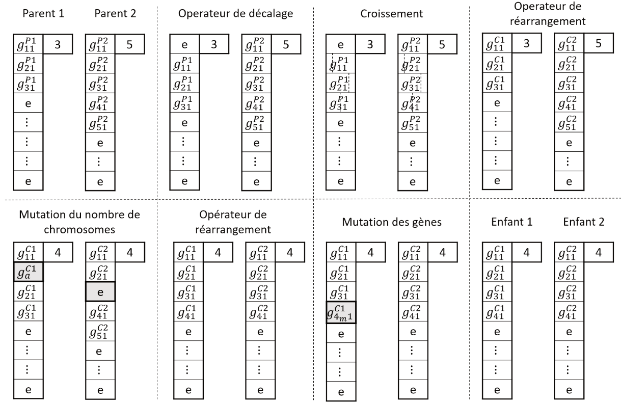
FIGURE 3.11 – Phase de reproduction modifiée entre deux individus appartenant à des espèces différentes
