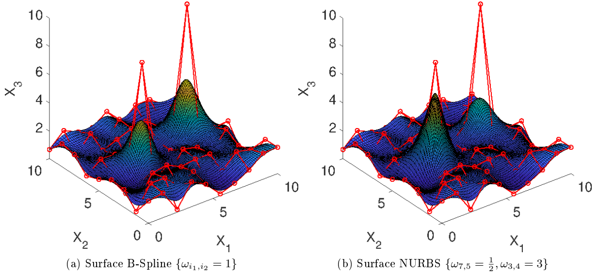
FIGURE 3.4 – Exemple de surfaces NURBS et B-Spline avec les mêmes degrés, points de contrôle et knot-vector
