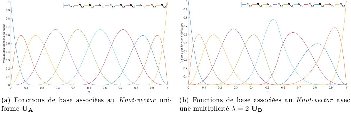
FIGURE 3.1 – Fonctions de forme pour des courbes B-Splines/NURBS de degré p = 3 et d'indice maximal de point de contrôle n = 9
