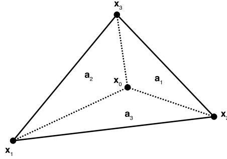
FIGURE 2.2 – Exemple de pondération par voisinage naturel en dimension N = 2 avec des polygones de Thiessen
