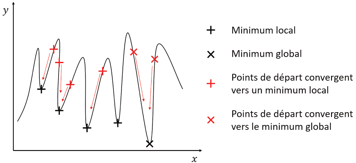
FIGURE 3.6 – Influence du point de départ pour la résolution de problème d'optimisation par des méthodes déterministes
