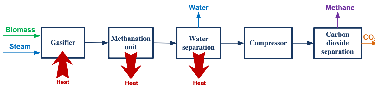
Fig. 4. Diagramme fonctionnel de la conversion du bois en méthane
