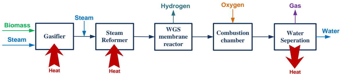
Fig. 3. Diagramme fonctionnel de la conversion du bois en hydrogène
