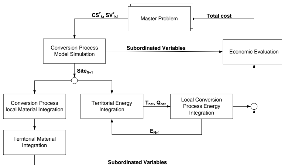
Fig. 1. Cadre de calcul du problème Maître-Esclave pour l'intégration des systèmes de conversion dans un territoire régi d'une gouvernance coopérative
