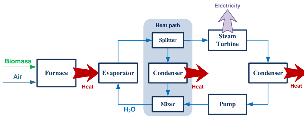
Fig. 5. Diagramme fonctionnel de la conversion du bois en énergie
