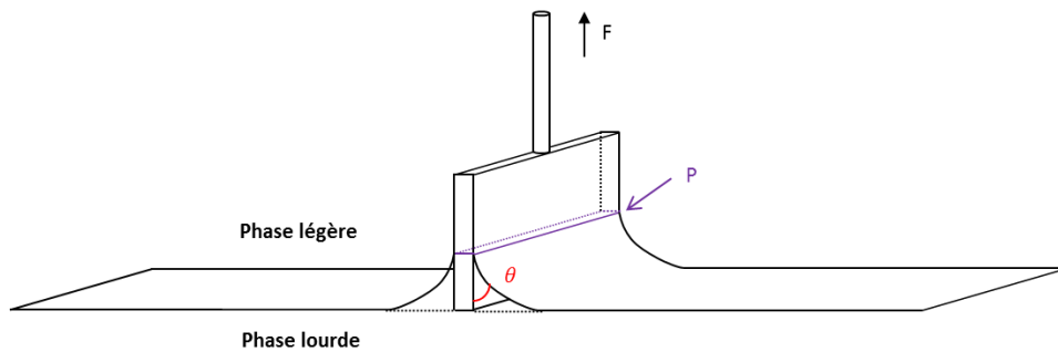
Figure 42 Méthode de la lame de Wilhelmy
