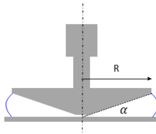
Figure 16 Géométrie cône-plan
