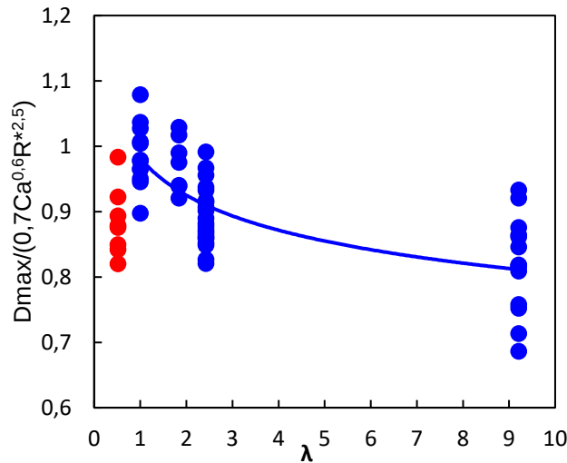
Figure 59 Evolution de \frac{D_{max}}{0.7 Ca^{0.6} R^{*2.5}} en fonction de \lambda pour tous les essais réalisés avec les couples mélanges d'huiles silicones / mélanges glycérol-eau dans le microsystème B
