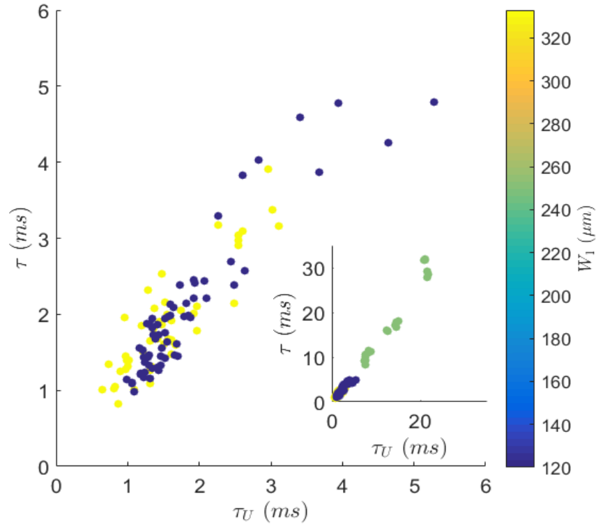
Figure 54 Temps de relaxation expérimental en fonction du temps de convection pour tous les essais réalisés avec les couples mélanges d’huiles silicones / mélanges glycérol-eau dans les microsystèmes B et C. Insert : Elargissement sur les points obtenus dans le microsystème A.
