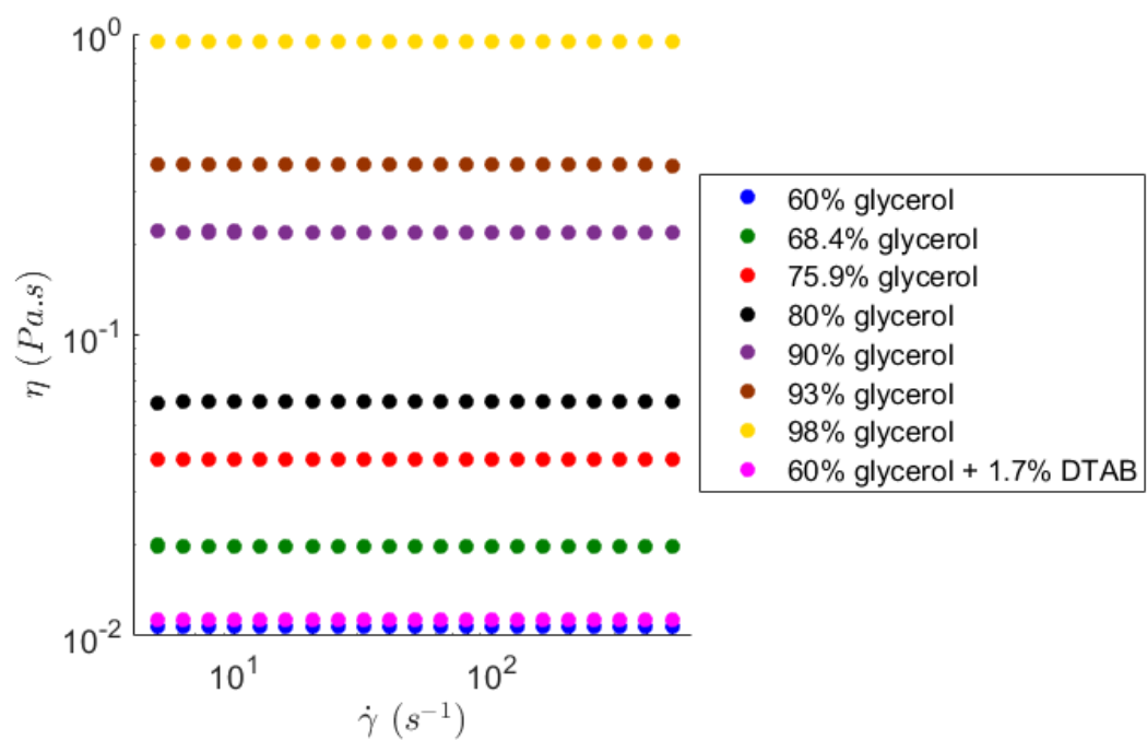
Figure 30 Viscosités à 20^\circ\text{C} des différents mélanges eau-glycérol étudiés
