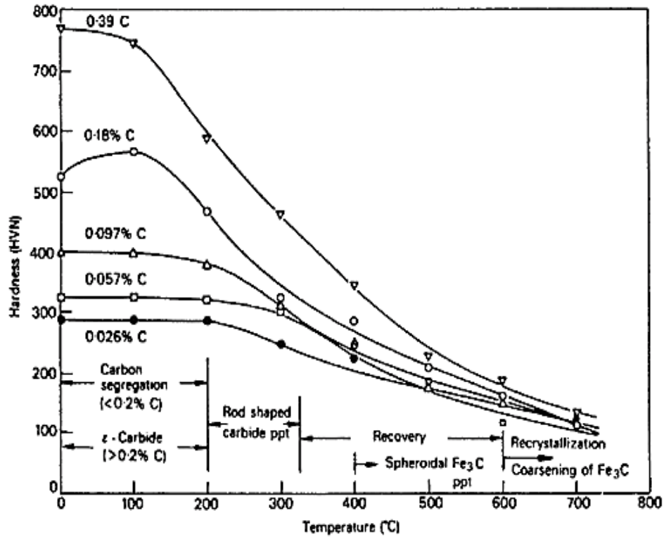
Figure I.12 : Variation de la dureté en fonction de la température de revenu des aciers Fe-C martensitiques, le revenu a été réalisé pendant 1h et les résultats sont issus de Speich et Leslie, 1972 [24].
