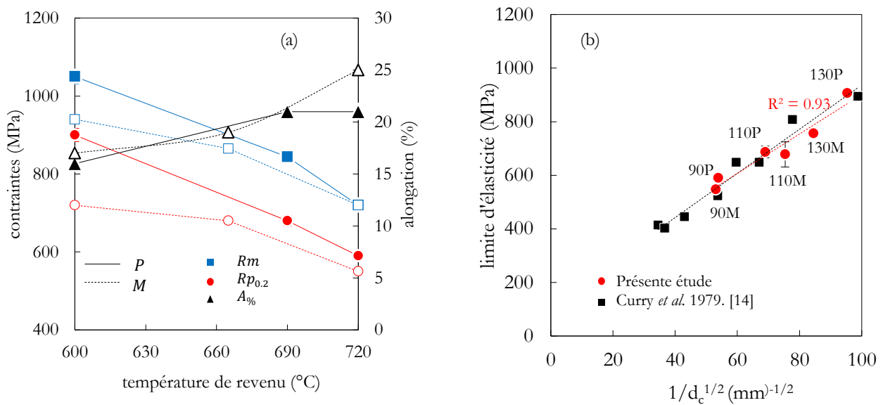
Figure III.14 : a) Evolution des propriétés en traction avec la température de revenu ; b) évolution de la limite d'élasticité avec la distance entre carbures.
