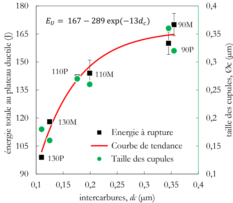
Figure IV.38 : Lien entre la distance moyenne intercarbure, l'énergie au plateau ductile et la taille moyenne des cupules
