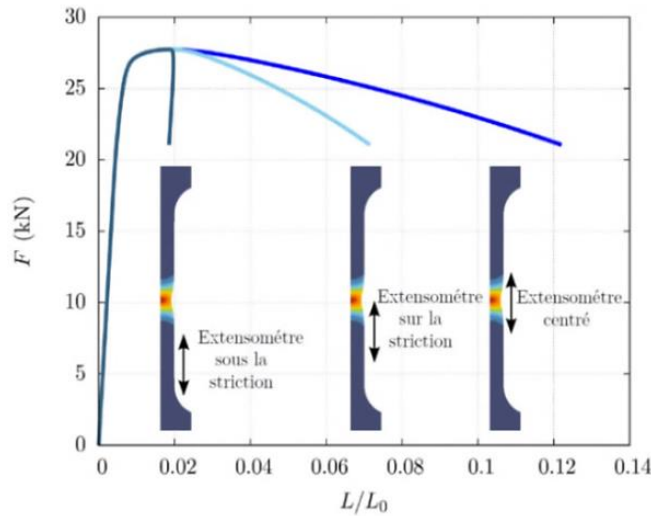
Figure III.1 : Effet de la position de l’extensomètre axial sur la mesure de déformation post-striction lors d’un essai de traction. Defaïsse, 2018 [3].
