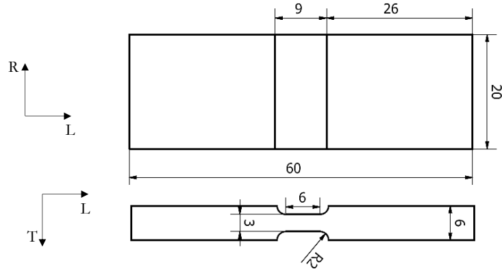
Figure III.9 : Géométrie des éprouvettes DP. Les dimensions données sont en mm.
