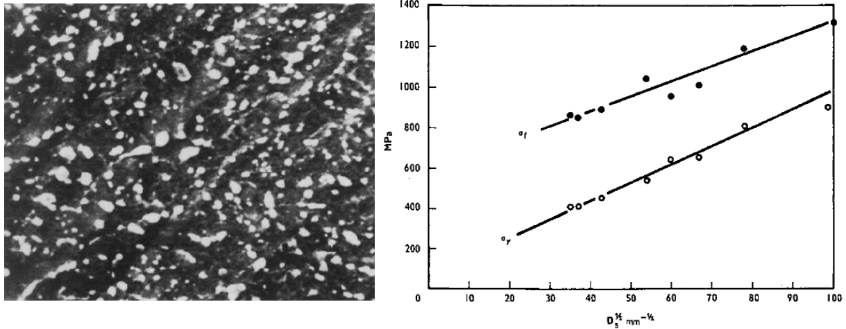
.Figure I.20 : a) Microstructure trempée-revenue d'un acier proche de la nuance 4140, grandissement \times 1200 tel que fournie par l'étude et b) Lien entre la résistance maximale en traction et la limite d'écoulement sur la distance intercarbures D_5 . Résultats issus de Curry et Pratt, 1979 [30]. \sigma_f est la résistance en traction et \sigma_y la limite d'écoulement.
