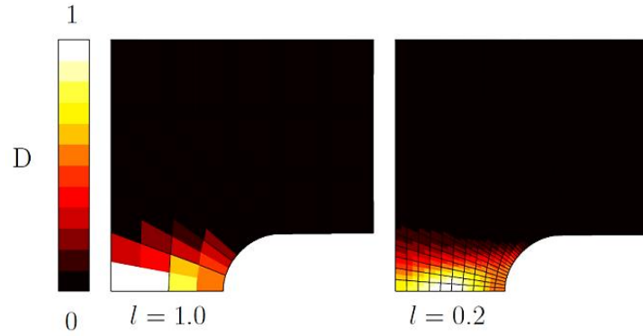
Figure V.10 : Effet de la taille des mailles sur l'emplacement du lieu d'endommagement maximal ( D=1 ) d'amorçage des éprouvettes AE , d'après Defaïsse, 2018 [10].
