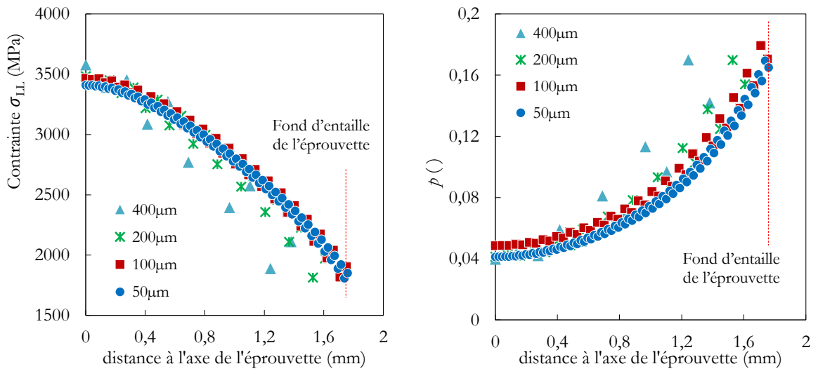
Figure V.14 : Champs locaux le long du ligament des éprouvettes AE à l'instant de rupture.
