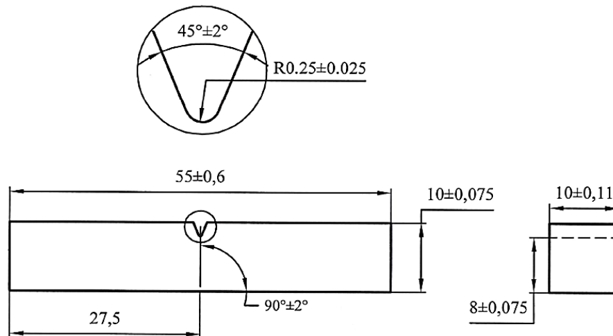
Figure IV.2 : Plan des éprouvettes de résilience avec entaille en V.
