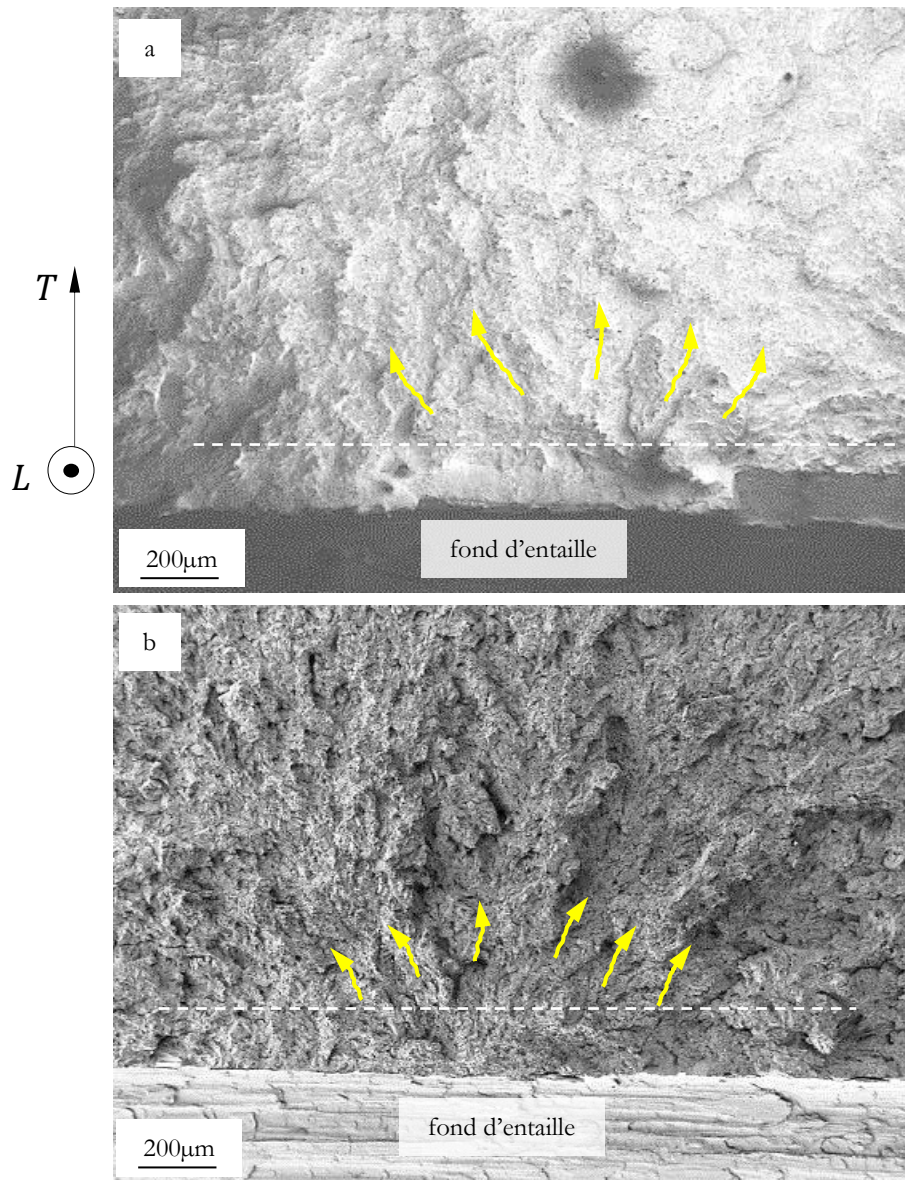
Figure IV.26 : Vue macroscopique des faciès de rupture à -196°C des microstructures a) 130P et b) 130M montrant une zone d'amorçage relativement large avec les sites d'amorçage potentiels. Les flèches jaunes indiquent la première propagation.
