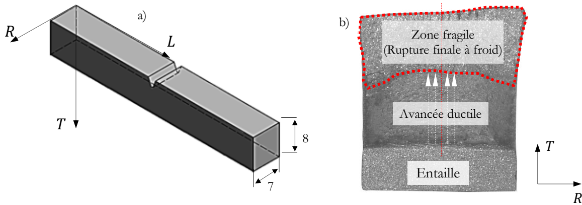
Figure IV.7 : a) Géométrie des mini éprouvettes de résilience, longueur 55 mm et b) mesure de l'avancée ductile au terme des essais de résilience sur mini éprouvette Charpy. Les dimensions de l'entaille sont les mêmes que pour une éprouvette Charpy normale.
