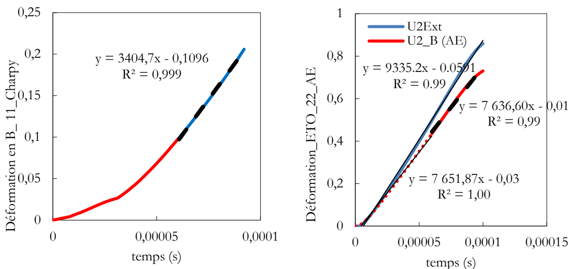
Figure 5 : Estimation des vitesses de sollicitation au point B. Comparaison entre la vitesse globale et celle du point B.
