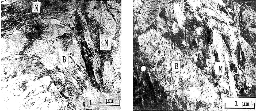
Figure I.24 : Microstructures en transmission des échantillons constitués de martensite et 25% de bainite inférieure avec : a) 0.2%C et b) 0.4%C, d'après Tomita et al. , 1991 [32].
