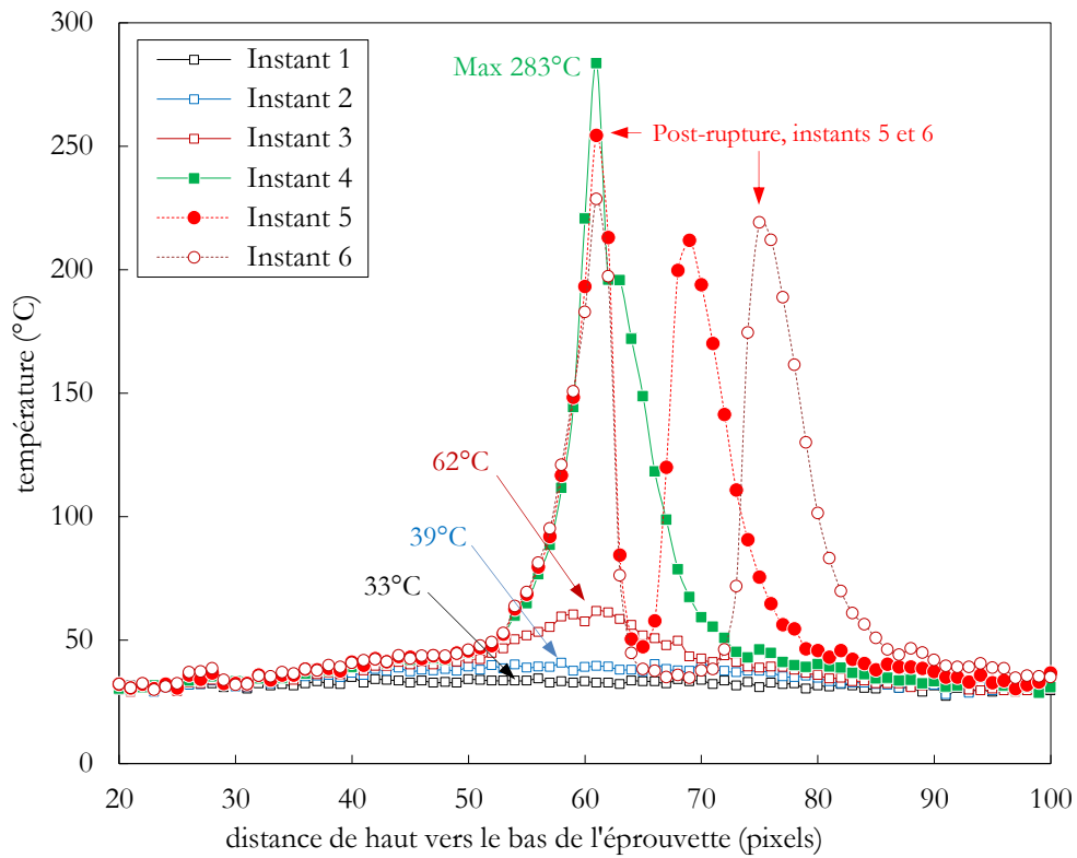
Figure III.24 : Profil de température le long des éprouvettes de traction rapide. Les profils correspondent aux instants de mesure de la fig.III.23 sur l'essai à 100\text{s}^{-1} sur le 130P.
