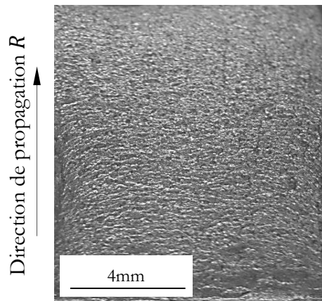
Figure IV.20 : Propagation en vague dans le sens R d'un essai Charpy d'une éprouvette 130P à la température ambiante.
