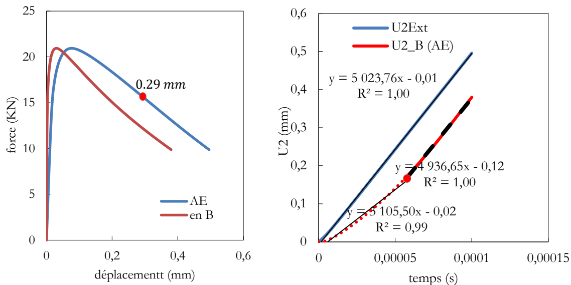
Figure 4 : Estimation des vitesses de sollicitation au point B. Comparaison entre la vitesse globale et celle du point B.
