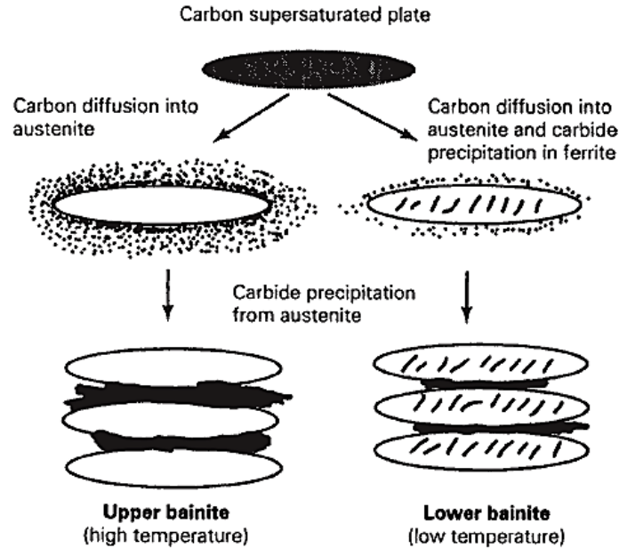
Figure I.10 : Illustration de la transition de la bainite supérieure à la bainite inférieure d'après Takahashi et Bhadeshia, 1990 [19].
