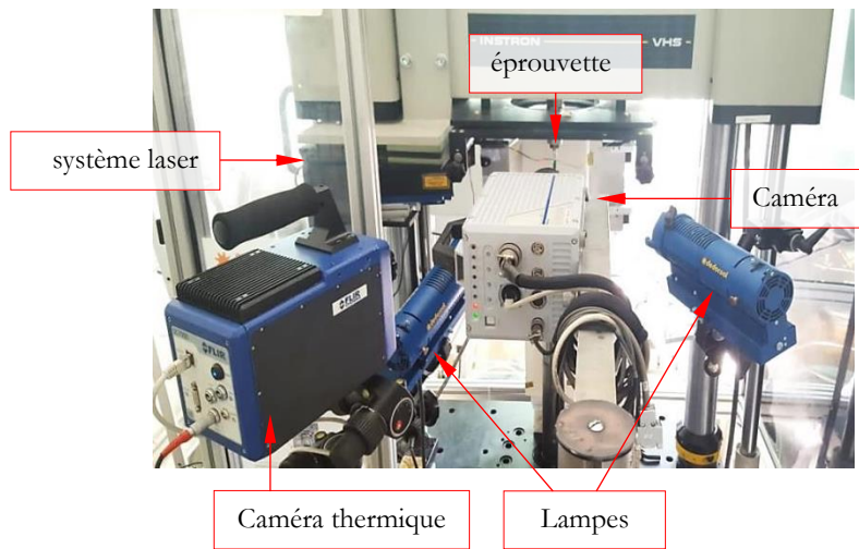
Figure III.5 : Montage expérimental des essais à la TGV.
