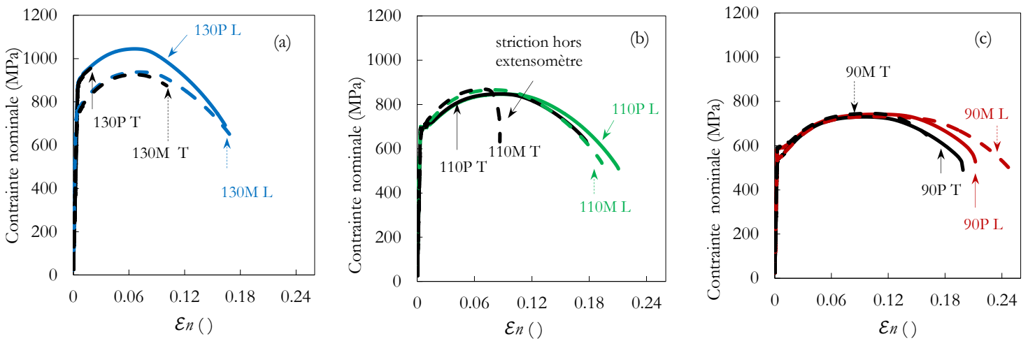
Figure III.11 : Courbes contrainte-déformation des essais AL_6 suivant les directions de sollicitation L et T. Essais réalisés à la température ambiante.
