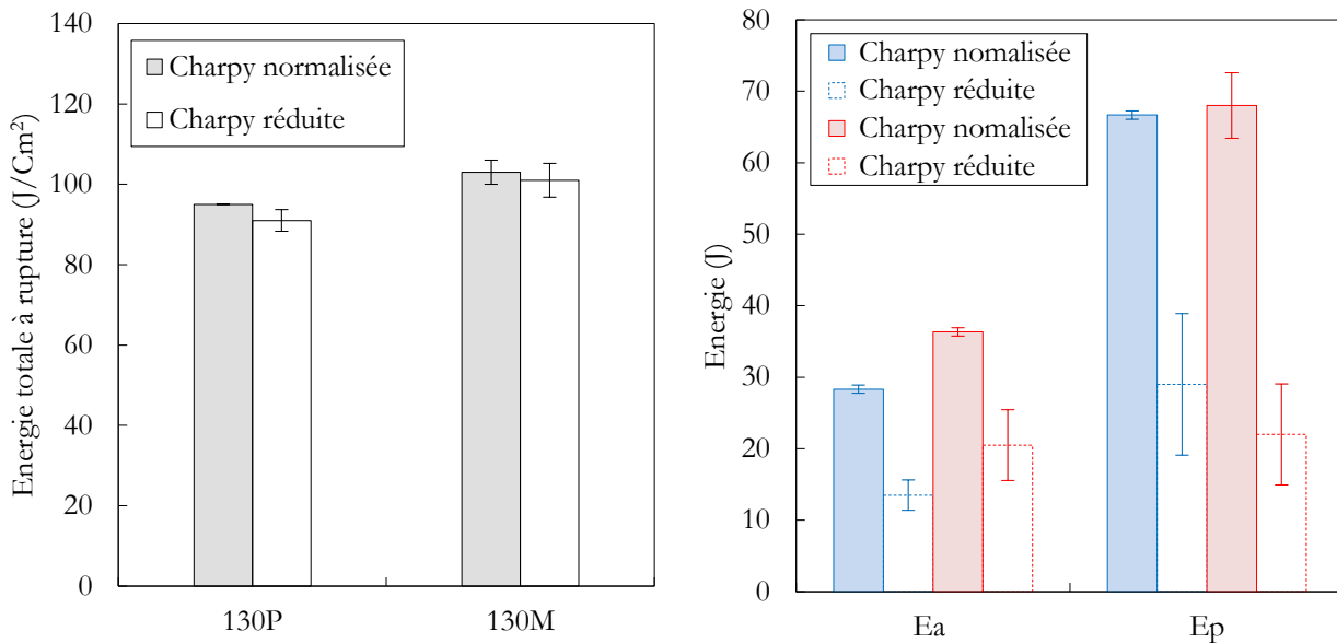
Figure IV.23 : a) Effet de la dimension des éprouvettes Charpy sur les énergies à rupture par unité d'aire des essais Charpy entre éprouvettes normalisées et éprouvettes réduites, b) Comparaison des énergies d'amorçage et de propagation.
