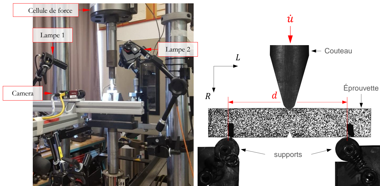
Figure IV.4 : Montage expérimental des essais Charpy en quasi-statique.
