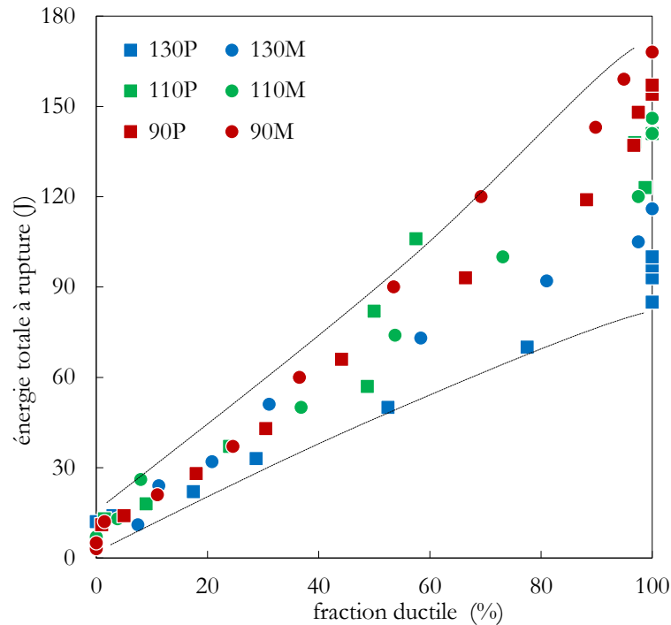
Figure V.28 : Evolution de l'énergie totale à rupture avec la fraction de zones ductiles à l'échelle du faciès de rupture des éprouvettes Charpy.
