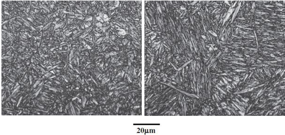
Figure I.29 : Microstructures des échantillons 1153 et 1373 trempés et revenus à 450°C pendant 90min, d'après Takebayashi et al. 2013 [44].
