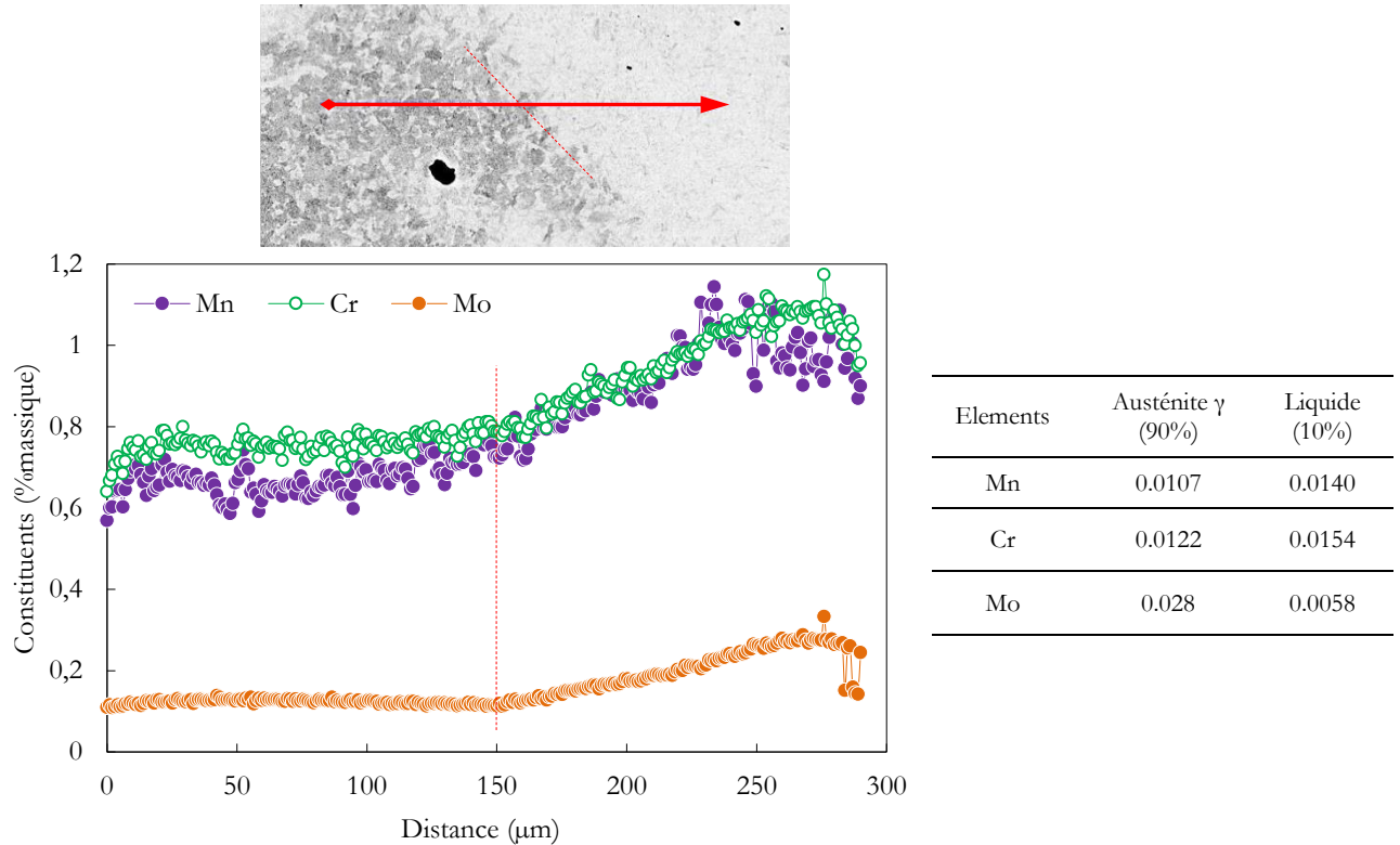
Figure II.11 : Profil EDS des éléments majeurs entre une zone ségréguée et zone appauvrie. Mesures faites sur l'échantillon de dilatométrie TDIL262 (M) contenant 20% de bainite. Prédiction des teneurs par calcul T-Calc.
