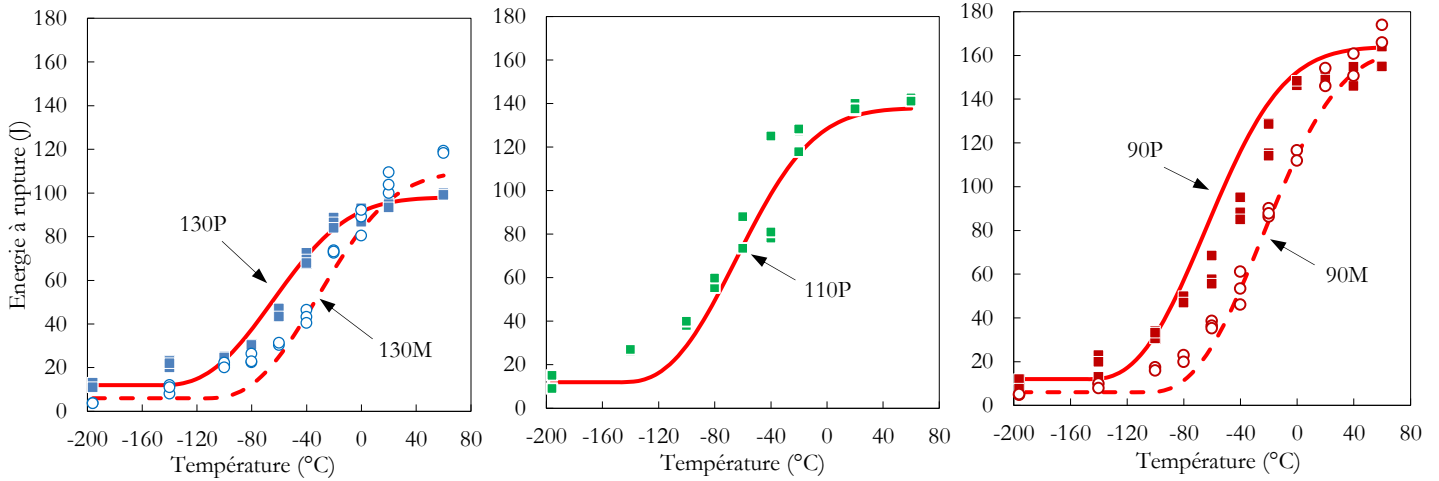
Figure V.34 : Prédiction des courbes de résilience de cinq microstructures de l'étude, effet du paramètre local T_o .
