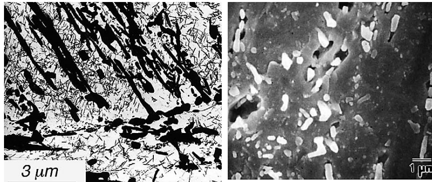
Figure I.28 : a) Réplique extractive au carbone typique d'un acier SA508 cl. III observé en transmission et b) coupe polie sous le faciès d'une éprouvette de traction uniaxiale, d'après Im et al. 2001 [42].
