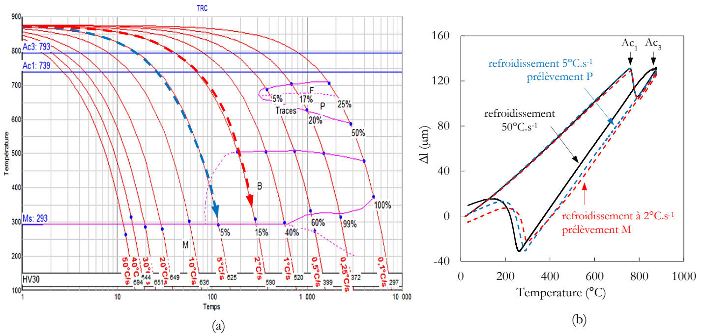
Figure II.6 : a) Diagramme TRC d'un acier 40CrMo4 nommée ici « acier TRC », austénitisé à 875°C pendant 20 min, b) Courbes de dilatométrie des microstructures aux positions P et M. d'après M. Saby, 2015 [4]
