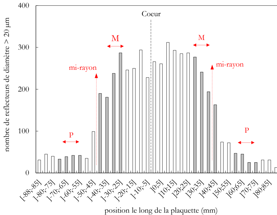
Figure II. 24 : Distribution de la répartition des réflecteurs de la peau vers le cœur de la barre suivant le plan travers.
