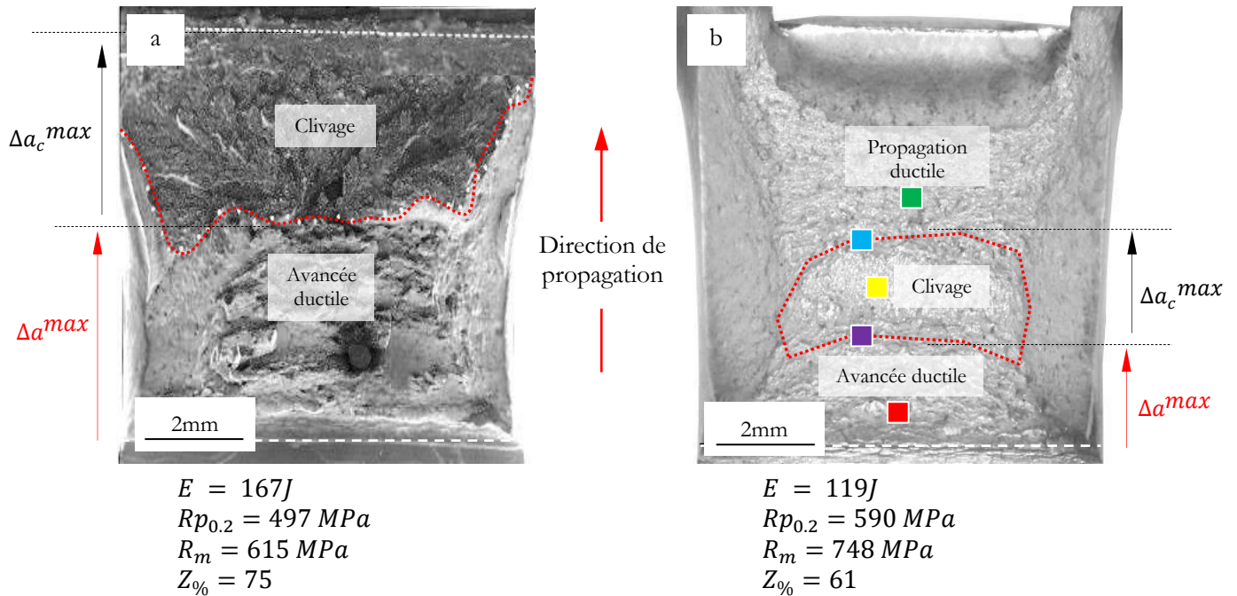
Figure IV.12 : Faciès de rupture dans le domaine de transition ductile-fragile pour les nuances : a) acier 16MnNiMo5 d'après B. Tanguy, 2001 [6] et b) acier de l'étude (90P). Les essais ont été réalisés à -20^{\circ}C et les boîtes en rouge, violet, jaune, cyan et vert indiquent les lieux des images sur la fig.IV.13.
