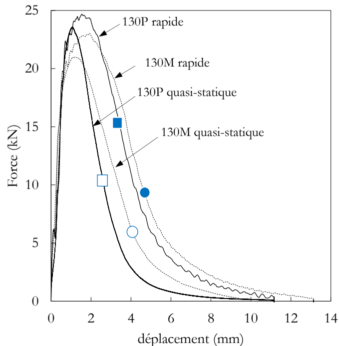
Figure IV.21 : Courbes charge-déplacement des essais à la température ambiante en conditions quasi-statique et rapide. Les essais ont été réalisés sur des éprouvettes en sens long LT .
