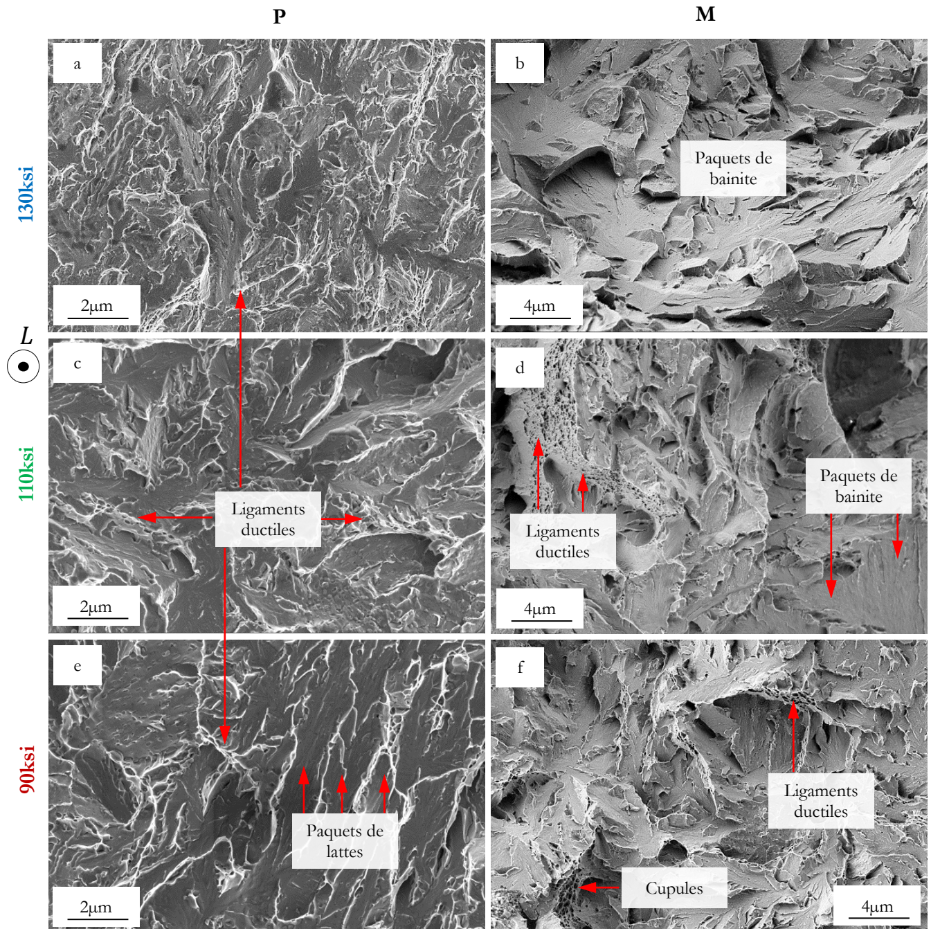
Figure IV.30: Propagation dans le domaine de transition ductile – fragile. Les facès correspondent à des essais réalisés à : a) -60°C pour le 130P, b) -40°C 130M, c) -60°C pour le 110P, d) -60°C pour le 110M, e) -40°C pour le 90P et f) -20°C pour le 90M.
