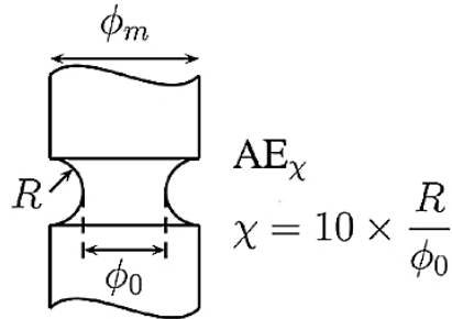
Fig. III.8 : Dimensions caractéristiques de l'entaille des éprouvettes AE par Besson et al. 2004 [6].
