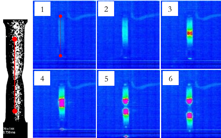
Figure III.23 : Cartographies thermiques à différents instants de mesure de l'échauffement local le long du fût de l'éprouvette. Cas de l'essai réalisé à 100\text{s}^{-1} sur le 130P.
