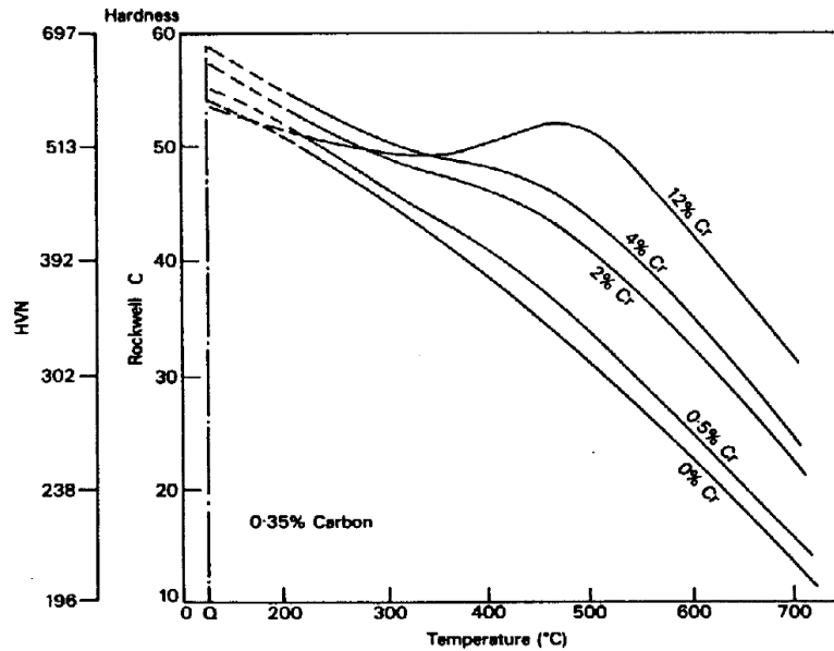
Figure I.15 : Effet du chrome sur la dureté après revenu d'un acier à 0.35%C, d'après Bain et Paxton, 1961 [25].
