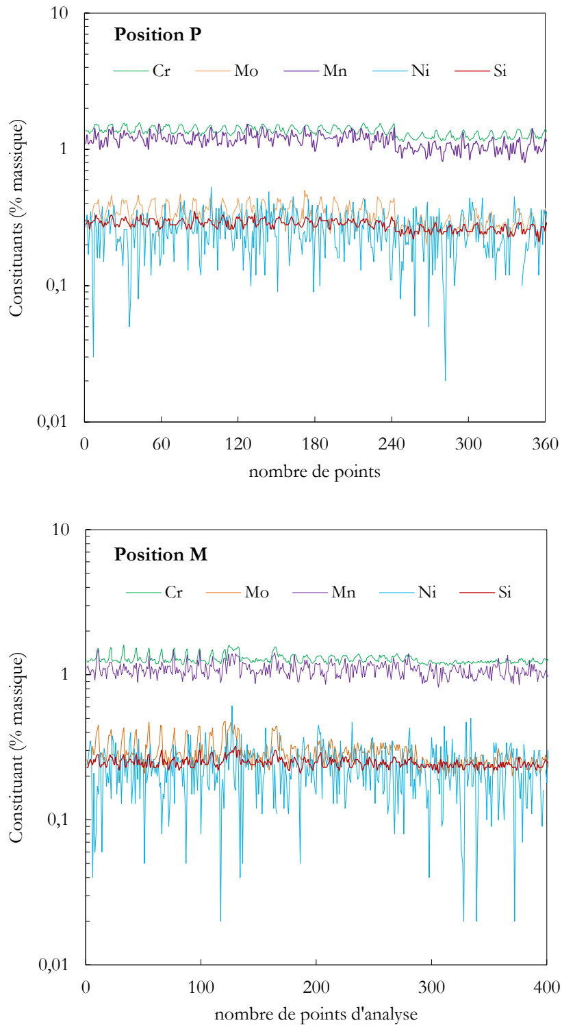
Figure II.5 : Composition chimique des éléments d'addition majeurs à l'échelle locale. Les mesures ont été faites à la microsonde de Castaing avec une distance entre points de 10 \mu m
