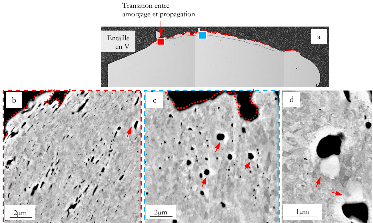
Figure IV.37 : Endommagement ductile sur coupe polie d'une éprouvette de résilience 90P, l'essai a été réalisé à +60°C. On a : a) Vue d'ensemble, b) Endommagement dans la zone de transition entre amorçage et propagation ductile, c) Endommagement dans la zone de propagation et d) Décohésion entre carbures (phases claires) et matrice. Les flèches rouges indiquent les carbures et les images ont été prises en électrons rétrodiffusés.
