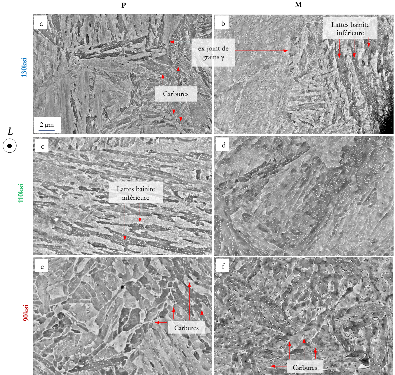
Figure II.18 : Microstructure sur lames minces des microstructures a) 130P, b) 130M, c)110P, d) 110M, e) 90P et f) 90M. Observations faites au MEB en électrons rétrodiffusés
