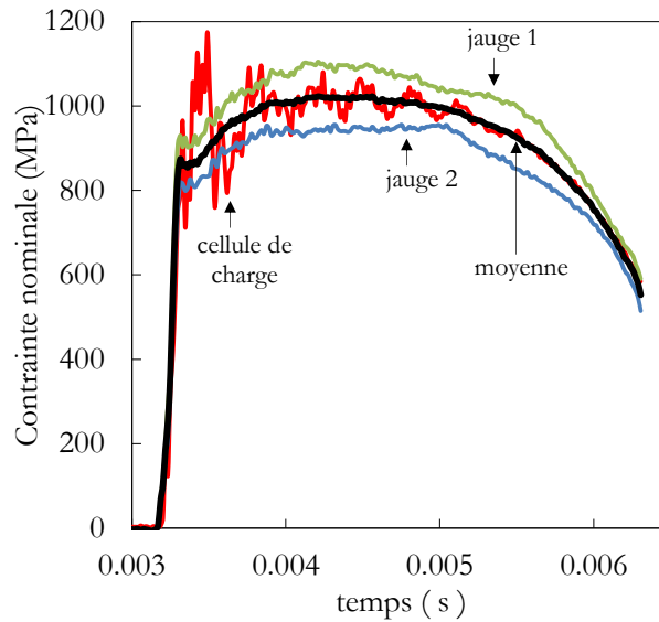
Figure III.7 : Dépouillement des résultats des essais à la TGV ; cas de l'essai réalisé à 100\text{s}^{-1} sur le 130M.
