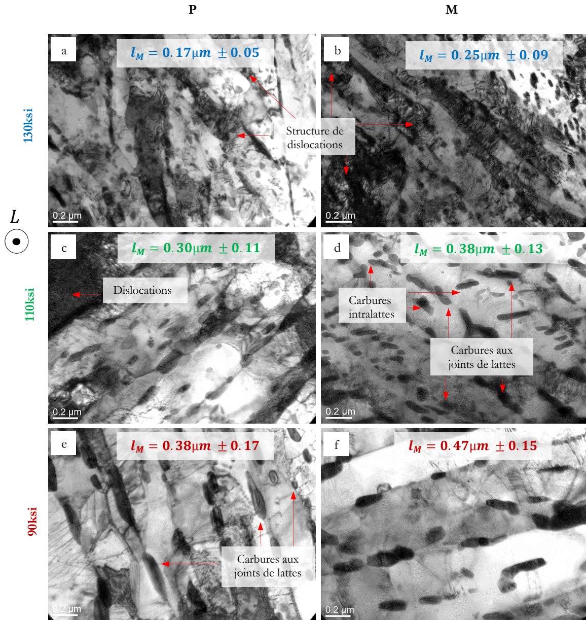
Figure II.20 : Micrographies MET en champ clair à l'échelle des lattes des microstructures : a) 130P, b) 130M, c) 110P, d) 110M, e) 90P et f) 90M. Images faites en champ clair sur lames minces.
