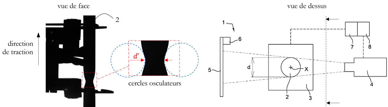
Figure III.2 : Montage expérimental et mesure de la réduction de diamètre courant sur une éprouvette axisymétrique [3].
