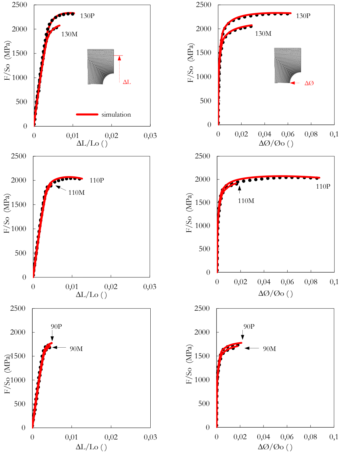
Figure V.15 : Comparaison entre la prédiction par le modèle et les valeurs expérimentales du comportement à rupture à -196°C des éprouvettes AE .
