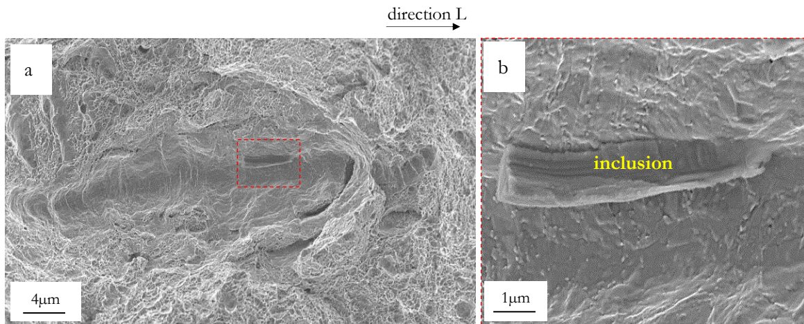
Figure III.12 : Faciès de rupture d'une éprouvette de traction en sens travers, cas du 130P sens T.
