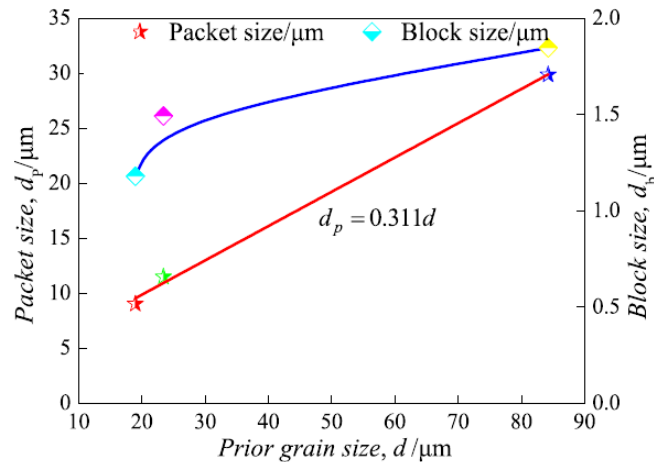
Figure I.5 : Relation entre la taille des paquets d_p et la taille des blocs d_b avec la taille de grain d'austénite primaire d , d'après Liang et al. 2017 [8].
