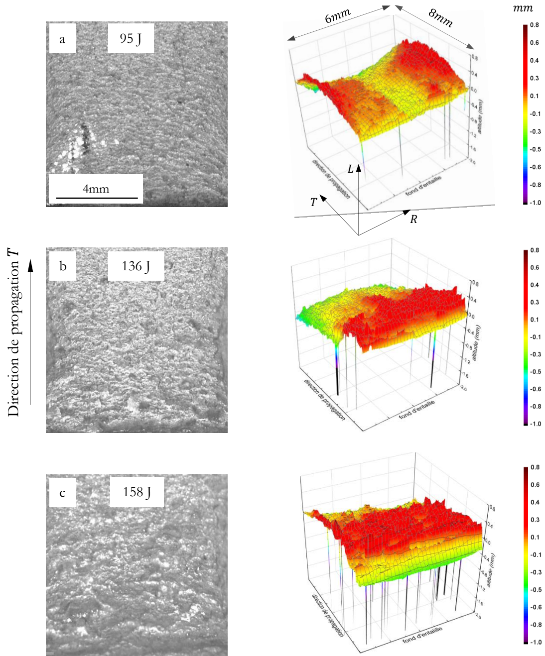
Figure IV.19 : Zone d'intérêt et mesures topographiques correspondantes des faciès de rupture sur le plan travers RT , cas des microstructures a) 130P (95J), b) 110P (136J) et c) 110P (158J). Les vues macroscopiques sont au même grandissement.
