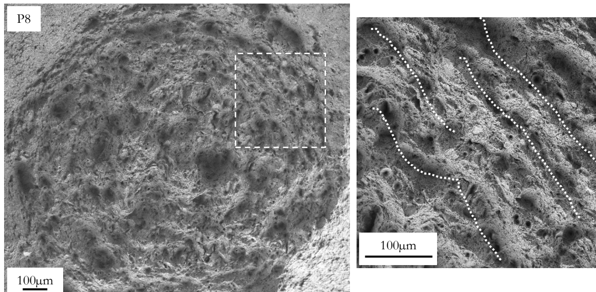
Figure 11 : Identification des vagues sur le faciès de l'éprouvette P8 (vitesse rapide)
