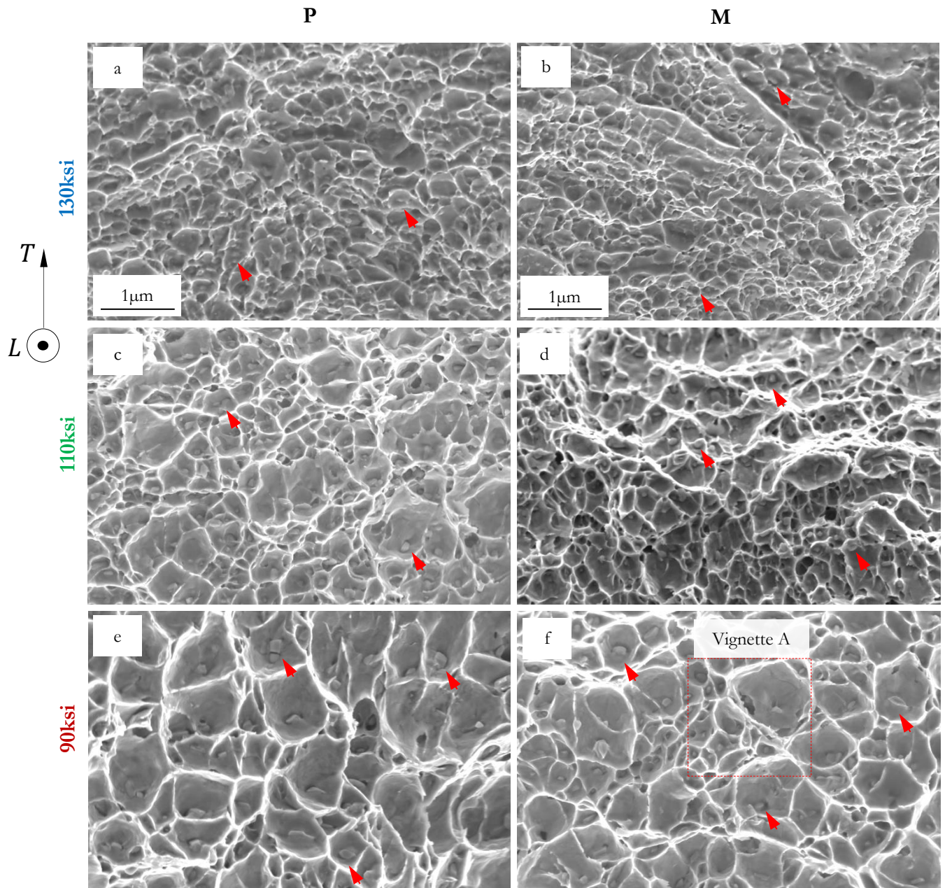
Figure IV.34 : Faciès de rupture sur le plateau ductile des six microstructures au même grandissement : a) 130P à 100J, b) 130M à 120J, c) 110P à 142J, d) 110M à 147J, e) 90P à 160J et f) 90M à 170J. Les faciès de rupture sont ceux des essais réalisés à +60°C et les flèches rouges indiquent certains carbures.
