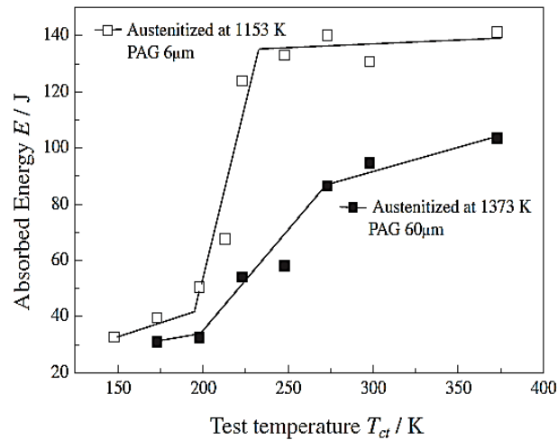
Figure I.30 : Transition ductile-fragile des échantillons 1153 et 1373 trempés et revenus à 450°C pendant 90min, d'après Takebayashi et al. 2013 [44].
