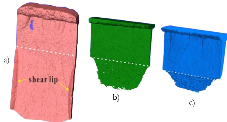
Figure IV.16 : Images de tomographie 3D des rayons X des éprouvettes de ténacité d'un acier 4340 revenues à : a) 180°C, b) 350°C et c) 500°C par Li et al. 2018 [3].
