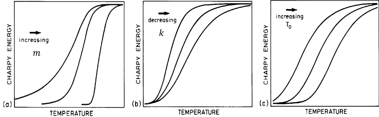
Figure V.27 : L'effet des paramètres a) de forme, b) d'échelle et c) local sur la fonction de Burr ; d'après Windle et al. 1996 [21]
