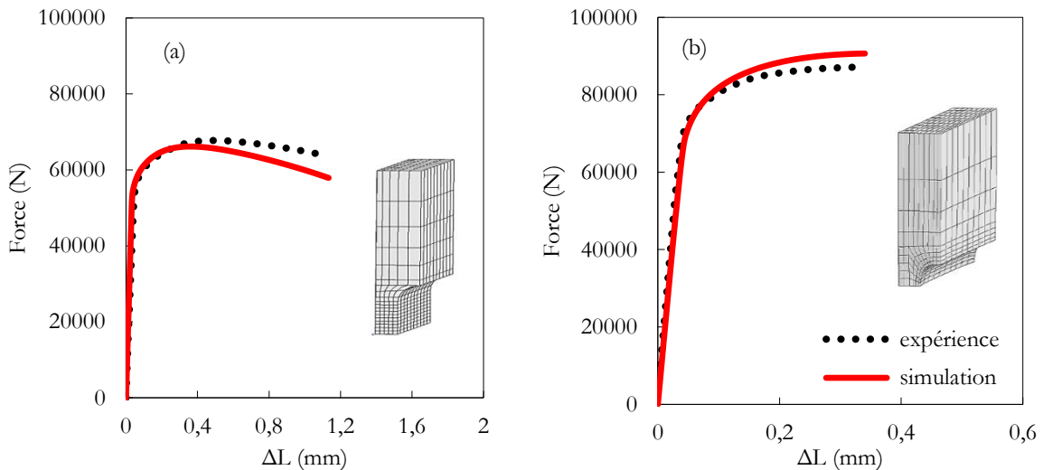
Figure V.2 : Résultats des calculs numériques réalisés pour les essais de traction à la température ambiante des éprouvettes : a) DP et b) DPU, d'après Tioguem, 2016 [2] , microstructure 130P. Les maillages correspondant aux deux géométries sont également fournis pour chacune des figures.
