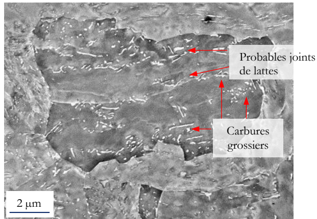
Figure II.19 : Probable paquet de bainite supérieure observé en électrons rétrodiffusés dans le 130M
