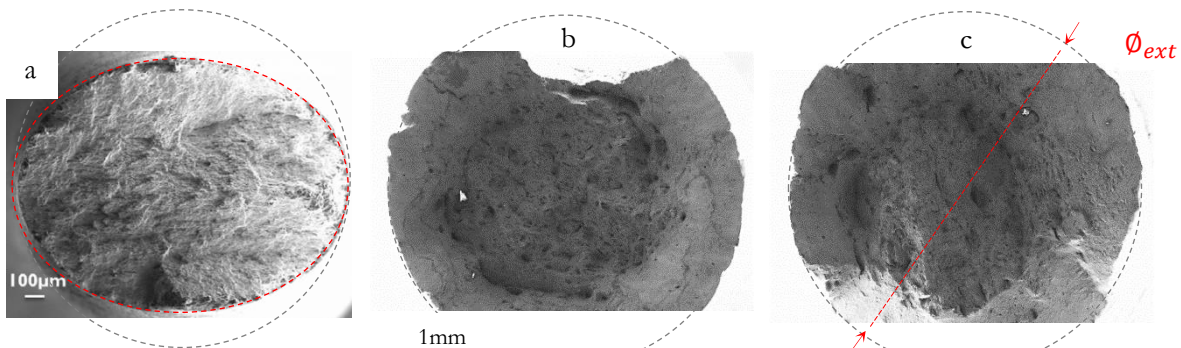
Figure III.13 : Vue macroscopique des faciès de rupture de traction en post-mortem : a) Striction elliptique à 700°C d'un acier 12Cr-ODS [8], b) 130P sens T et c) 130P sens L.
