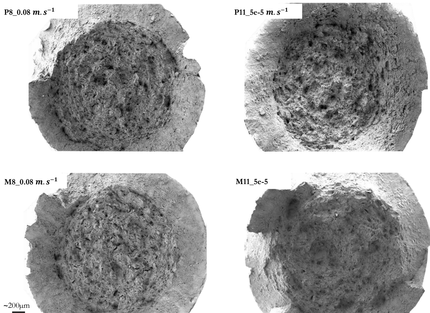
Figure 9 : Vue d'ensemble des faciès de rupture des éprouvettes AE sollicitées à vitesse rapide et en quasistatique.
