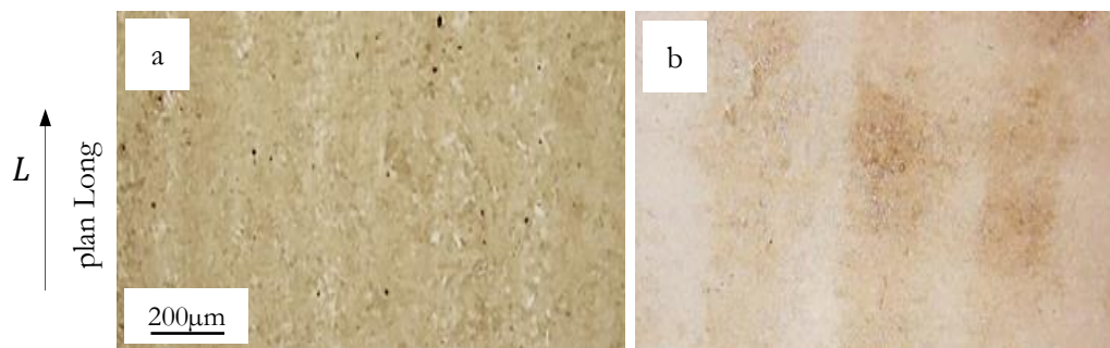
Figure II.15 : Evolution des bandes de ségrégation avec le revenu pour les microstructures : a) 130M, b) 110M et 90M
