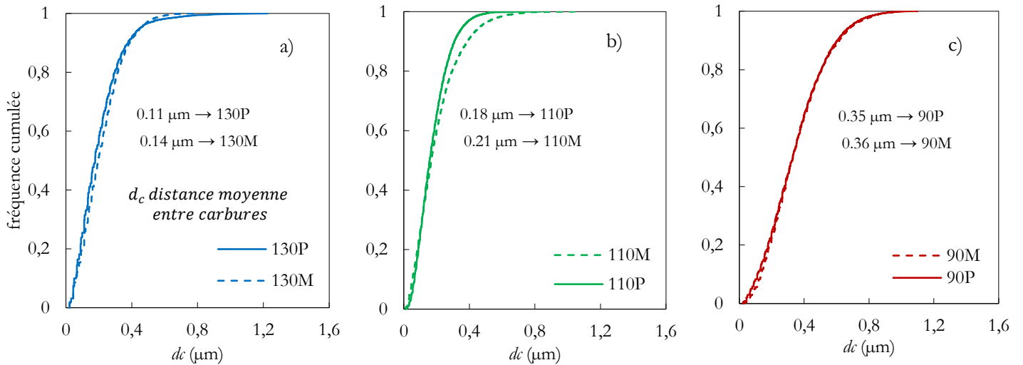
Figure II.32 : Distribution des distances intercarbures ( d_c ) pour les microstructures des configurations : a) 130ksi, b) 110ksi et c) 90ksi
