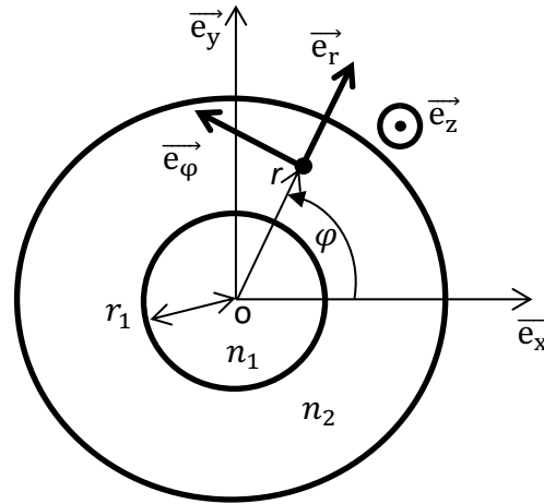
Figure 2.3 : Section droite dans une fibre optique à saut d'indice représentée en coordonnées polaires cylindriques.
