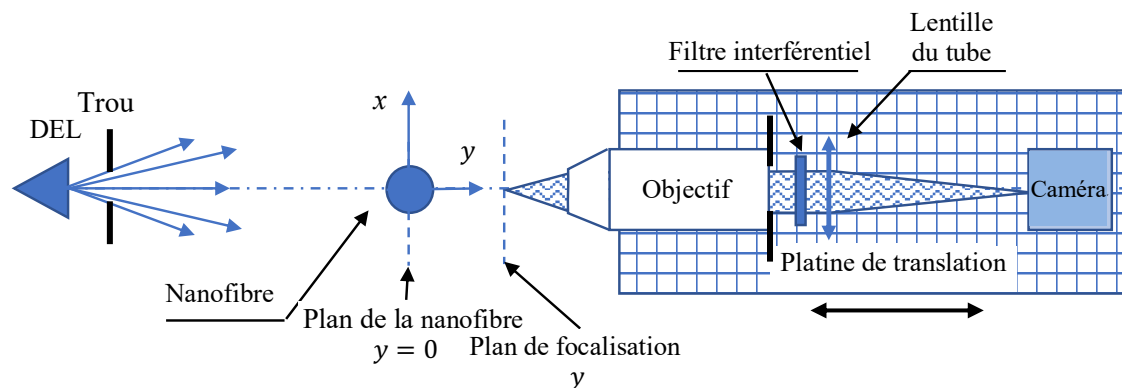
Figure 5.3 : Schéma du microscope.
