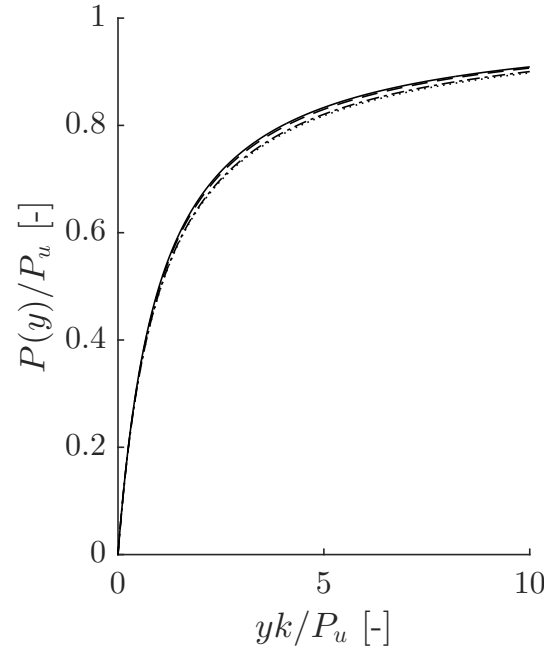
(d) for hyperbolic P - y curve
