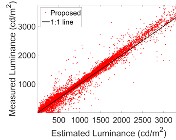
(b) Luminance mesurée par rapport à la luminance estimée
