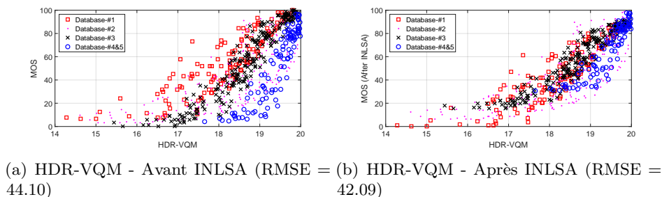
Figure B.8 – Diagrammes des scores MOS par rapport aux scores objectifs de qualité pour le HDR-VQM avant et après l’alignement INLSA. Afin de comparer quantitativement le diagramme de dispersion, l’erreur quadratique moyenne (RMSE - root mean squared error) des données est rapportée pour chaque cas.
