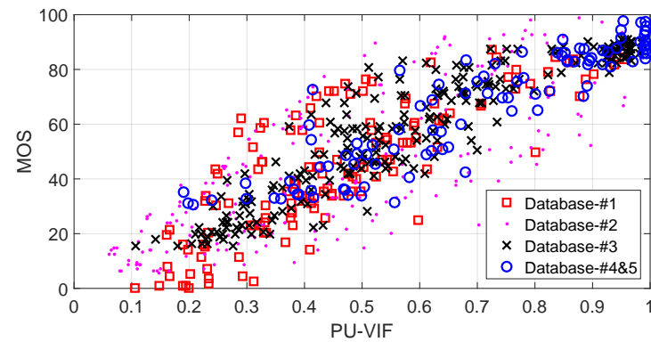
(d) PU-VIF - After INLSA (RMSE = 57.96)
