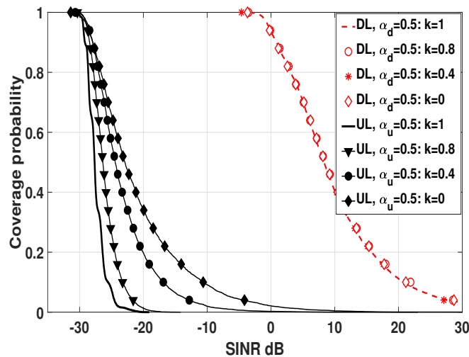
Figure 5 – Probabilité de couverture en DL et en UL pour un réseau macro avec différent facteur de control de puissance fractionnel.
