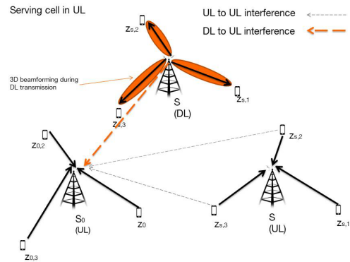
Figure 11 – D-TDD durant la transmission en UL
