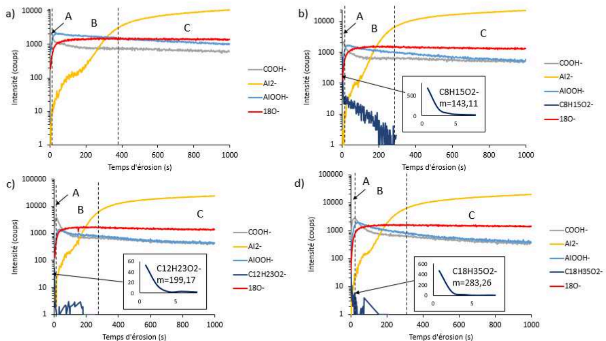
Figure V-5 : Profils réalisés sur les surfaces d'aluminium a) référence immergée 1h dans l'éthanol b) échantillon immergé 1h dans C8 c) échantillon immergé 1h dans C12 d) échantillon immergé 1h dans C18.
