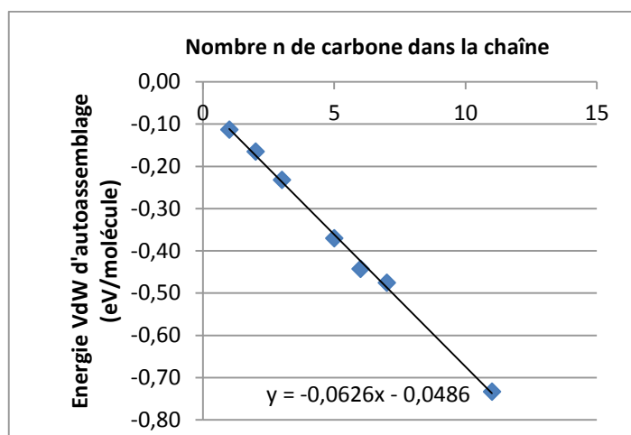
Figure IV-4 : Energie VdW de formation des couches organiques en fonction du nombre n de carbones dans la chaîne alkyle.
