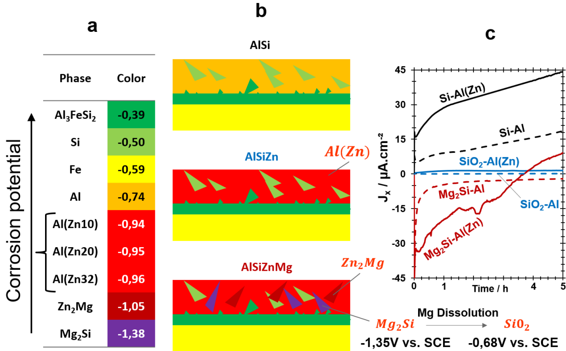
Figure 11 : (a) Phases triées par potentiel de corrosion dans une solution aqueuse de NaCl 1 % massique. De Si en vert clair (-0,170 V vs. SCE) à \text{Mg}_2\text{Si} en violet (-1,35 V vs. SCE). (b) Schéma des microstructures de AlSi, AlSiZn et AlSiZnMg avec échelle de couleur. (c) Courant de couplage galvanique entre Si et Al ou Al(Zn32) dans une solution de NaCl 1 % massique.
