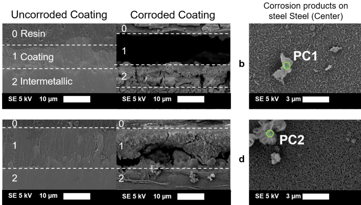
Figure 8 : Les images électroniques secondaires d'arrêtes coupées d'aciers revêtus d' (a) AlSiZn et (b) AlSiZnMg après 48h d'immersion dans une solution aqueuse NaCl 1 % massique à pH initial 7. 0: résine; 1: Revêtement; 2: Intermétallique.
