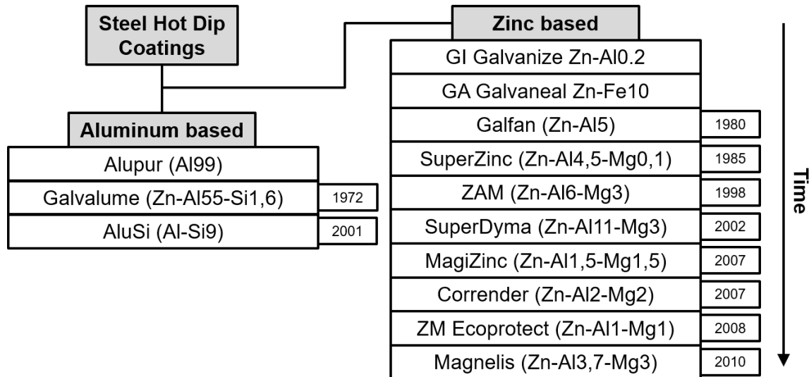
Figure 1 : Revêtements anticorrosion à base d'aluminium (Al-based) ou de zinc (Zn-based) utilisés dans l'industrie (Compositions données en pourcentage massique)
