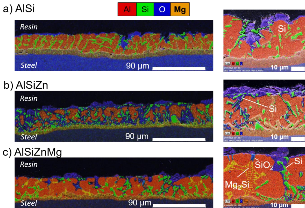
Figure 3 : Cartes EDS montrant la distribution des produits de corrosion après 12 cycles de test VDA 233-102 dans les tranches d'aciers revêtus par (a) AlSi, (b) AlSiZn et (c) AlSiZnMg.
