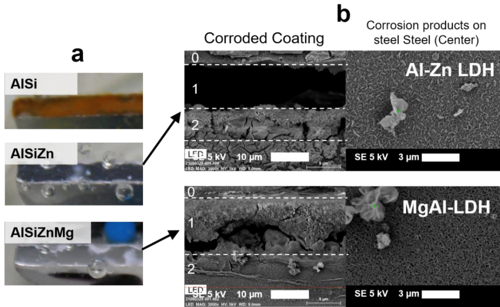
Figure 13 : (a) Aspect des arêtes de coupe typiques des revêtements AlSi, AlSiZn, AlSiZnMg après 48h d'immersion dans une solution aqueuse de NaCl 1 % en masse à pH initial 7. (b) Imagerie en électrons secondaires de bord coupés d'aciers revêtus par AlSiZn et AlSiZnMg après 48h d'immersion dans une solution aqueuse de NaCl 1 % en masse à pH initial 7. 0: résine; 1: Revêtement; 2: Intermétallique.
