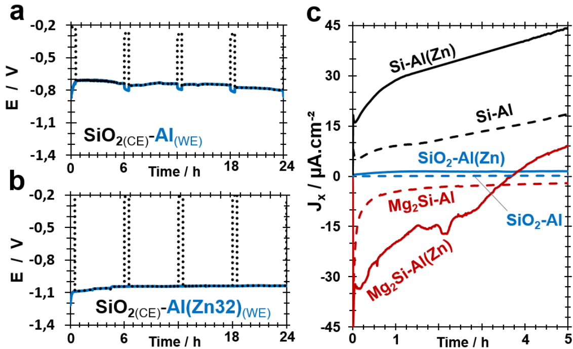
Figure 7 : Potentiels libres de phases pures pendant les essais de couplage pour (a) SiO 2 -Al et (b) SiO 2 -Al (Zn32) dans une solution aqueuse de NaCl 0,172 M. (c) Courant de couplage entre les phases contenant du silicium et Al ou Al (Zn32) dans une solution aqueuse de NaCl 0,172 M.
