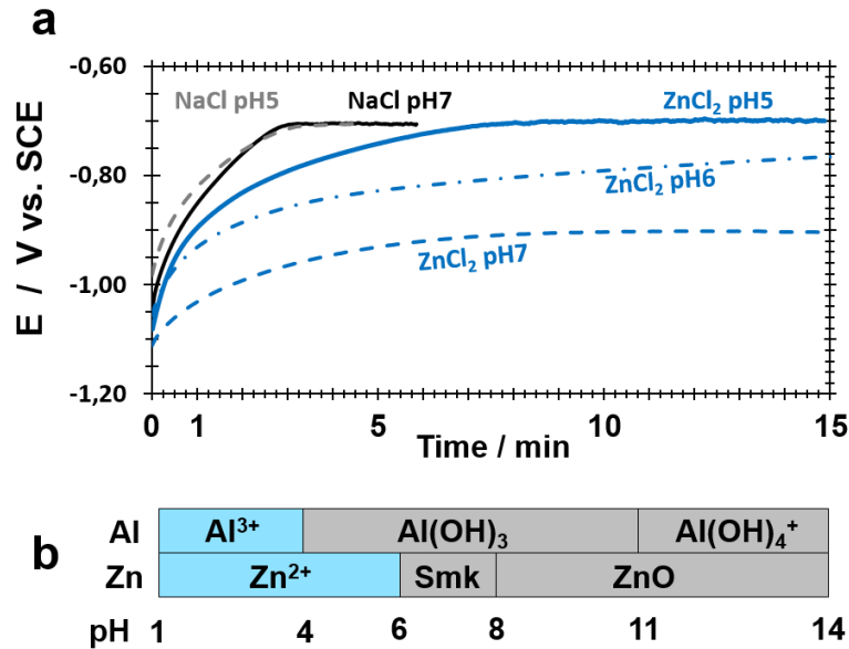
Figure 6 (a) Potentiel en circuit ouvert de l'aluminium pur en fonction du temps dans une solution aqueuse de NaCl 0,172 M ou ZnCl_2 0,086 M à pH 5 à 7 (ajusté avec une solution aqueuse de NaOH 1 M). (b) Espèce prédominante simulée contenant Al / Zn
