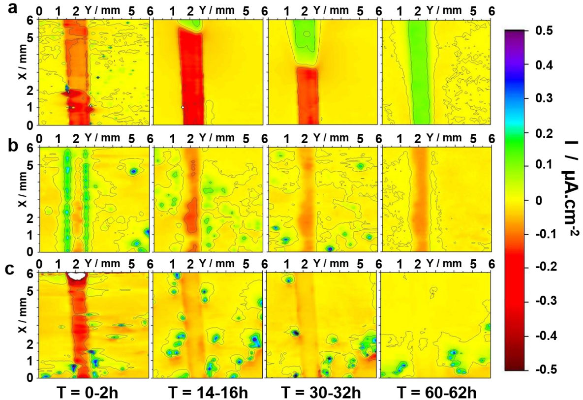
Figure 9 : Cartographie par électrode vibrante en continu d'aciers revêtus par (a) AlSi (b) AlSiZn et (c) AlSiZnMg (rayés) dans NaCl 100 mg.L -1 .
