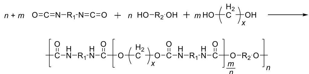
Figure 1. Structure générale des PU linéaires, monophasés ( m = 0 ) et à phases séparées ( m = 1, 2 ) à l'échelle micrométrique. Les segments rigides et flexibles sont distribués statistiquement.
