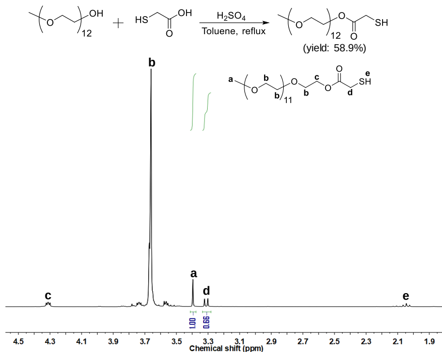
Figure 13. Schéma synthétique et spectre RMN ^1\text{H} du mPEG 12 -SH.
