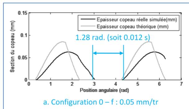
Figure I-57 : Estimation des moments d'interruption de la coupe sur la simulation de la hauteur de copeau (Jallageas 2013).
