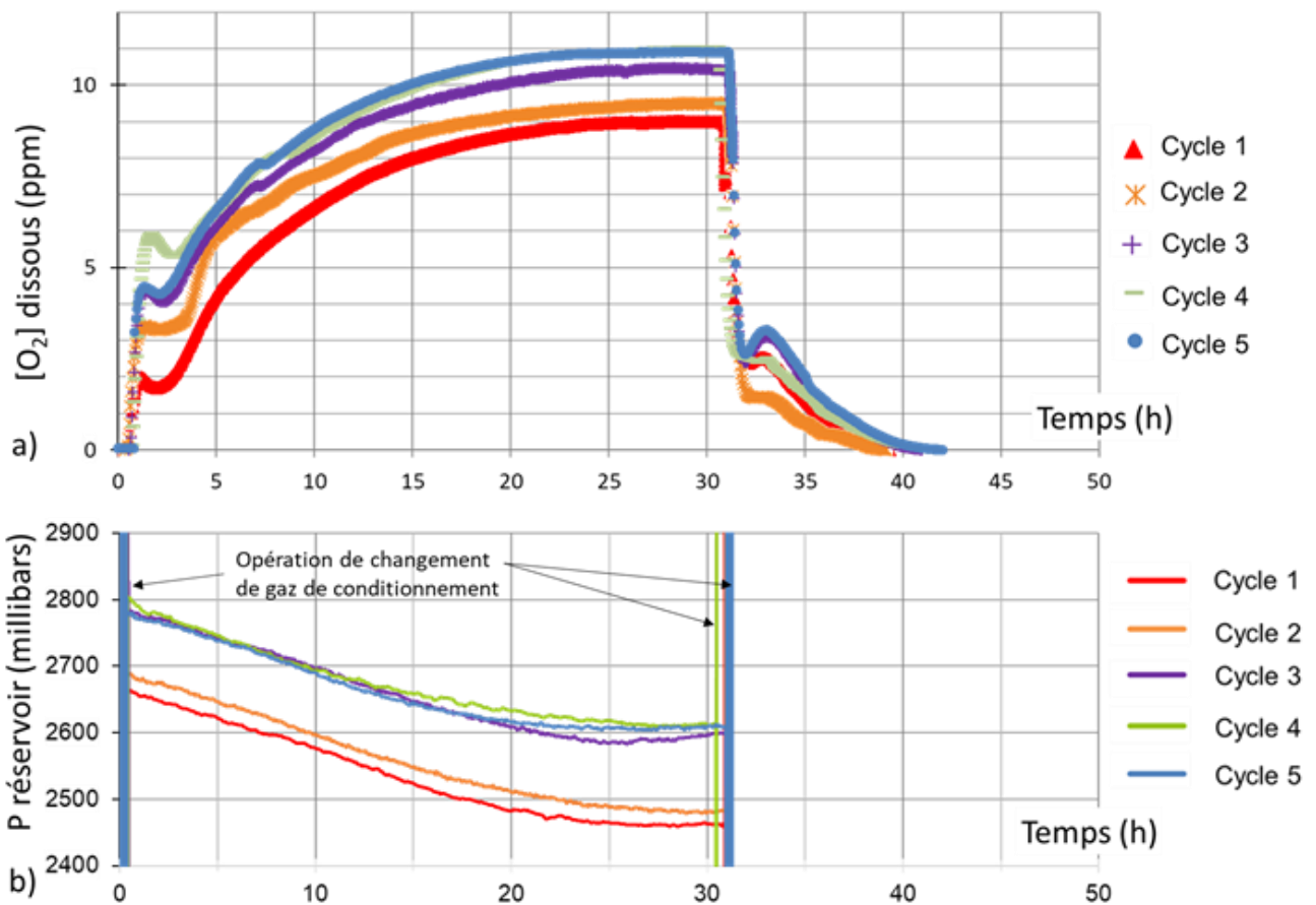
Figure 81 Superposition : a) de la teneur en oxygène dissous et b) de la pression dans le réservoir de milieu pour les 5 cycles de l'essai avec transitoires oxygénés T1. Pour chaque cycle, t = 0 correspond au début du changement de gaz de conditionnement ( H_2 \rightarrow air synthétique). Le changement de gaz (air synthétique \rightarrow H_2 ) a lieu vers t = 31h
