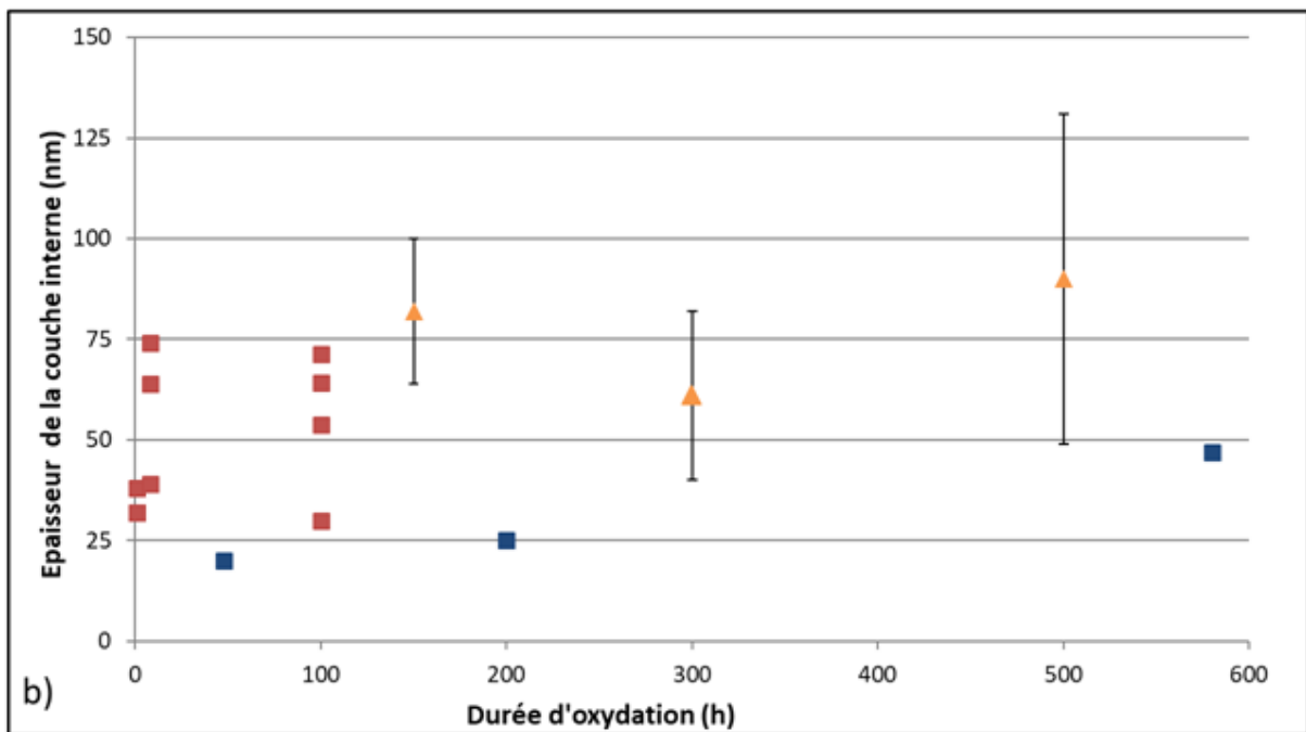
Figure 7 Épaisseur de la couche interne en fonction du temps pour trois aciers inoxydables 316L à l'état hypereutecté oxydés en milieu primaire REP nominal à 320°C et 325°C, d'après Bach, Dumerval et Matthews (Bach, 2018 ; Dumerval, 2014 ; Matthews, 2019). a) Cinétique complète, et b) Valeurs pour les premières centaines d'heures. Les résultats de Dumerval et Matthews correspondent à une mesure ponctuelle de l'épaisseur. Les points de Matthews correspondent à l'épaisseur maximale. Au contraire, les résultats de Bach sont des valeurs moyennes d'épaisseur obtenues à partir de plusieurs dizaines de mesures ponctuelles.
