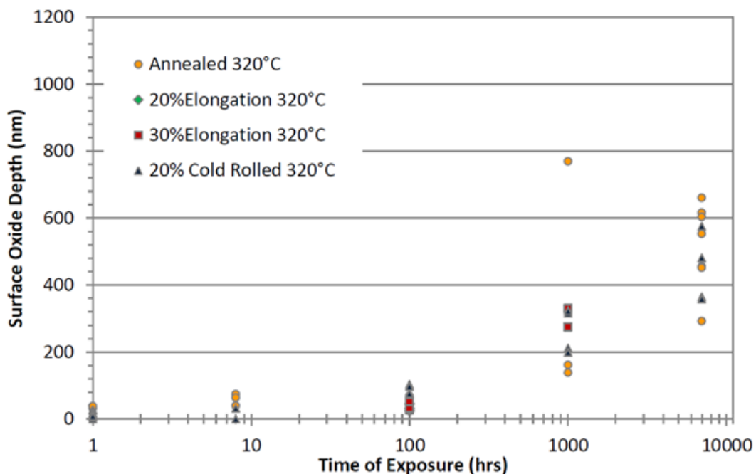
Figure 20 Epaisseur de la couche interne d'oxyde formée à 320°C sur un acier inoxydable 316L à l'état hypereffé ou prédéformé (par traction ou par laminage à froid). D'après (Matthews, 2019).
