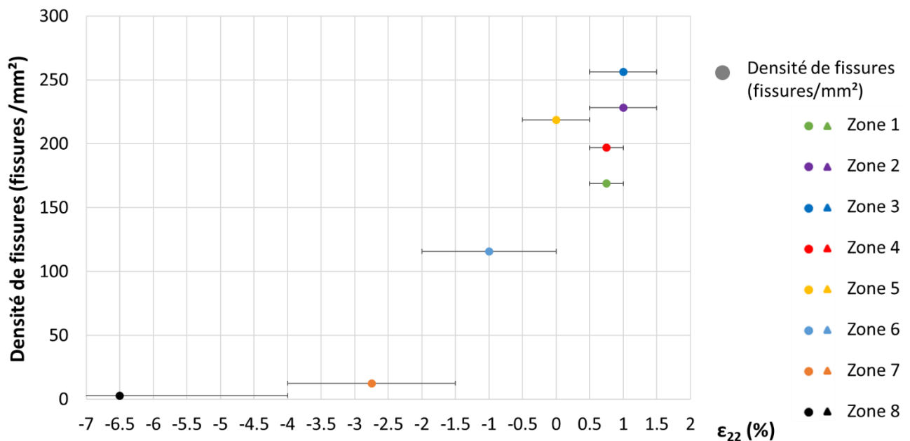
Figure 75. Densité de fissures en surface en fonction de \epsilon_{22}
