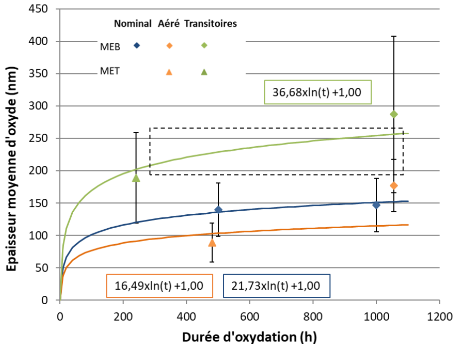
Figure 143 Cinétiques d'oxydation obtenues à 340°C en milieu primaire nominal, aéré, et avec transitoires oxygénés sur des coupons non prédéformés.
