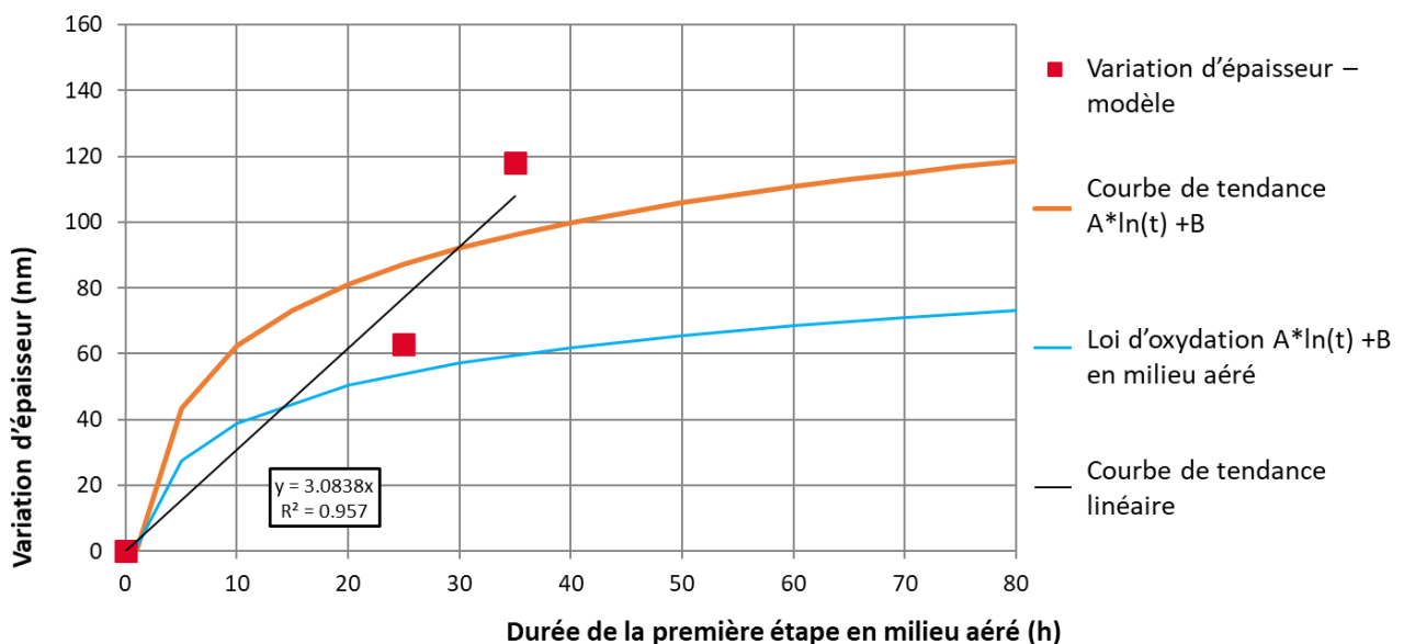
Figure 145 Variation de l'épaisseur de la couche interne pendant la première étape en milieu aéré.
