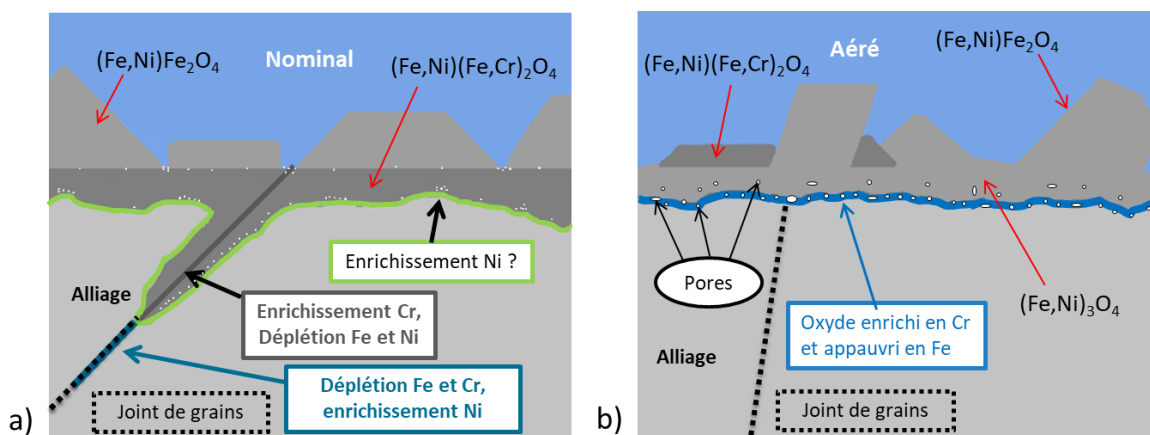
Figure 133 Schémas récapitulatifs de la couche d'oxyde formée en surface de la phase austénitique pour les coupons non prédéformés oxydés en : a) milieu primaire nominal ; b) milieu primaire aéré.
