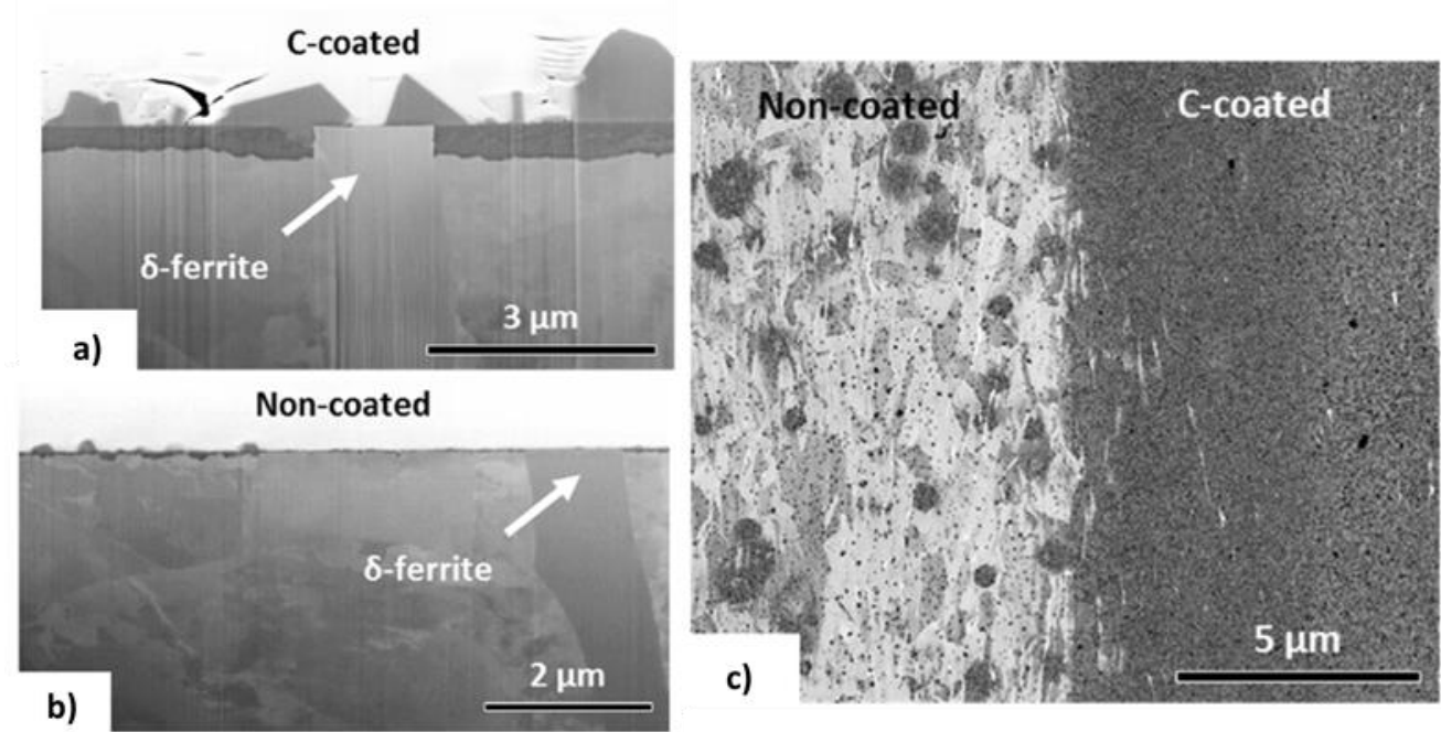
Figure 22 Micrographies MEB de coupons issus d'une tôle forgée à chaud et oxydés en milieu primaire nominal à 300°C. a) et b) Vues en coupe des couches d'oxyde sur deux échantillons avec et sans dépôt de carbone, respectivement et c) Vue de surface d'un coupon pour lequel un dépôt de carbone est déposé sur une moitié de l'échantillon avant oxydation. D'après (Mukahiwa et al., 2019).
