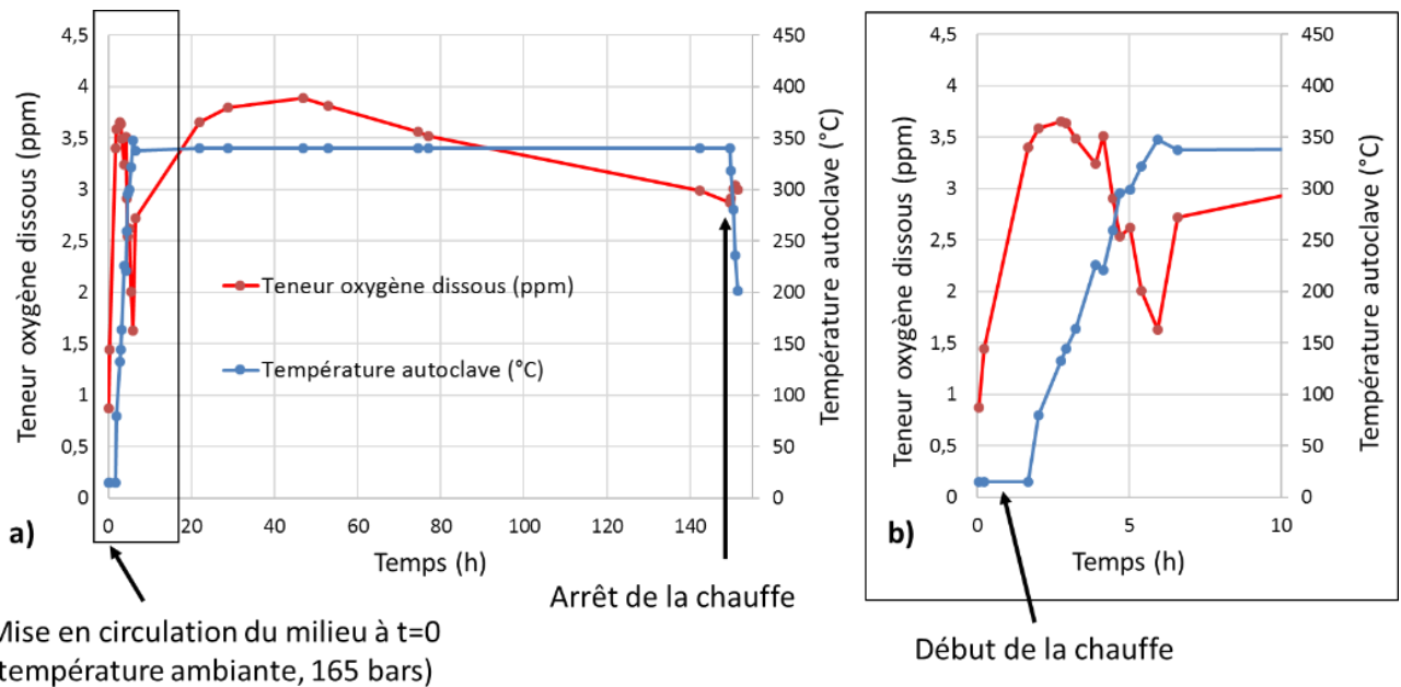
Figure 51. Suivi en fonction du temps de la teneur en oxygène dissous mesurée par la sonde et de la température de l'autoclave : a) pendant toute la durée de l'essai préliminaire ; b) zoom sur les dix premières heures.
