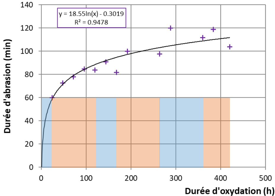
Figure 142 Durées d'abrasion (analyses XPS) en fonction de la durée d'oxydation, telles que le signal de l'oxygène atteint la moitié de sa valeur maximale. Les rectangles bleus et orange représentent respectivement les étapes en milieu nominal et aéré de l'essai. D'après (Xu et al., 2015). Les essais sont réalisés à 290°C.
