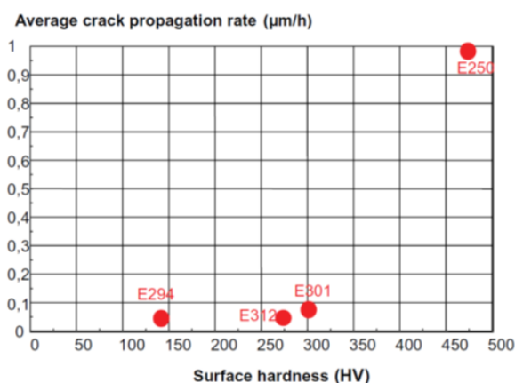
Figure 27 Vitesse de fissuration en fonction de la dureté initiale d'éprouvettes prédéformées par grenillage testées en traction lente ( 1,5 \times 10^{-7} \text{ s}^{-1} , 360°C). D'après (Raquet et al., 2005).
