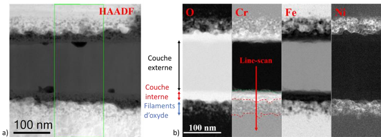
Figure 12 Oxydes formés sur les flancs d'une fissure intergranulaire de CSC en milieu primaire nominal : a) Micrographie STEM-HAADF et b) Cartographies EELS (compositions relatives) correspondantes pour l'oxygène, le chrome, le fer, et le nickel. D'après (Shen et al., 2019).
