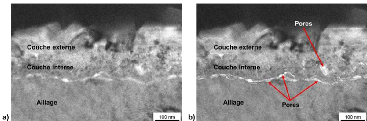
Figure 95 Micrographies MET en fond clair des couches d'oxyde de surface pour le coupon C10 (480h à 340°C en milieu primaire aéré) : a) Image focalisée ; b) Image défocalisée, mettant en évidence les pores.
