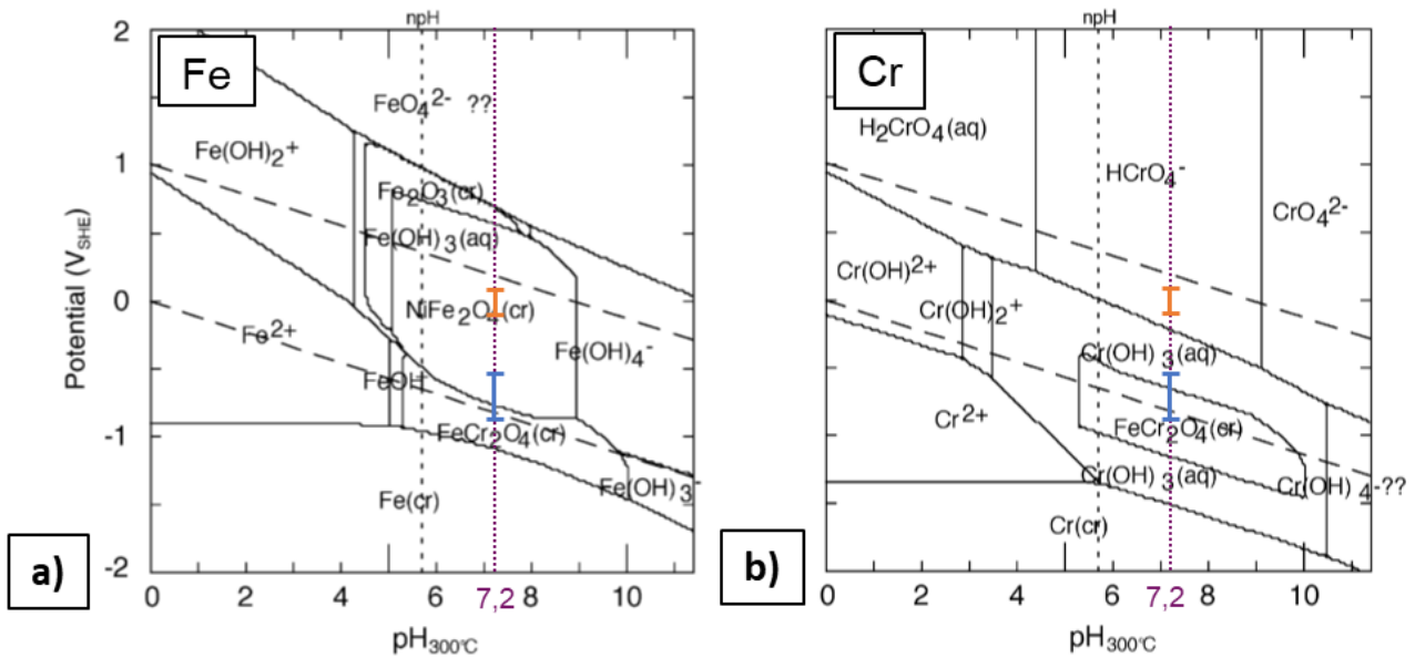
Figure 36 Diagrammes de Pourbaix pour le système Fe-Cr-Ni-H 2 O-H 2 à 300°C, avec [Cr]_{aq}=[Fe]_{aq}=[Ni]_{aq}=10^{-8} mol/L, pour les espèces stables du Fe (a) et du chrome (b). D'après (Beverkog et al., 1999). Les points bleu et orange correspondent aux conditions du milieu primaire REP nominal et aéré, respectivement. Nous considérons que le potentiel des aciers inoxydables est de -0,675 \pm 0,175 V/ESH en milieu primaire nominal, et de 0 \pm 0,1 V/ESH en milieu primaire aéré, sur la base de la présente revue bibliographique.
