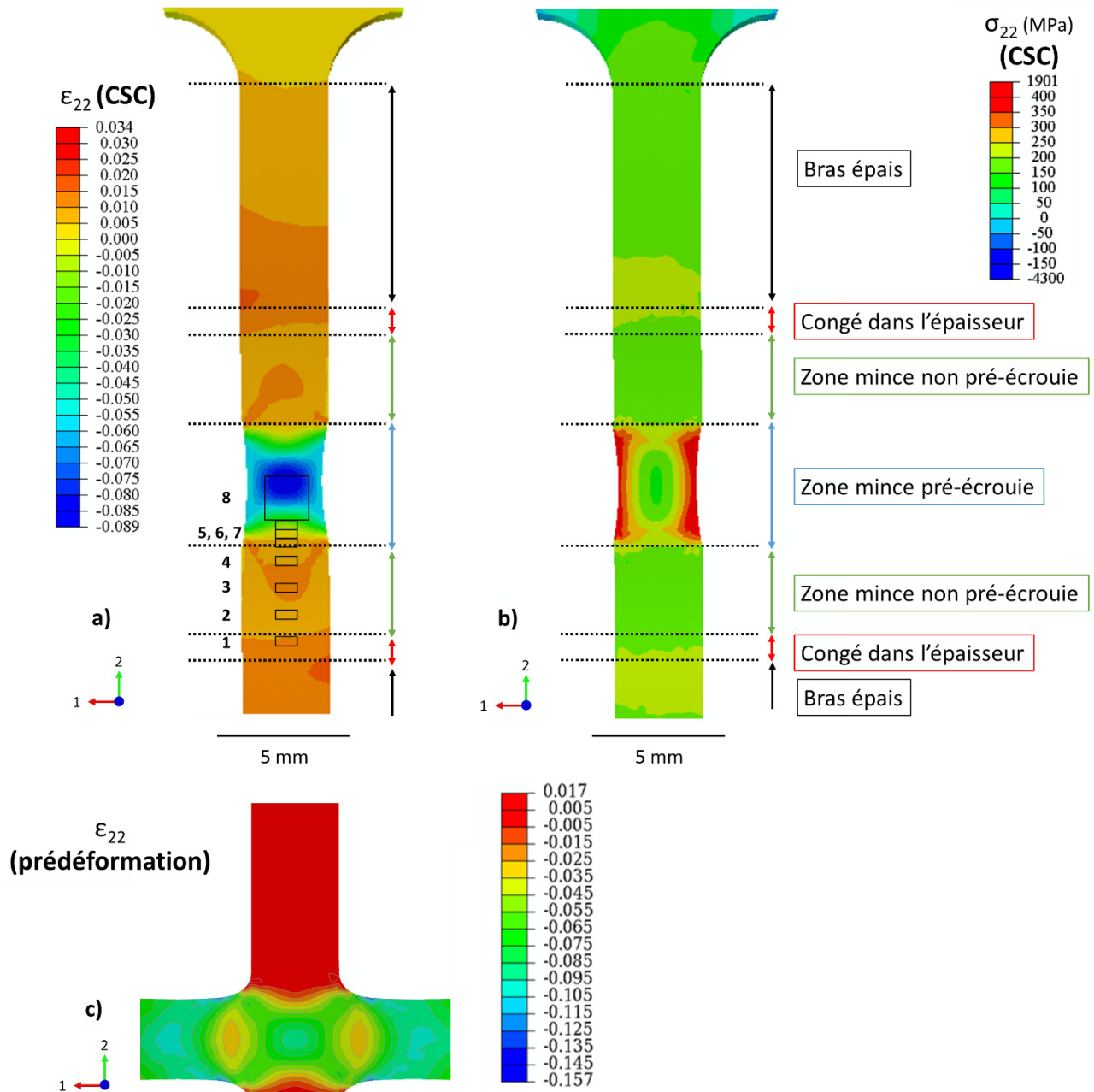
Figure 74. Cartographies de la déformation plastique (a) et de la contrainte (b) cumulées selon 22, calculées à la fin de l'essai de CSC, et de la déformation selon 22 à la fin de l'étape de prédéformation (c). Les 8 zones dépouillées pour la quantification du réseau de fissures en surface sont replacées sur la cartographie a).
