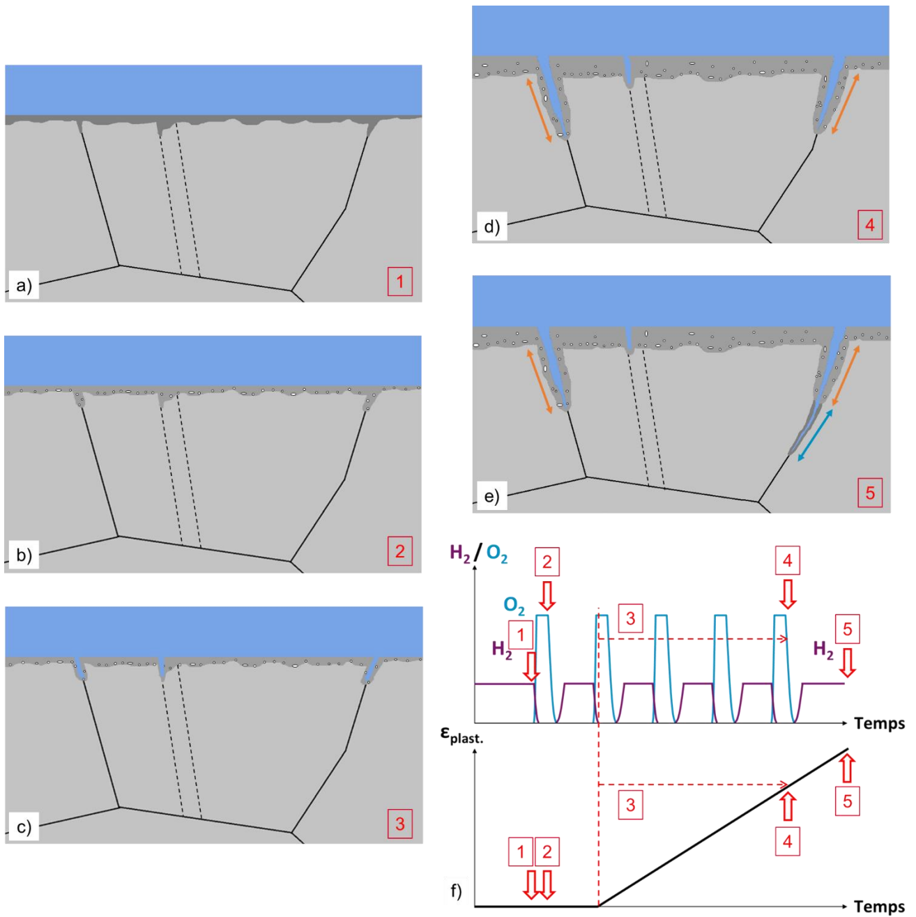
Figure 147 Scénario proposé pour l'amorçage de fissures intergranulaires de CSC, lors de l'essai de CSC avec transitoires oxygéné de cette étude : a) à e) étapes 1 à 5 du scénario ; f) Evolutions de la teneur en hydrogène et oxygène dissous et de la déformation plastique, en fonction du temps ; les étapes du scénario sont encadrées en rouge.
