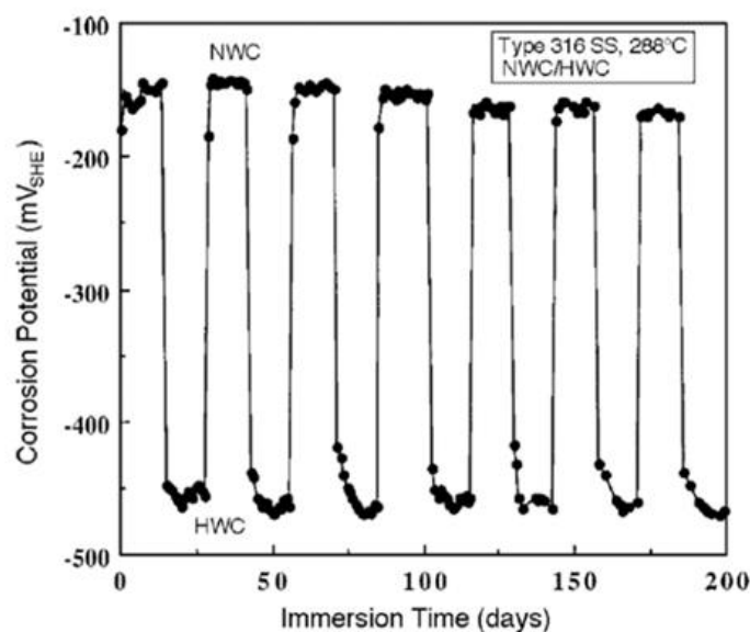
Figure 32 Potentiel de corrosion d'un acier 316 oxydé alternativement en milieu REB NWC et HWC, d'après (Kim, 1995).
