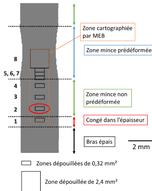
Figure 68 Emplacements des zones où la quantification du réseau de fissures en surface a été effectuée. Les résultats sont détaillés pour la zone n°2.
