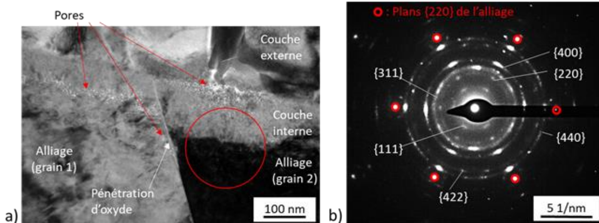
Figure 100 : a) Micrographie MET en fond clair sous-focalisée de l'oxyde formé en surface et le long d'un joint de grains du coupon C2 (milieu primaire nominal, 500 h à 340°C) ; b) Cliché de diffraction électronique acquis à l'interface métal-oxyde interne (cercle rouge de l'image a). Les anneaux de diffraction proviennent de l'oxyde interne et les taches cerclées de rouge correspondent aux plans {220} de l'alliage en axe de zone \langle 111 \rangle .
