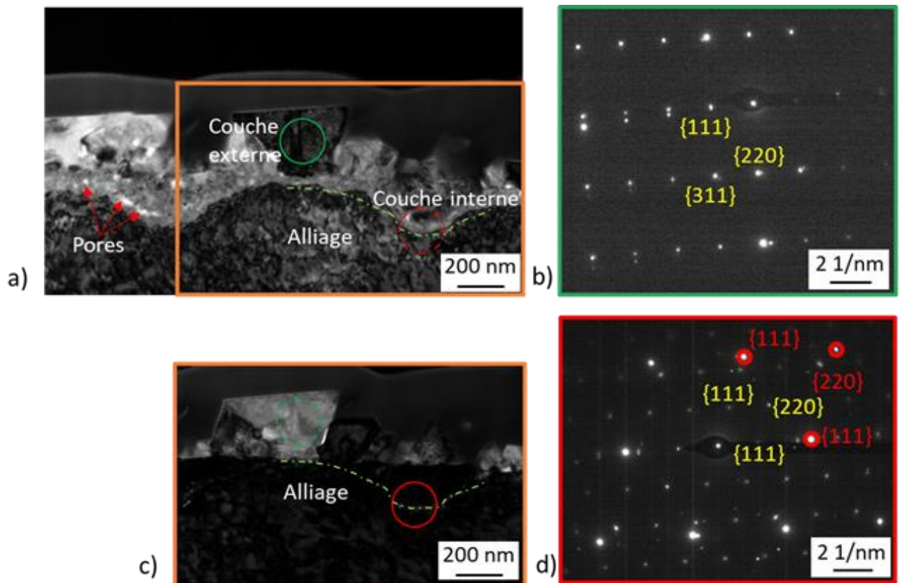
Figure 109 a) Micrographie MET en fond clair défocalisée de la couche d'oxyde de surface du coupon C25 (transitoires oxygénés, 340°C, 240h) ; b) Cliché de diffraction acquis au niveau de la cristallite externe en axe de zone de type \langle 112 \rangle sur l'image a) (cercle vert) ; c) Micrographie MET en fond clair, correspondant au cadre orange sur l'image a), avec la couche interne en axe de zone \langle 011 \rangle ; d) Cliché de diffraction acquis à l'interface alliage/couche interne (cercle rouge de l'image c). Les plans correspondants à l'alliage sont entourés en rouge sur ce cliché.
