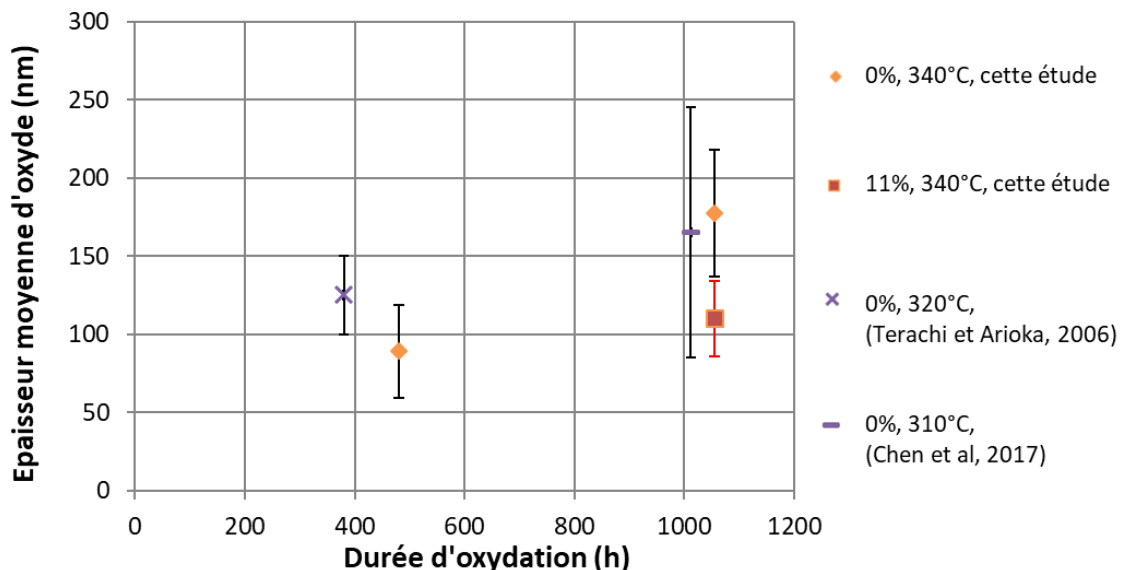
Figure 135 Epaisseur moyenne de la couche interne en fonction de la durée d'oxydation en milieu primaire REP aéré. D'après cette étude, ainsi que (Chen et al., 2017 ; Terachi et al., 2006).
