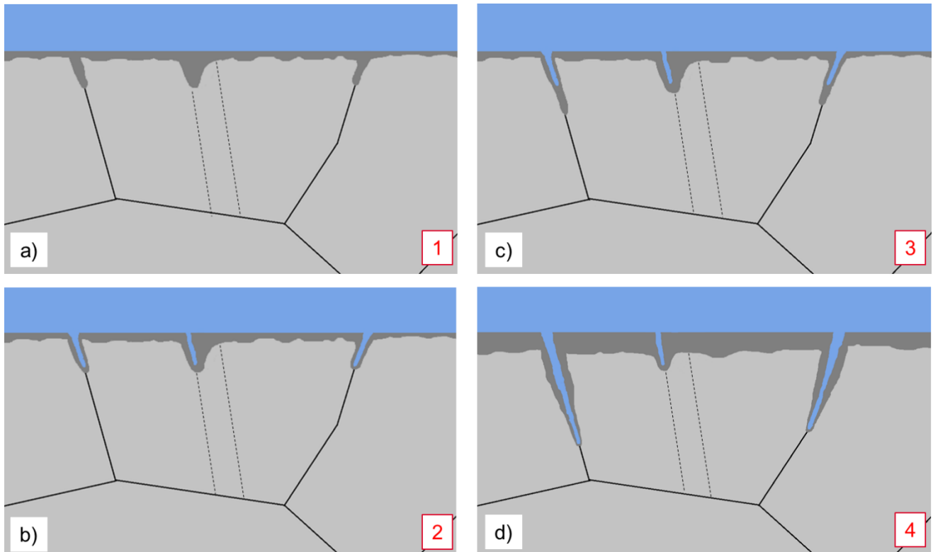
Figure 131 Scénario proposé pour l'amorçage de fissures de CSC en milieu primaire nominal.
