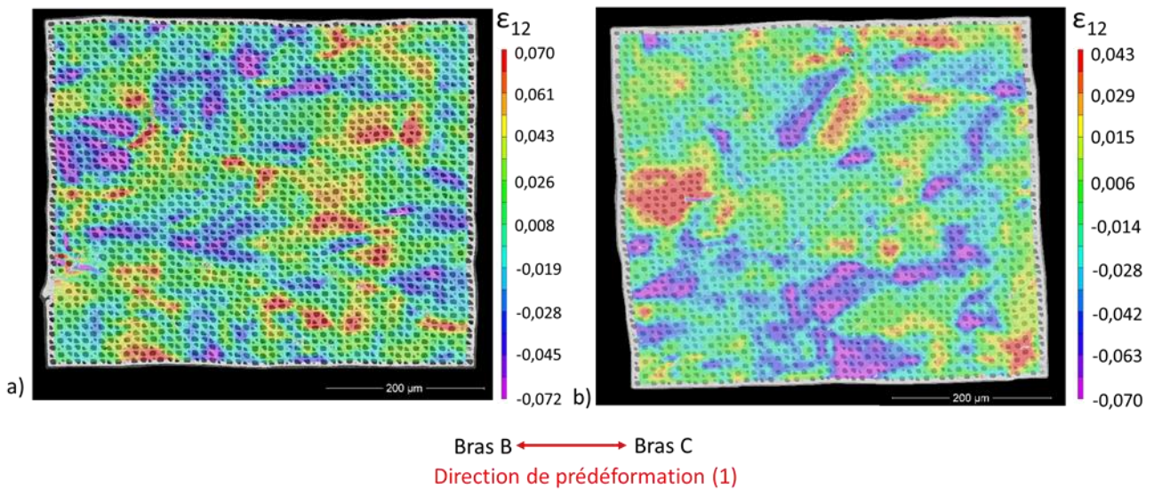
Figure 63 Cartographies de déformation en cisaillement ( \epsilon_{12} ) après l'étape de prédéformation : a) grille S, b) grille V.
