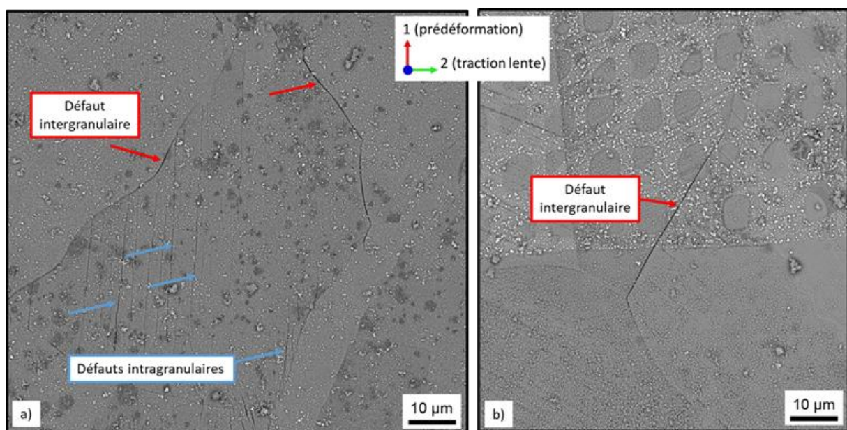
Figure 65. Micrographies MEB en électrons rétrodiffusés de défauts de surface après l'essai de CSC N1 : a) Zone mince pré-déformée. présentant des défauts intergranulaires (flèches rouges) et intragranulaires (flèches bleues). b) Zone centrale, près de la grille V.
