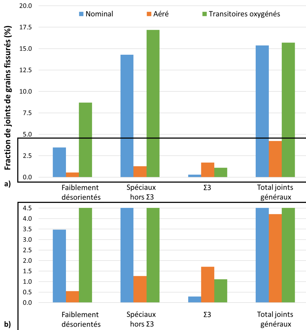
Figure 88 a) Fraction de joints de grains fissurés par CSC en fonction de la nature et de la désorientation des joints de grains, pour les essais de CSC N2, A2, et T1 ; b) Détail de l'histogramme a), correspondant au cadre noir.
