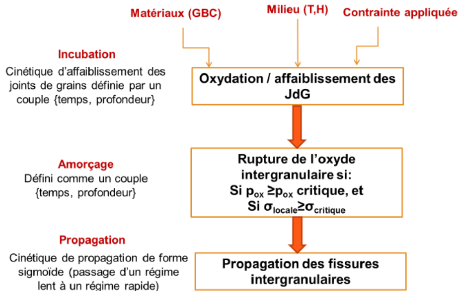
Figure 130 Principe du modèle local de CSC intergranulaire (Caballero Hinostrroza, 2016).
