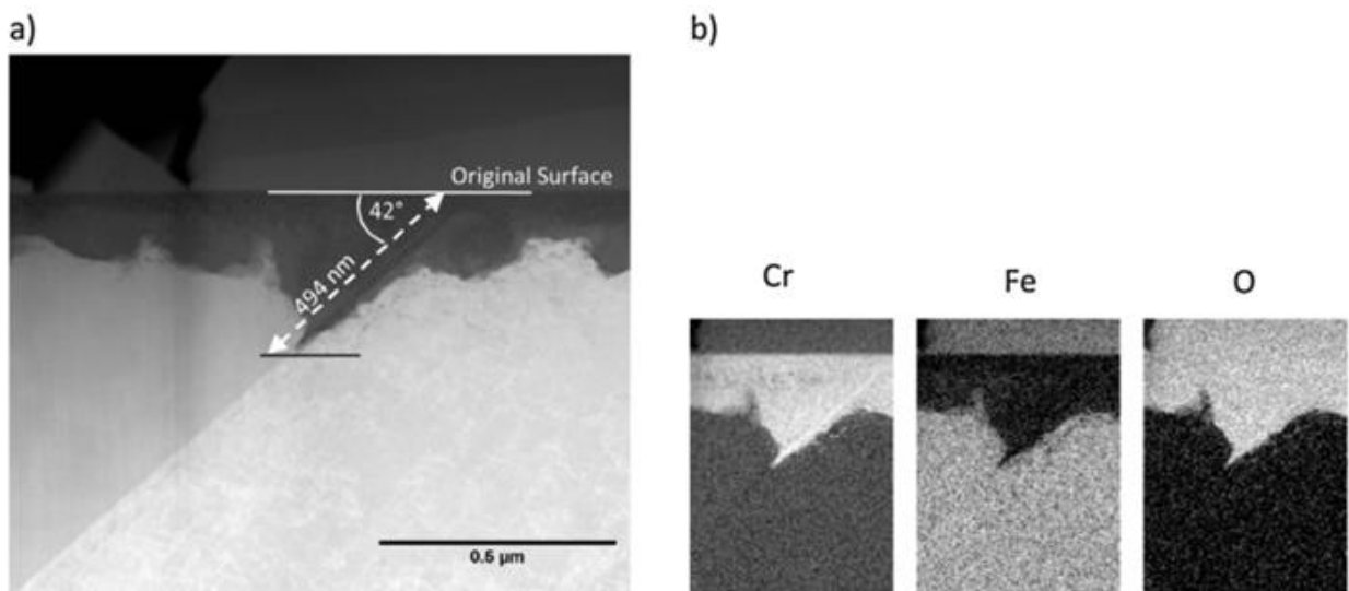
Figure 17 a) Micrographie STEM-HAADF d'une pénétration intergranulaire, échantillon prédéformé (laminage 20% à froid) oxydé 1000h en milieu primaire nominal à 320°C. b) Cartographies EELS associées du chrome, du fer, et de l'oxygène. D'après (Matthews et al., 2017).
