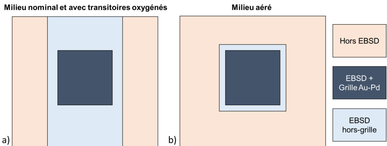
Figure 84 Représentation schématique des zones dépouillées pour déterminer l'effet de l'analyse EBSD et du dépôt de microgrilles d'or-palladium : a) en milieu primaire nominal et avec transitoires et b) en milieu primaire aéré. Dans le cas a), les grilles analysées par EBSD sans correction de tilt sont choisies car la zone couverte par l'analyse EBSD est plus étendue. Dans le cas b) la zone analysée par EBSD sans grille est trop réduite pour pouvoir être dépouillée seule.
