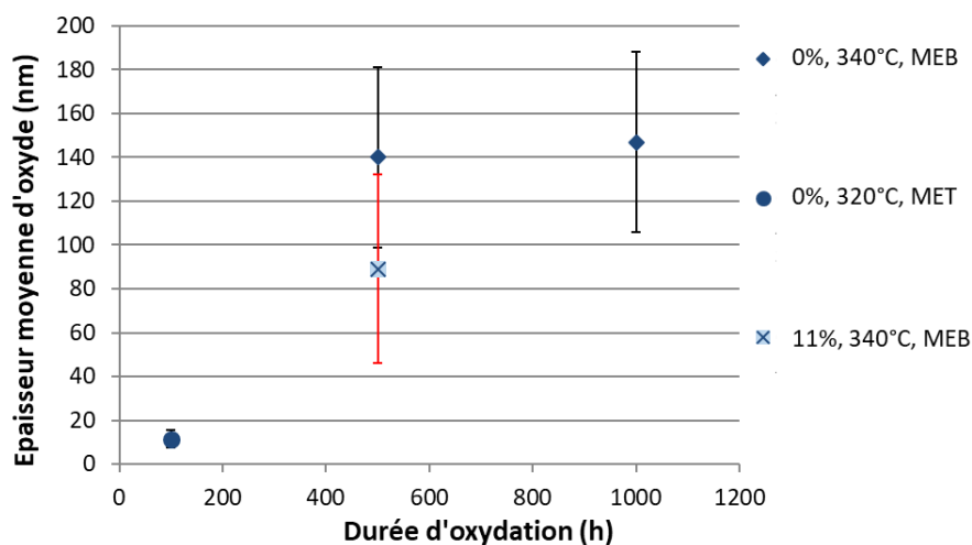
Figure 119 Epaisseur moyenne de la couche interne en fonction de la durée d'oxydation en milieu primaire nominal, mesurée sur des coupons et sur une éprouvette prédéformée à 11% par traction. La barre d'erreur pour l'éprouvette prédéformée est en rouge.
