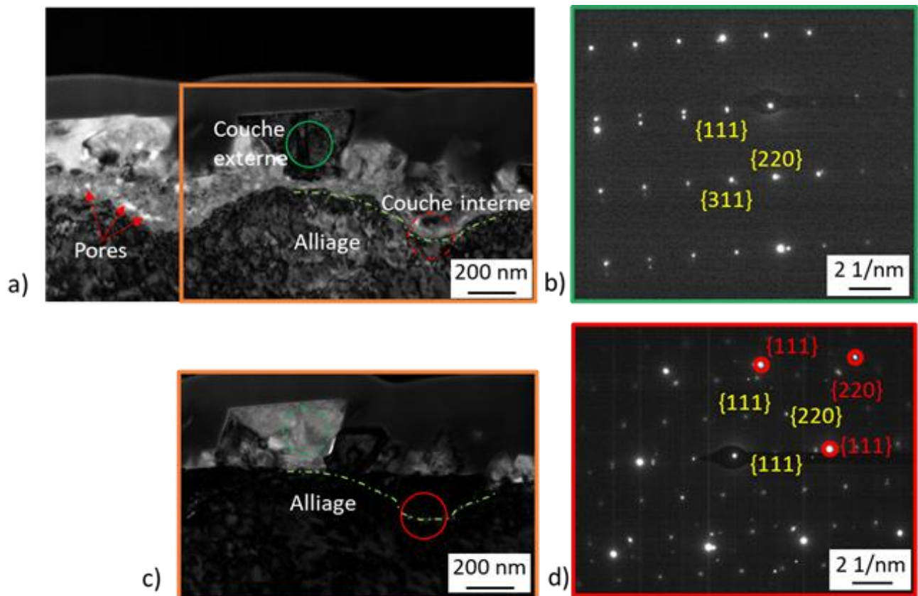
Figure 109 a) Micrographie MET en fond clair défocusée de la couche d'oxyde de surface du coupon C25 (transitoires oxygénés, 340°C, 240h) ; b) Cliché de diffraction acquis au niveau de la cristallite externe en axe de zone de type \langle 112 \rangle sur l'image a) (cercle vert) ; c) Micrographie MET en fond clair, correspondant au cadre orange sur l'image a), avec la couche interne en axe de zone \langle 011 \rangle ; d) Cliché de diffraction acquis à l'interface alliage/couche interne (cercle rouge de l'image c). Les plans correspondants à l'alliage sont entourés en rouge sur ce cliché.
