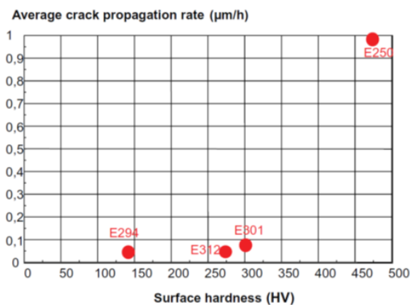
Figure 27 Vitesse de fissuration en fonction de la dureté initiale d'éprouvettes prédéformées par grenillage testées en traction lente ( 1,5 \times 10^{-7} \text{ s}^{-1} , 360^\circ\text{C} ). D'après (Raquet et al., 2005).
