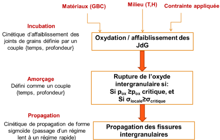
Figure 130 Principe du modèle local de CSC intergranulaire (Caballero Hinostriza, 2016).
