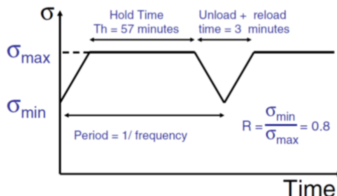
Figure 25 Chargement trapézoïdal utilisé pour les essais d'amorçage de (Huguenin et al., 2013).
