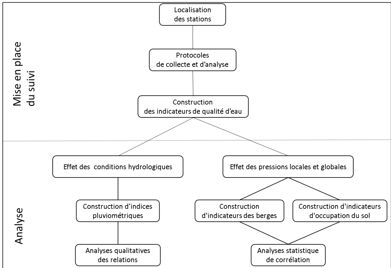
Figure 20. Méthode suivie pour répondre à la question : Les indices réglementaires sont-ils efficaces pour rendre compte de la qualité de l'eau ?
