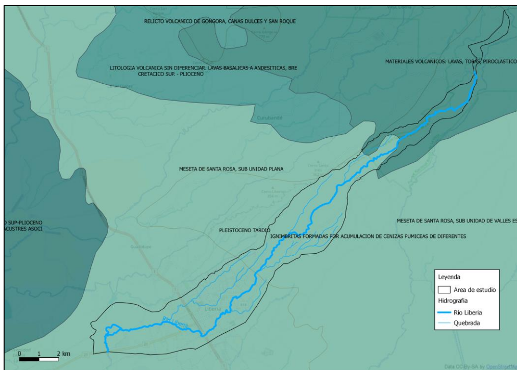
Figure 5. Carte géologique de la zone d'étude.
