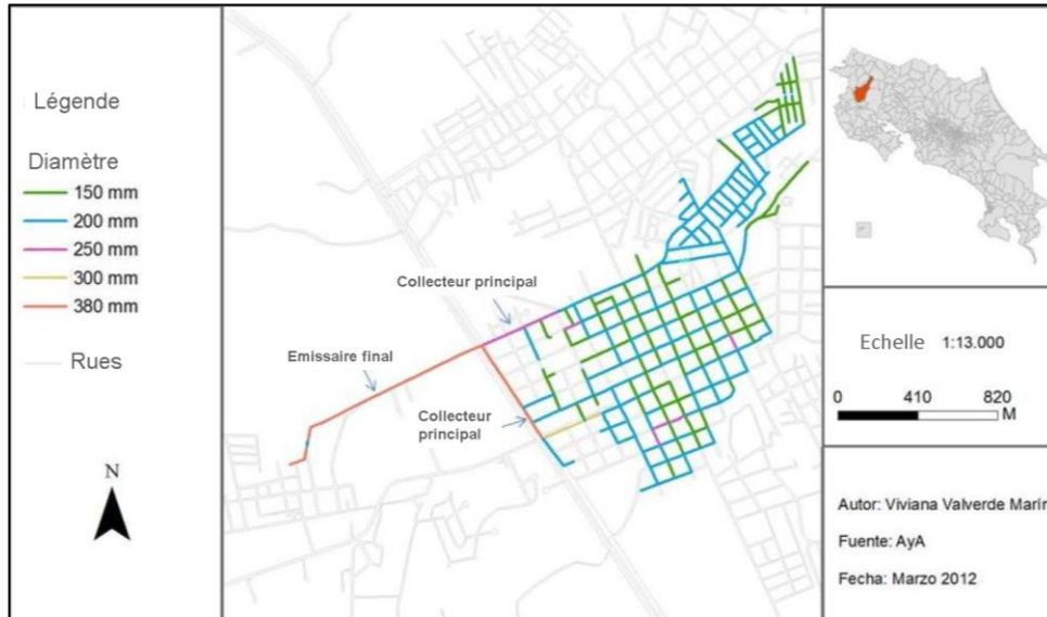
Figure 15. Diamètres du système collectif d'assainissement d'eau usées (Valverde Marin, 2012).
