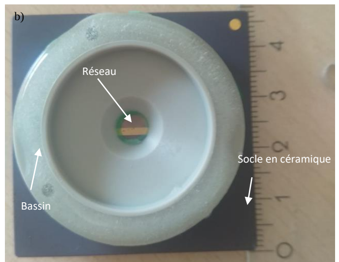
Figure 56 a) Dispositif expérimental de mesure montrant les différentes tensions appliquées à un transistor, b) Photographie d'une puce sur laquelle a été imprimés 48 transistors à effet de champ à base du graphène. La puce est collée sur un socle céramique et un bassin plexiglass permet de déposer un électrolyte de mesure.
