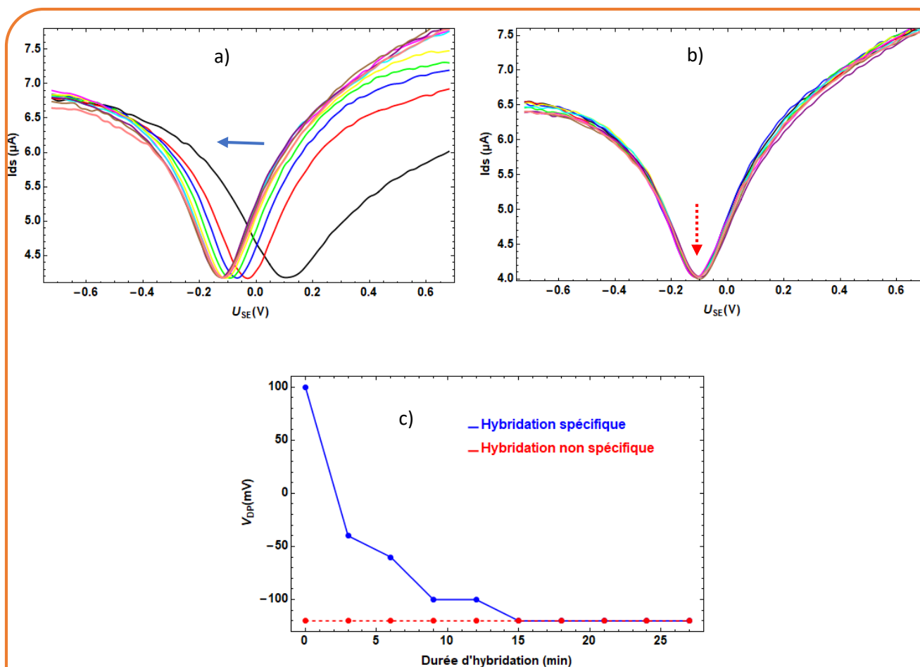
Figure 75 Comportement d'un transistor en temps réel lors de l'hybridation. Les déplacements du point de Dirac avec les cibles complémentaires (a) et avec les cibles non complémentaires (b). et c) les shifts du point de Dirac avec les cibles (en bleu) et les cibles non complémentaires en rouge pointillé V_{ds} = 50\text{mV} , 0.1XPBS
