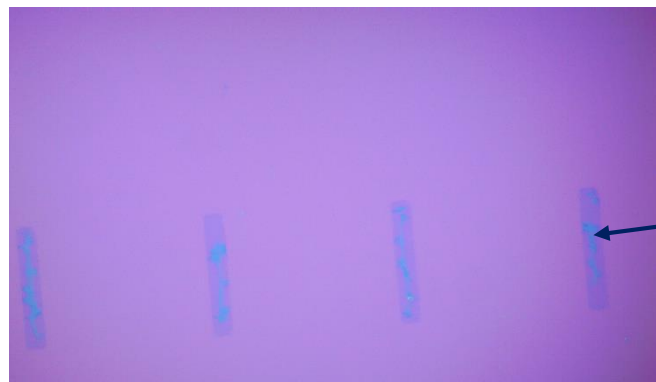
Figure 39. Mise en évidence de la non adhérence de l'alumine au graphène. On voit qu'après le lift-off, les 3nm d'aluminium oxydé s'enlève en partie et expose le graphène à la résine et au développeur qu'on utilisera à la prochaine lithographie
