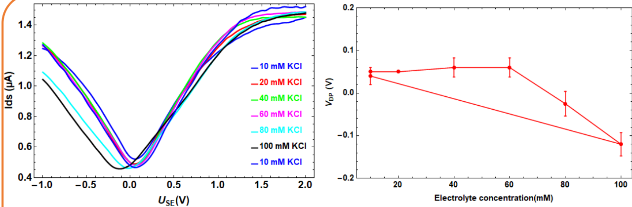
Figure 62. Réponse d'un transistor aux variations de la concentration de l'électrolyte. A gauche, nous avons les caractéristiques I_{ds}(V_g) puis à droite les shifts du point de Dirac
