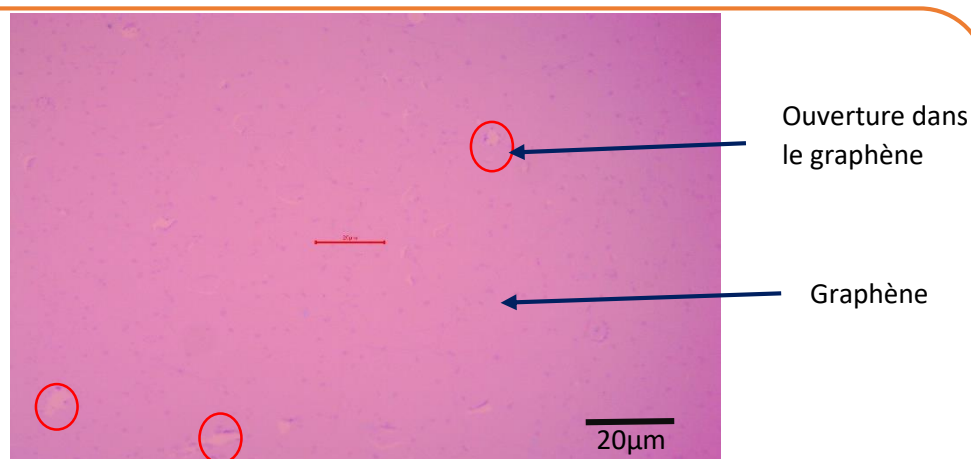
Figure 35. Image d'un transfert de graphène réussi sur du 280 nm de \text{SiO}_2 . Les encadrés en rouge montrent des trous qui peuvent être causés par éclatement des bulles de gaz ou des agressions mécaniques subites par le graphène lors du transfert
