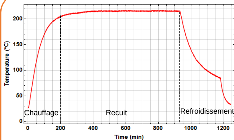
Figure 54 Profil de l'évolution de la température lors d'un recuit
