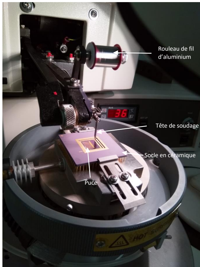
Figure 55 : Photographie de la machine de bonding manuelle « Ball & Wedge bonding antycip Technologies »
