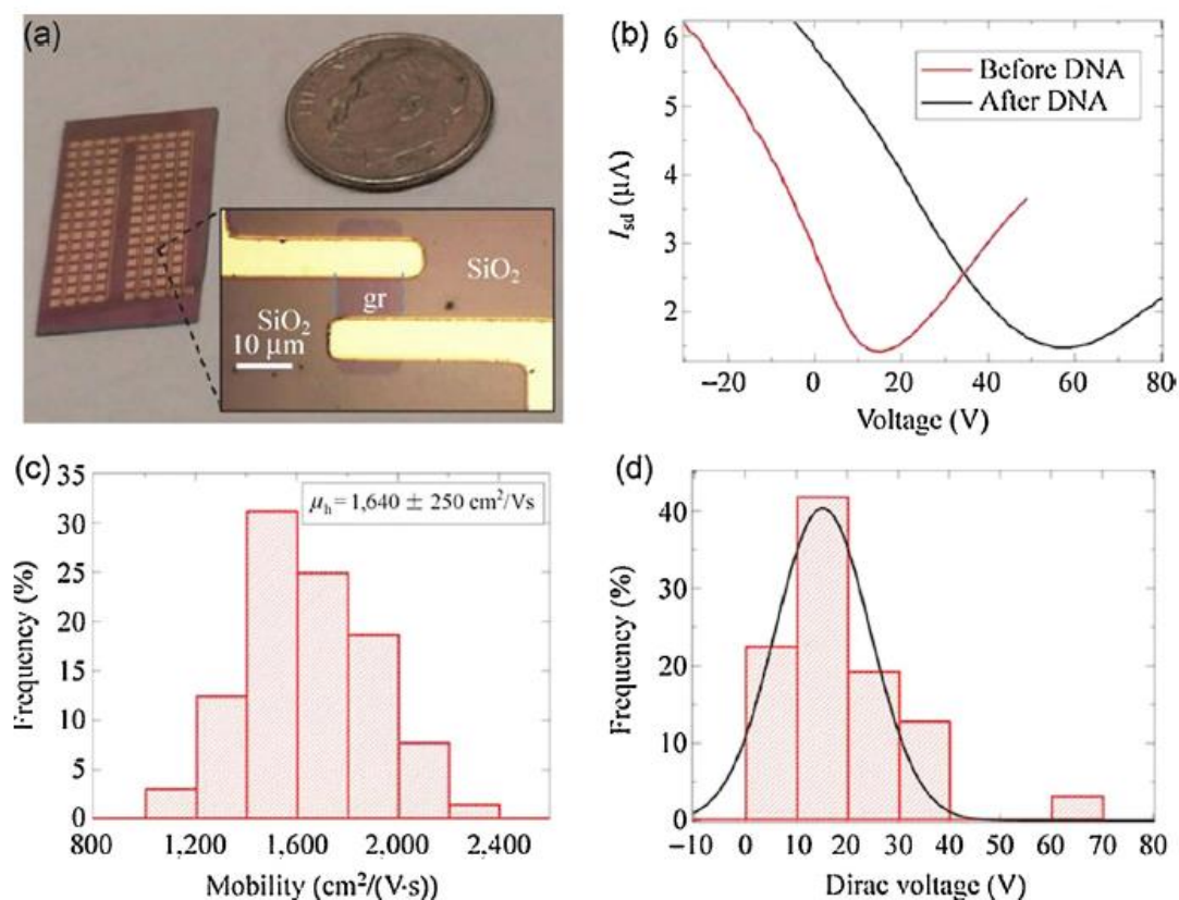
Figure 30 a) Dispositif expérimental contenant 112 transistors de taille 10µm x 15µm. a) réponse d'un transistor avant et après le dépôt d'ADN, c) évolution de la mobilité des différents transistors du réseau, d) position relative du point de Dirac. [70]
