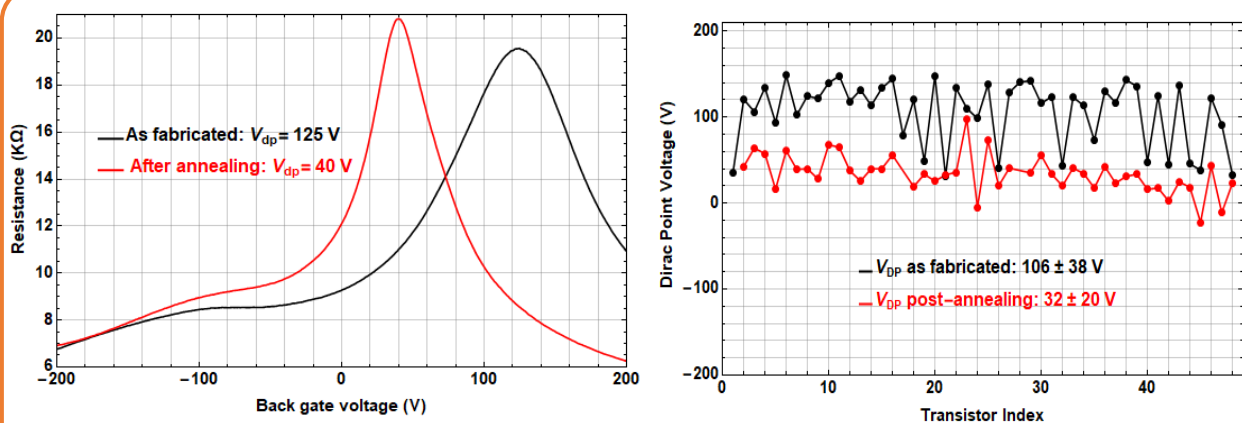
Figure 52. Mesure avant (en noir) et après le recuit (en rouge) d'un transistor individuel à gauche et de l'ensemble du réseau à droite.
