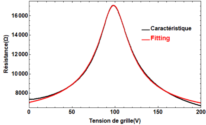
Figure 49 Extraction de la mobilité. En noir la mesure expérimentale et en rouge l'ajustement théorique.
