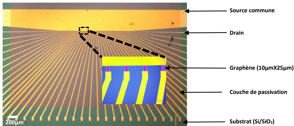
Figure 44. Photographie d'une puce après passivation. On voit les 48 drains individuels et la source commune qui connectent les canaux du graphène
