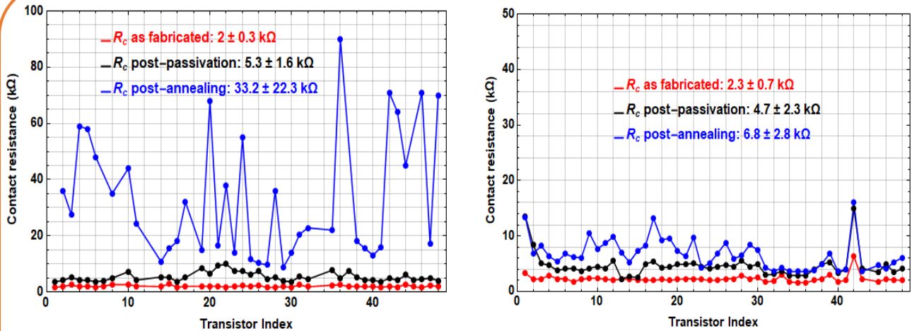
Figure 53. Etude comparative des contacts en Cr/Au à gauche et Ti/Au à droite. On peut remarquer que la valeur de la résistance de contact est 16 fois plus grande après le recuit quand on utilise les électrodes en Cr/Au avec une perte de 10% des transistors initialement qui marchaient alors qu'avec les électrodes en Ti/Au on assiste à une augmentation de l'ordre de 3 fois la valeur initiale des résistances de contact et tous les transistors marchent après le recuit
