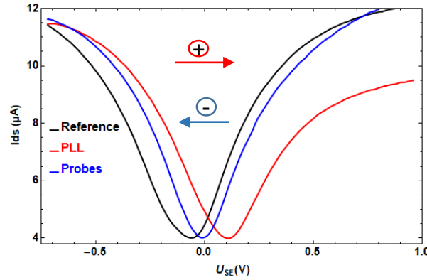
Figure 66. Réponse d'un transistor suite à l'adsorption de la PLL (rouge) et à la fixation de des sondes (bleu)
