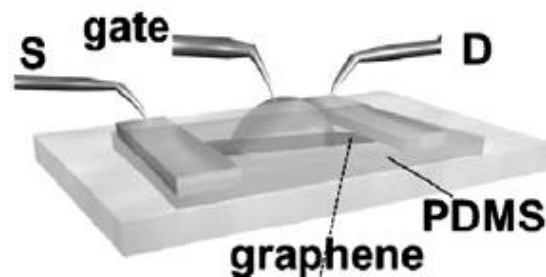
Figure 31. Vue d'artiste d'un transistor à effet de champ à base de graphène à grille liquide [73]
