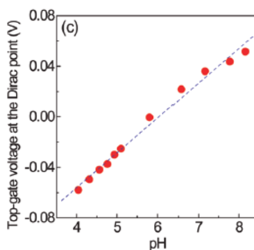
Figure 29 a) Variation de la conductance suite à l'augmentation de la concentration de protéine, c) dépendance linéaire de la tension au point de Dirac en fonction du pH de l'électrolyte. Source [65]
