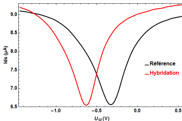
Figure 77. Détection de l'hybridation des produits THRCA, le signal détecté est beaucoup plus prononcé que ce qu'on a l'habitude de voir avec les oligonucléotides
