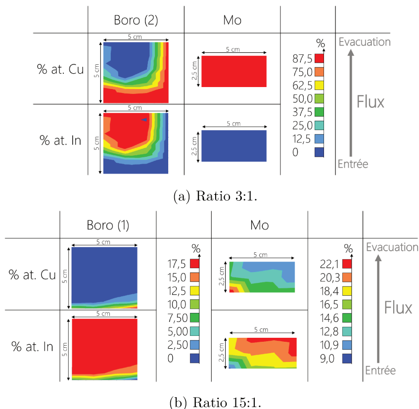
FIGURE 4.23 – Cartographies XRF obtenues en analysant les films déposés sur les substrats de verre boro (1-3) et Mo (4). Dépôt réalisé avec le programme du CIS, à T_{dep} = 160 °C, pour trois ratios [\text{In}_2\text{S}_3]:[\text{Cu}_x\text{S}] . Comparer avec Figure 4.17.
