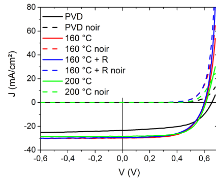
(b) Courbes J(V) pour 10 nm d' \text{In}_2\text{S}_3 .
