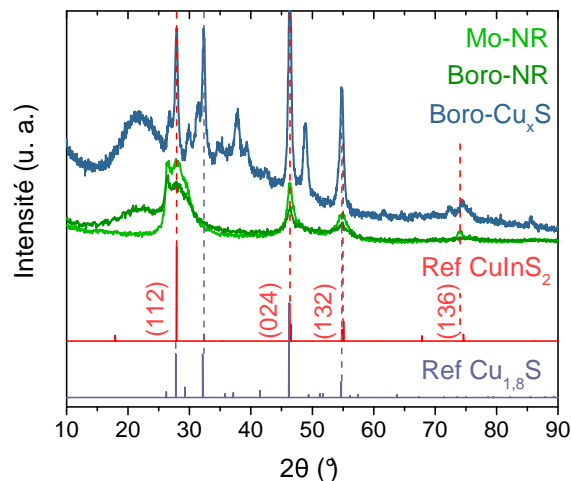
FIGURE 4.47 – Diffractogrammes GIXRD du film CIS non-recuit (NR) déposé sur substrat boro et Mo, ainsi que d'un film de \text{Cu}_x\text{S} déposé sur substrat boro. Références : \text{CuInS}_2 (ICDD 00-047-1372) ; \text{Cu}_{1,8}\text{S} (ICDD 00-047-1748).
