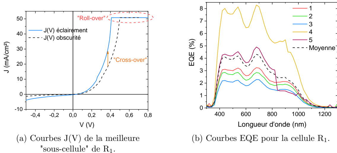
FIGURE 4.55 – Caractérisations de la cellule R_1 (a) Courbes J(V) sous éclairé et dans l'obscurité pour la "sous-cellule" la plus efficace; (b) Répétition d'une mesure d'EQE pour une même "sous-cellule" à différents instants.
