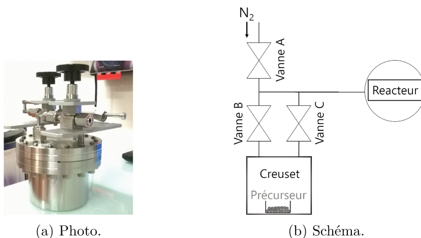
FIGURE 1.25 – Photo (a) et schéma (b) illustrant la source solide Beneq HS-300 reliée à la chambre de réaction et mettant en évidence la position des électrovannes.
