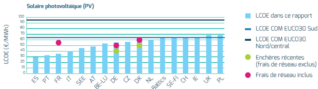
FIGURE 1.3 – Coûts actualisés de l'énergie (LCOE) du solaire PV par pays de l'Europe, estimés pour 2030, comparés aux hypothèses du scénario EUCO30 et aux résultats des derniers appels d'offres [17].
