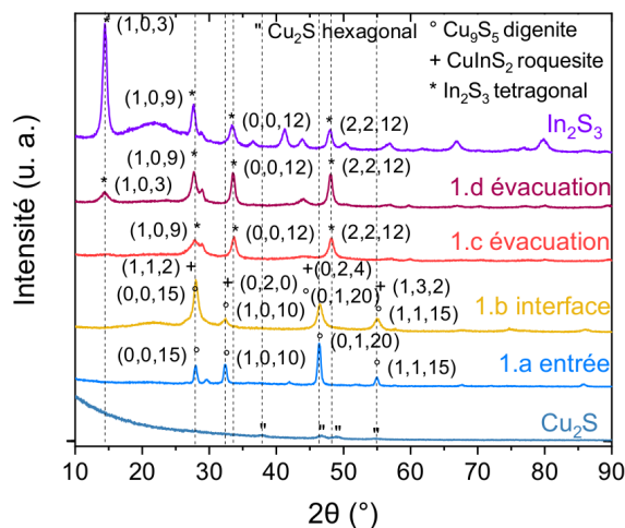
FIGURE 4.18 – Diffractogrammes GIXRD mesurés en différentes positions de la chambre du réacteur Beneq TFS-200. Comparaison avec les diffractogrammes GIXRD d'un film d' \text{In}_2\text{S}_3 (30 nm) et d'un film de \text{Cu}_x\text{S} (10 nm) synthétisés à T_{dep} = 160 °C dans le réacteur Beneq TFS-200.
