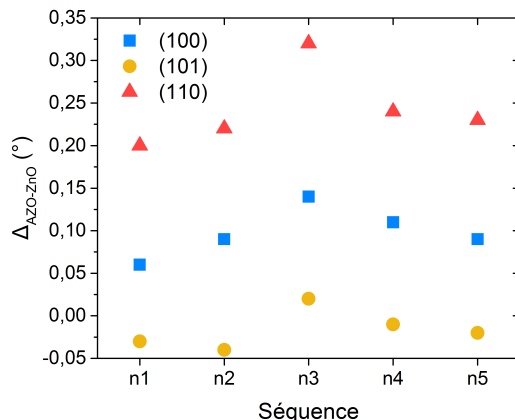
FIGURE 2.22 – Positions des pics de diffraction des films de ZnO:Al ( 2\theta en ^\circ ) pour les trois plans principaux (100), (101) et (110) et comparaison avec l'i:ZnO (ICDD 00-036-1451).
