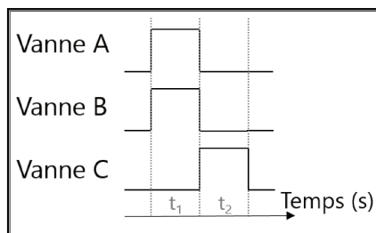
FIGURE 3.3 – Schéma illustrant le fonctionnement du mode de transport "booster" utilisé lors du pulse de l' \text{In}(\text{acac})_3 . Les temps t_1 et t_2 ont été variés et peuvent différer. La position des vannes par rapport à la source et au réacteur est indiquée sur la Figure 1.25b.
