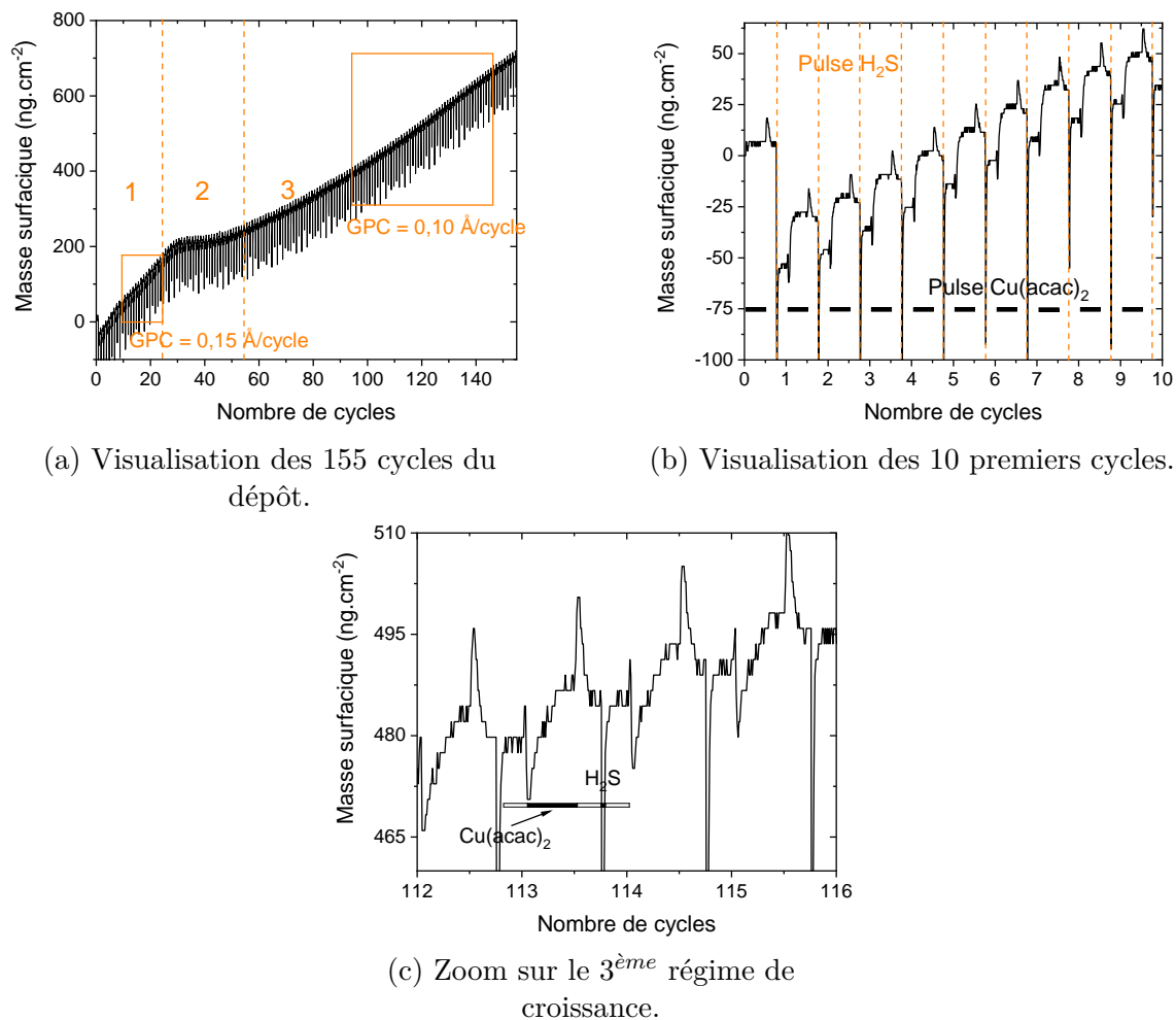
FIGURE 4.42 – Mécanismes de croissance du \text{Cu}_x\text{S} sur un substrat d' \text{In}_2\text{S}_3 d'épaisseur 115 \text{ \AA} , visualisation (a) de 155 cycles; (b) des 10 premiers cycles; (c) zoom sur le 3 ème régime de croissance. Programme [\text{Cu}(\text{acac})_2]/\text{N}_2/\text{H}_2\text{S}/\text{N}_2 = [0,5/0,2/0,5/10/0,5]/5/0,5/5 \text{ s} et T_{\text{réacteur}} = 160 \text{ }^\circ\text{C} .
