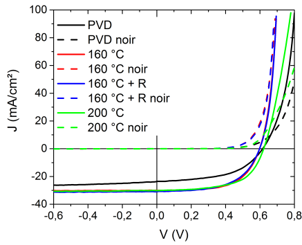
(a) Courbes J(V) pour 5 nm d' \text{In}_2\text{S}_3 .
