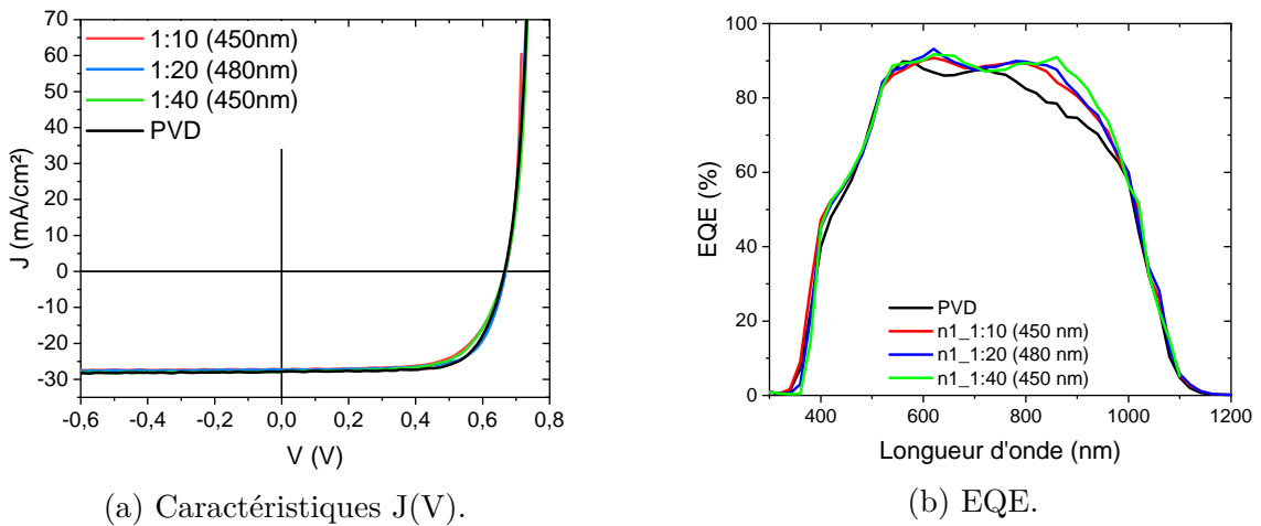
FIGURE 2.32 – (a) Courbes J(V) sous éclaircissement et (b) EQE des meilleures cellules des échantillons. L'empilement de la couche fenêtre i:ZnO/ZnO:Al est déposée par ALD (courbes rouge, verte et bleue) ou par PVD (pulvérisation cathodique) (courbe noire).
