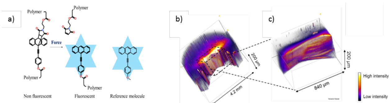
Figure 1. a) Schéma d'activation du mécanophore et molécule de référence. Reconstruction 3D de la pointe de fissure à faible b) et plus fort grossissement c) (le signal fluorescent correspond à l'endommagement moléculaire).
